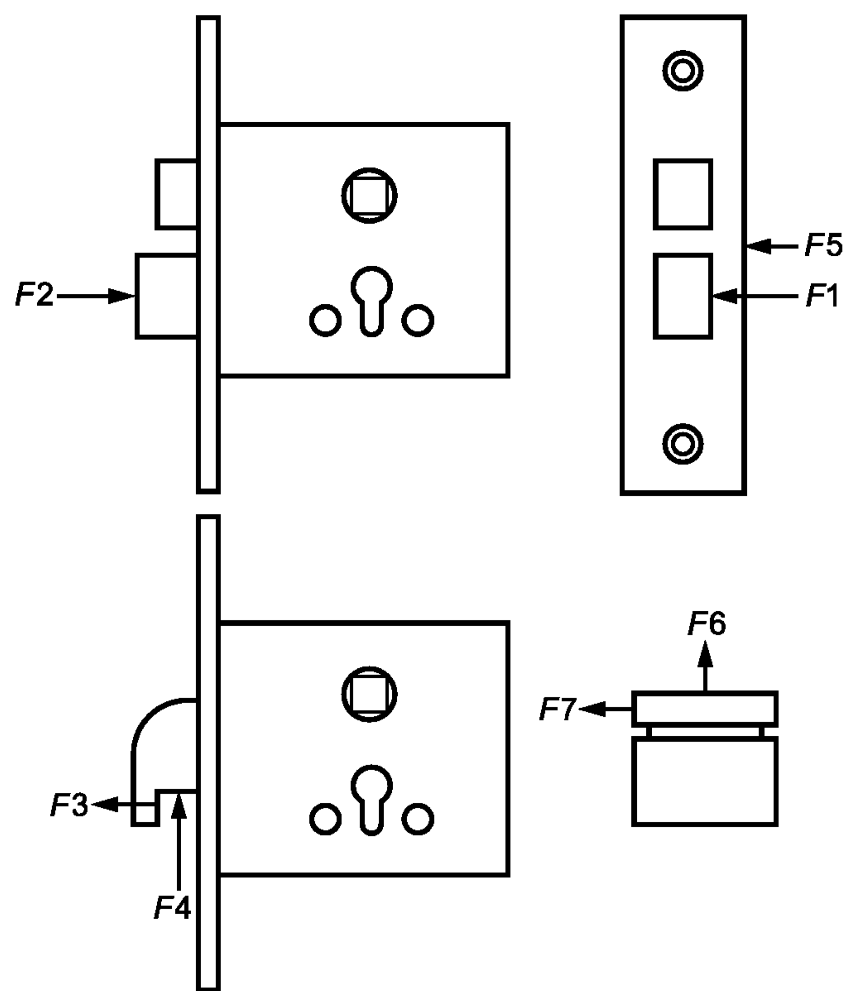
Рисунок 1 — Точки приложения сил, воздействующих на механизм замка
