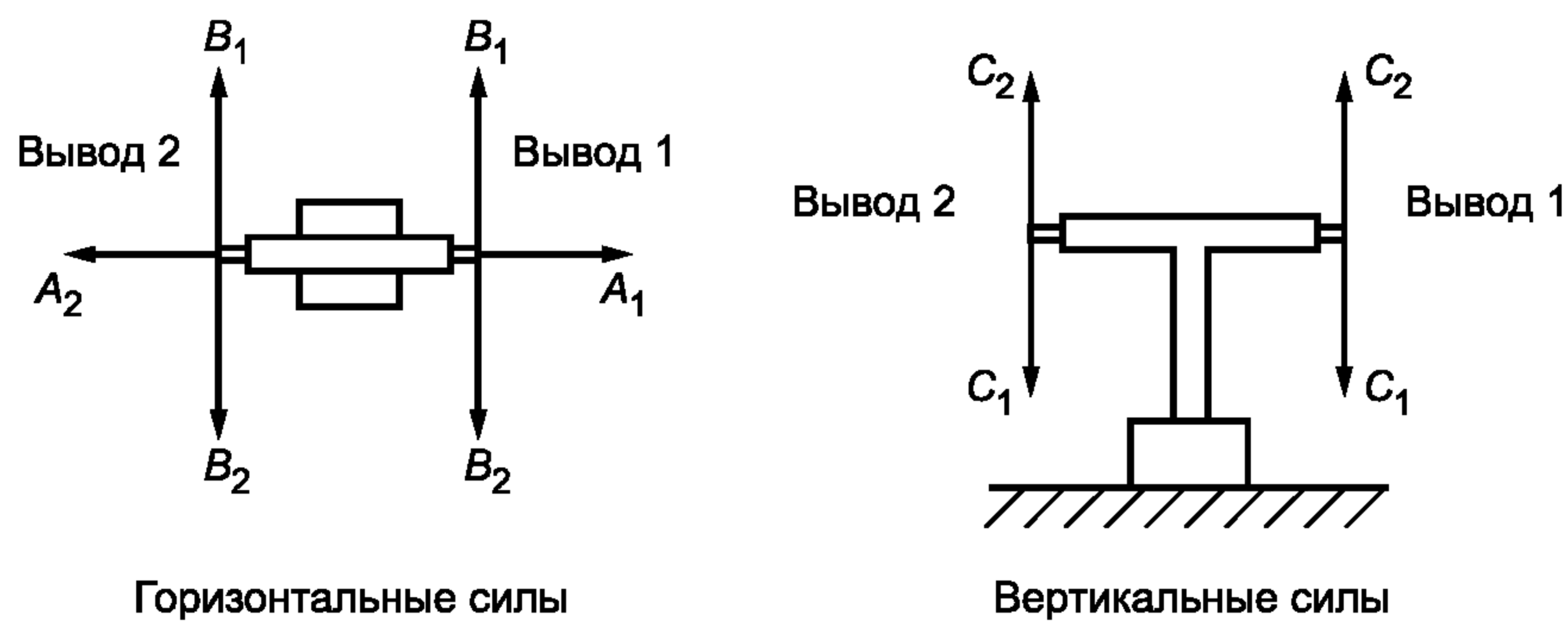
а) Статические нагрузки на выключатель
