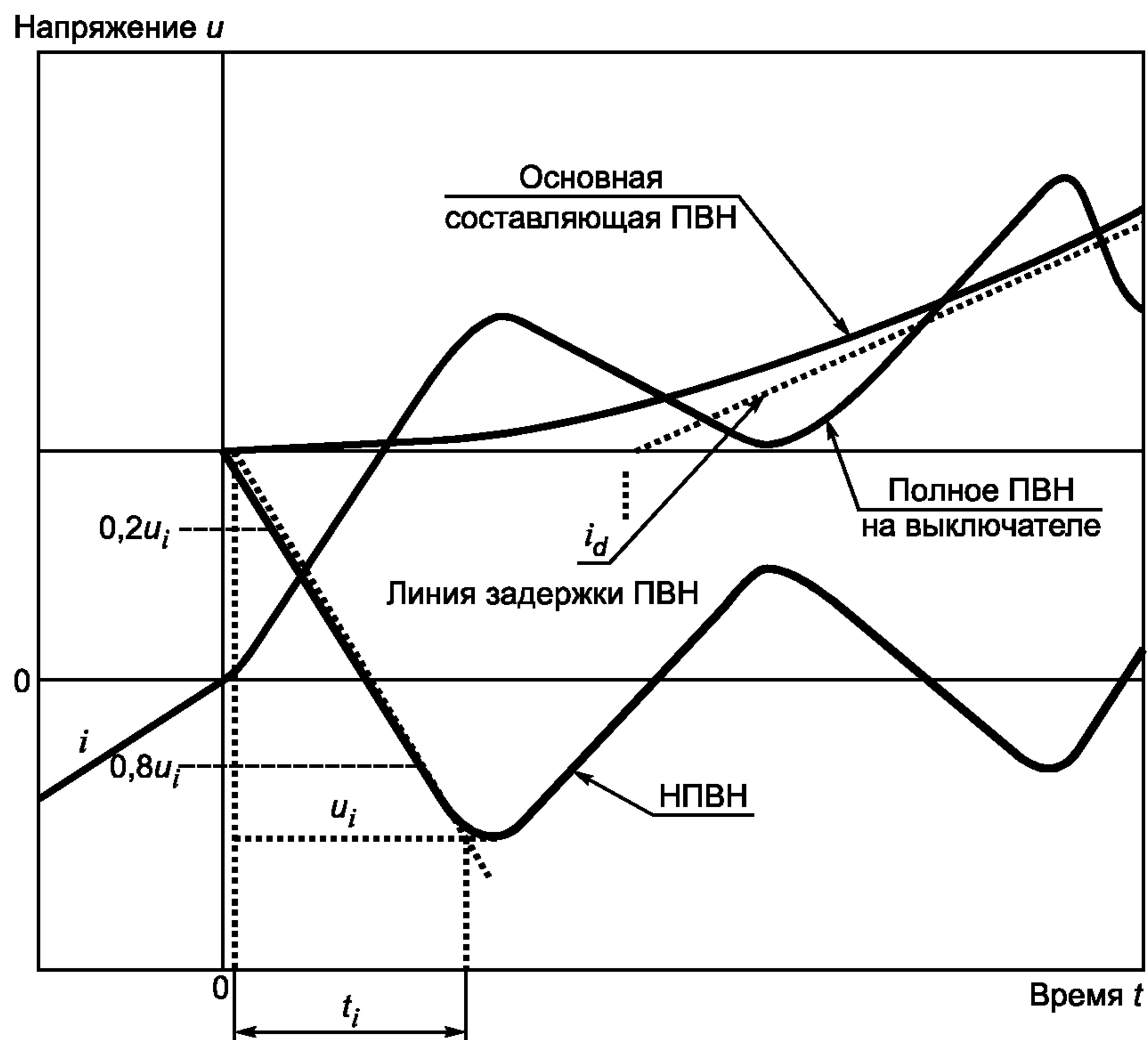
Рисунок 6 — Начальная часть переходного восстанавливающегося напряжения (НПВН)
