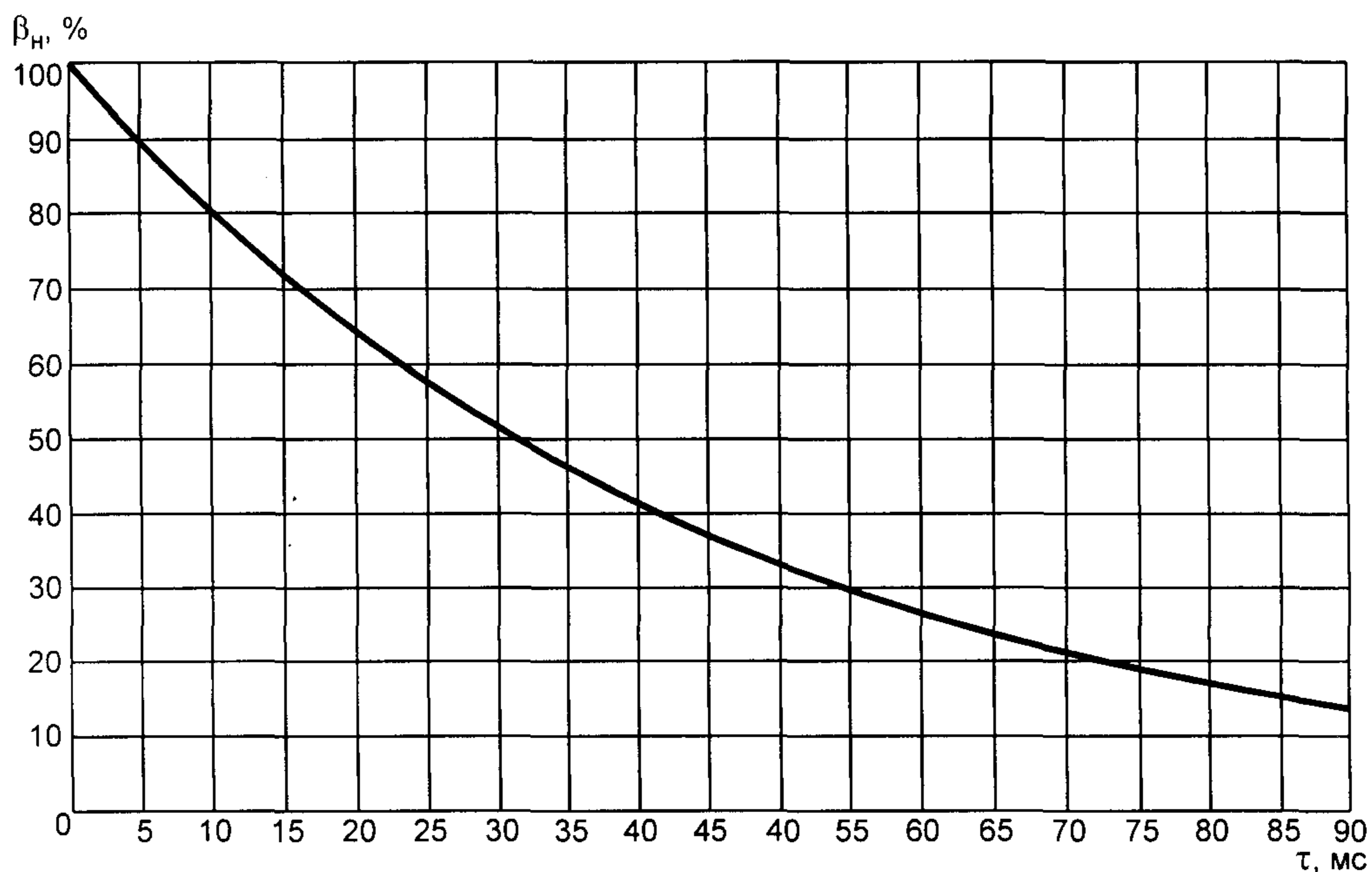
Рисунок 3 — Содержание аperiodической составляющей в процентах
