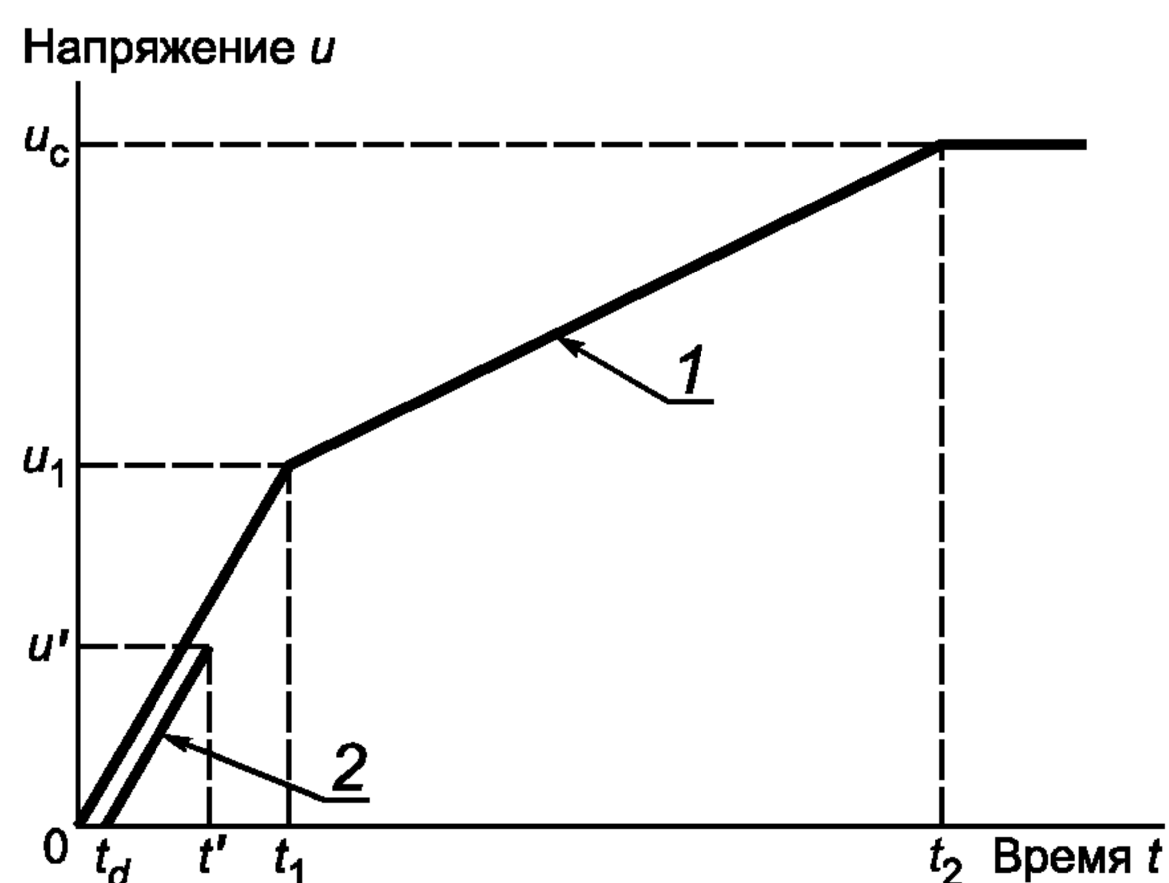
Рисунок 5 — Нормированные характеристики ПВН, определяемого четырьмя параметрами
