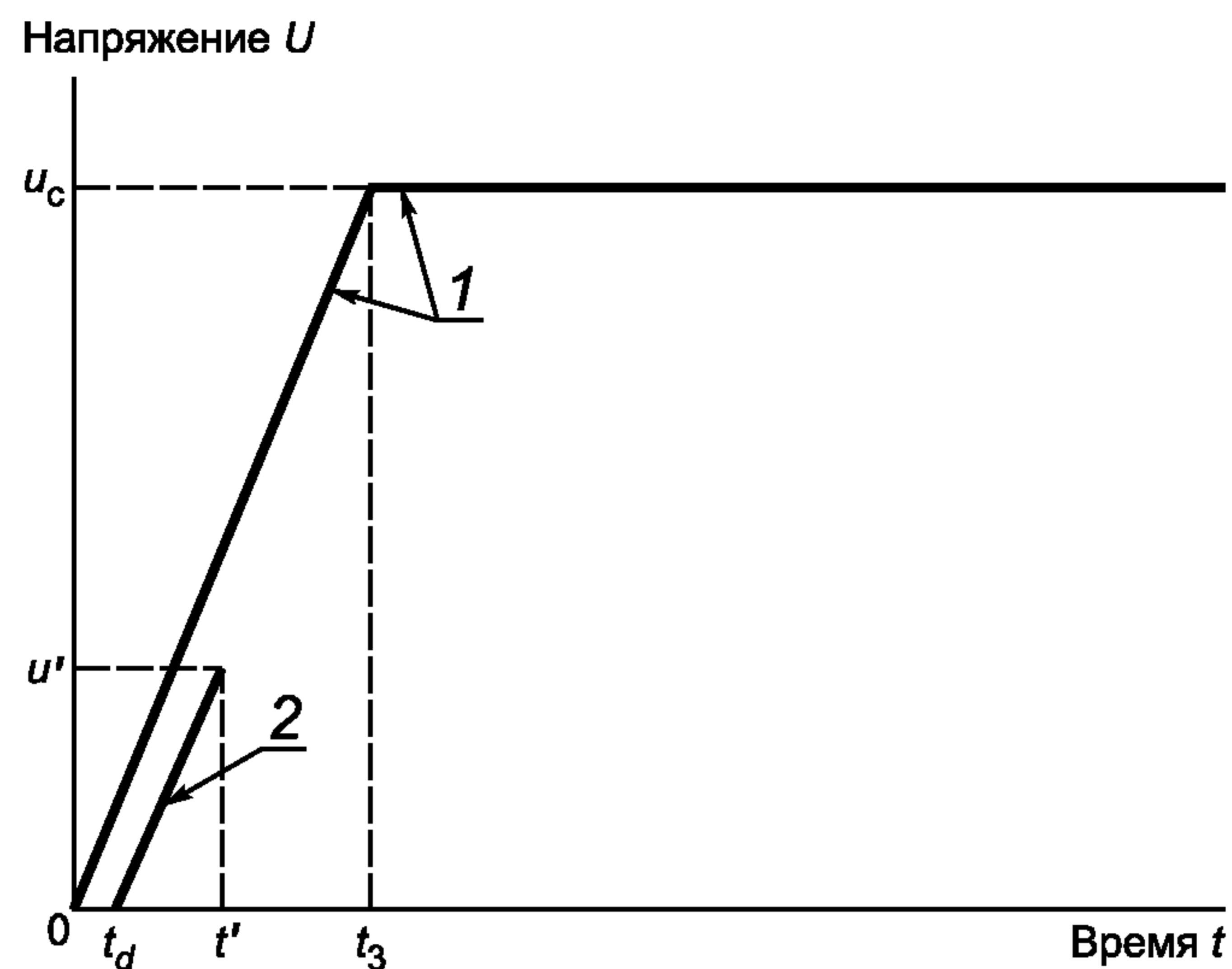
Рисунок 4 — Нормированные характеристики ПВН, определяемого двумя параметрами
