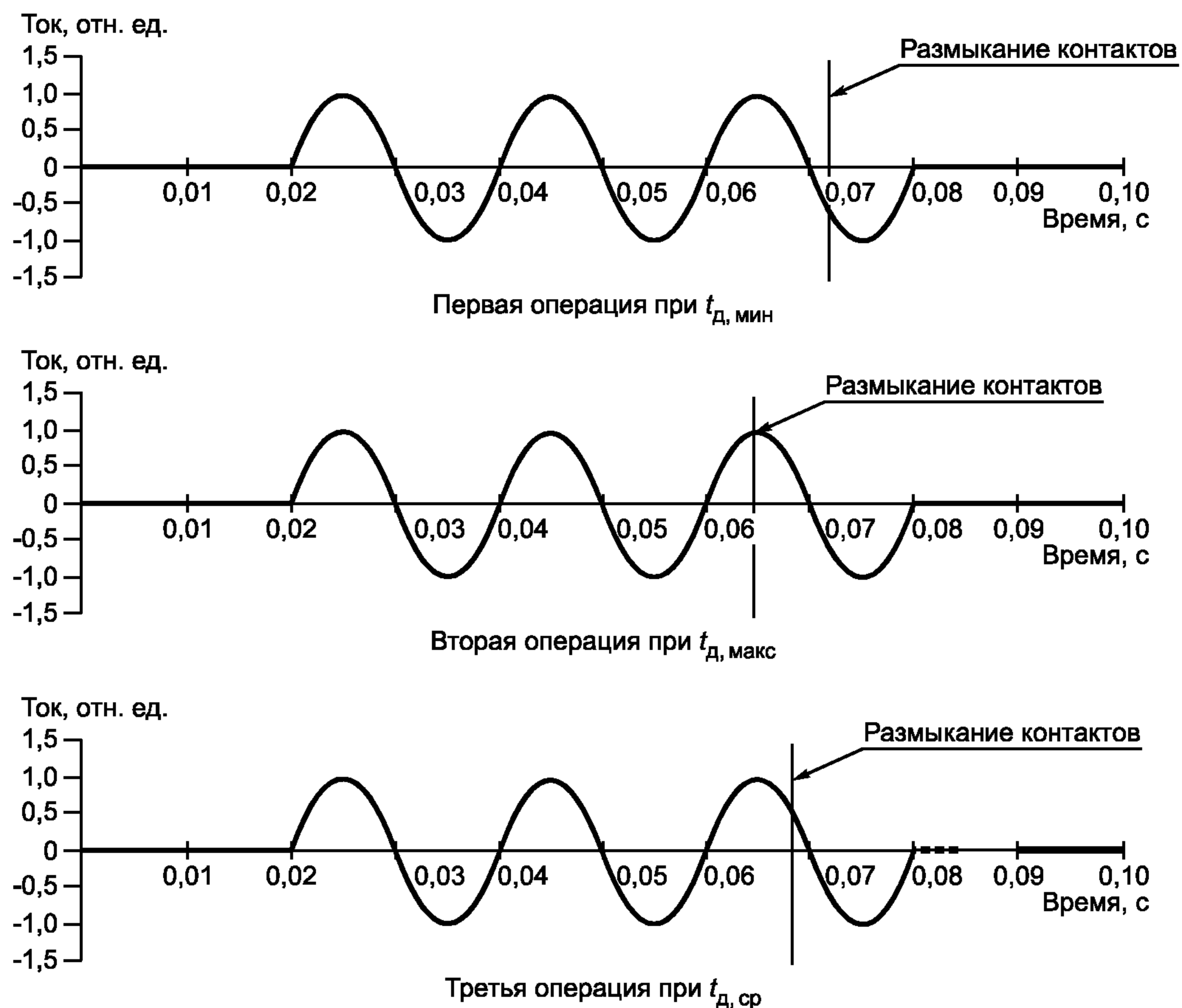
Рисунок 11 — Регулирование момента размыкания контактов относительно фазы тока при однополюсном отключении симметричного тока в режимах Т10, Т30, Т60, Т100с, Тсг1, Тсг2, Тсг3 выключателями с U_{ном} \leq 35 кВ
