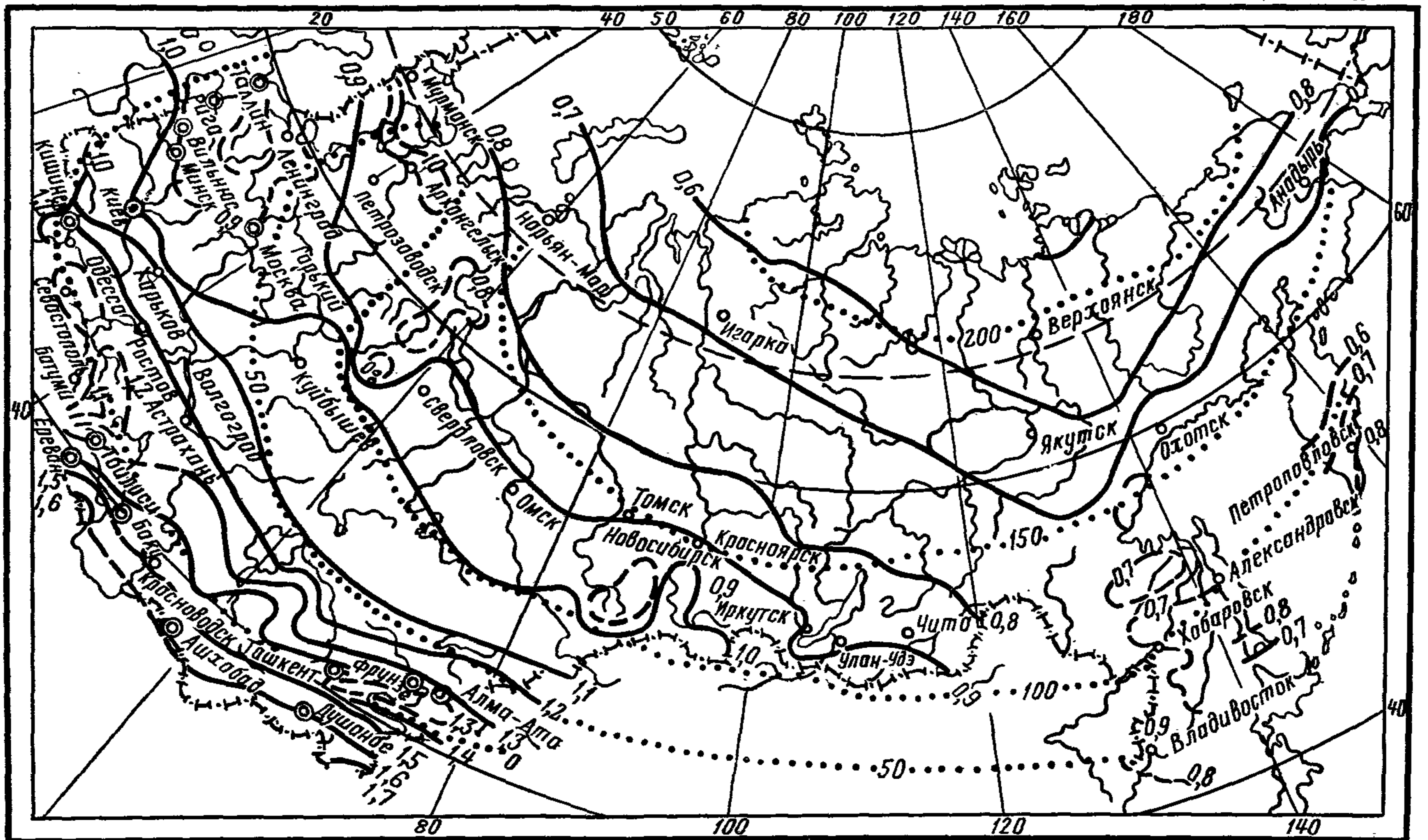
Рис. 5. Климатические коэффициенты для определения величины нагрузки на иловые площадки (сплошные и пунктирные линии) и продолжительности периода намораживания на иловых площадках в днях (точечные линии)
