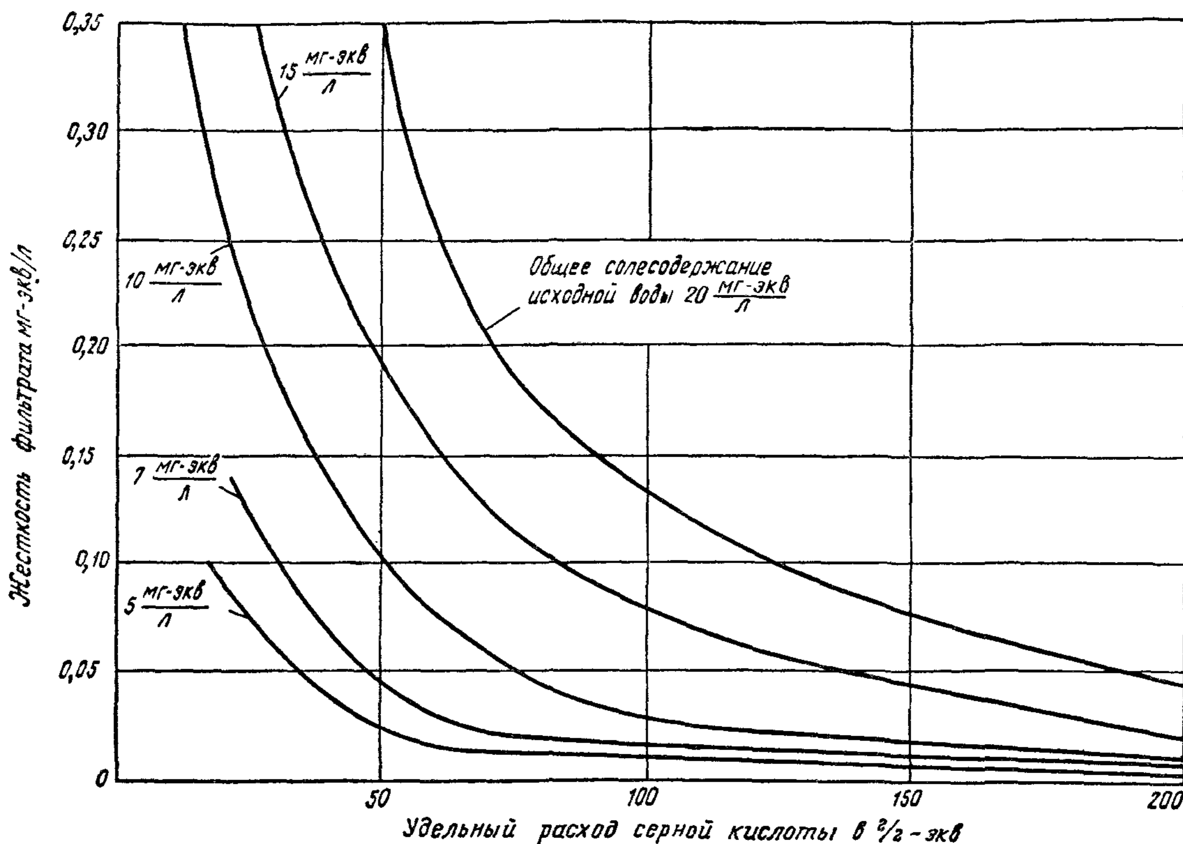
Рис. 7. График для определения жесткости воды, умягченной водород-катионированием
