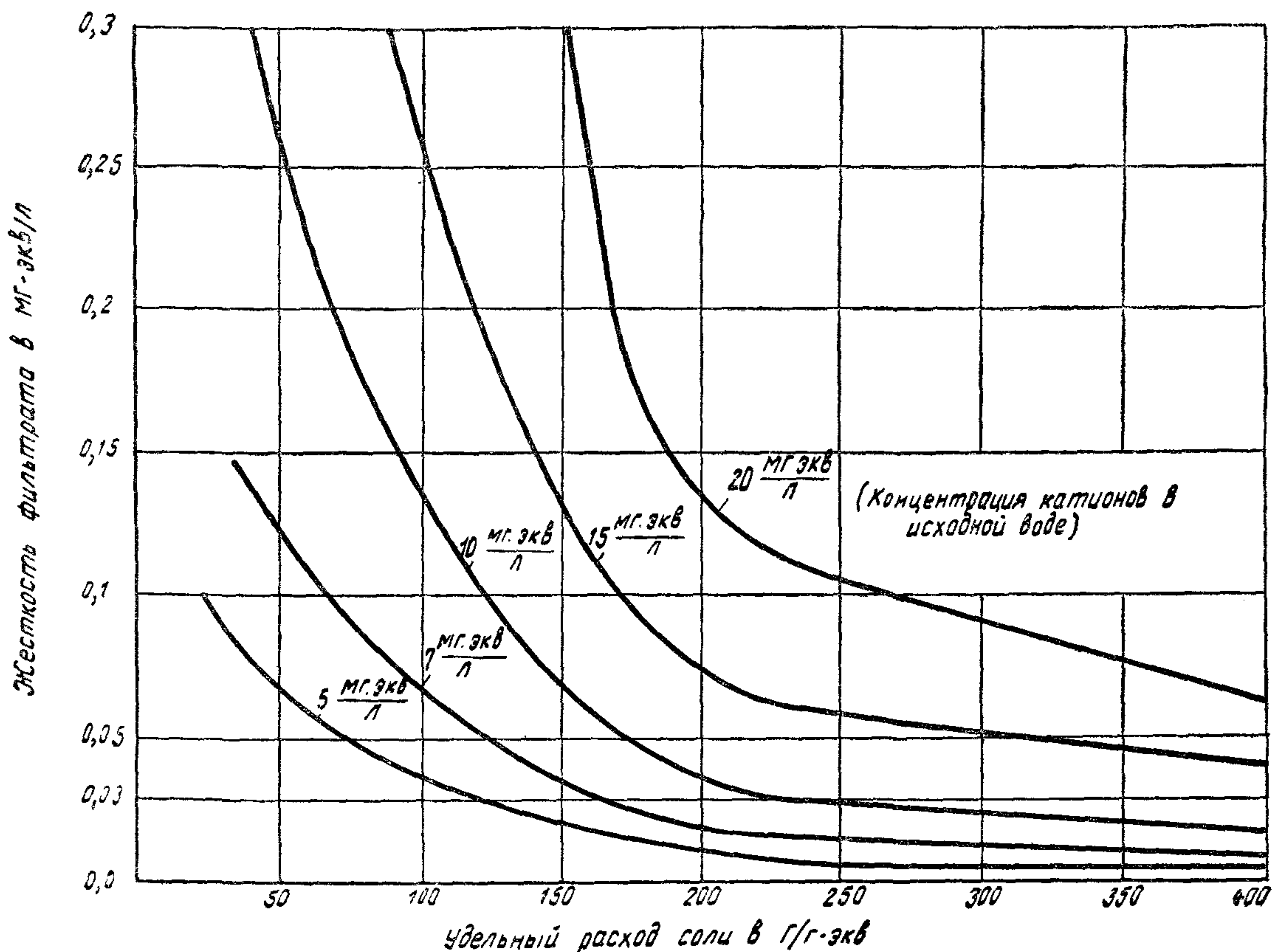
Рис. 6. График для определения жесткости воды, умягченной натрий-катионированием
