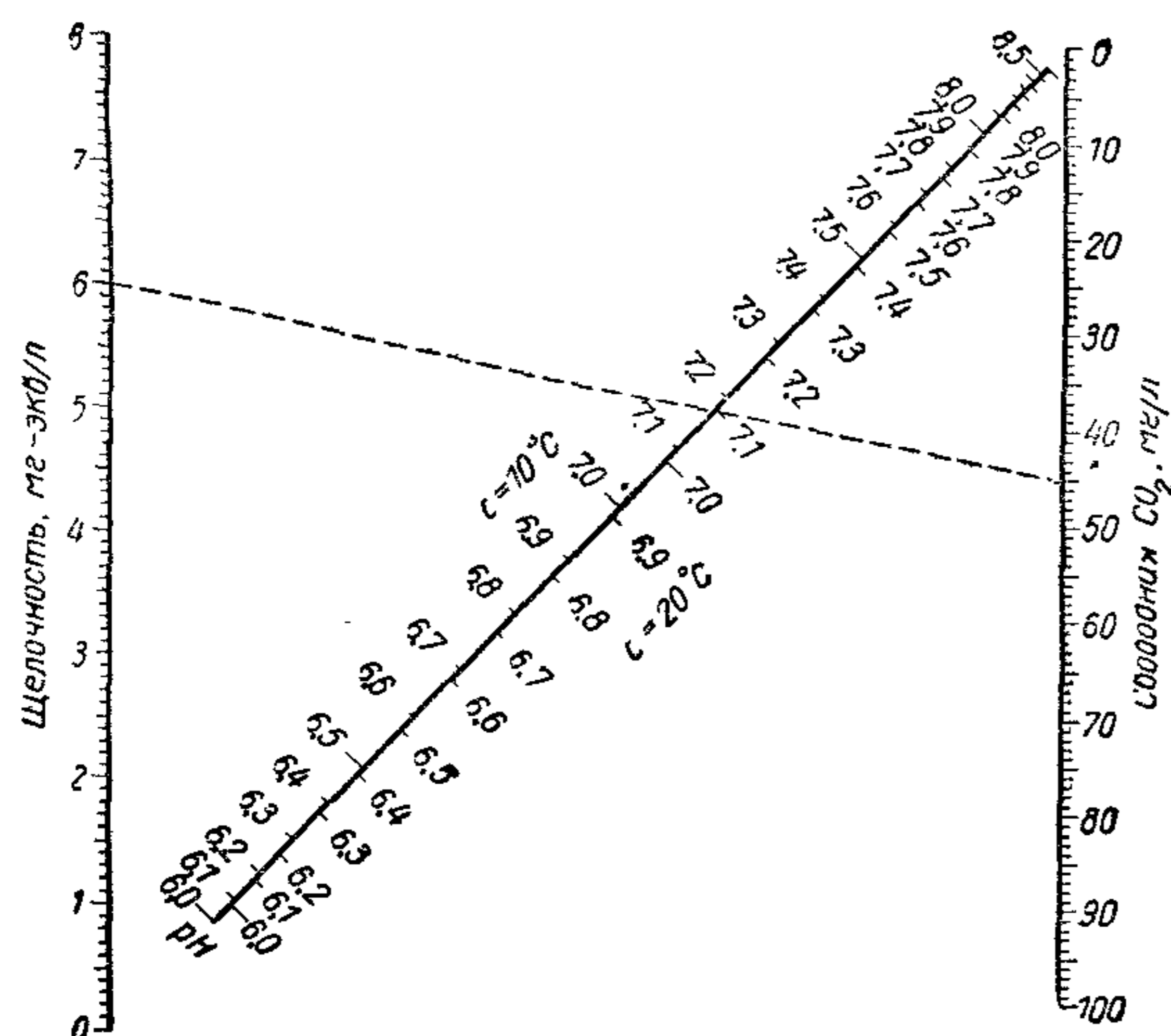
Рис. 2. График для определения рН коагулированной воды
