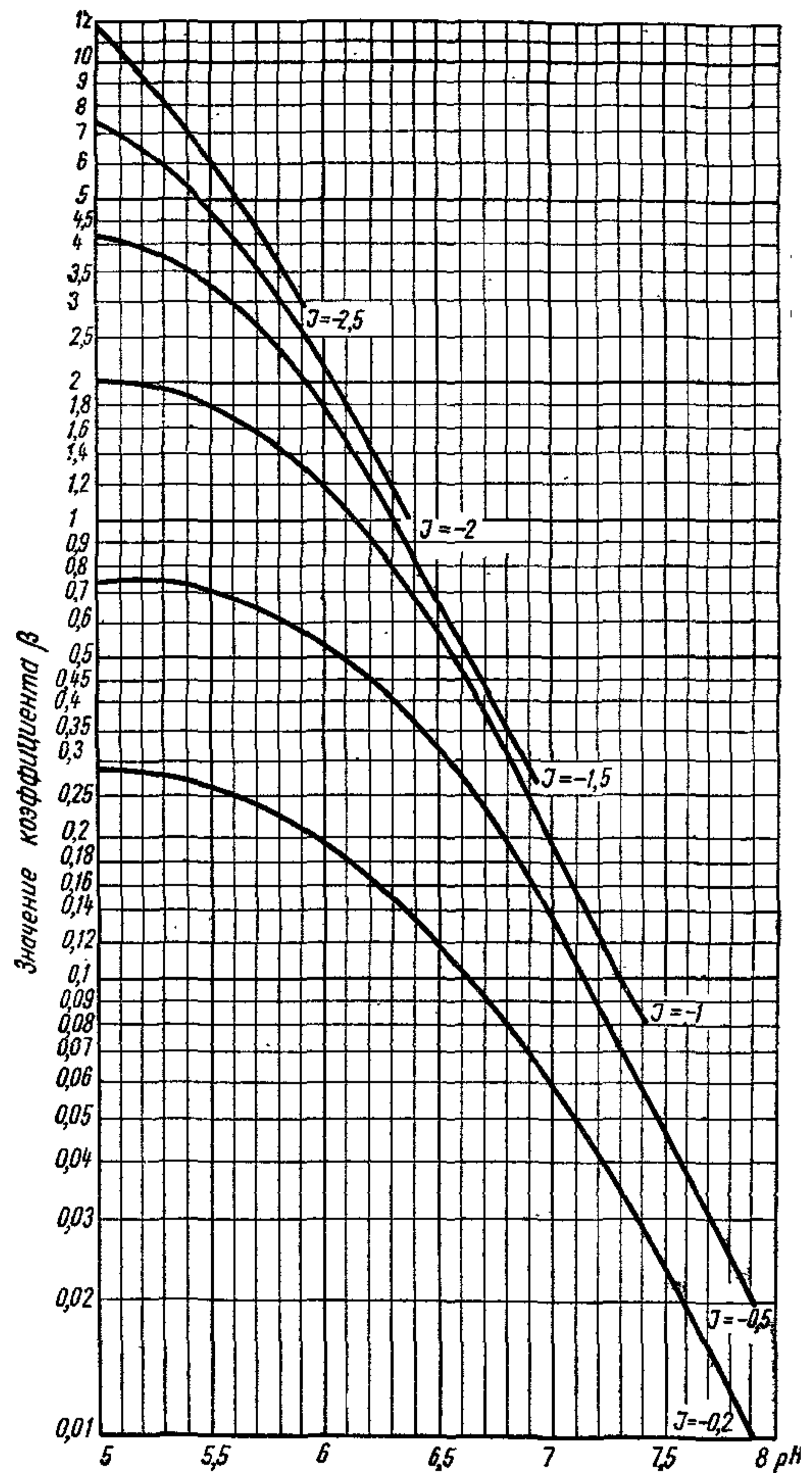
Рис. 4. График для определения коэффициента \beta при расчете дозы щелочи при \text{pH}_0 < \text{pH}_s < 8,4
