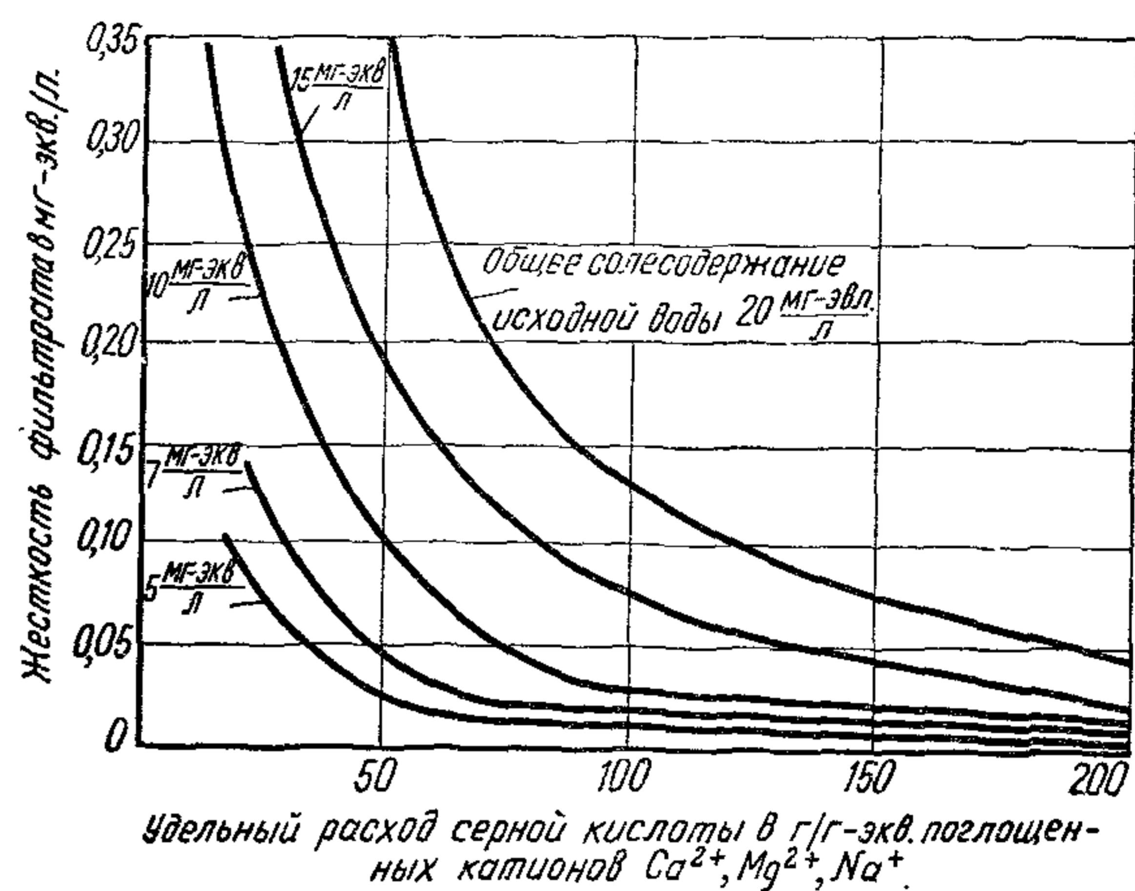
Рис. 7. График для определения жесткости воды, умягченной водород-катионированием
