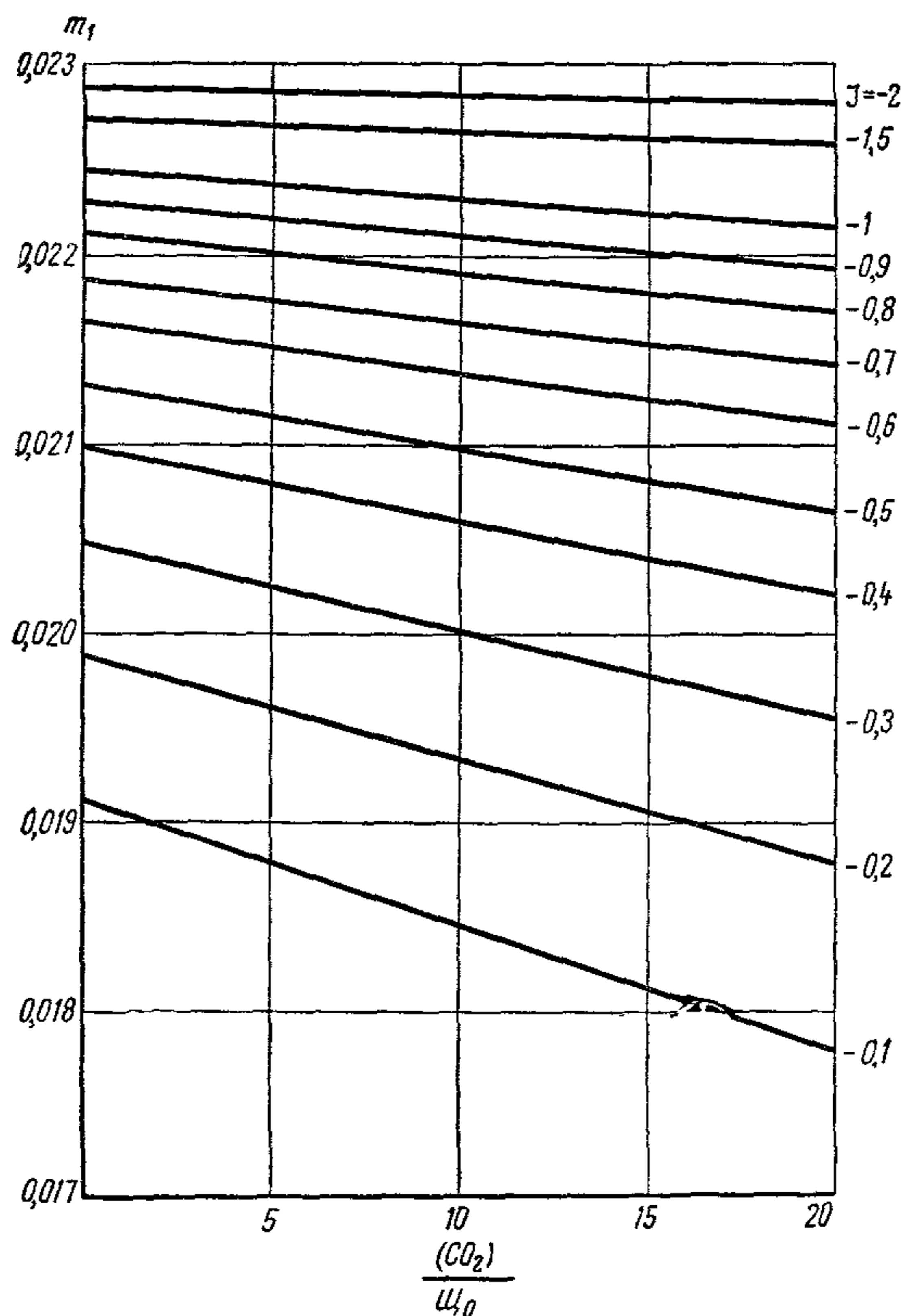
Рис. 8. График для определения коэффициента m_1
