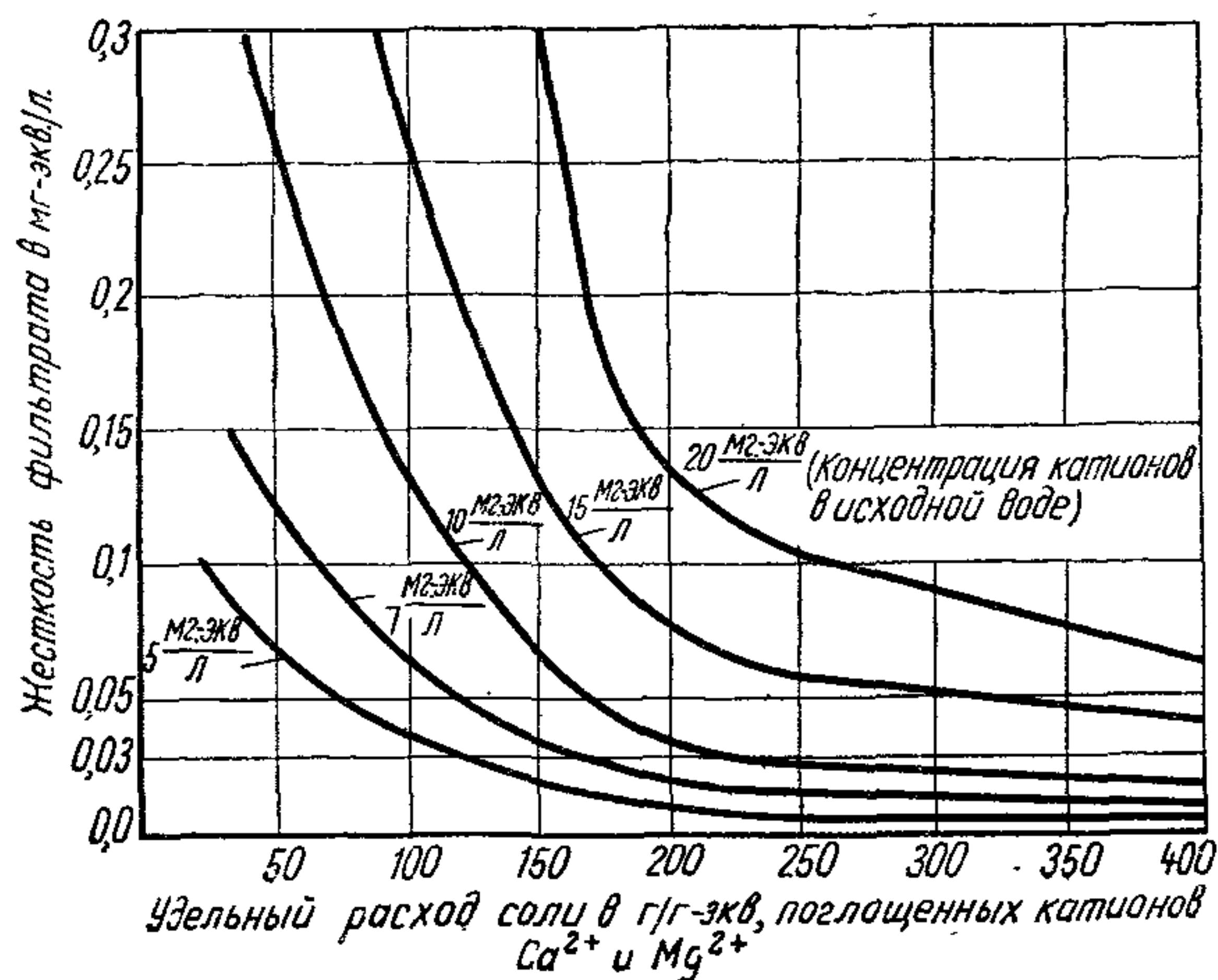
Рис. 6. График для определения жесткости воды, умягченной натрий-катионированием
