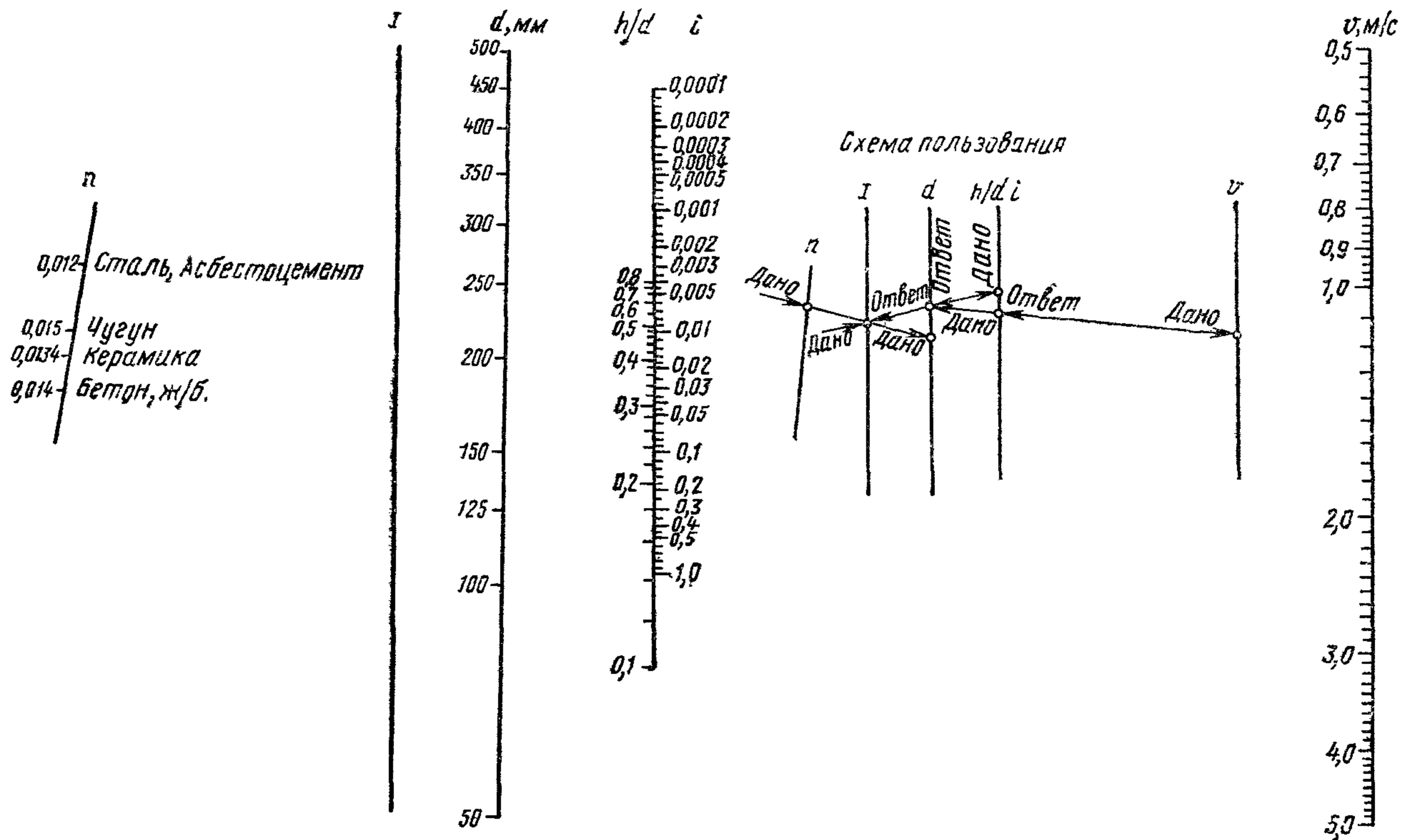
Рис. 1. Номограмма для определения гидравлического уклона канализационных трубопроводов
