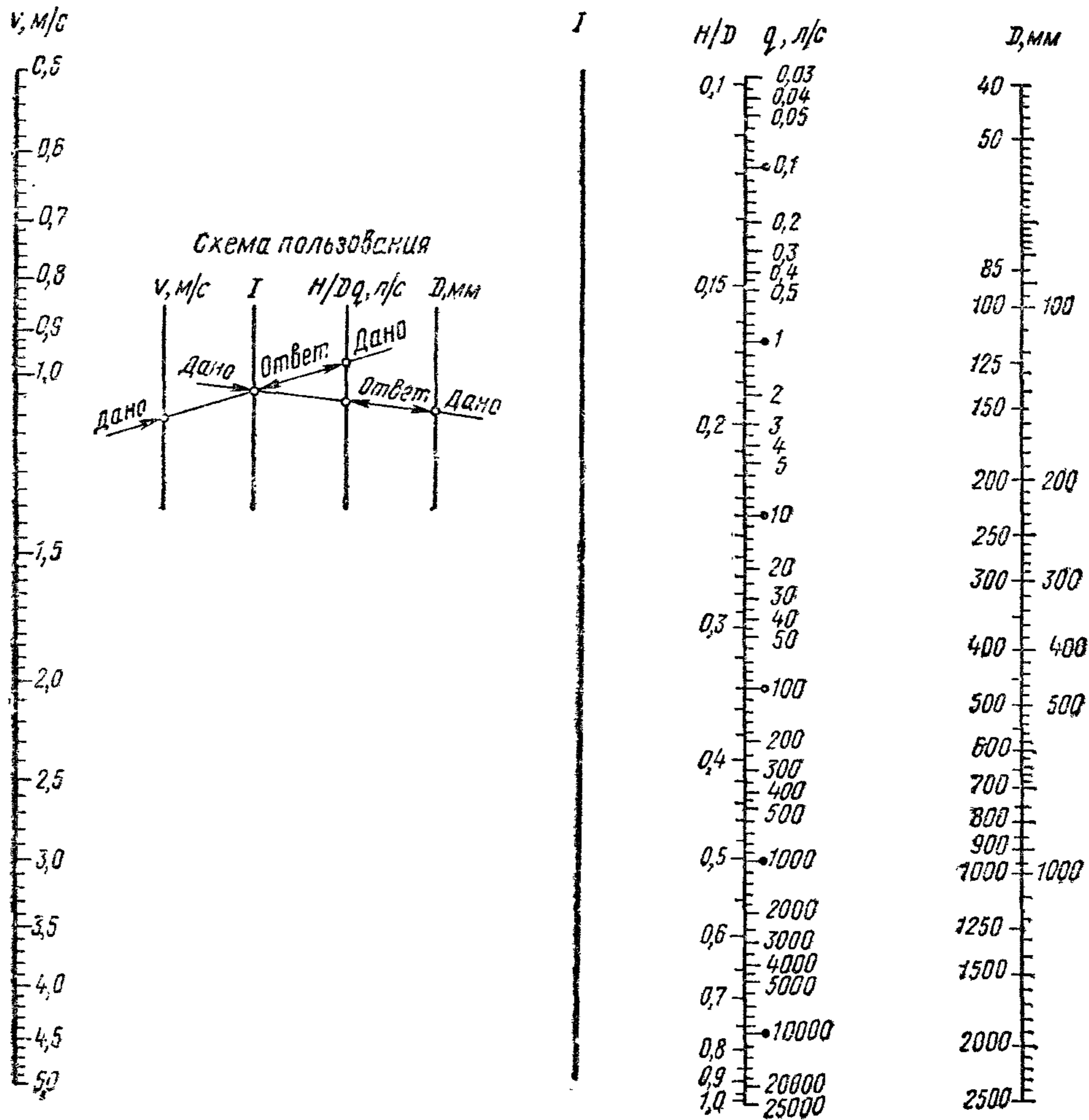
Рис. 2. Номограмма для определения диаметров канализационных трубопроводов
