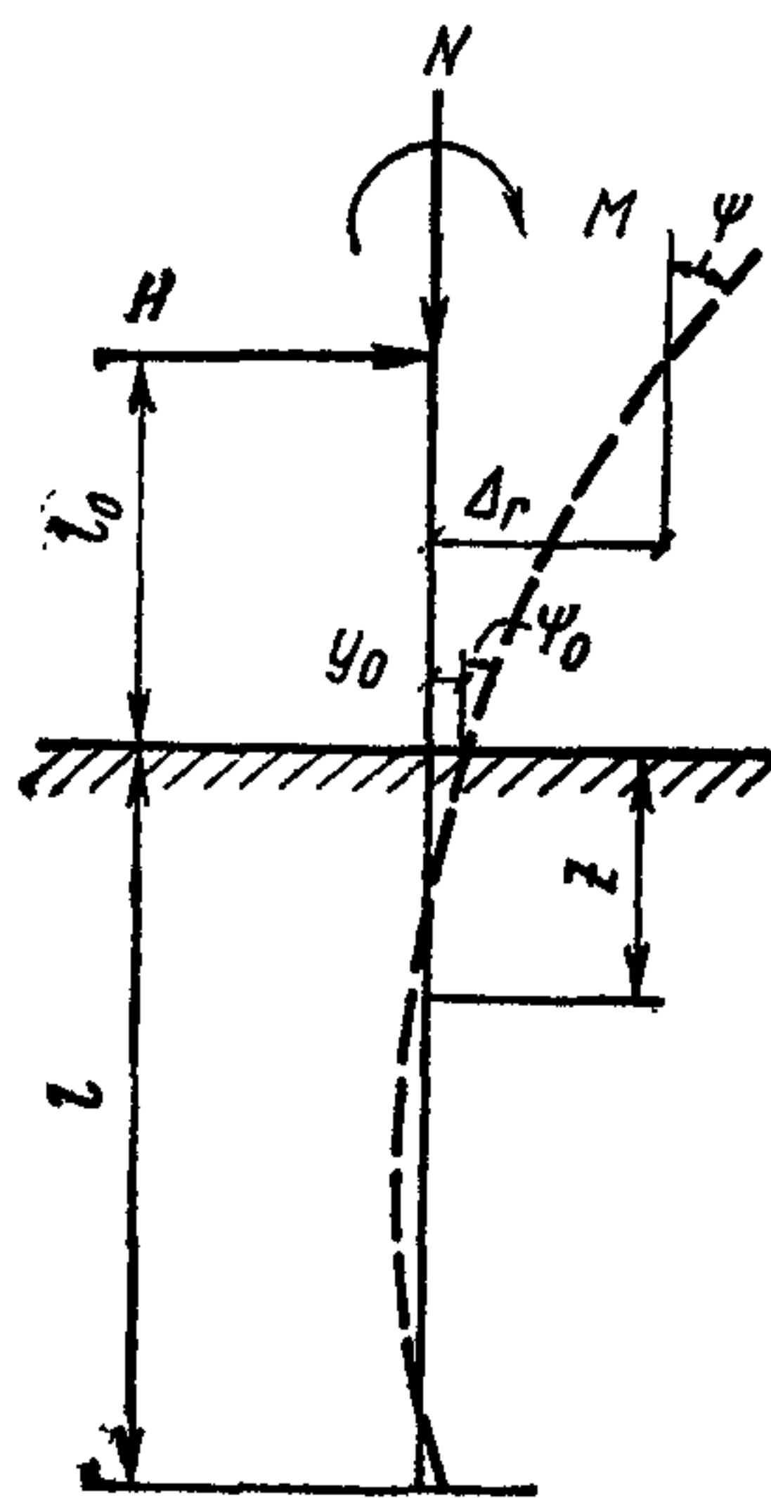
Рис. 1. Схема нагрузок на сваю
