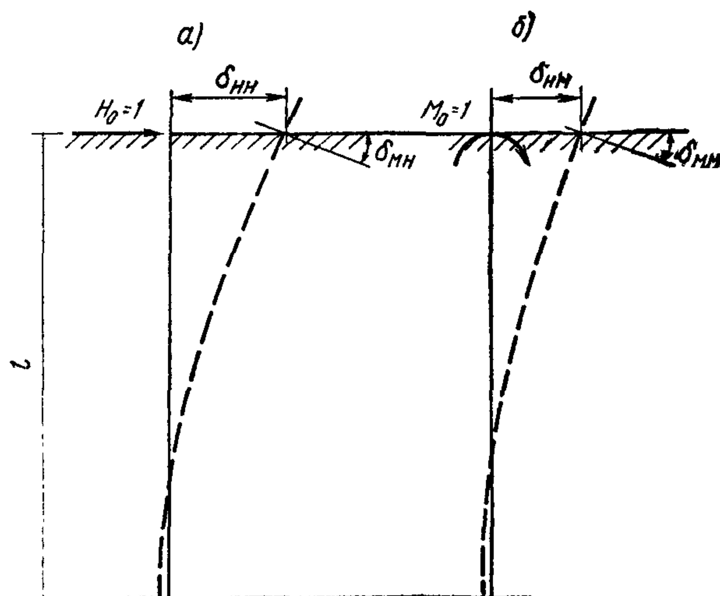
Рис. 2. Схема перемещений сваи в грунте а — от действия силы H_0=1 , приложенной в уровне поверхности грунта; б — от действия момента M_0=1
