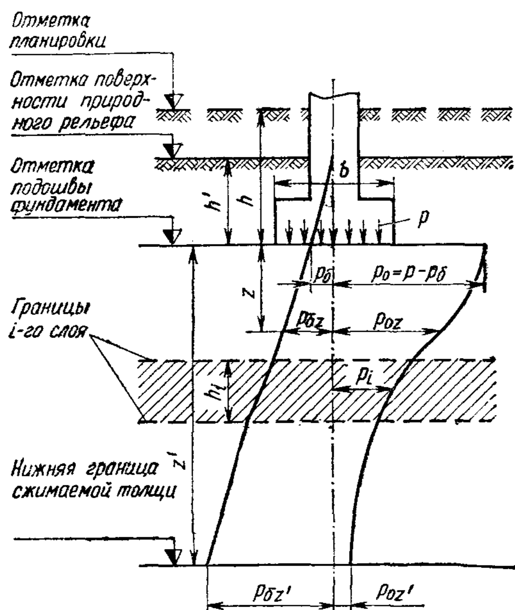
Рис. 1. Схема для расчета осадок методом послойного суммирования
