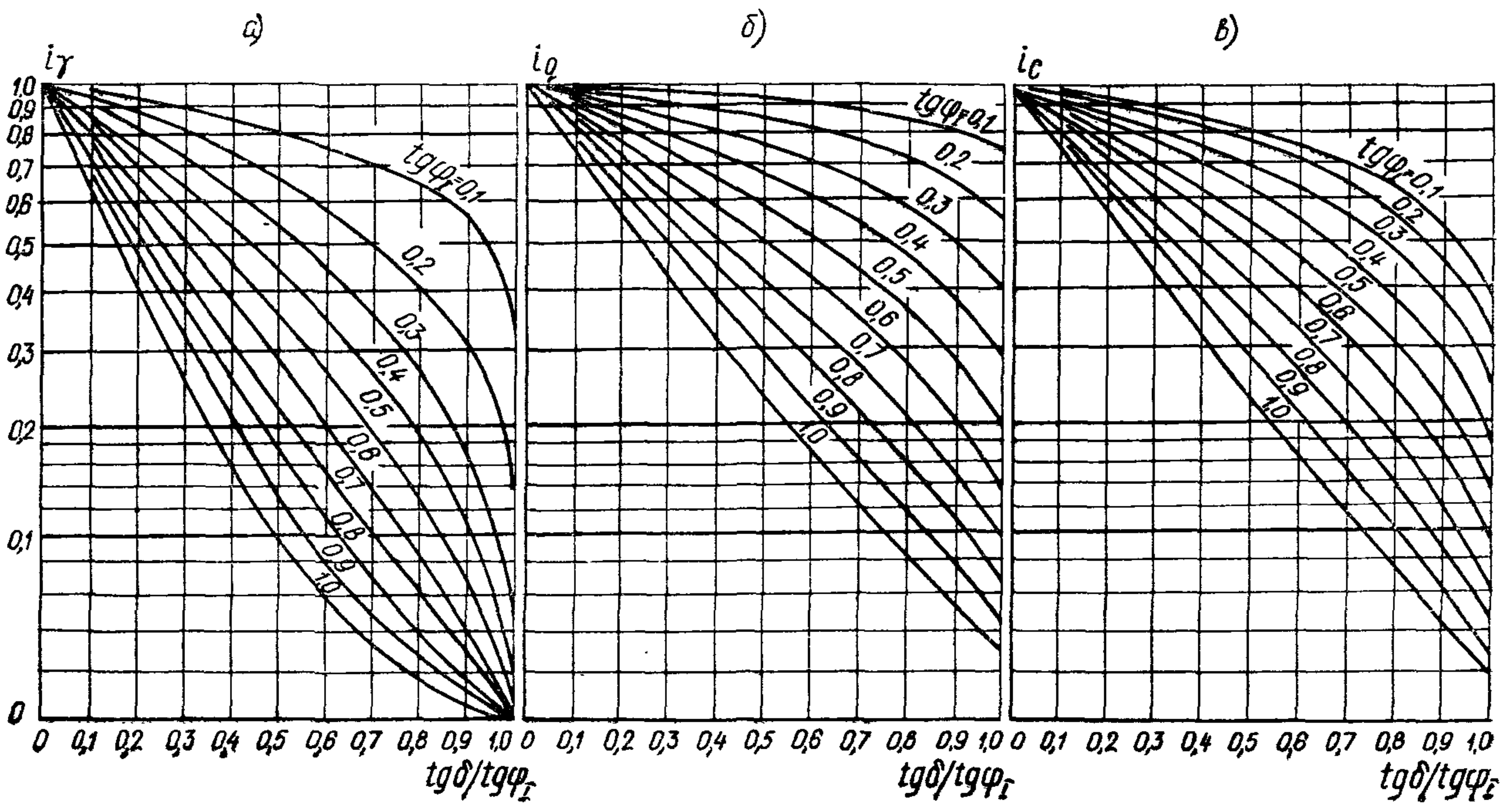
Рис. 2. Графики для определения коэффициентов наклона нагрузки
