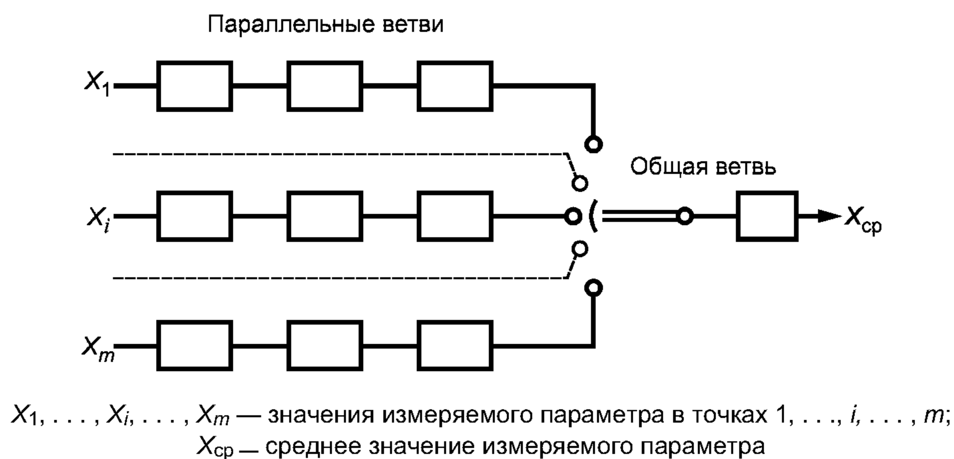
Рисунок Д.1
