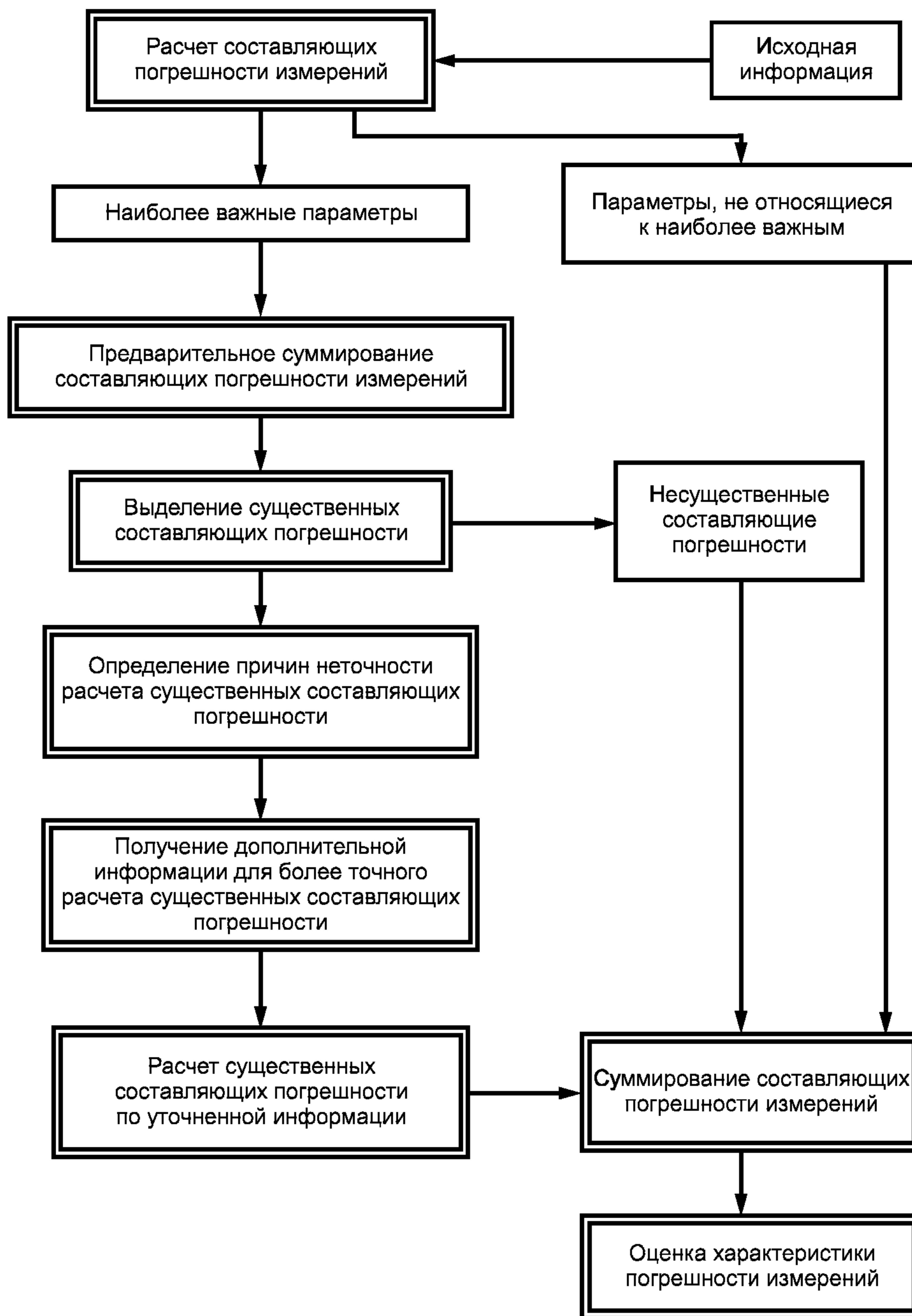
Рисунок 2 — Упрощенный алгоритм оценивания погрешности измерений
