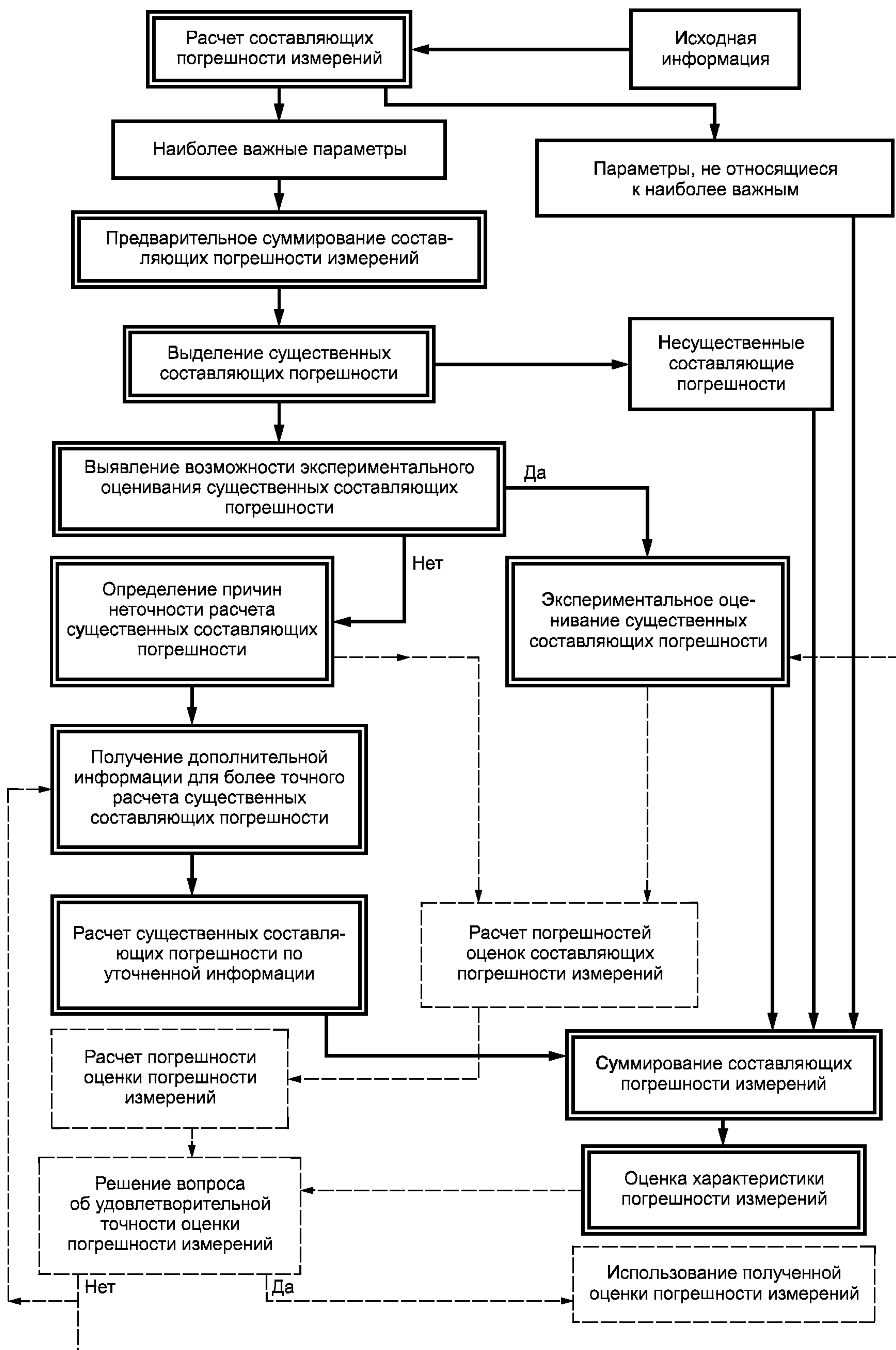
Рисунок 1 — Алгоритм оценивания погрешности измерений
