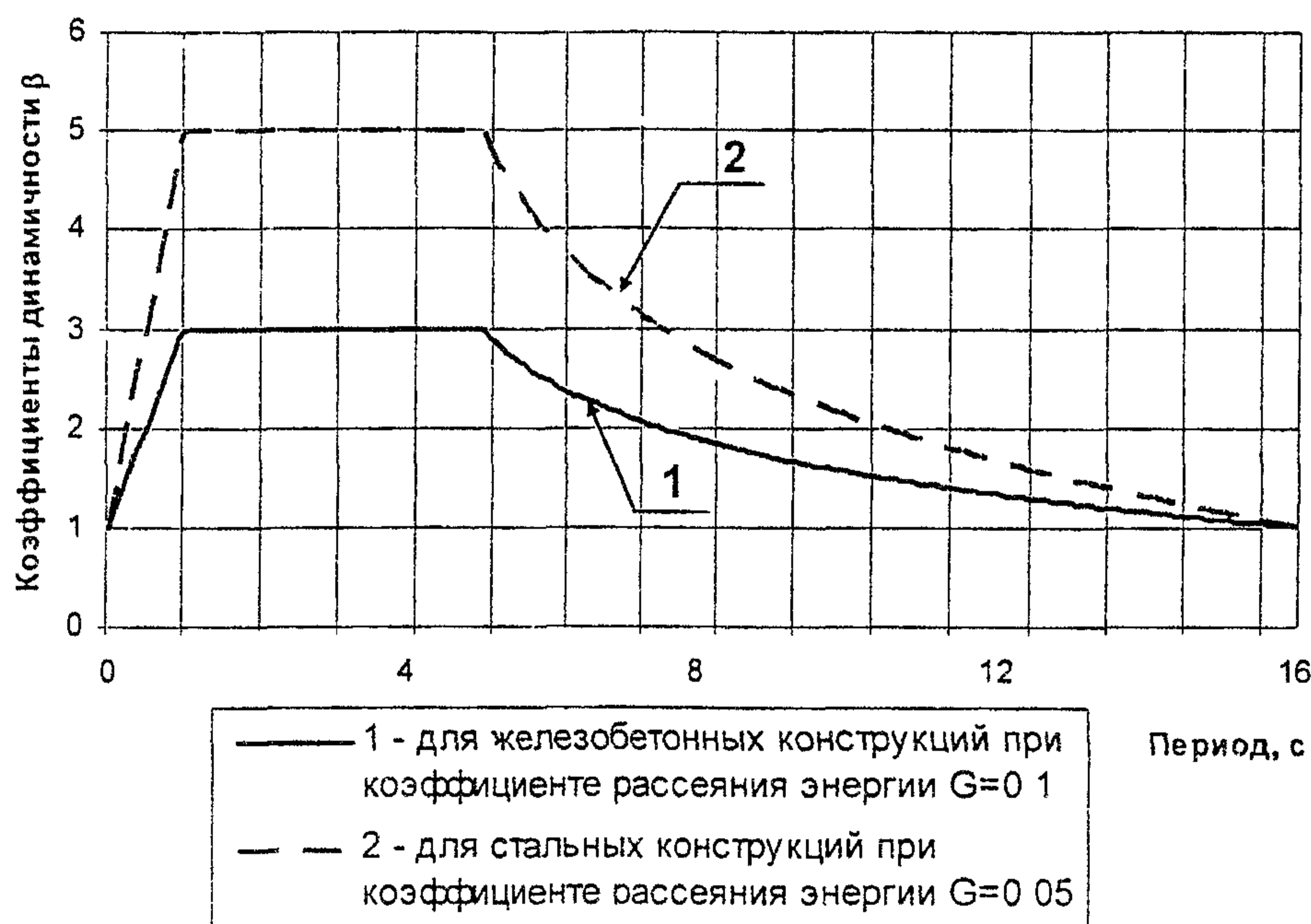
Рис. 5.2.3 Графики коэффициентов динамичности
