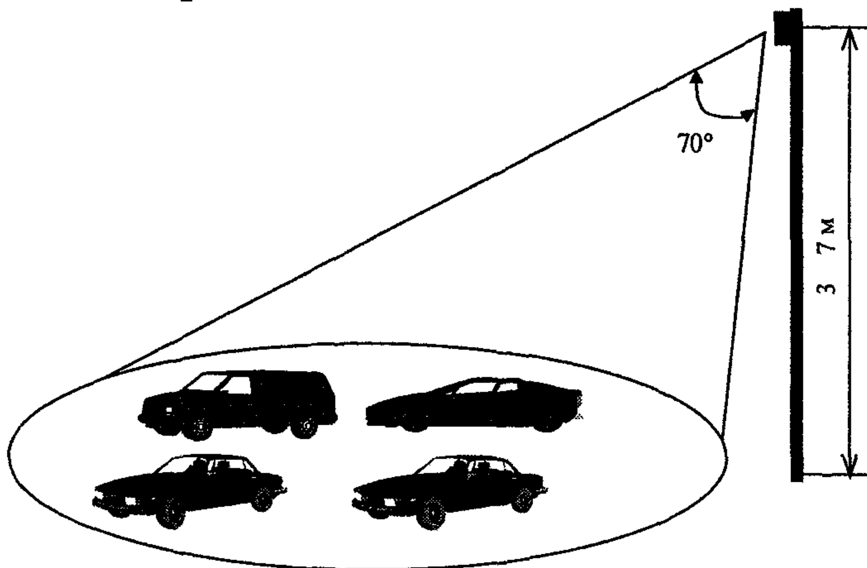
Вариант блокировки открытых площадок ( S, \text{м}^2 = 300...400 ) извещателем объемным радиоволновым
