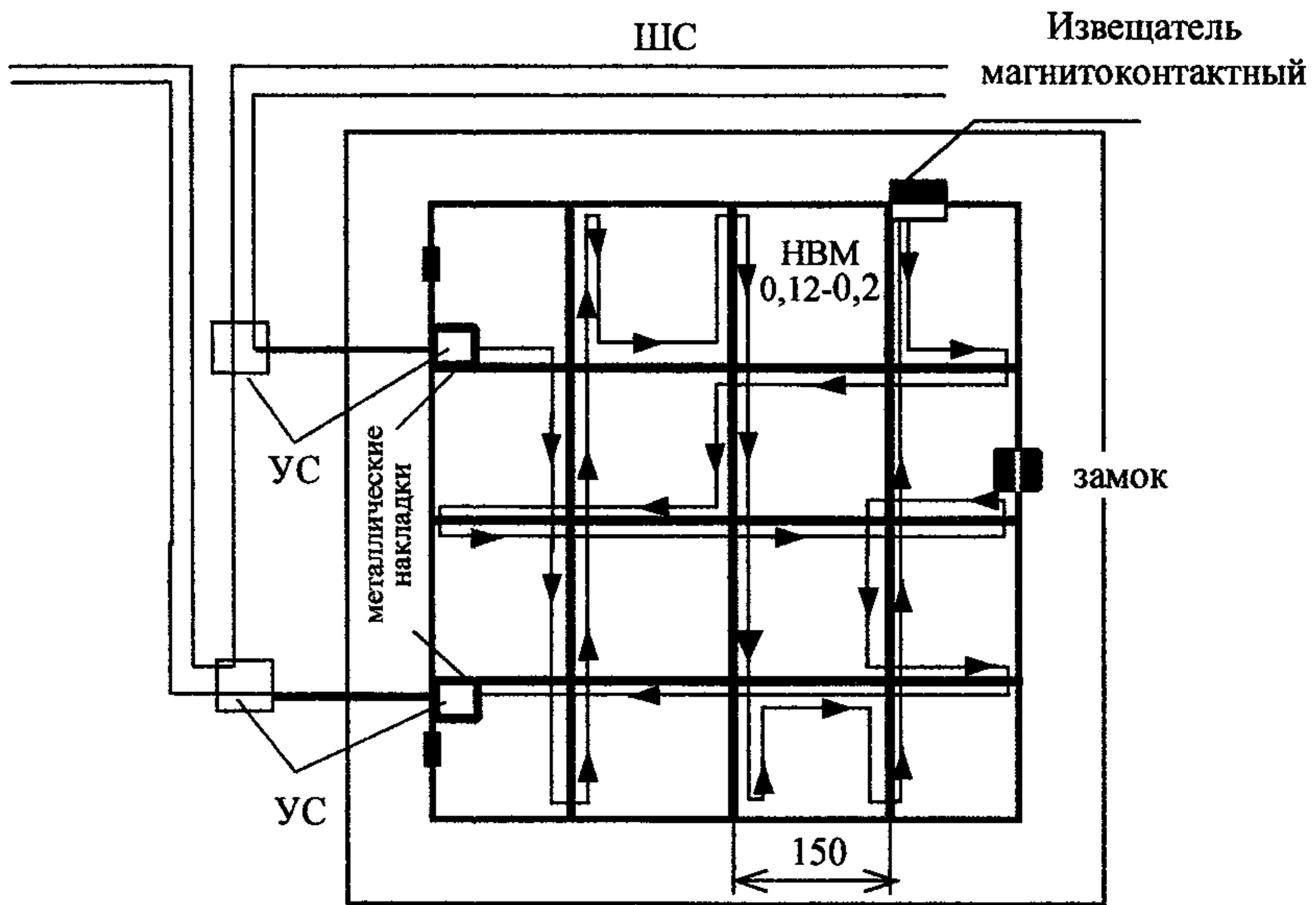
Вариант 3. Блокировка открывающихся решеток проводом
