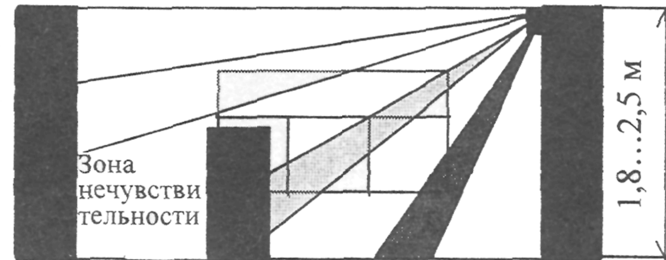
Вариант 7. Одновременная блокировка объема и отдельных предметов оптико-электронным извещателем
