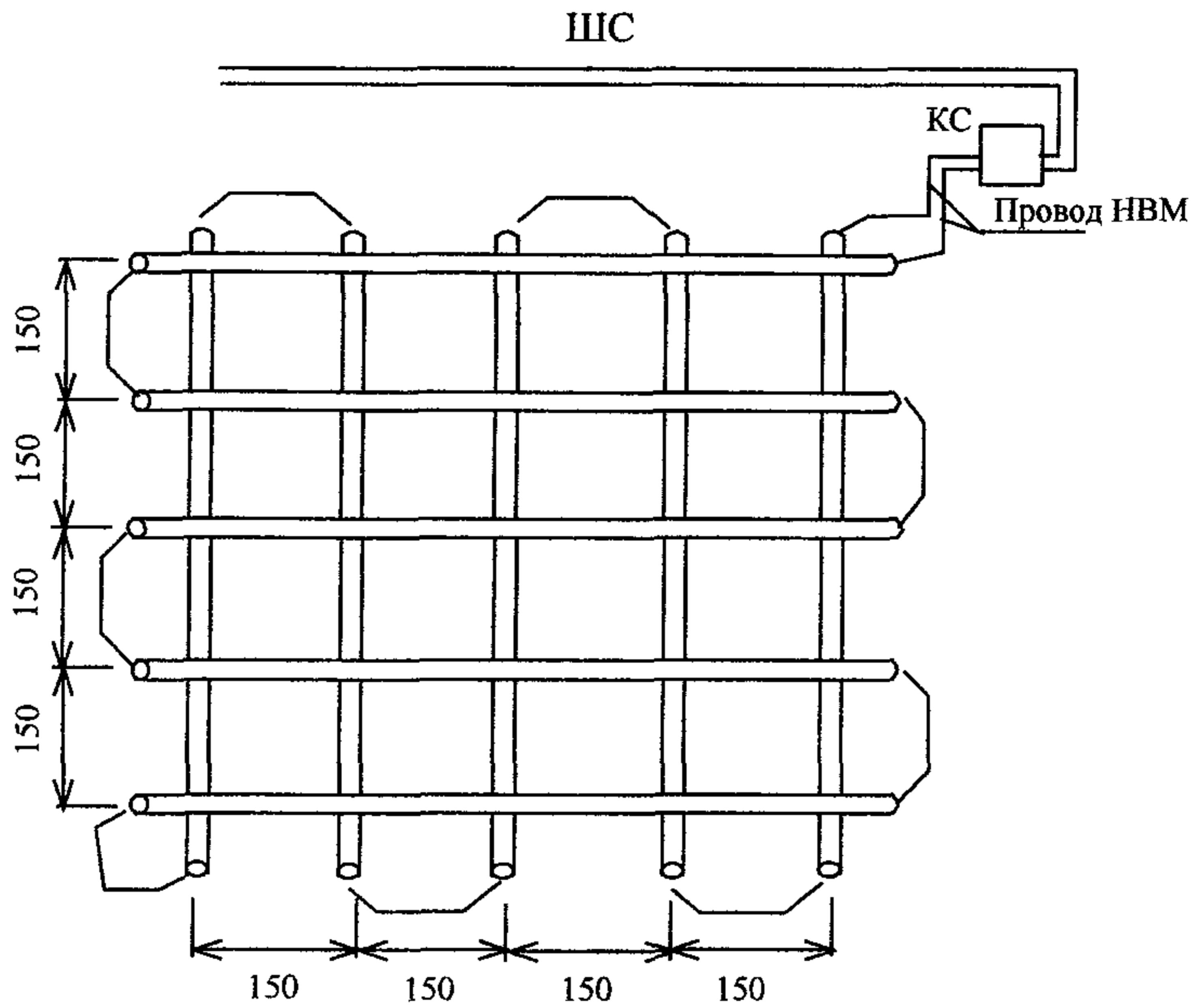
Вариант 1. Блокировка фальшрешетки проводом
