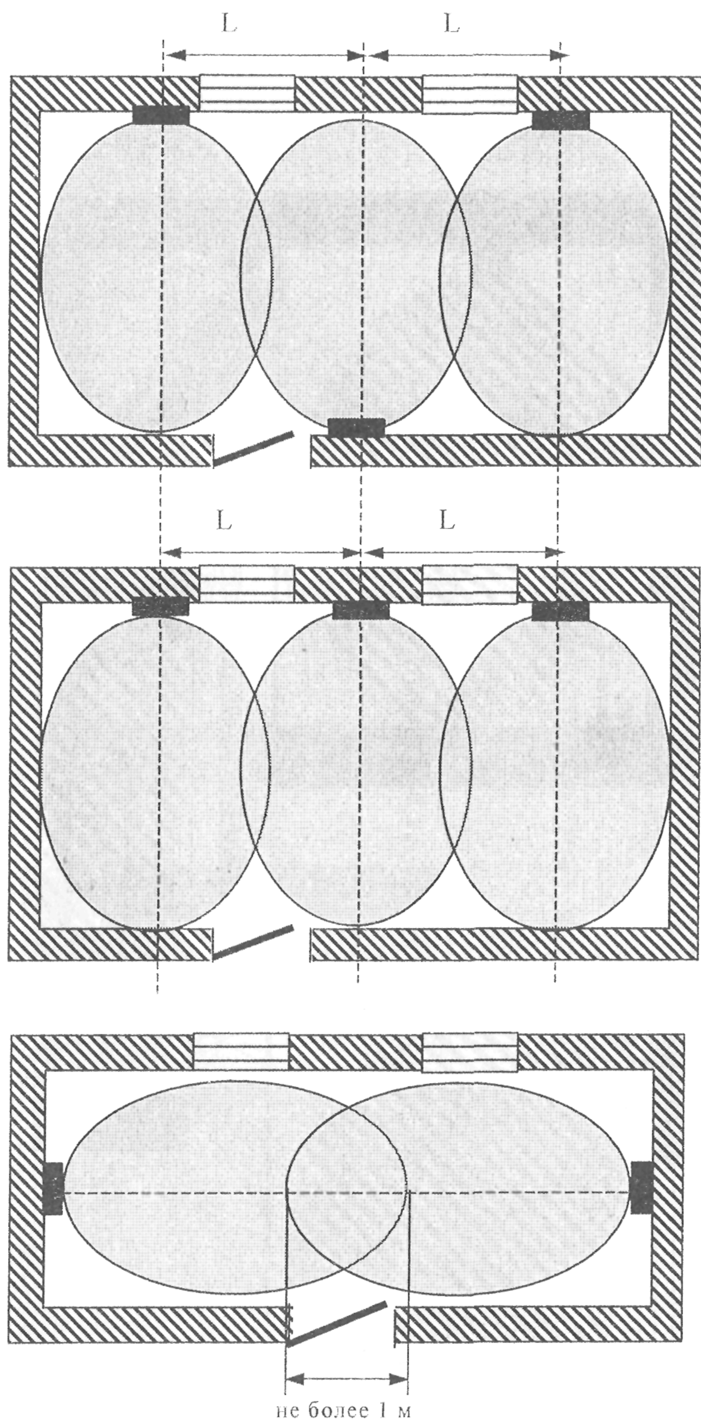
Вариант 2. Блокировка помещения несколькими объемными радиоволновыми (комбинированными) извещателями
