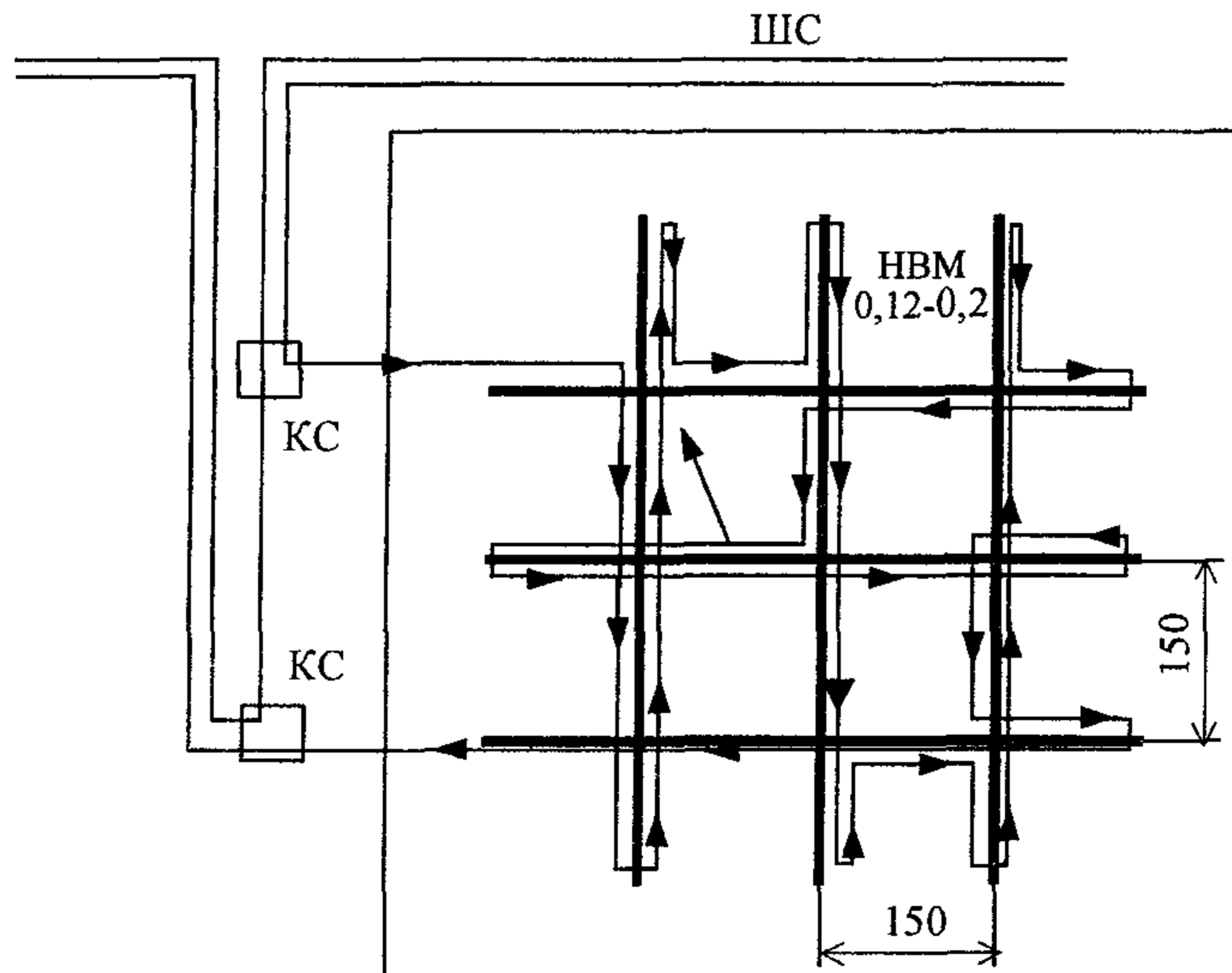
Вариант 2. Блокировка неоткрывающихся решеток проводом
