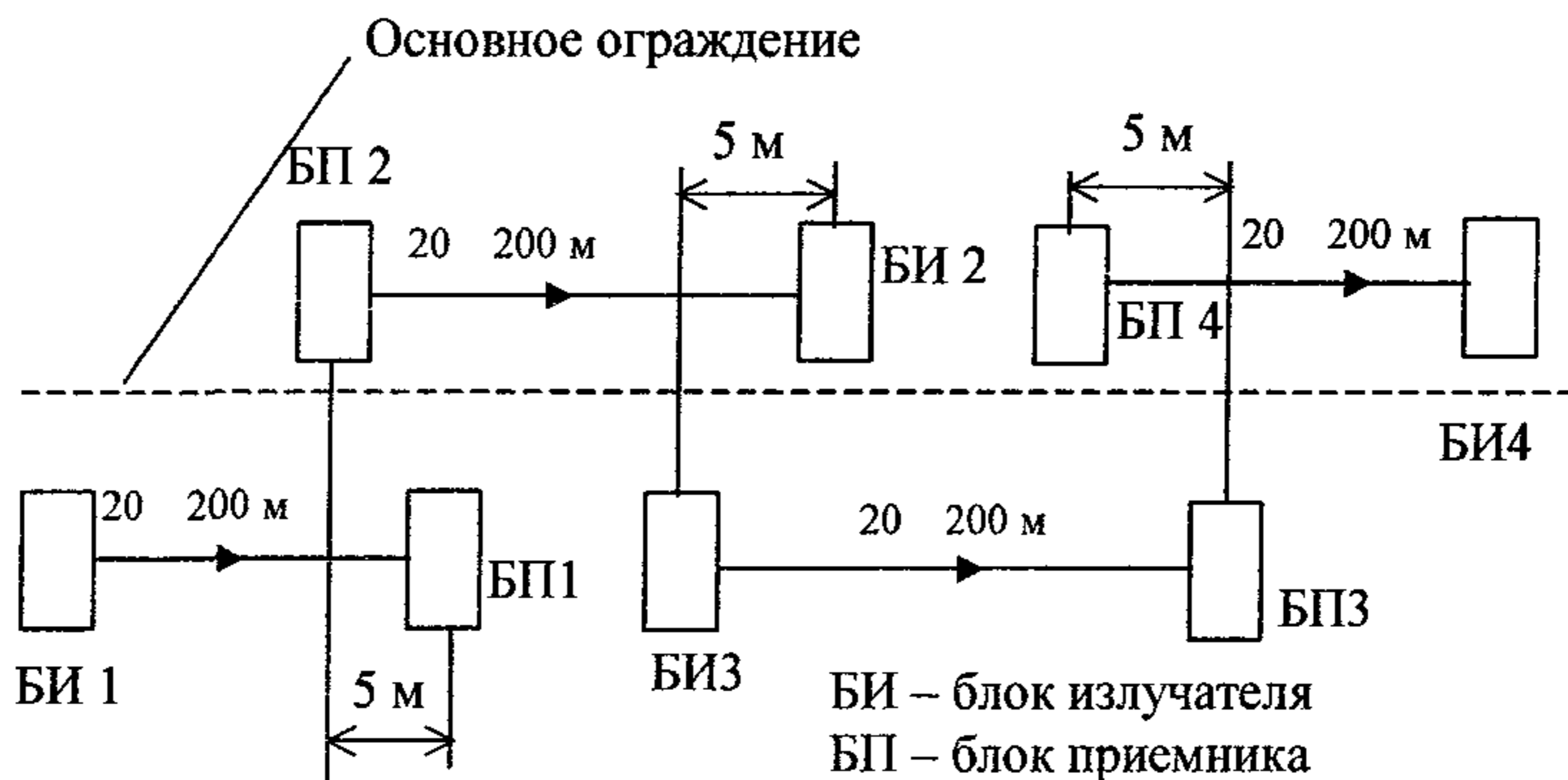
Вариант 1. Блокировка основного ограждения извещателями линейными радиоволновыми
