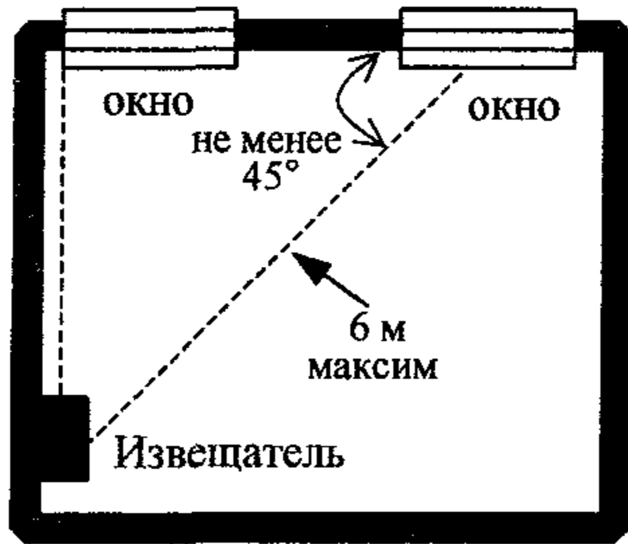
Вариант 6. Блокировка окон (витрин, витражей) на разбитие извещателями поверхностными звуковыми
