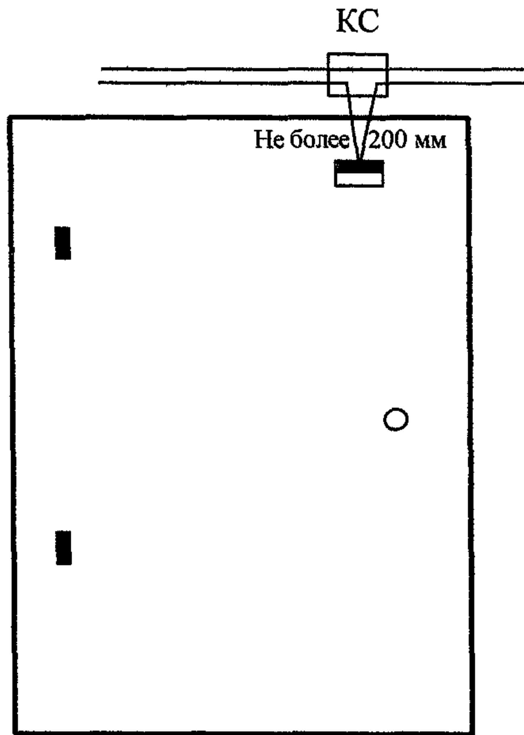
Вариант 2. Блокировка двери на открывание извещателем магнитоконтактным
