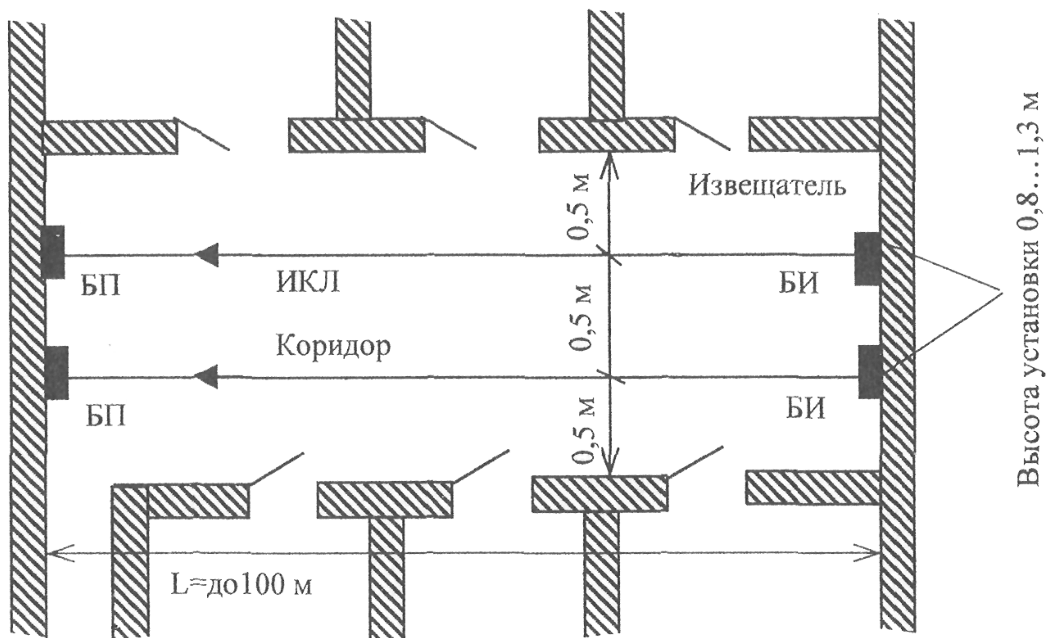
Вариант 1. Блокировка коридора извещателями активными линейными оптико-электронными
