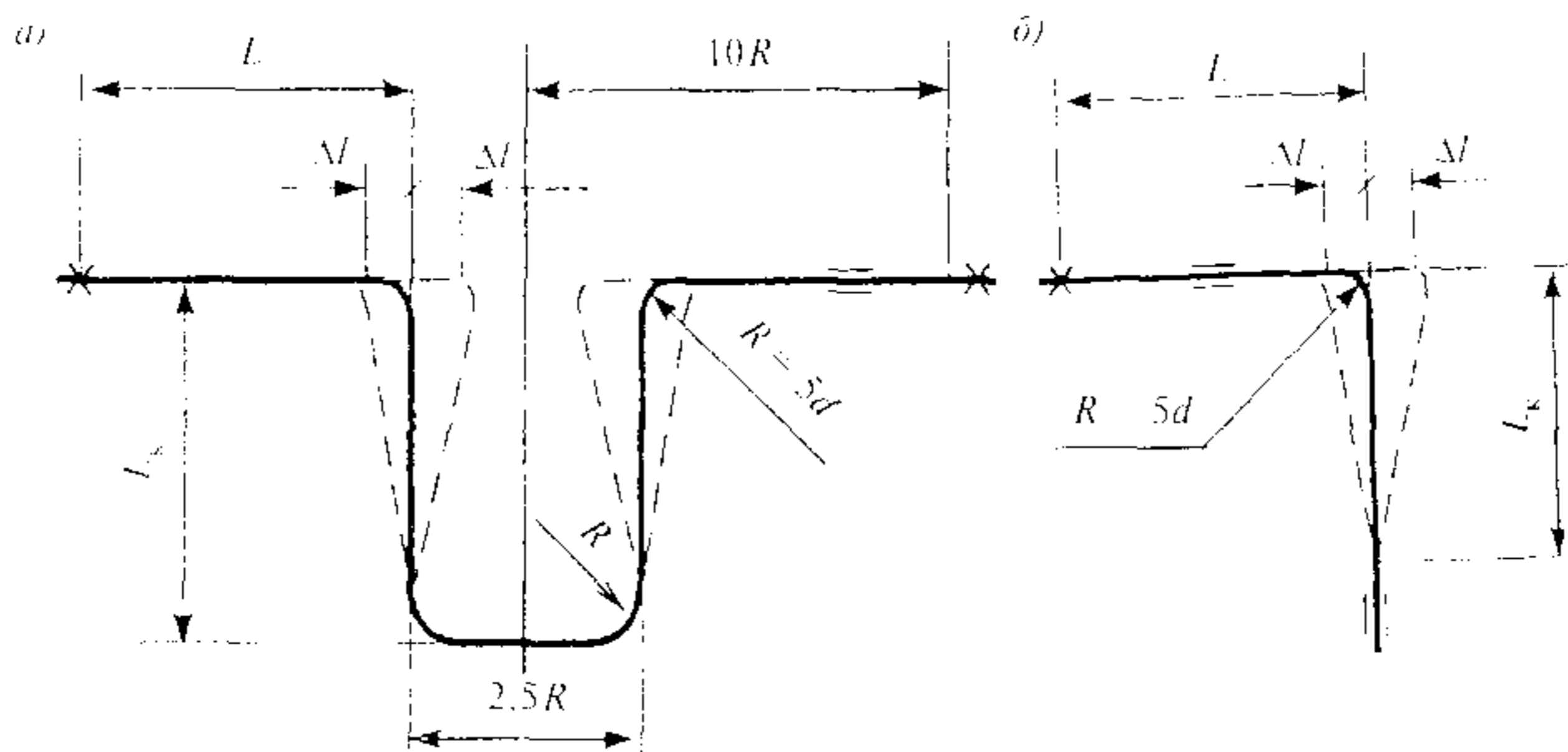
Рисунок 1 – Устройство П-образного (а) и Г-образного (б) компенсаторов
