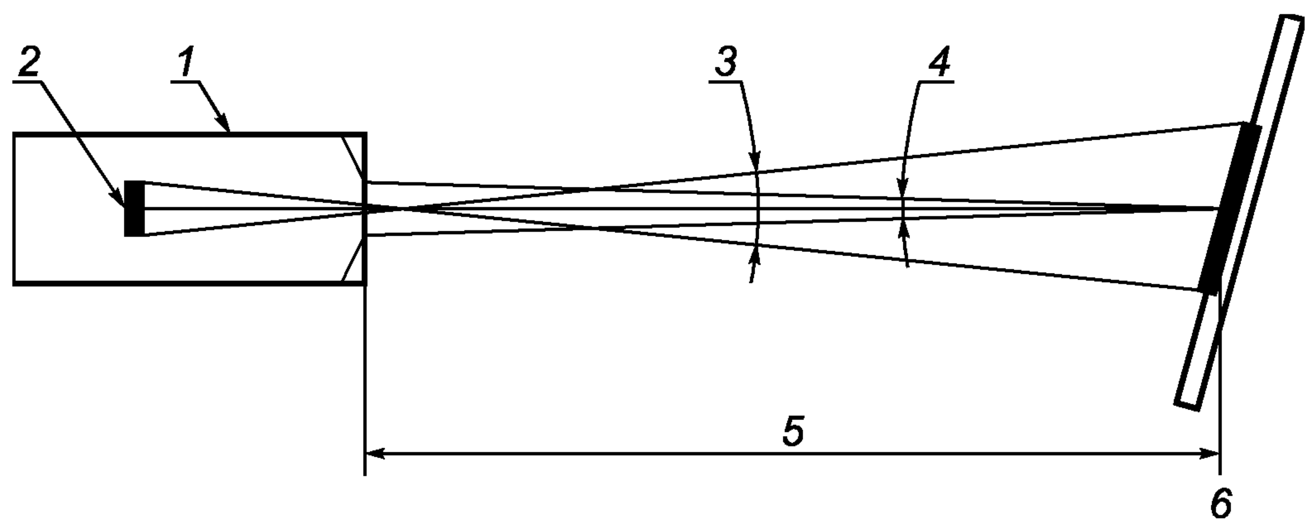
1 — фотометр; 2 — фоточувствительный элемент; 3 — поле обзора = поле зрения = угловой размер рассматриваемого объекта; 4 — приемный конус. Угол, образованный входным зрачком прибора на рабочем расстоянии; 5 — рабочее расстояние. Расстояние между передней линзой прибора и рассматриваемым объектом, который прибор может сфокусировать; 6 — EUT = испытуемое оборудование (см. 3.1.4)
