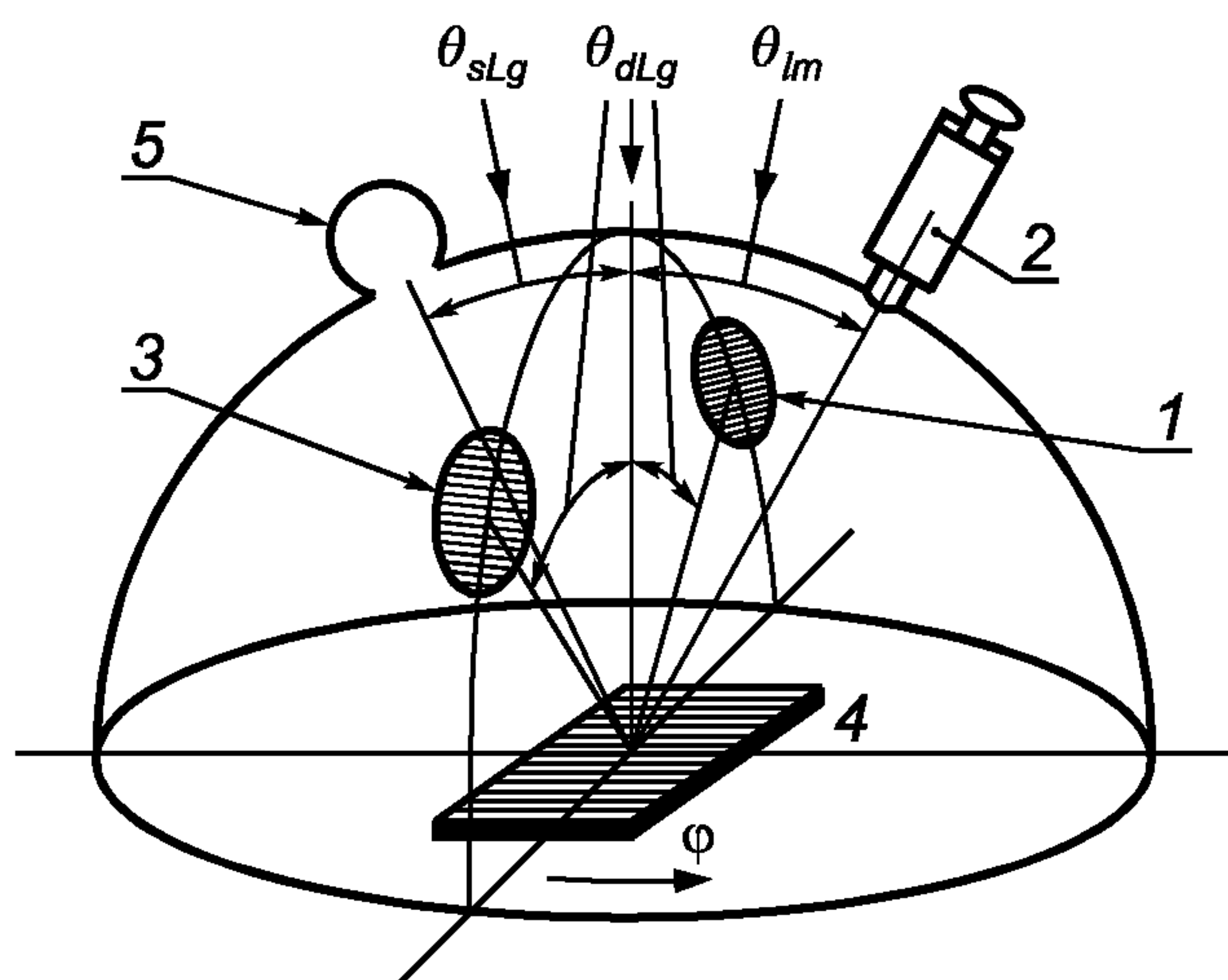
1, 3 — диффузные источники света; 2 — точечный фотометр с полем зрения от 0,5^\circ до 2^\circ ; 4 — эталон поверхности диффузного отражения; 5 — источник света для испытаний зеркального отражения
