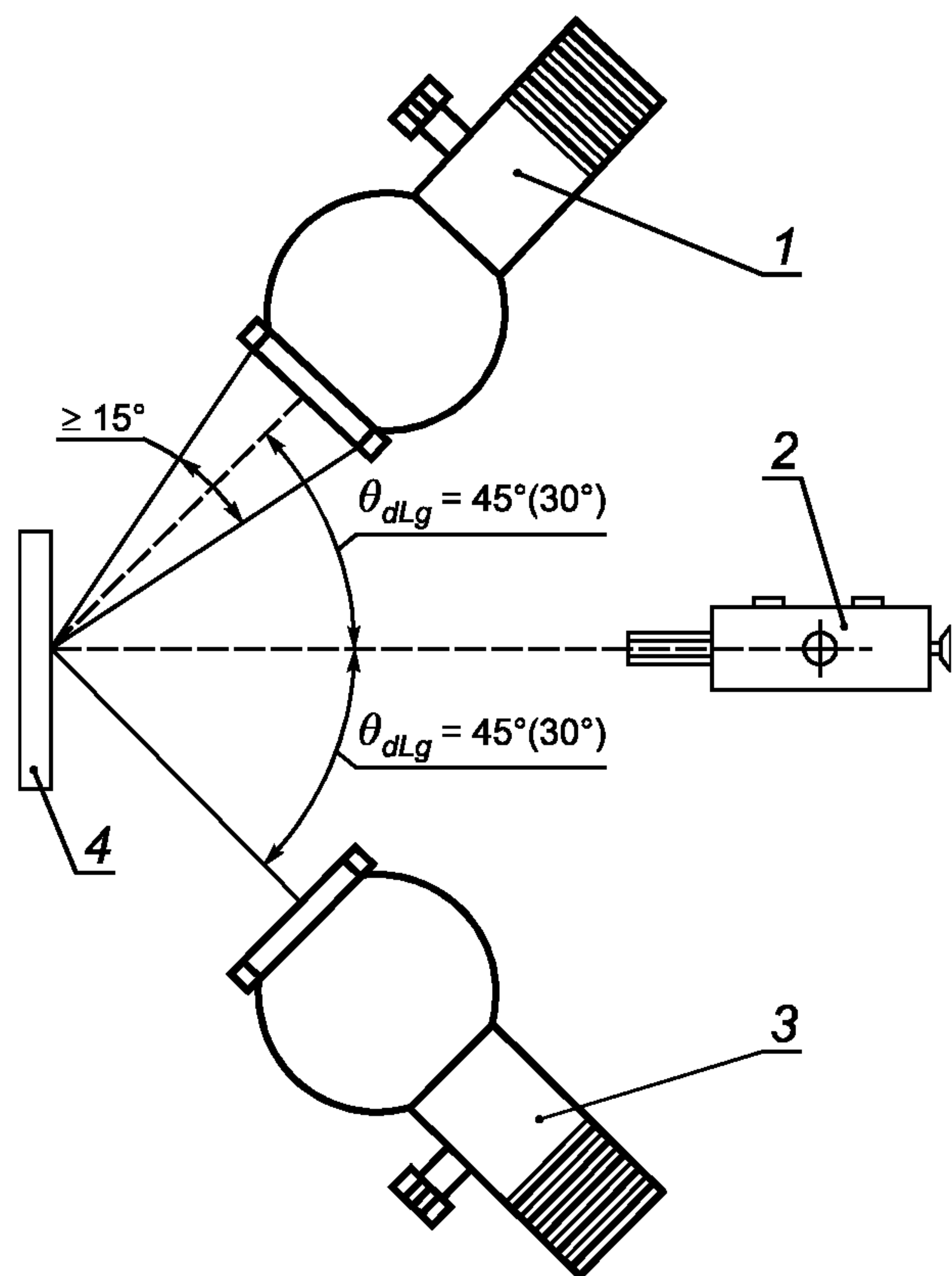
1, 3 — яркостные источники; 2 — точечный фотометр с полем зрения от 0,5° до 2°; 4 — эталон поверхности с диффузным отражением
