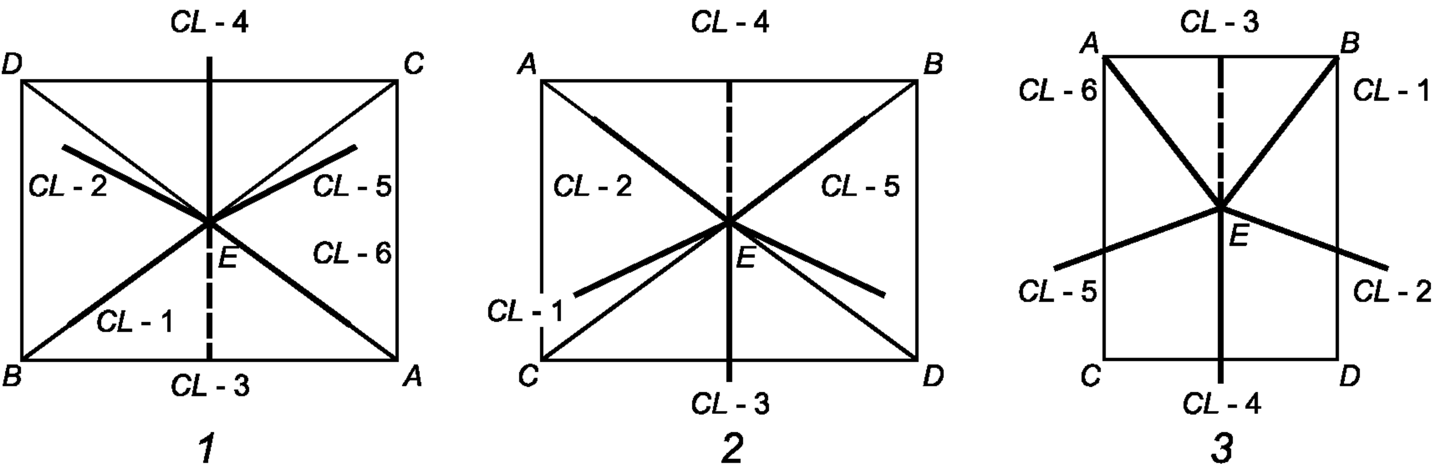
1 — пейзажная ориентация, \varphi_D = 90^\circ , \theta_D = 0^\circ и \varphi_C = 63,4^\circ (таблица 33); 2 — пейзажная ориентация, \varphi_D = 270^\circ , \theta_D = 0^\circ и \varphi_C = 63,4^\circ (таблица 34); 3 — портретная ориентация \varphi_D = 270^\circ , \theta_D = 10^\circ и \varphi_C = 71,6^\circ (таблица 35)
