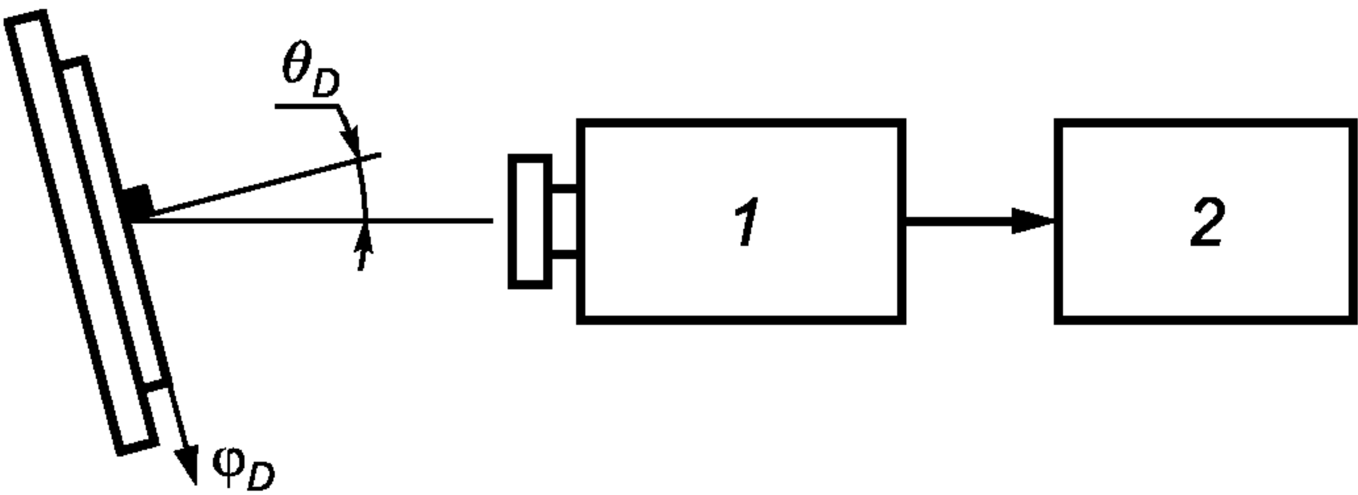
1 — фотометр; 2 — обработка данных
