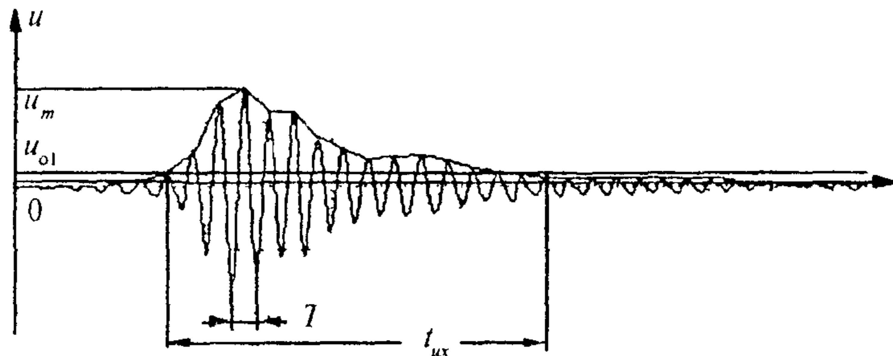
Рис. 1 Типичная импульсная характеристика ПАЭ
