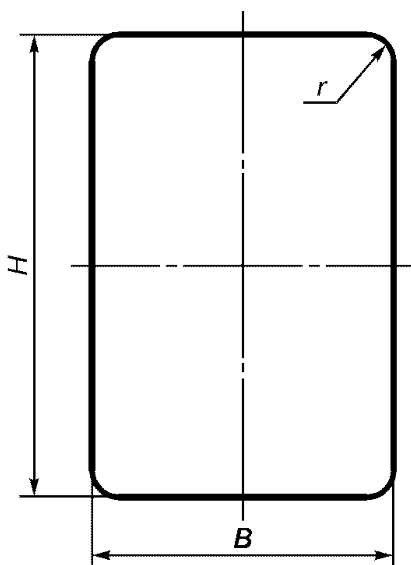
Рисунок Д.7 — Размеры прямоугольных знаков вертикального формата
