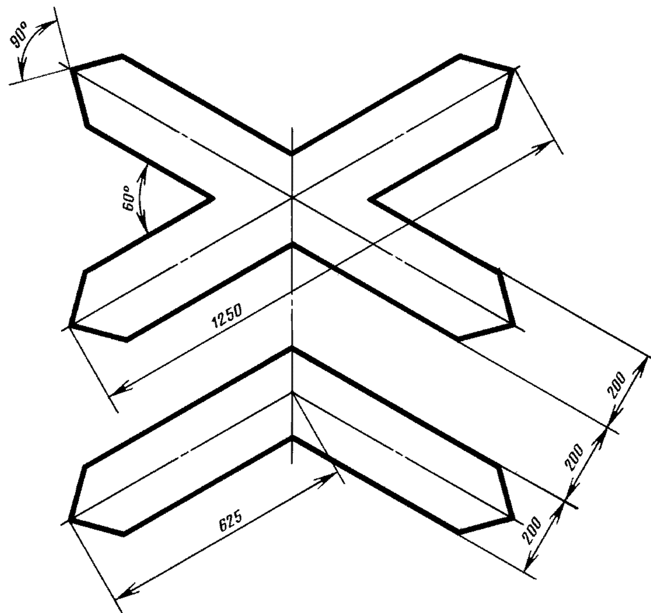
Рисунок Д.2 — Размеры знаков 1.3.1, 1.3.2
