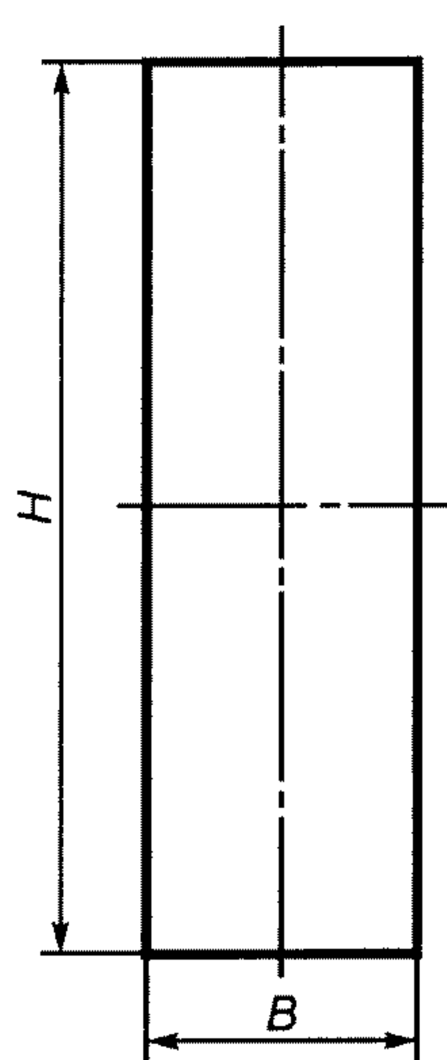
Рисунок Д.9 — Размеры знаков 8.22.1—8.22.3
