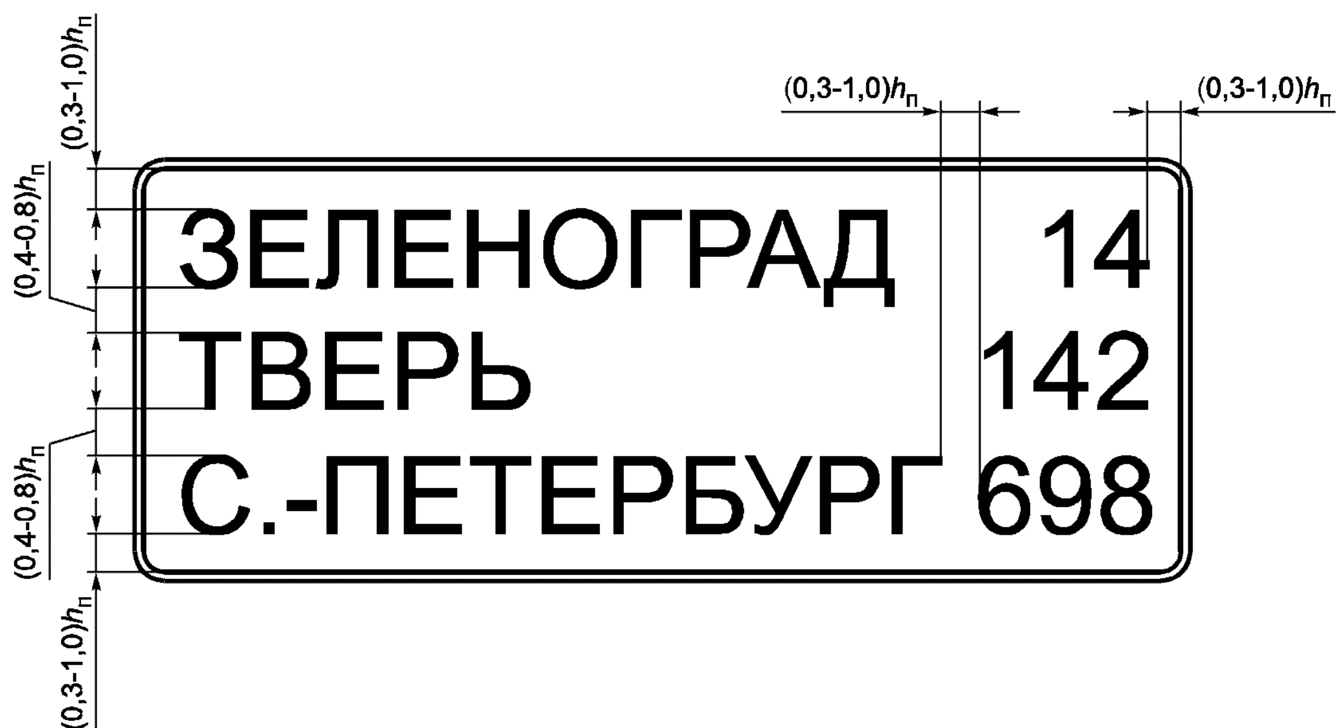
Рисунок Г.5 — Пример компоновки знака индивидуального проектирования 6.12
