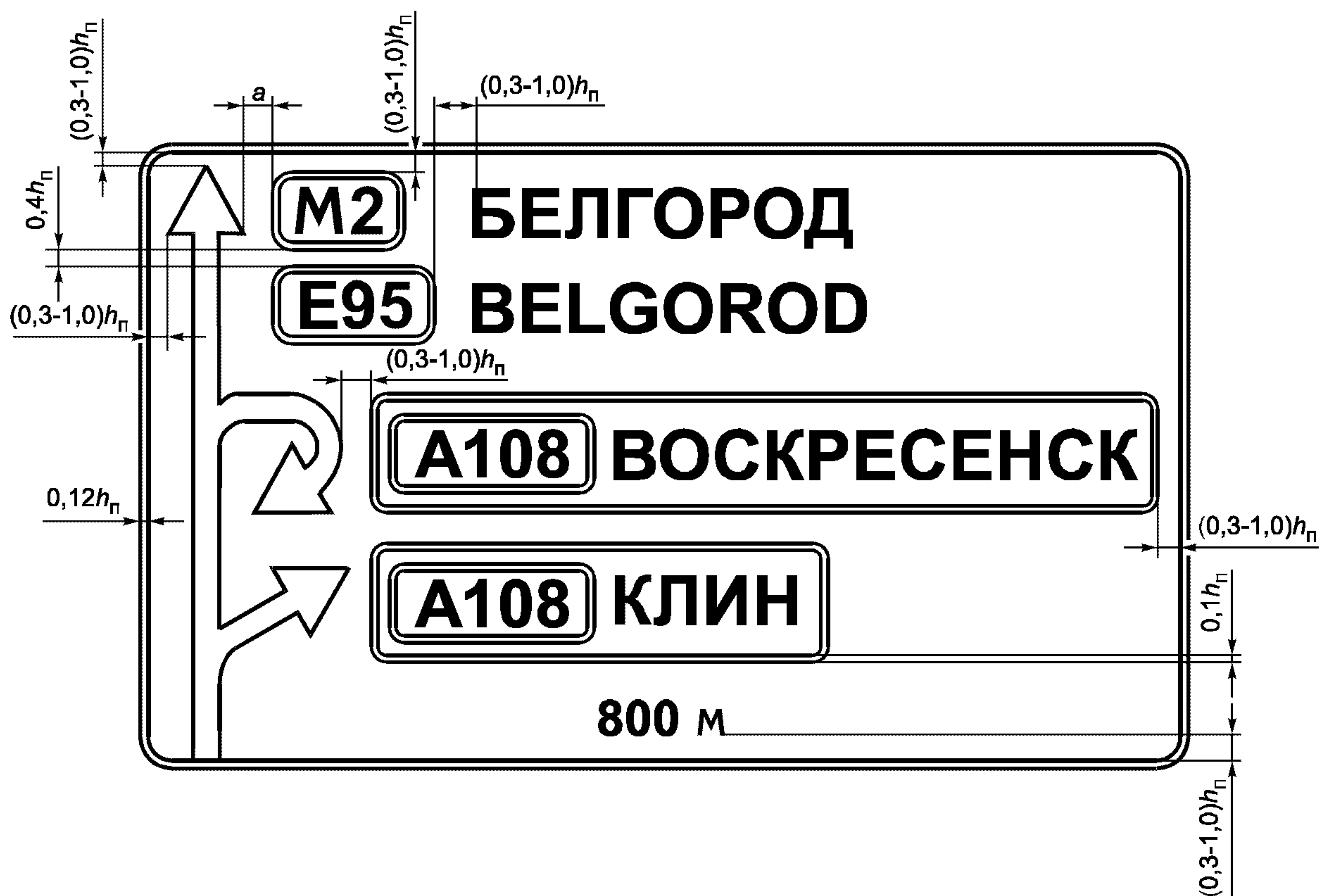
Рисунок Г.3 — Пример компоновки знака индивидуального проектирования 6.9.1
