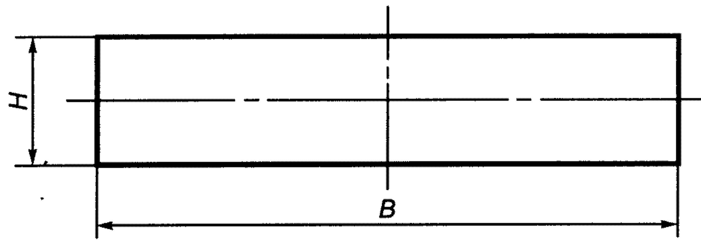
Рисунок Д.6 — Размеры знаков 1.34.1—1.34.3
