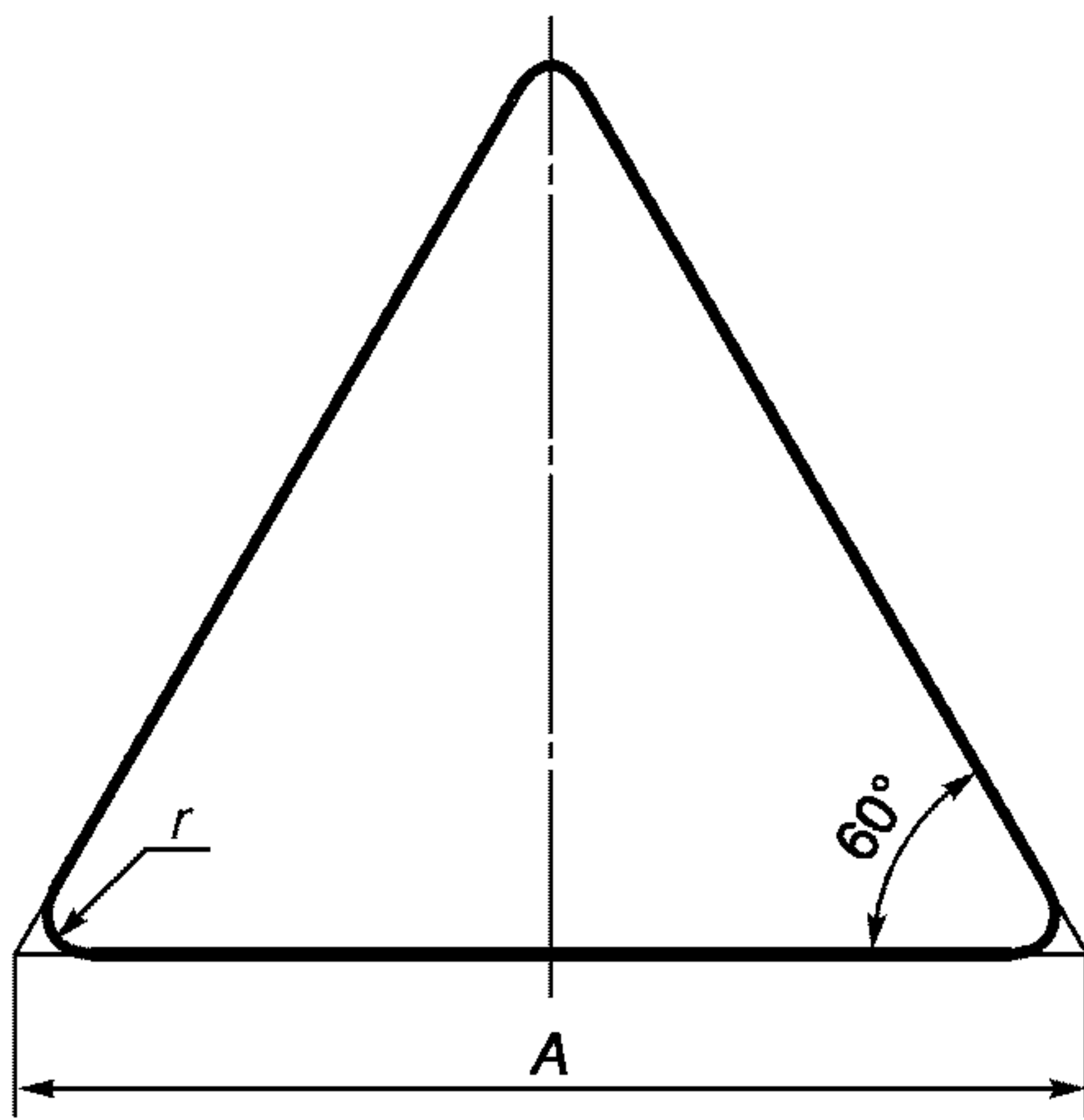
Рисунок Д.1 — Размеры треугольных знаков
