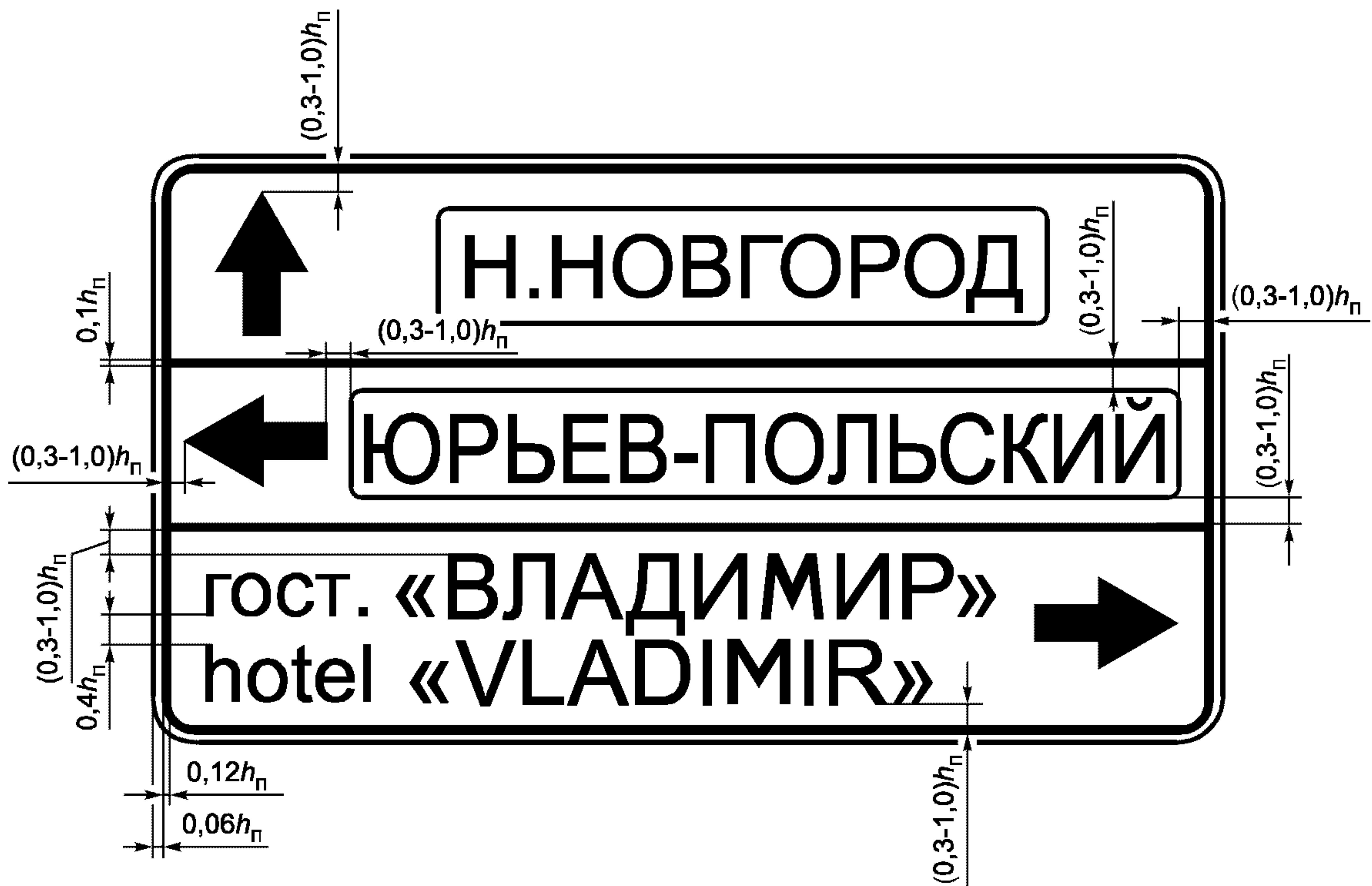
Рисунок Г.4 — Пример компоновки знака индивидуального проектирования 6.10.1
