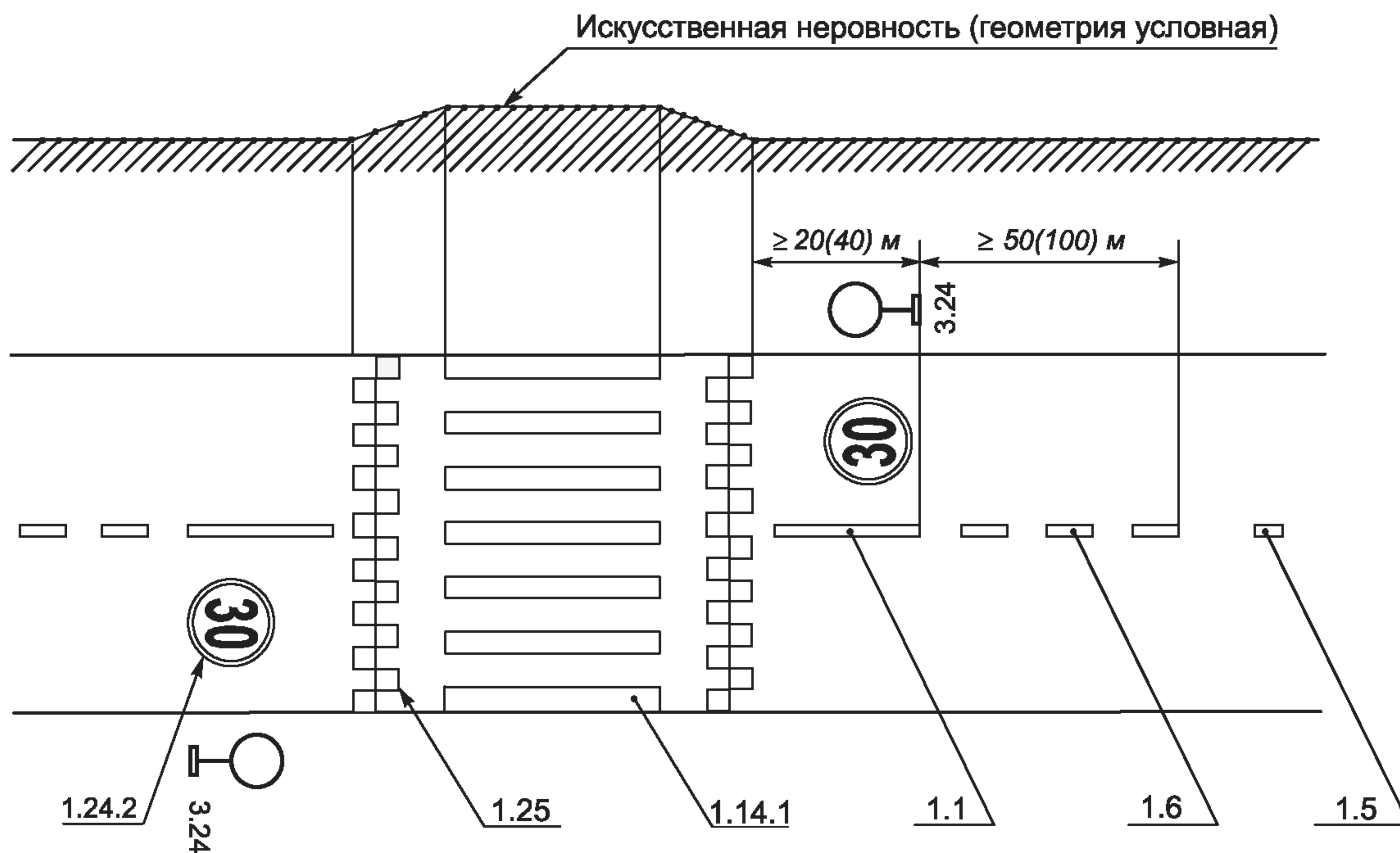
Рисунок В.19 — Пример нанесения разметки 1.25
