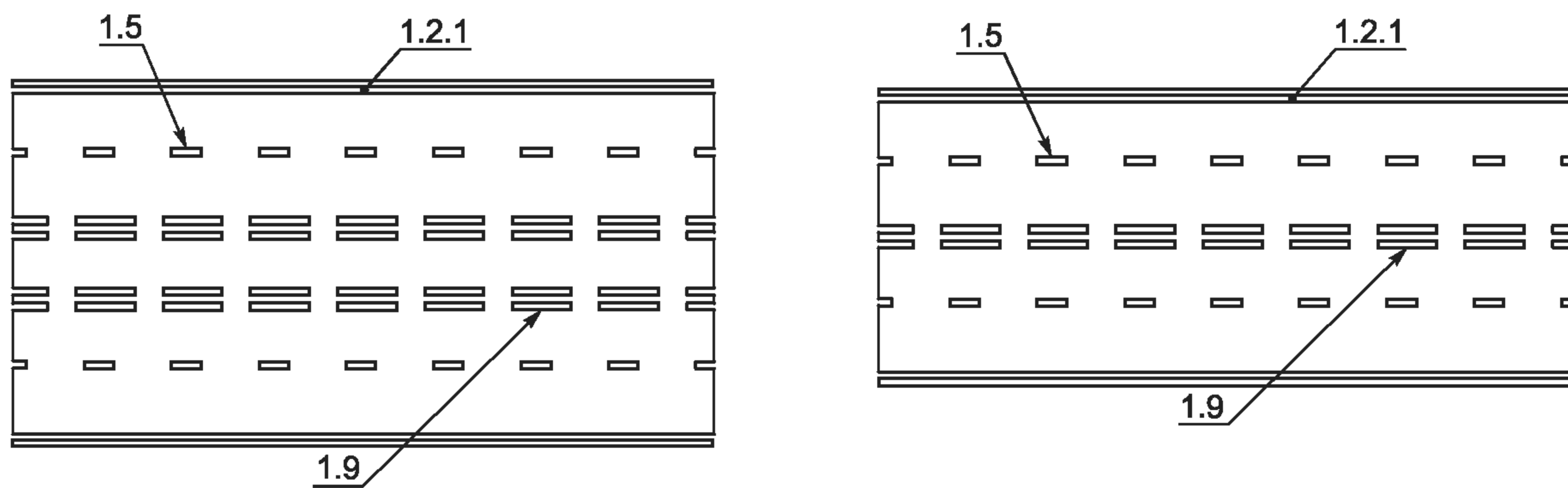
Рисунок В.16 — Примеры нанесения разметки 1.9
