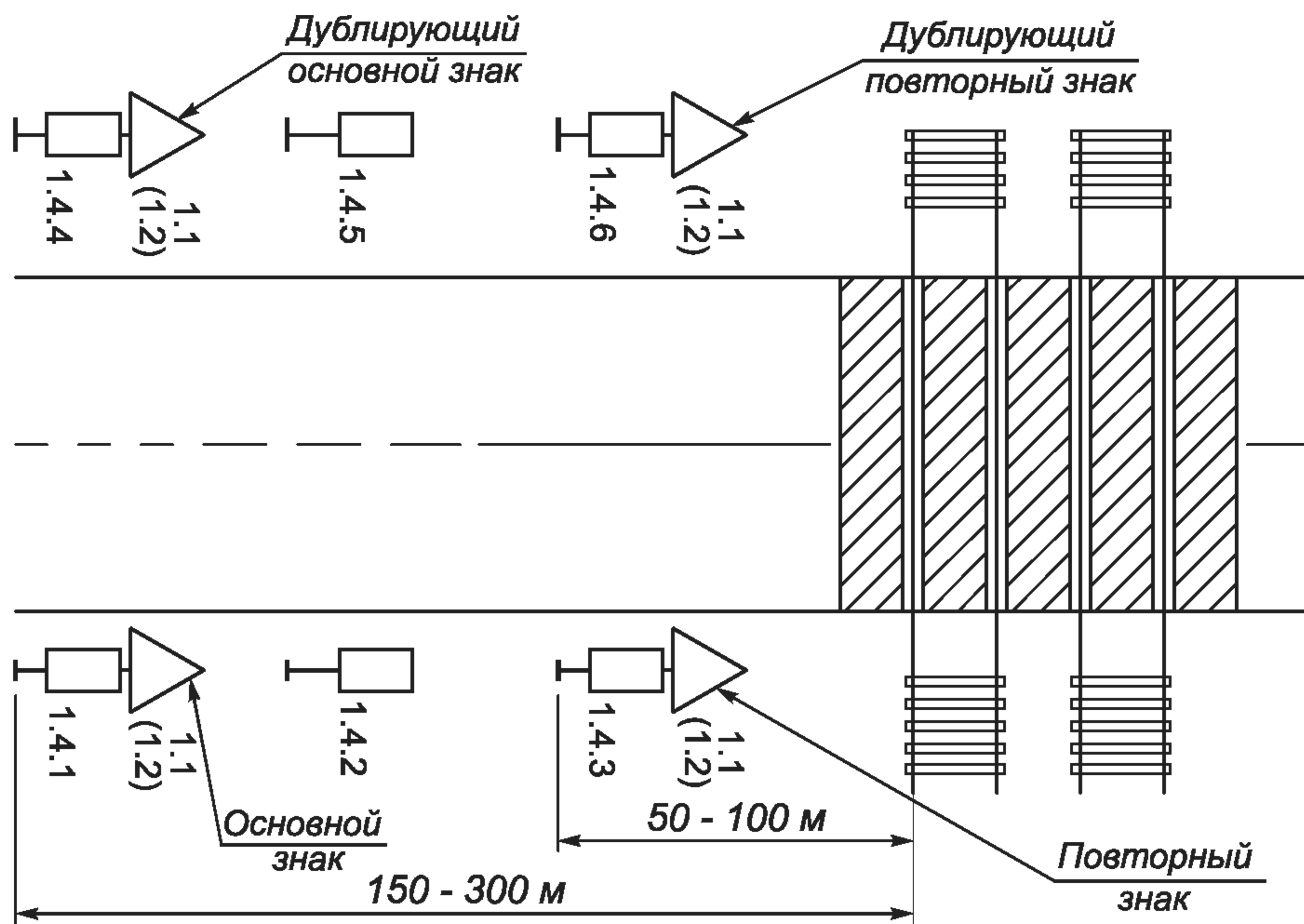
Рисунок В.3 — Размещение знаков 1.4.1—1.4.6
