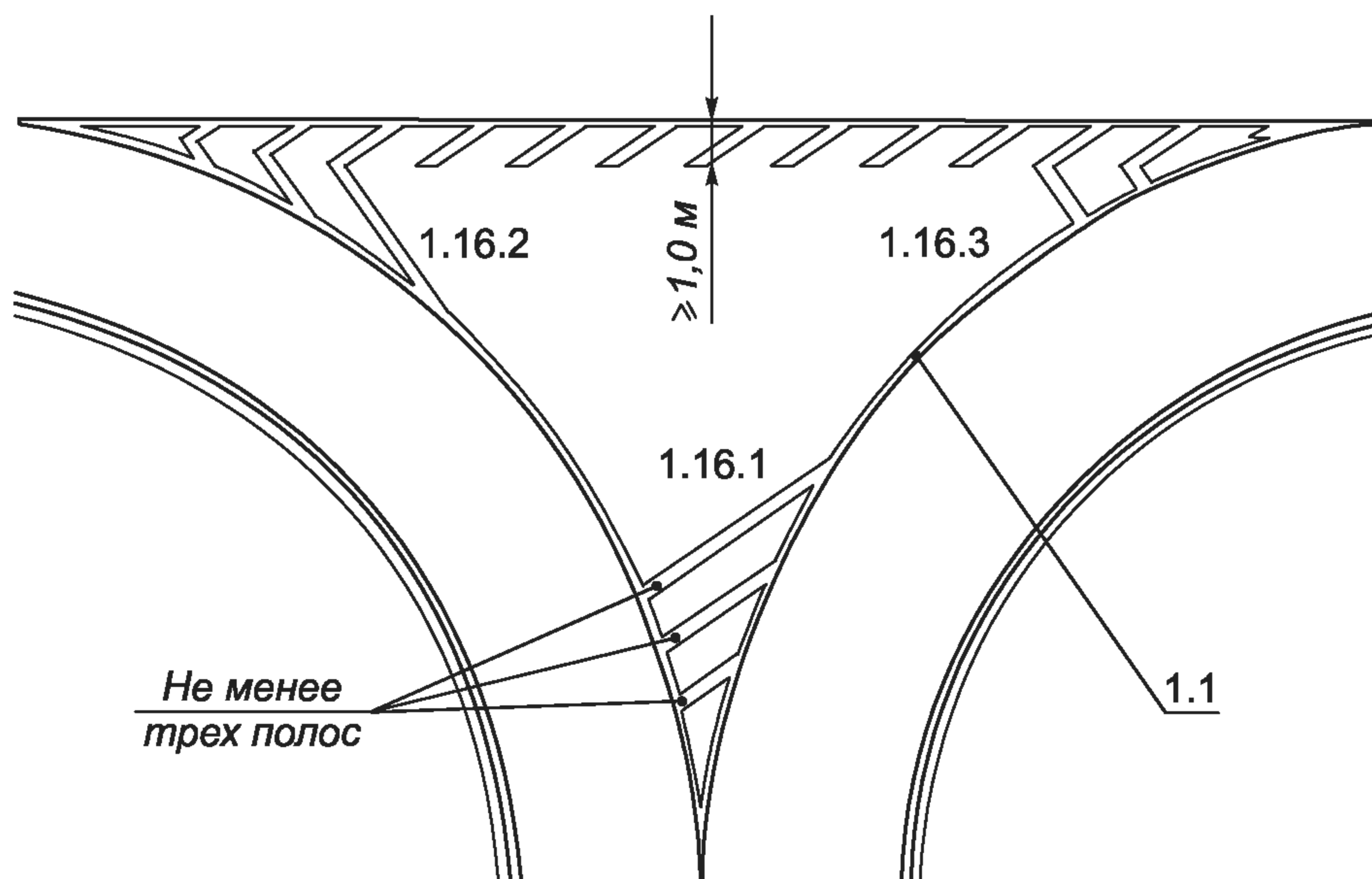
Рисунок В.12 — Пример нанесения разметки 1.16.1—1.16.3
