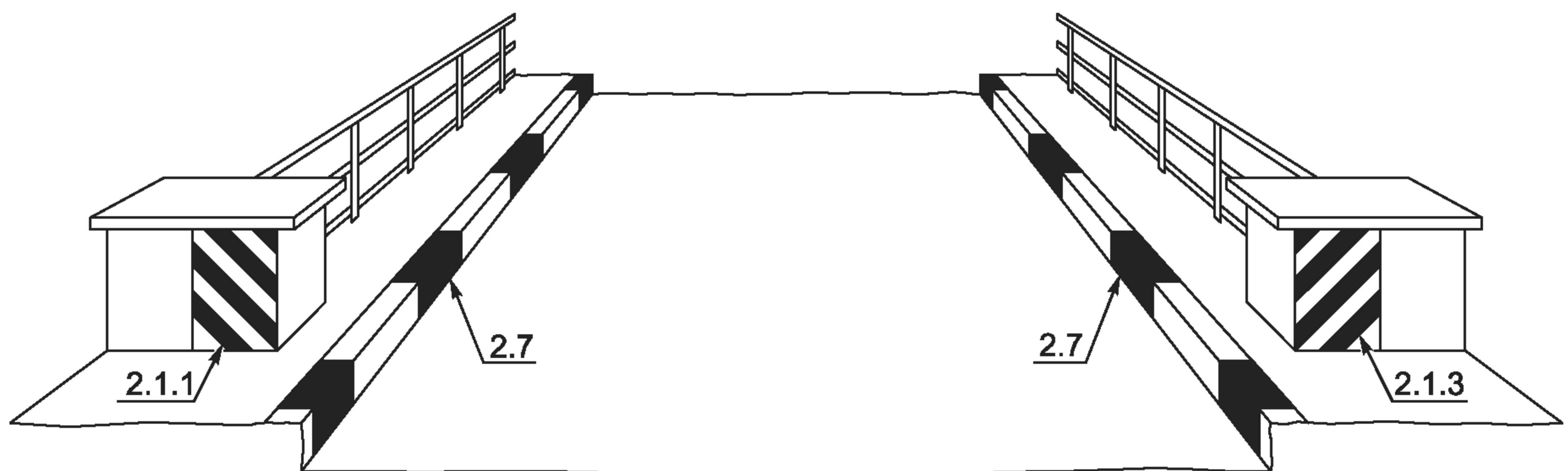
Рисунок В.21 — Пример нанесения разметки 2.1.1, 2.1.3 и 2.7
