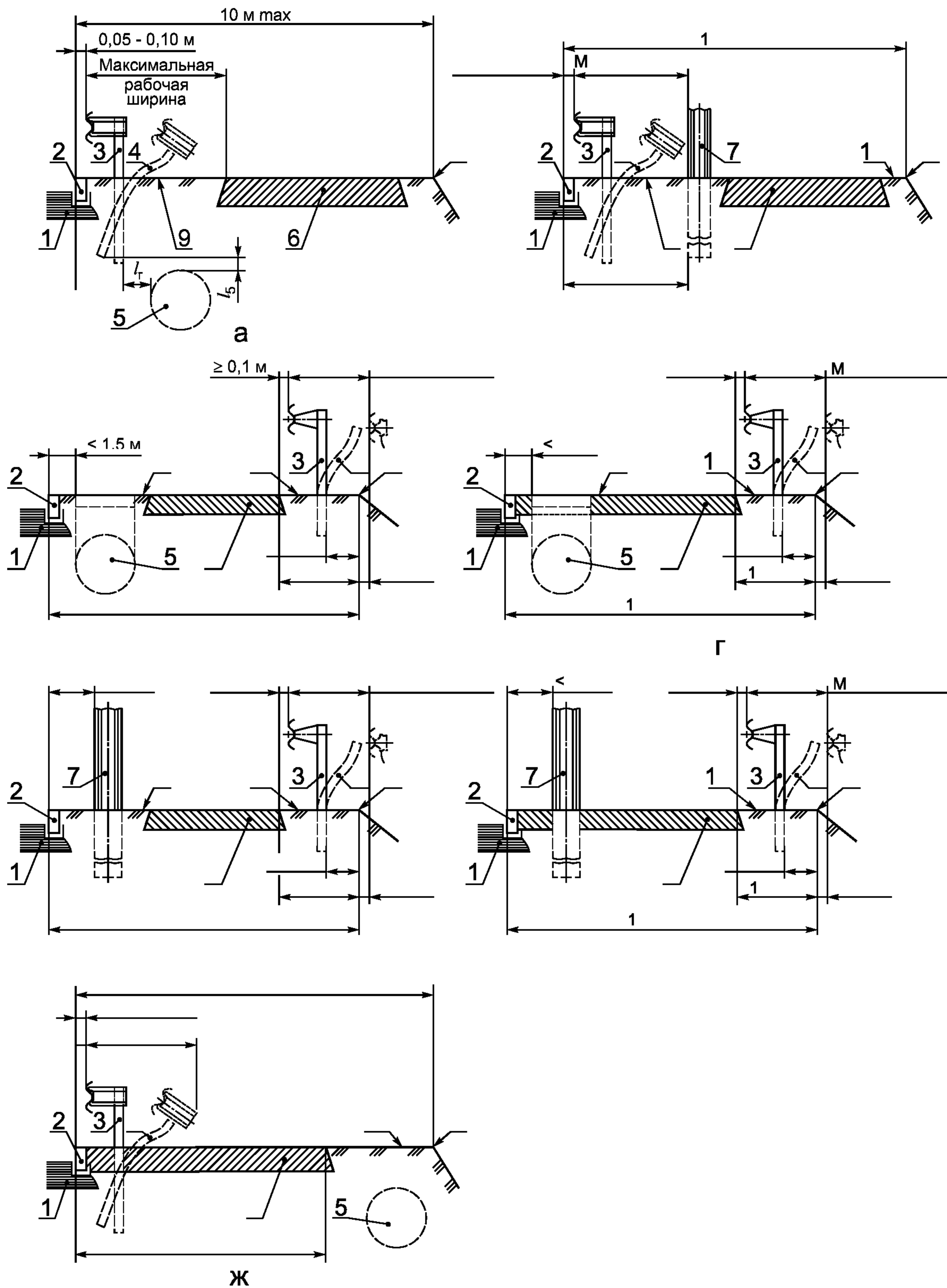
1 — проезжая часть; 2 — бортовой камень; 3 — недеформированное ограждение; 4 — деформированное ограждение; 5 — подземные инженерные сети; 6 — тротуар; 7 — массивная опора; 8 — бровка земельного полотна или край подпорной стены; 9 — газон; 10 — полоса между тротуаром и бровкой земельного полотна
