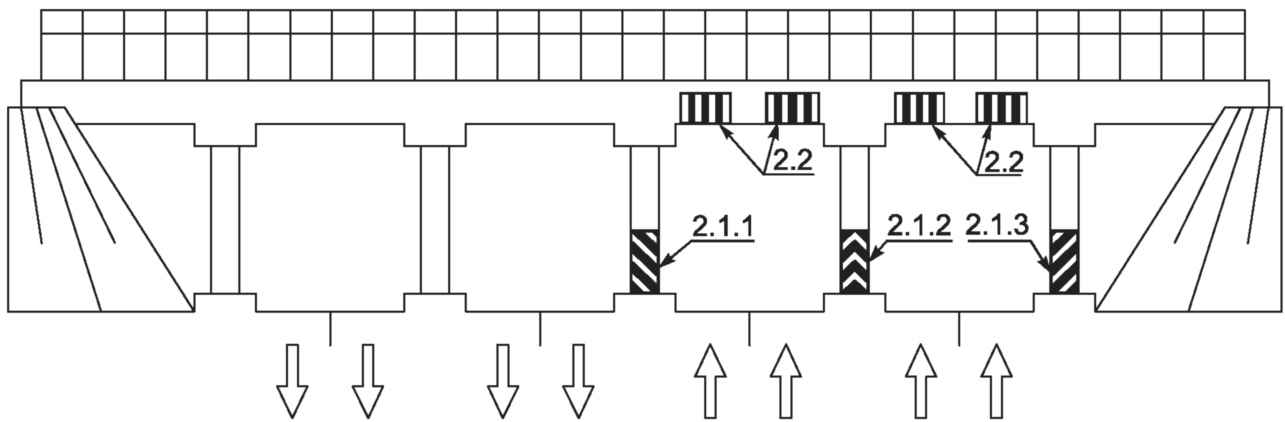
Рисунок В.20 — Пример нанесения разметки 2.1 и 2.2
