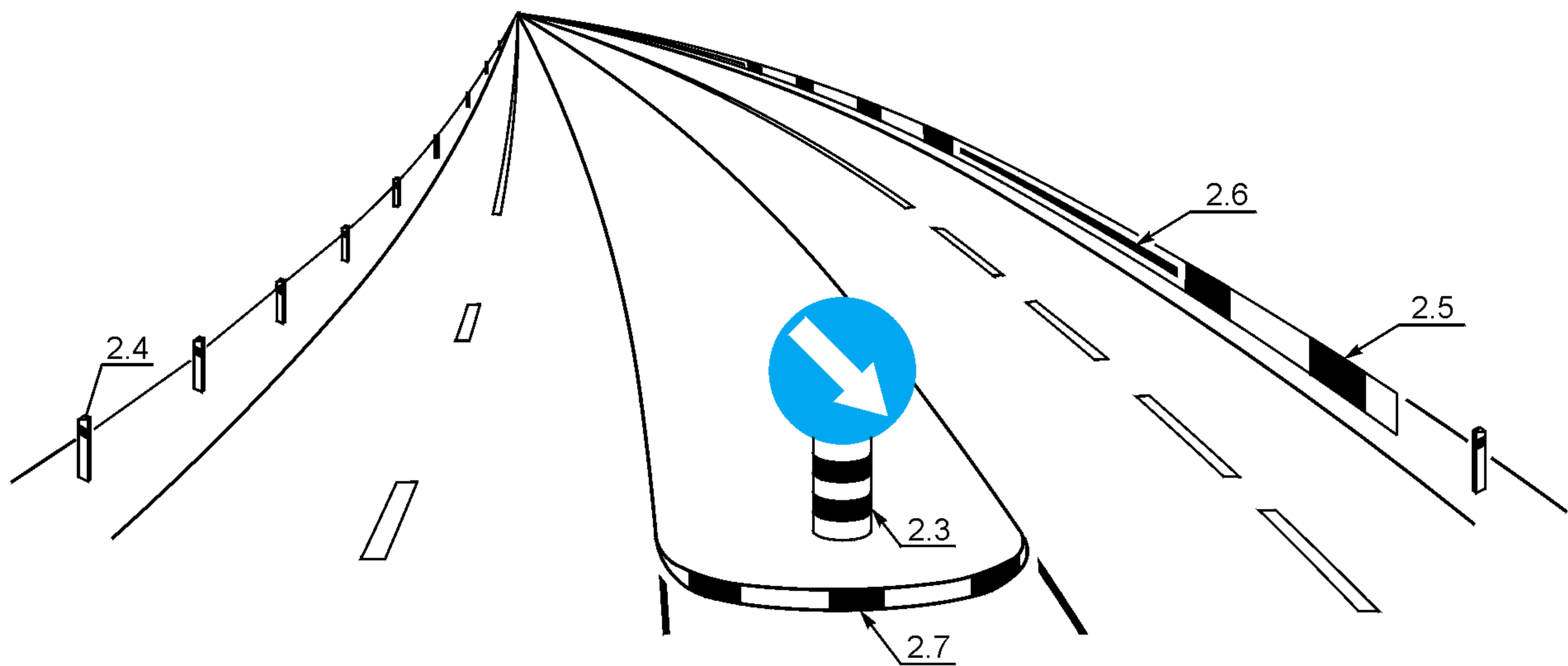
Рисунок В.22 — Пример нанесения разметки 2.3—2.7
