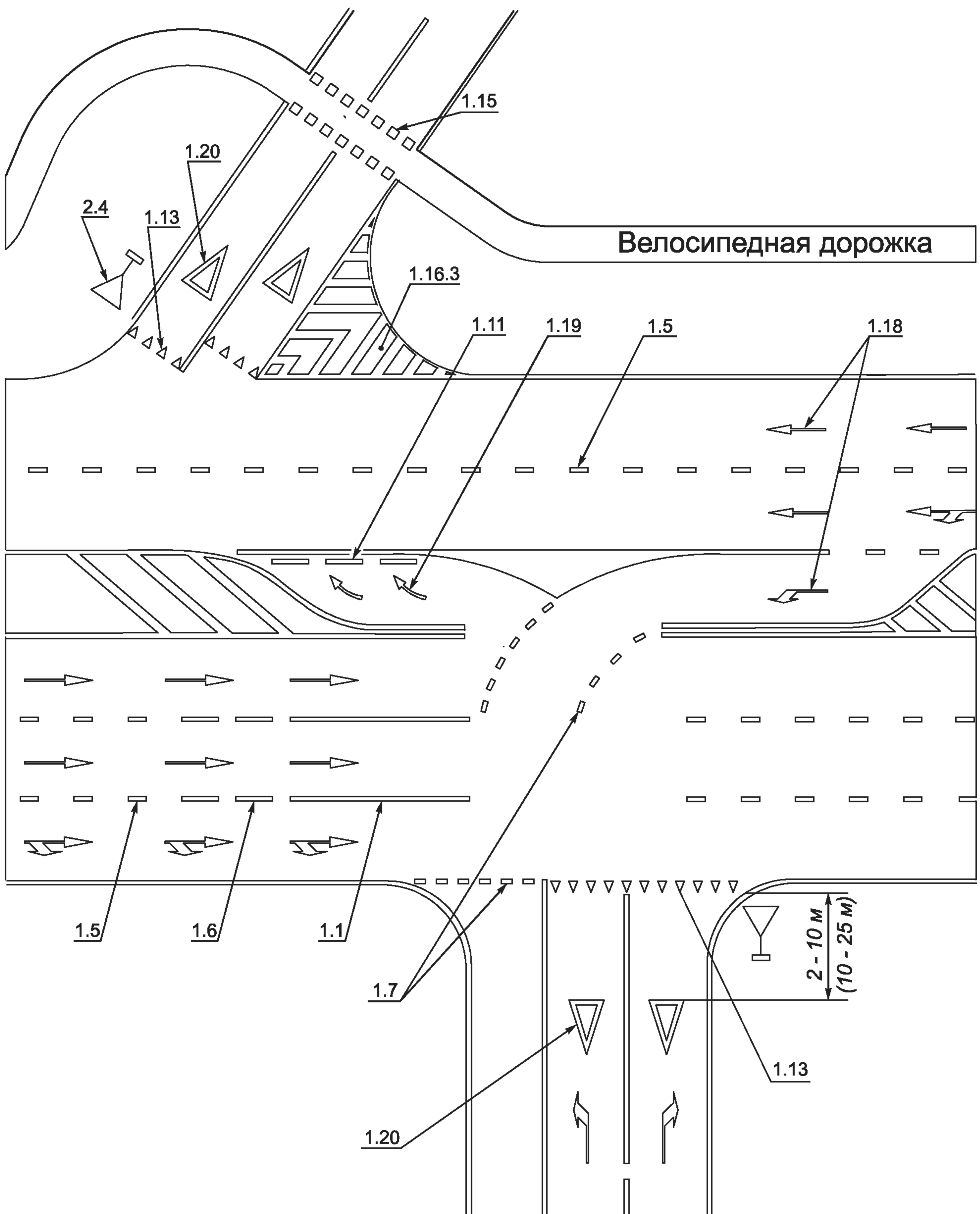
Рисунок В.10 — Пример нанесения разметки канализованного пересечения
