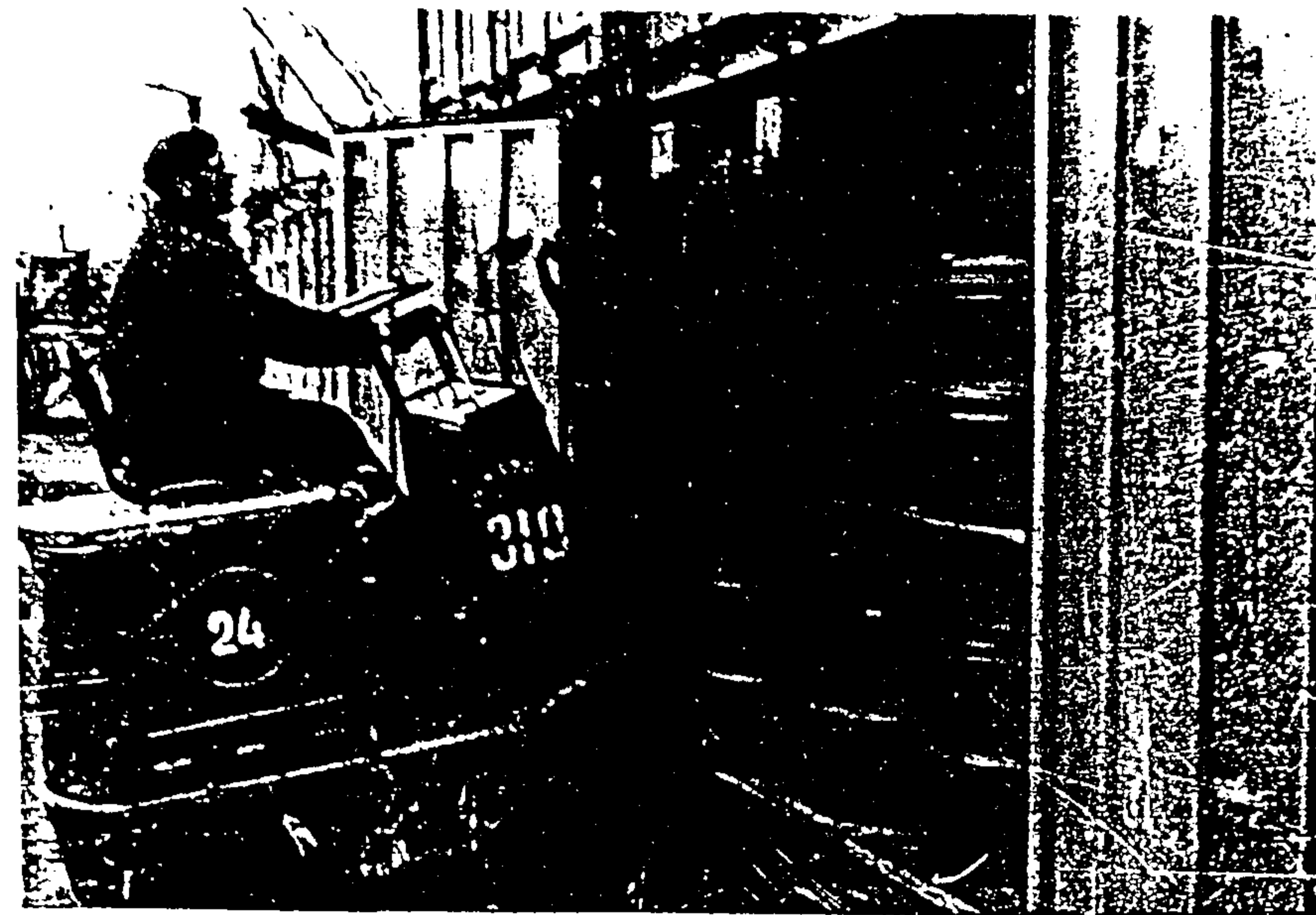
Рис.301.ЗК.2. Установка бочек в контейнере погрузчиком с торцевым захватом типа ЗГБ. Порт Находка
