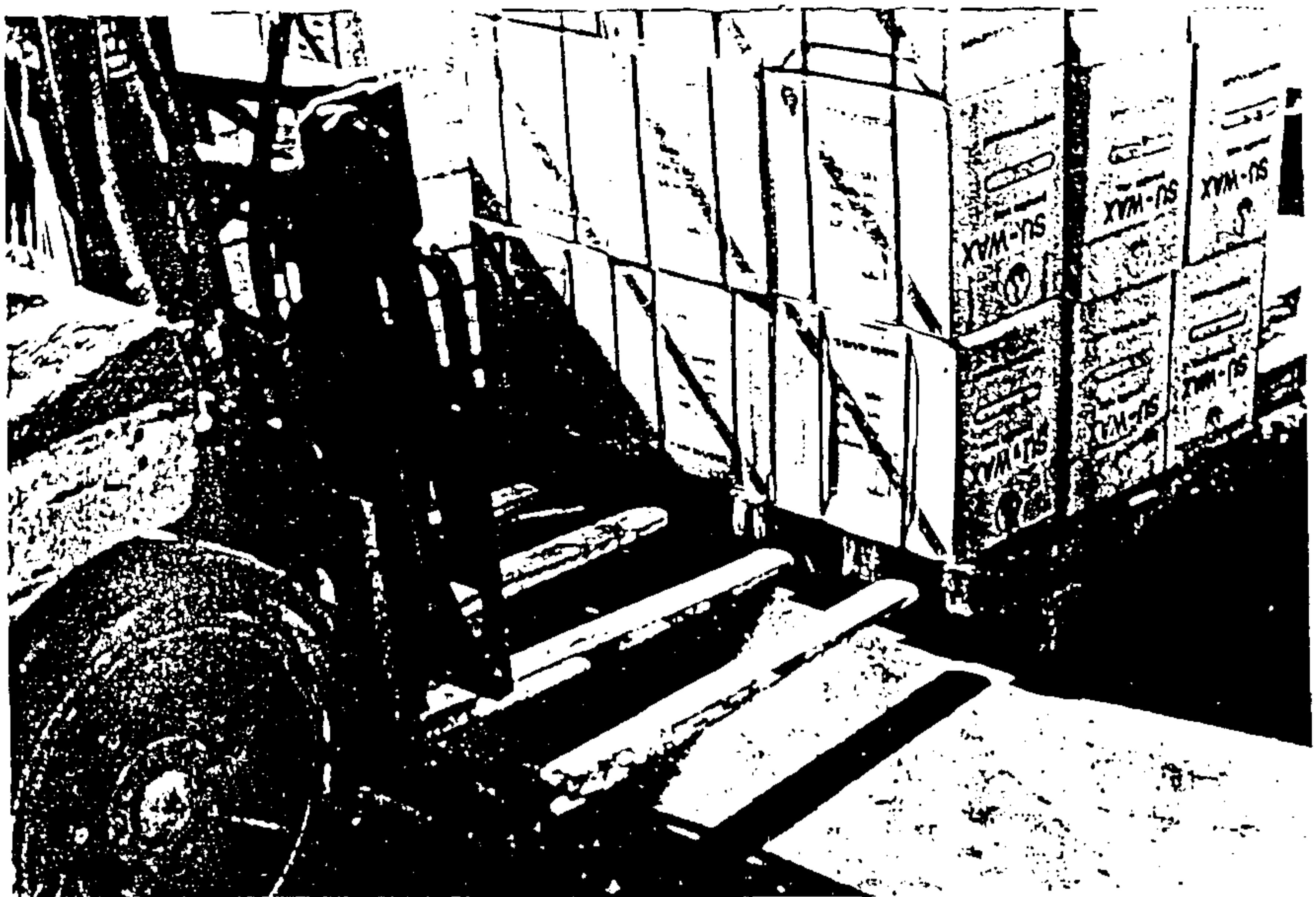
Рис. 502. ЗК. 1. Захват "подъема" с гребенчатого поддона погрузчиком с многовилочным захватом. Порт Ленинград.
