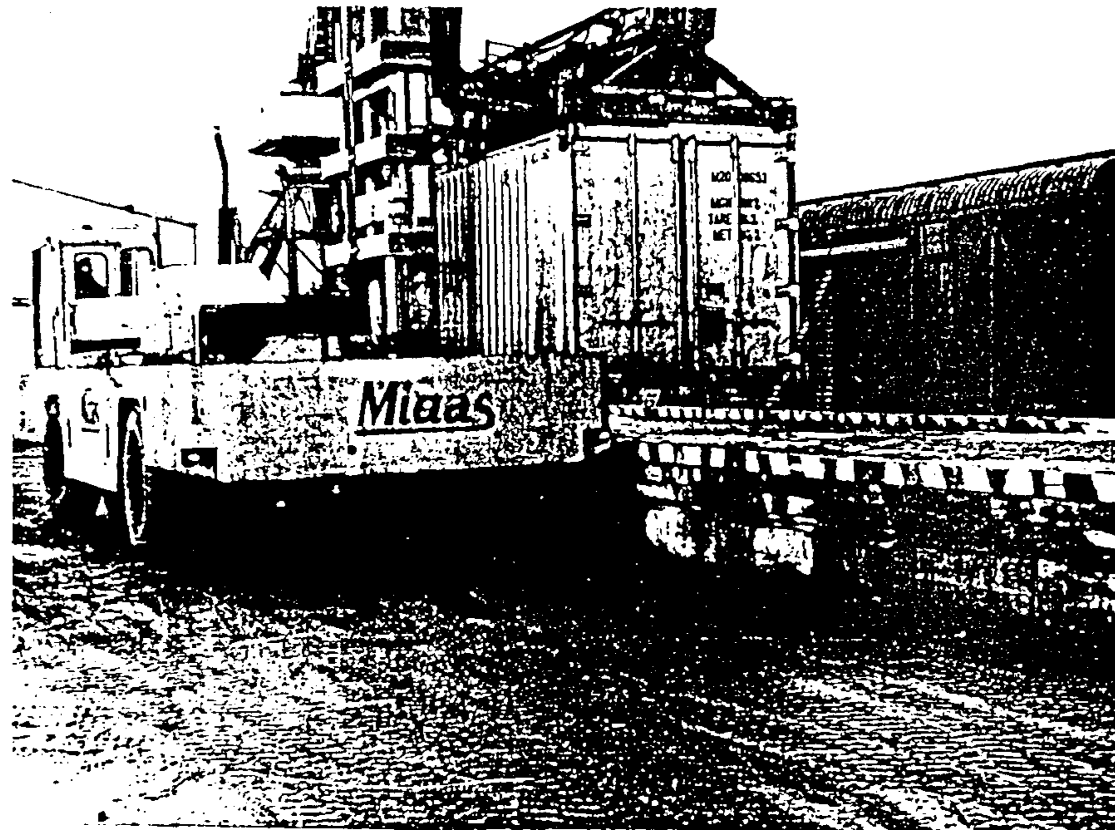
Рис. 3.2. Установка контейнера контейнерным автопогрузчиком на стационарную рампу. Порт Рига.
