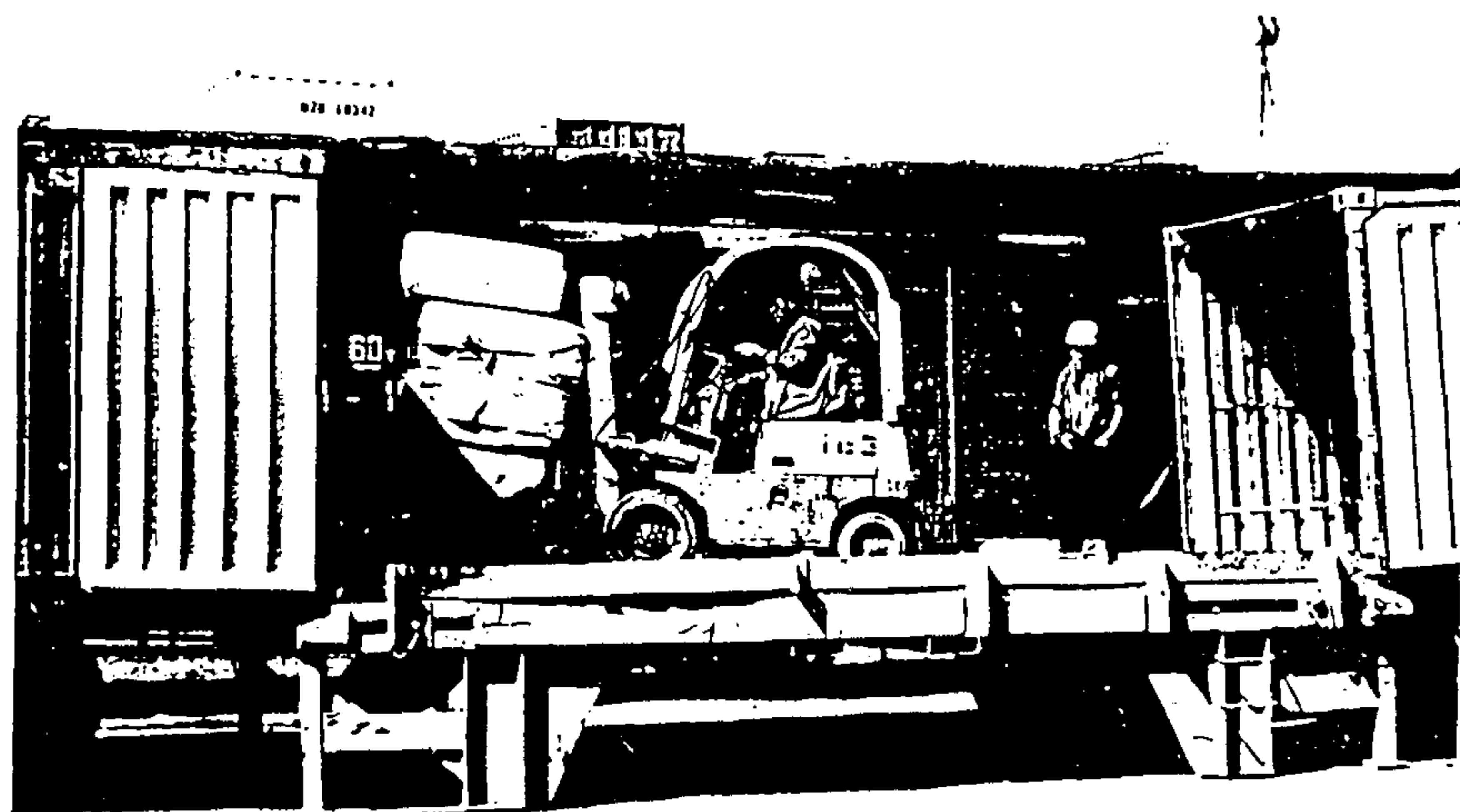
Рис. 205.5К.1. Перегрузка целлюлозы в кипах из вагона в контейнер погрузчиком с боковым захватом типа УЗРС. Порт Ильичевск.
