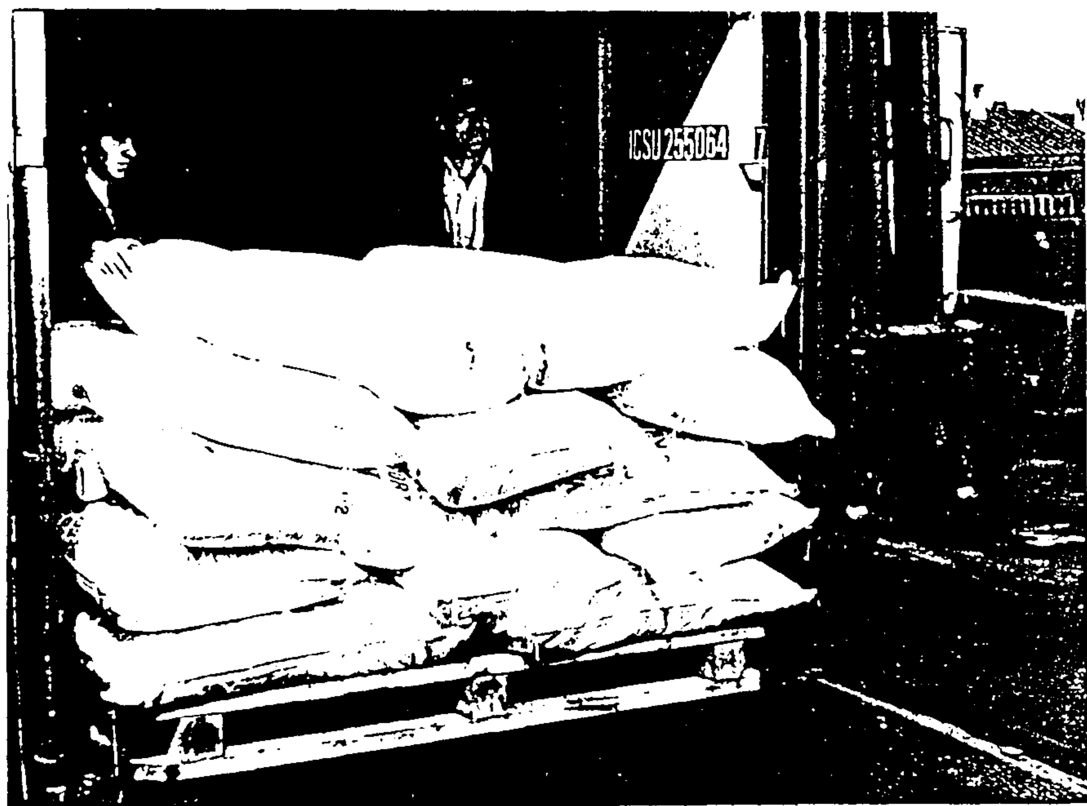
Рис. 102.ЗК.2. Формирование пакета груза на плоском поддоне. Порт Ленинград.
