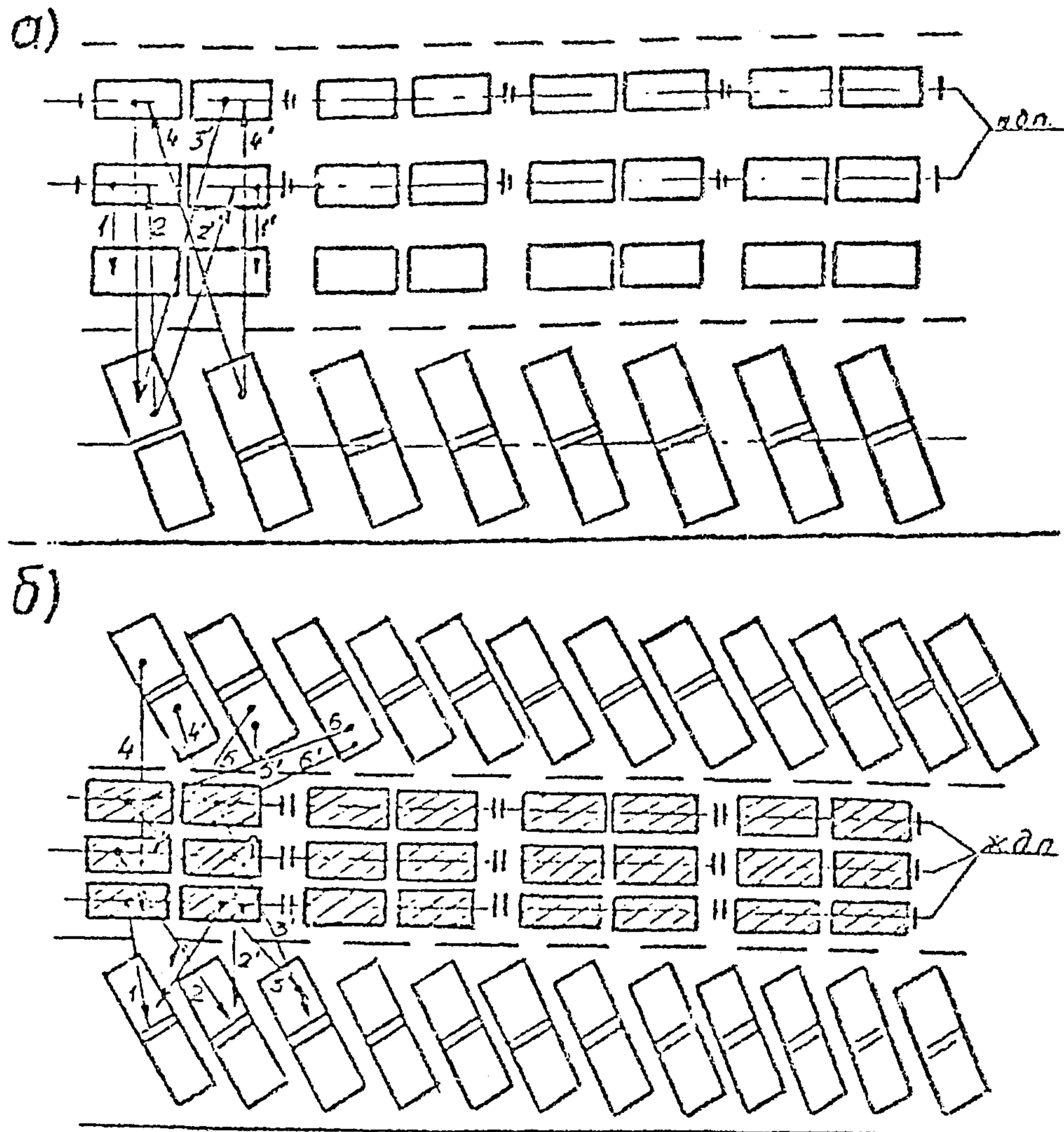
Рис. 7.01б2 Схема обработки подач при использо- вании портальных погрузчиков → без одновременного вывоза - подвоза контейнеров при одноконсольном (а) и двухконсольном (б) козловых кранах
