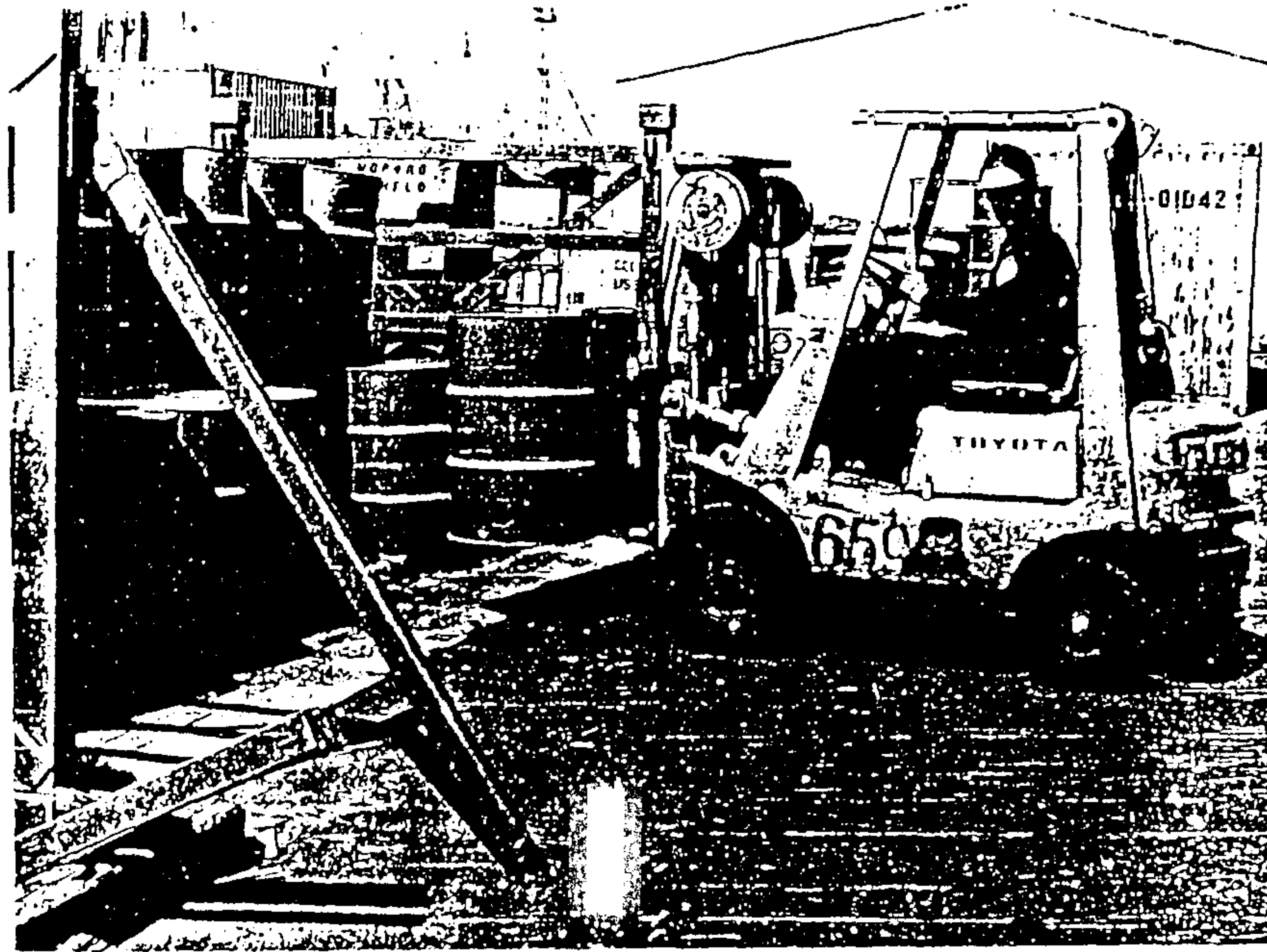
Рис. 301. КШ. I. Загрузка контейнер-платформы грузами в бочках погрузчиком с захватом ЗГБ-I. Порт Рига.
