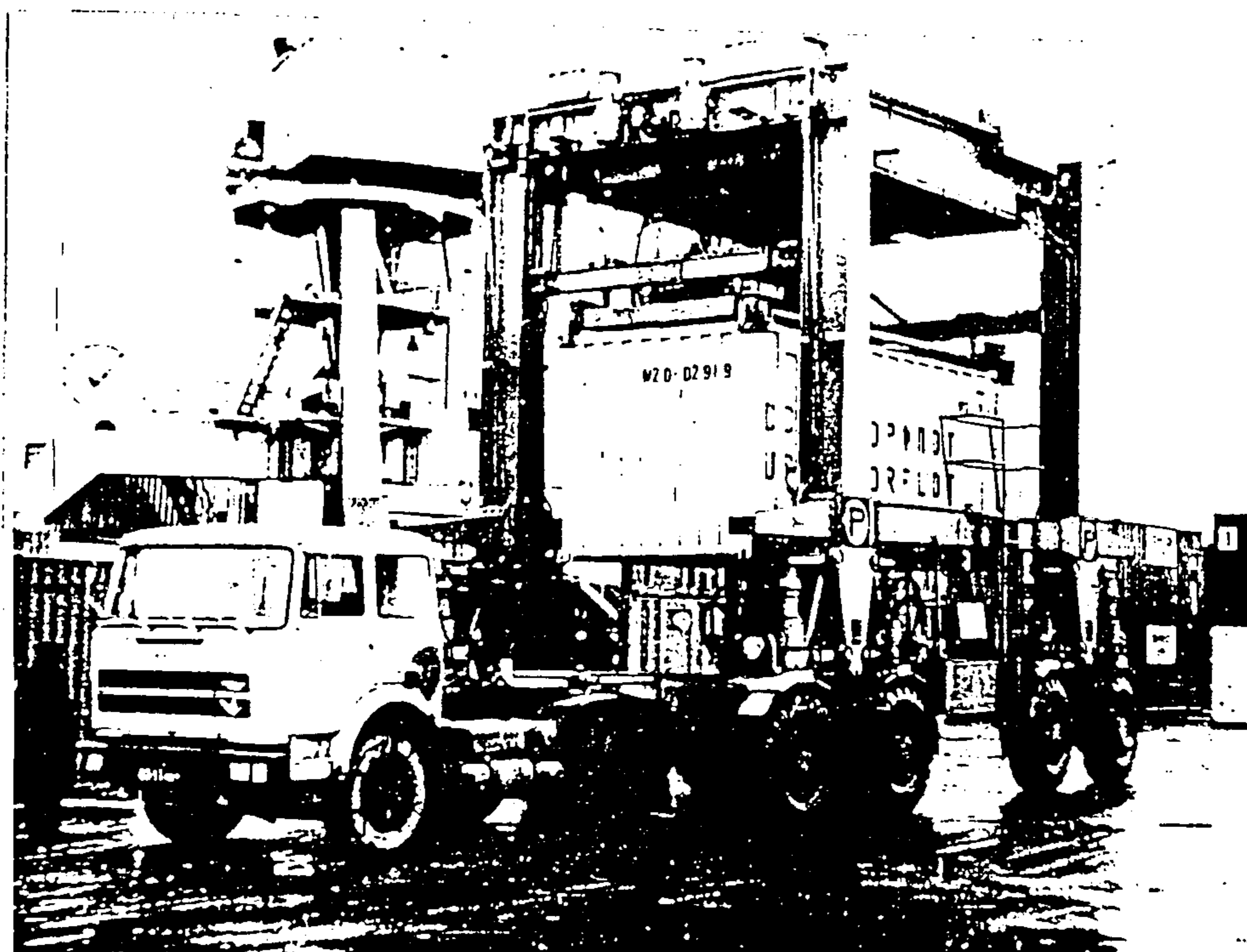
Рис.70Гр.2. УСТАНОВКА КОНТЕЙНЕРОВ НА КОНТЕЙНЕРНУЮ ТЕЛЕЖКУ ПОРТАЛЬНЫМ ПОГРУЗЧИКОМ. ПОРТ ЛЕНИНГРАД
