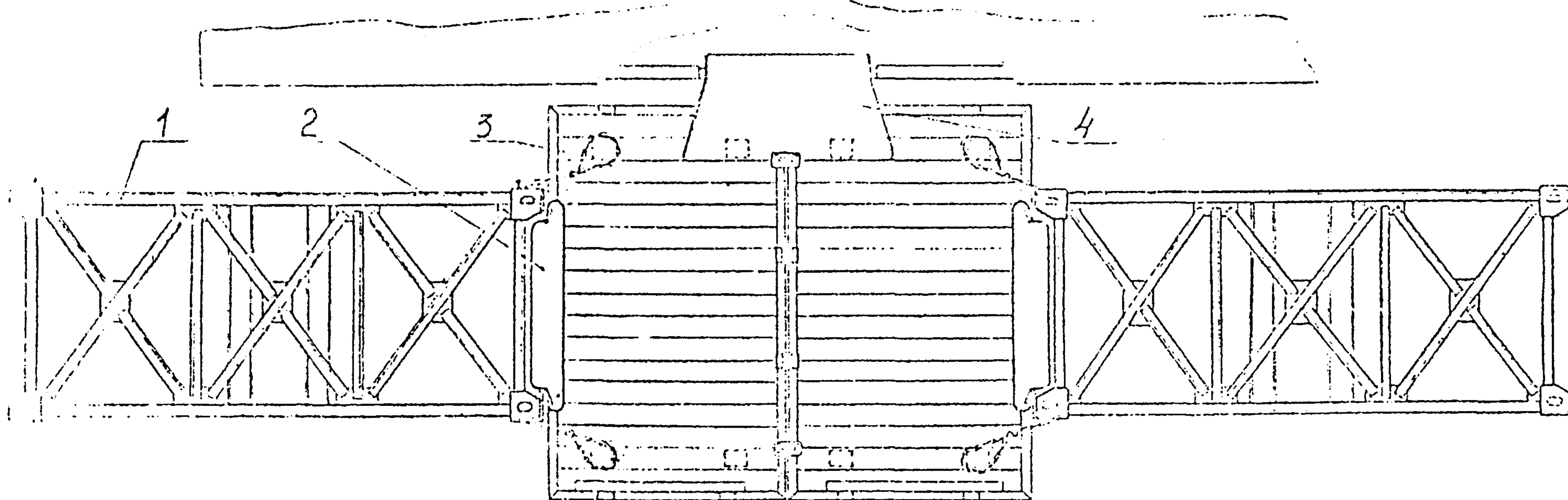
Рис. 3.3. Схема установки контейнеров у вагона при перегрузке грузов по прямому варианту вагон-контейнер и обратно: 1 - стол-приставка; 2 - трап перекидной контейнерный; 3 - грузовой стол; 4 - трап вагонный; 5 - контейнер; 6 - вагон.
