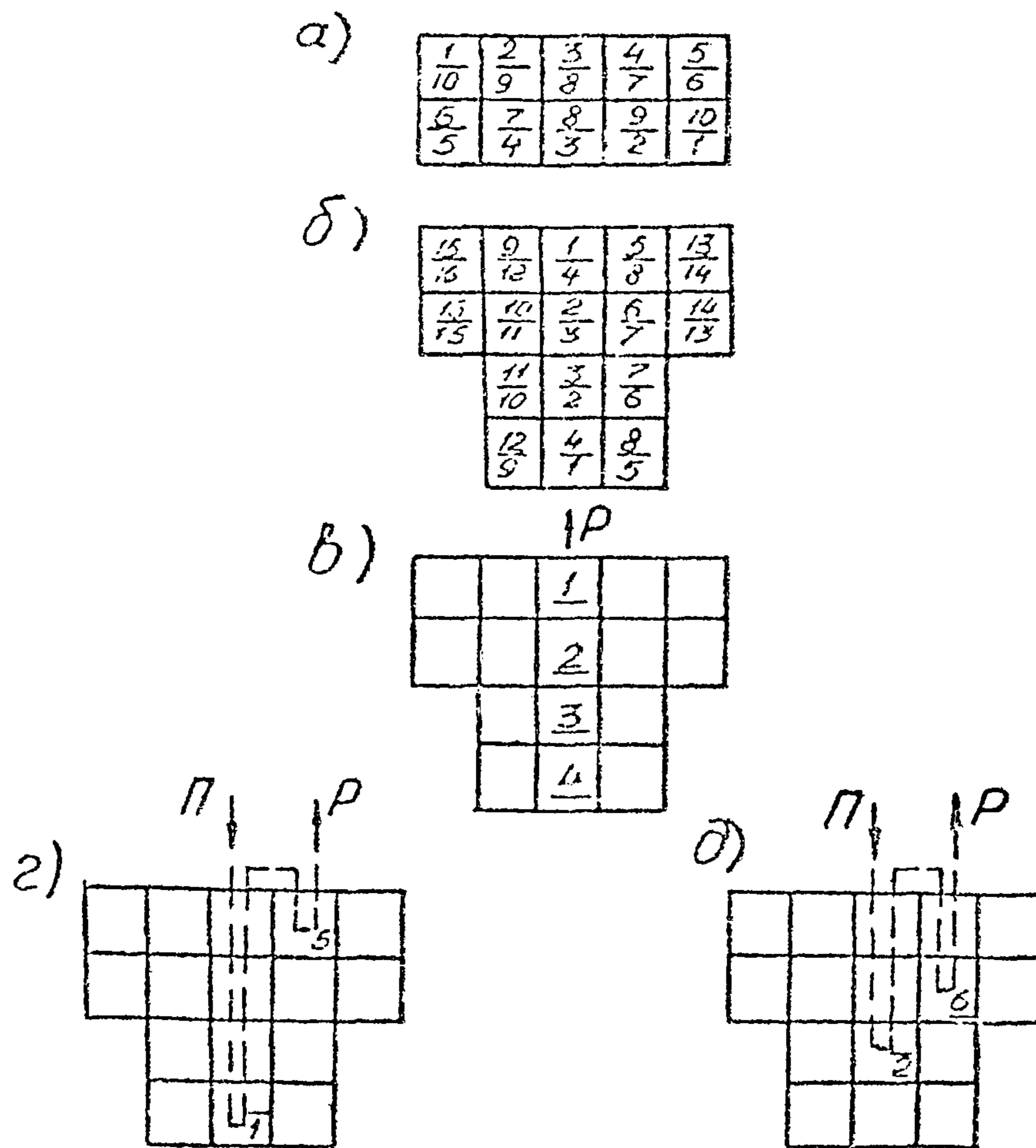
Рис. 7.01в.4 Последовательность разгрузки и загрузки контейнеров в секции судна а - палуба и б - трюм по простому циклу (числитель - последовательность раз- грузки, знаменатель - последовательность загрузки); в, г, д. - трюм по сложному циклу (Р - разгрузка, П - загрузка)
