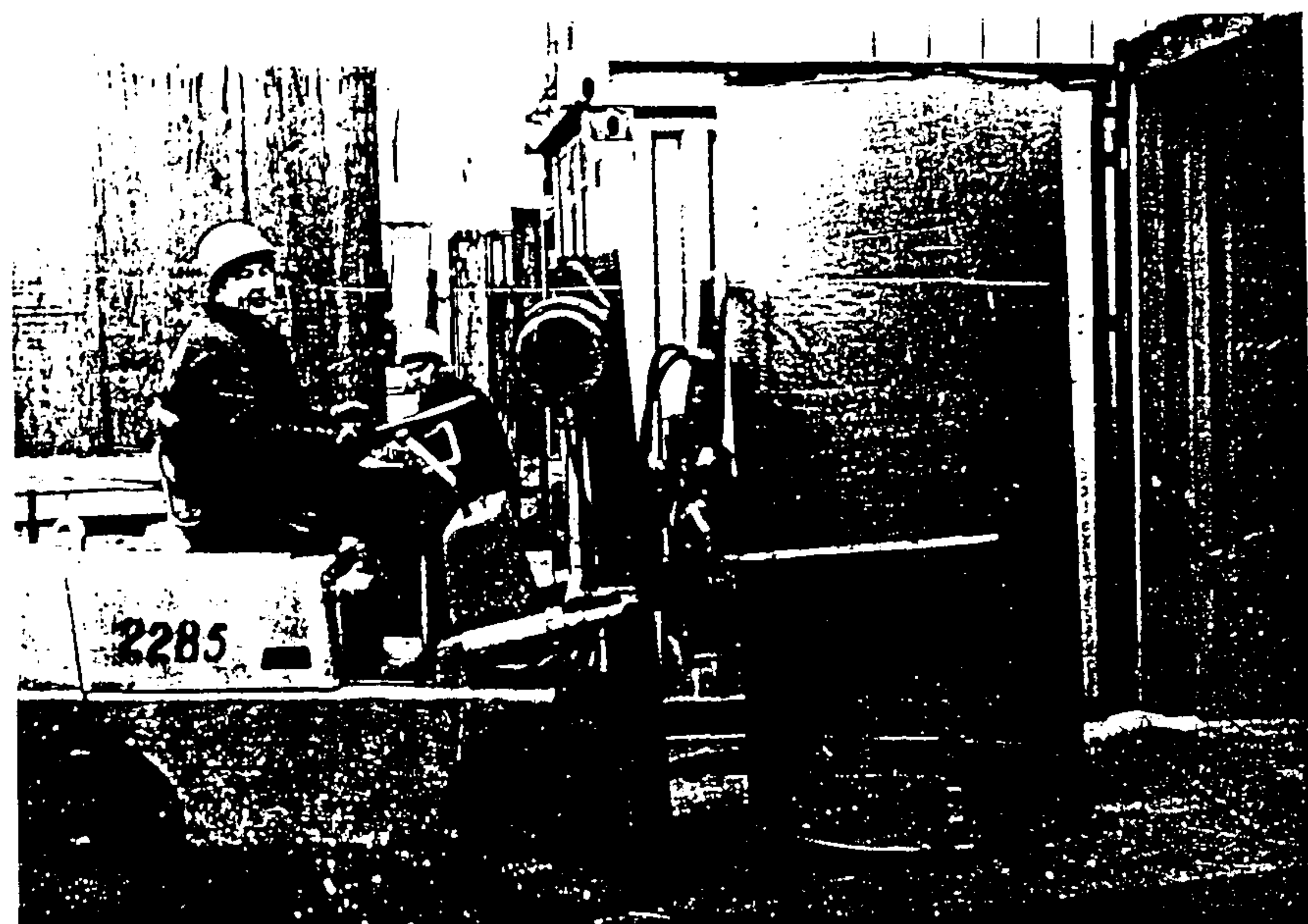
Рис. 401. ЭК. I Загрузка контейнера бумагой в рулонах погрузчиком с боковым захватом типа УЗРС. Порт Ленинград.
