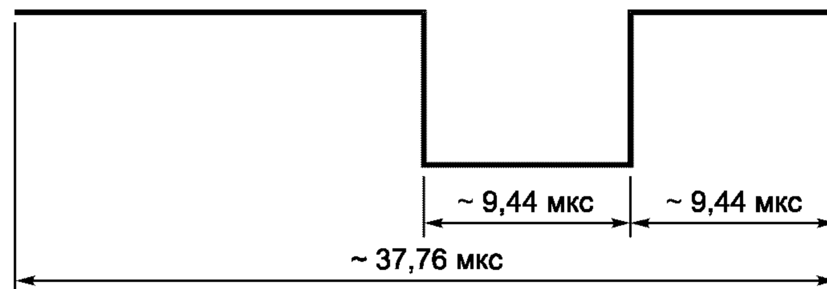
Рисунок 9 — Конец кадра при любом способе кодирования
