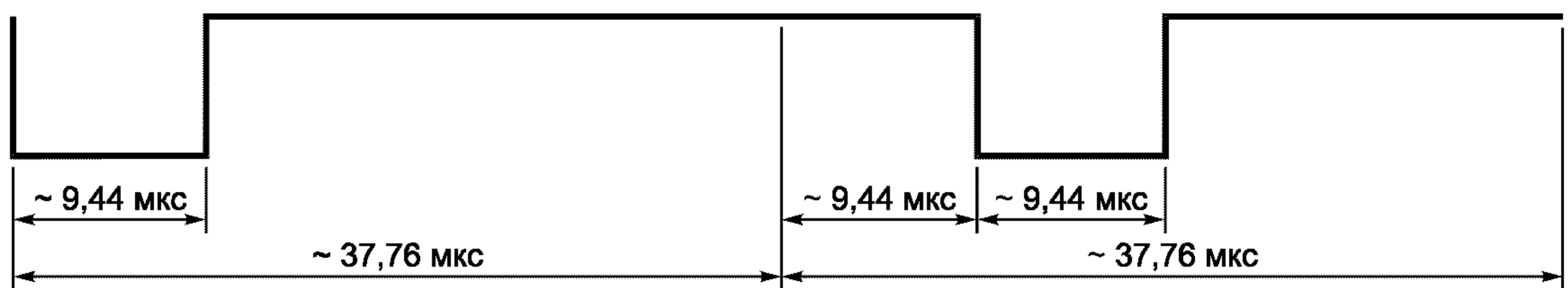
Рисунок 8 — Начало кадра при способе кодирования «1 из 4»
