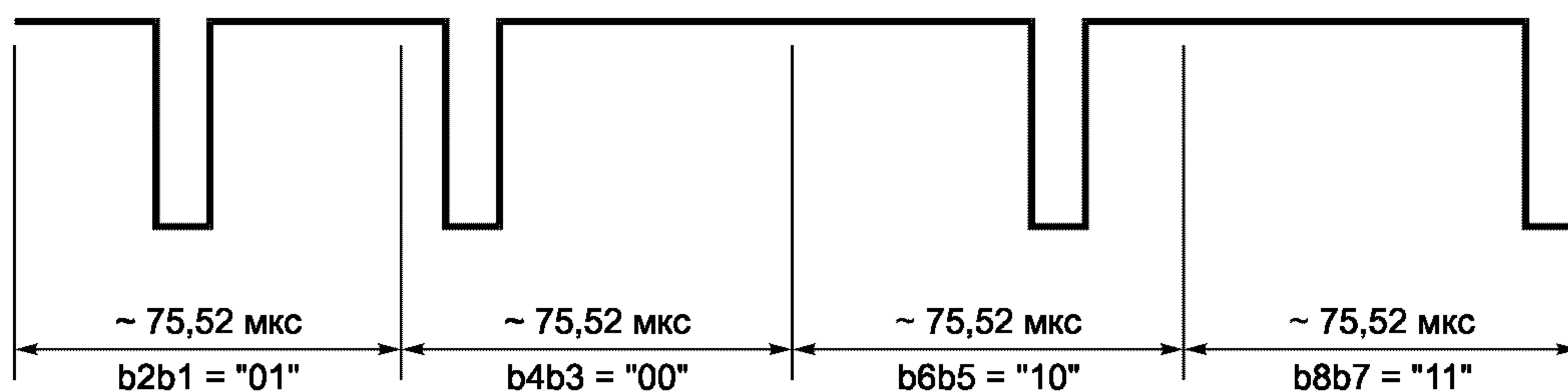
Рисунок 6 — Пример кодирования способом «1 из 4»
