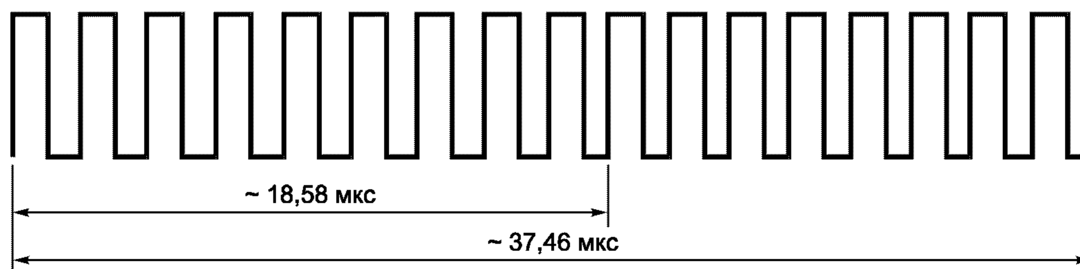
Рисунок 13 — Логическая единица
