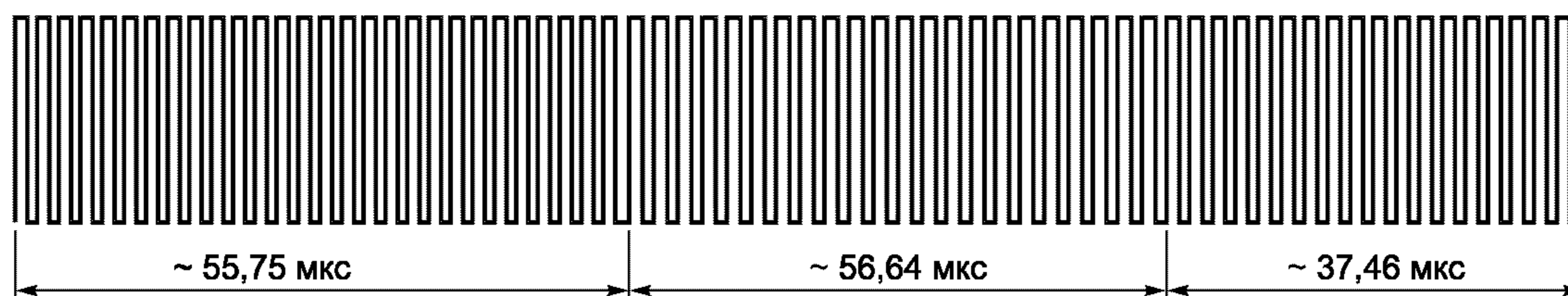
Рисунок 15 — Начало кадра при использовании двух поднесущих
