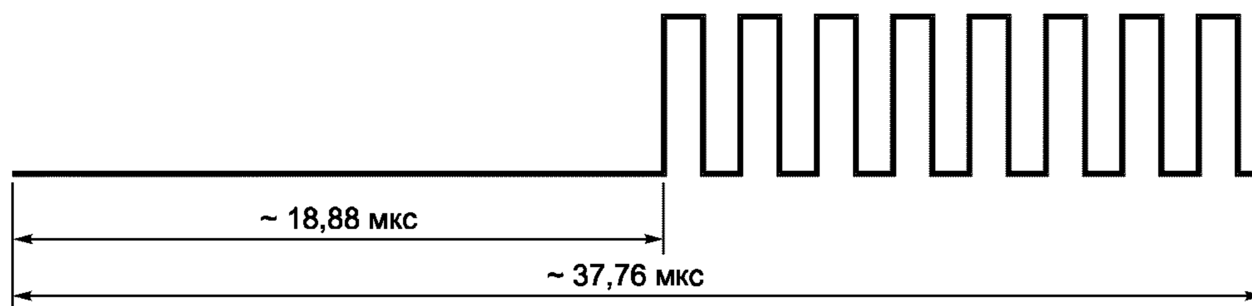
Рисунок 11 — Логическая единица
