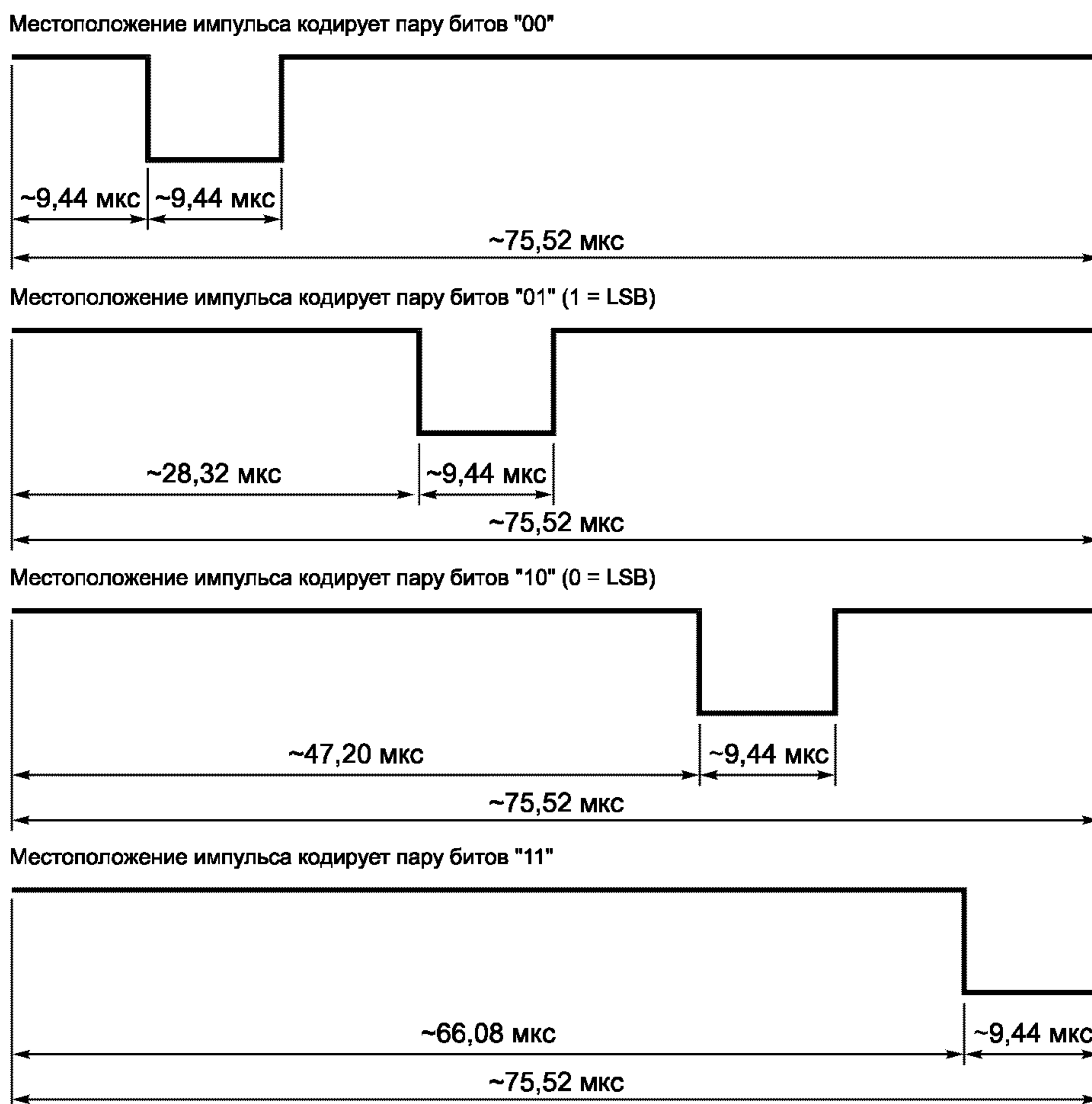
Рисунок 5 — Способ кодирования «1 из 4»
