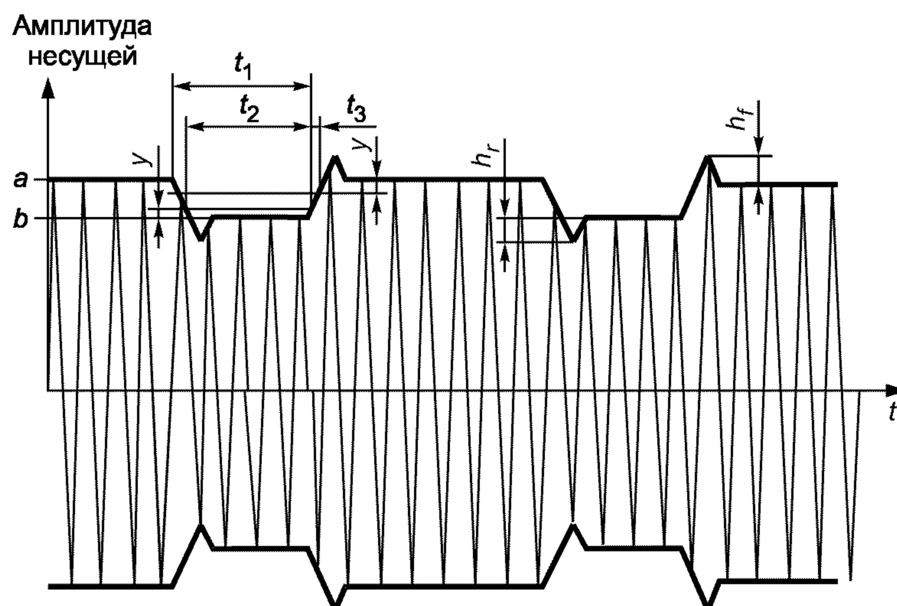
Рисунок 1 — Модуляция несущей для случая 100 % ASK
