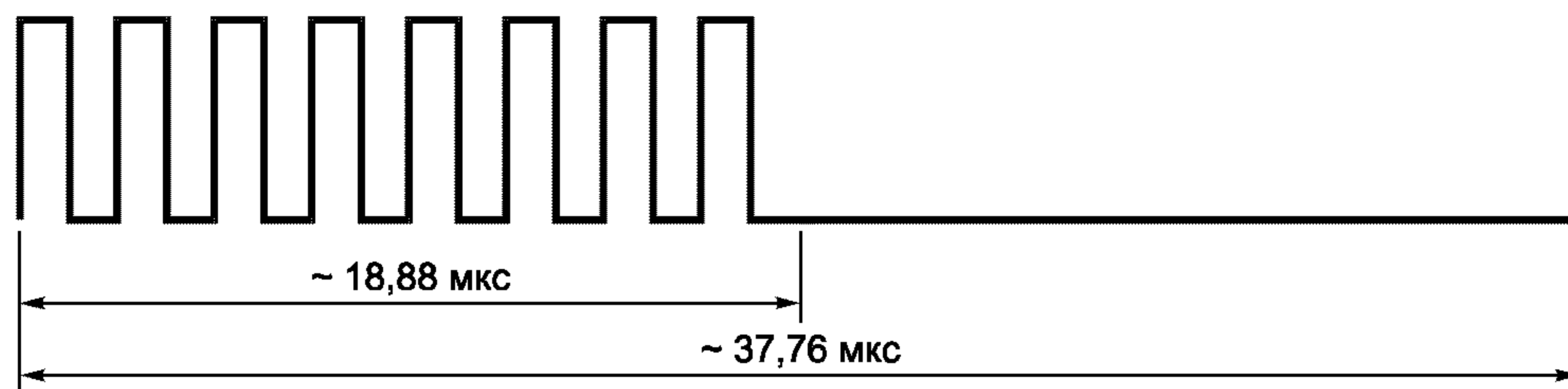
Рисунок 10 — Логический ноль
