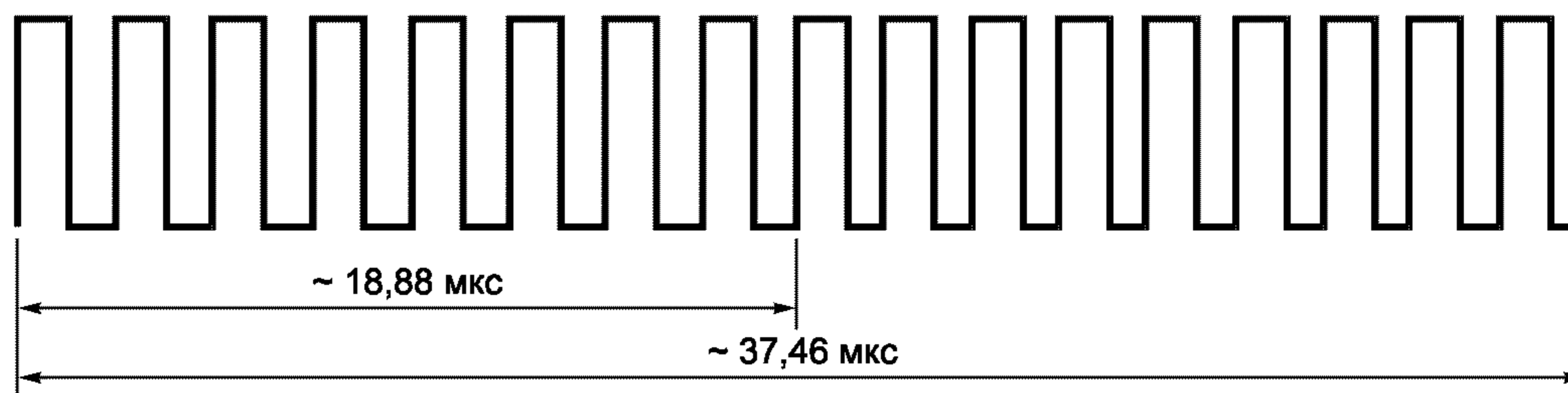
Рисунок 12 — Логический ноль
