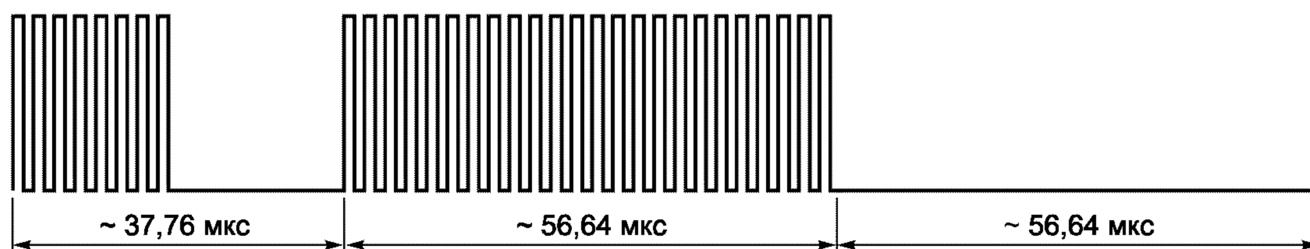
Рисунок 16 — Конец кадра при использовании одной поднесущей
