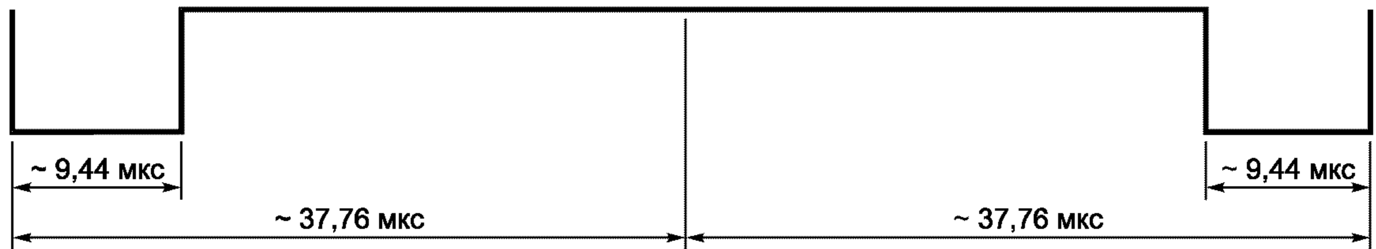
Рисунок 7 — Начало кадра при способе кодирования «1 из 256»
