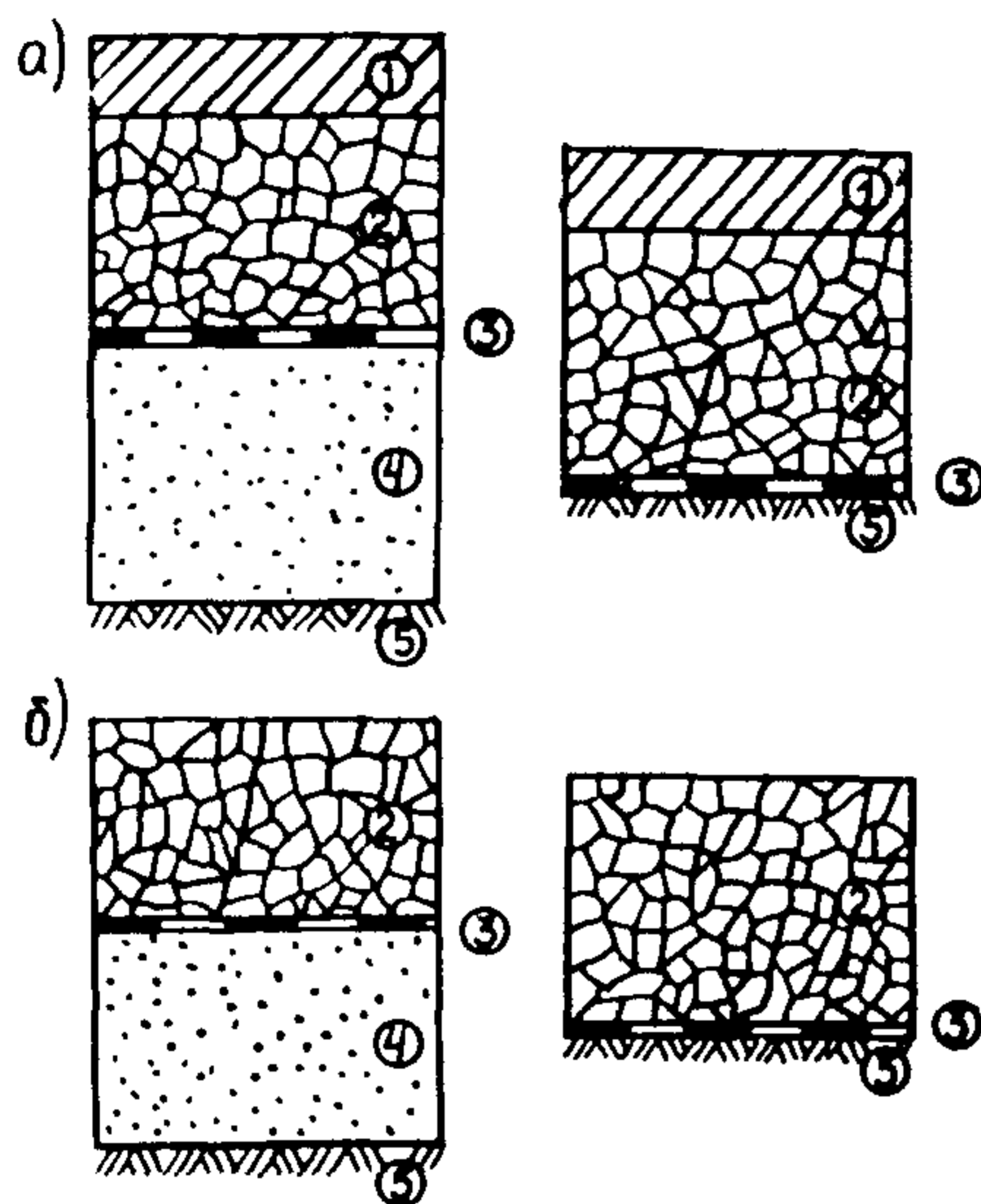
Рис.1. Конструкции армированных дорожных одежд усовершенствованного (а) и переходного (б) типов: 1-слои (слой) асфальтобетона; 2-щебеночный слой основания (покрытия); 3-армирующая сетка; 4-песчаный подстилающий слой; 5-грунт земляного полотна
