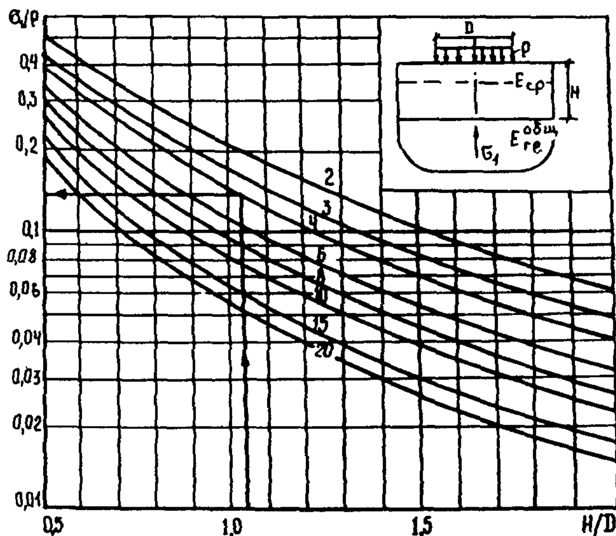
Рис.2. Номограмма для определения вертикального главного напряжения на уровне сетки (цифры на кривых - E_{cp}/E_{гр}^0 )
