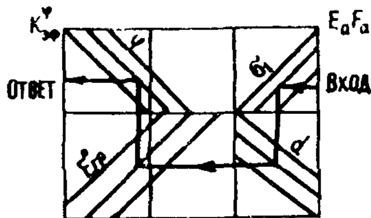
Рис.3. Номограмма для определения коэффициента эффективности армирования K_{эф}^{\psi} — средняя крупность зерен материала основания (покрытия) в зоне контакта с подстилающим грунтом, определяемая как среднее арифметическое между верхним и нижним пределами фракции щебня, мм; \psi — угол внутреннего трения грунта, подстилающего щебеночный слой, град.
