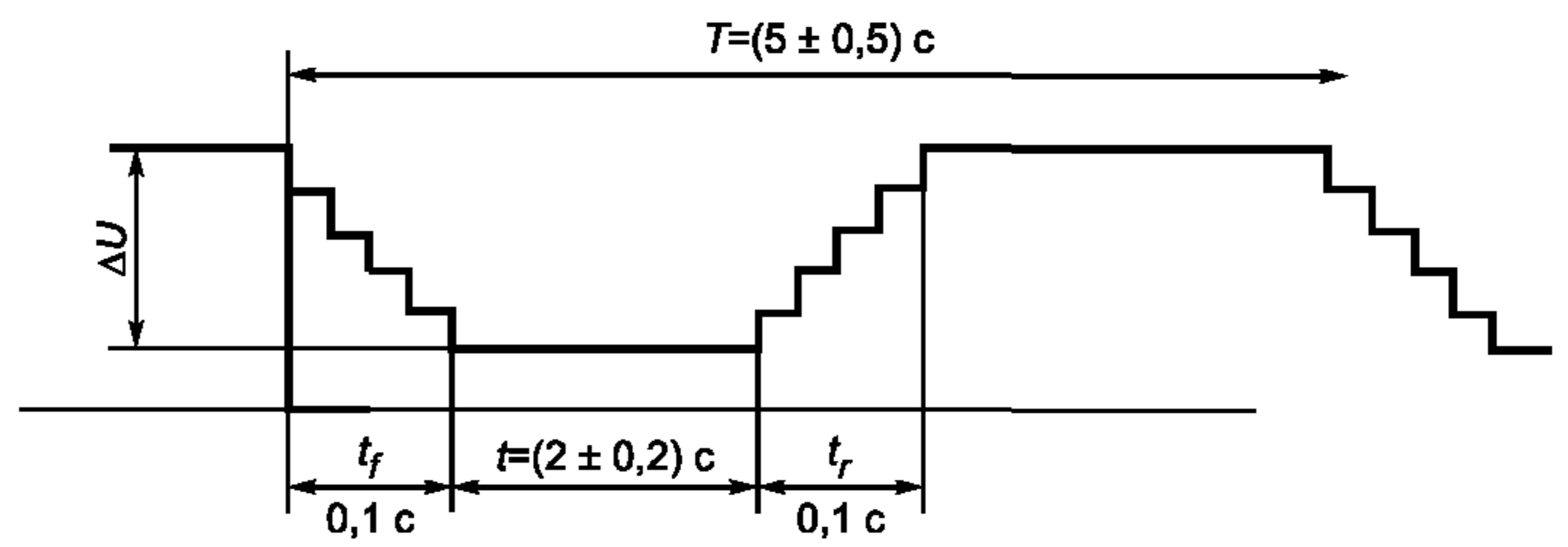
Рисунок 1б — Определение времени спада t_f и времени возрастания t_r при формировании ступенчатых изменений напряжения
