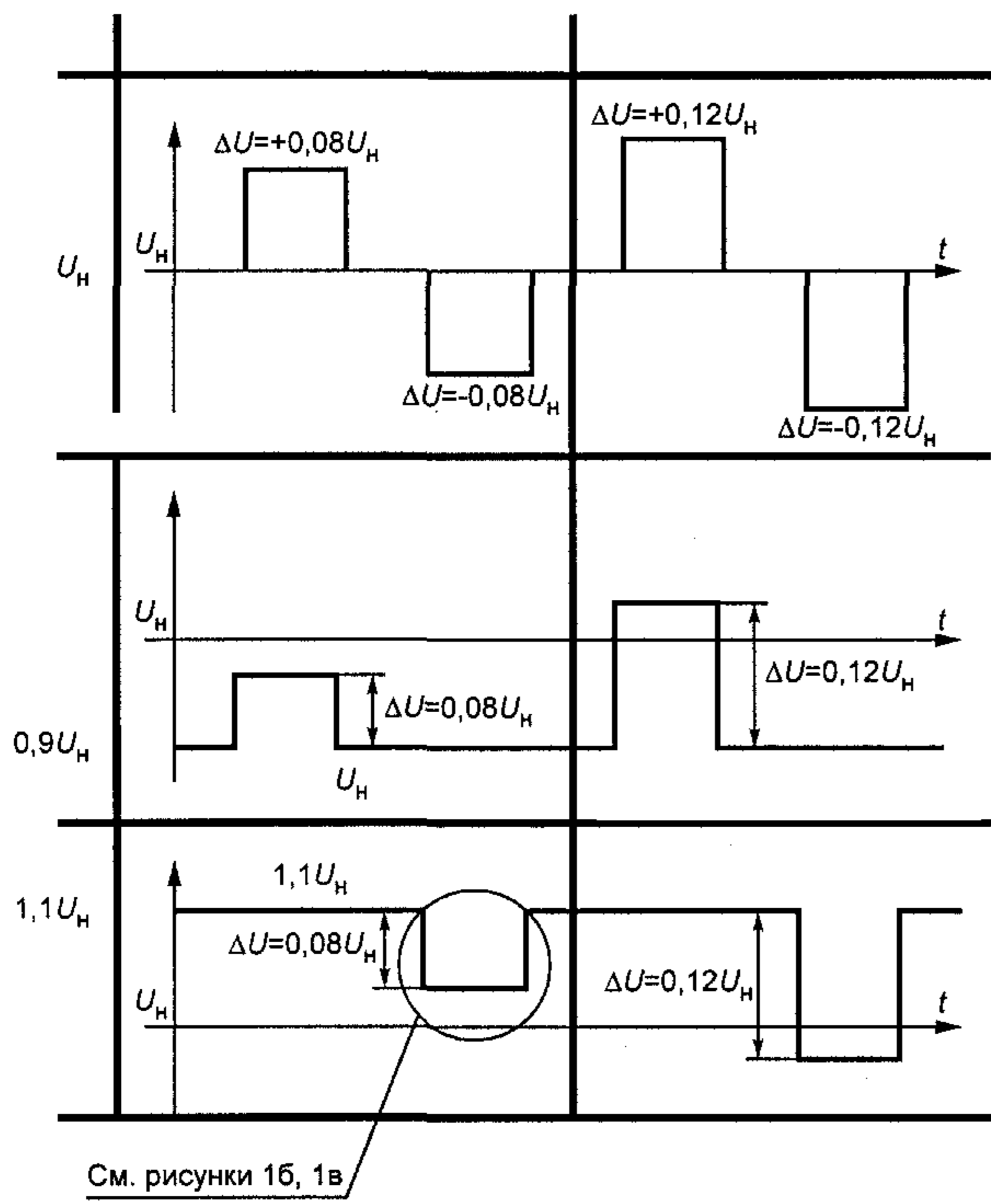
Рисунок 1а — Диаграмма колебаний напряжения
