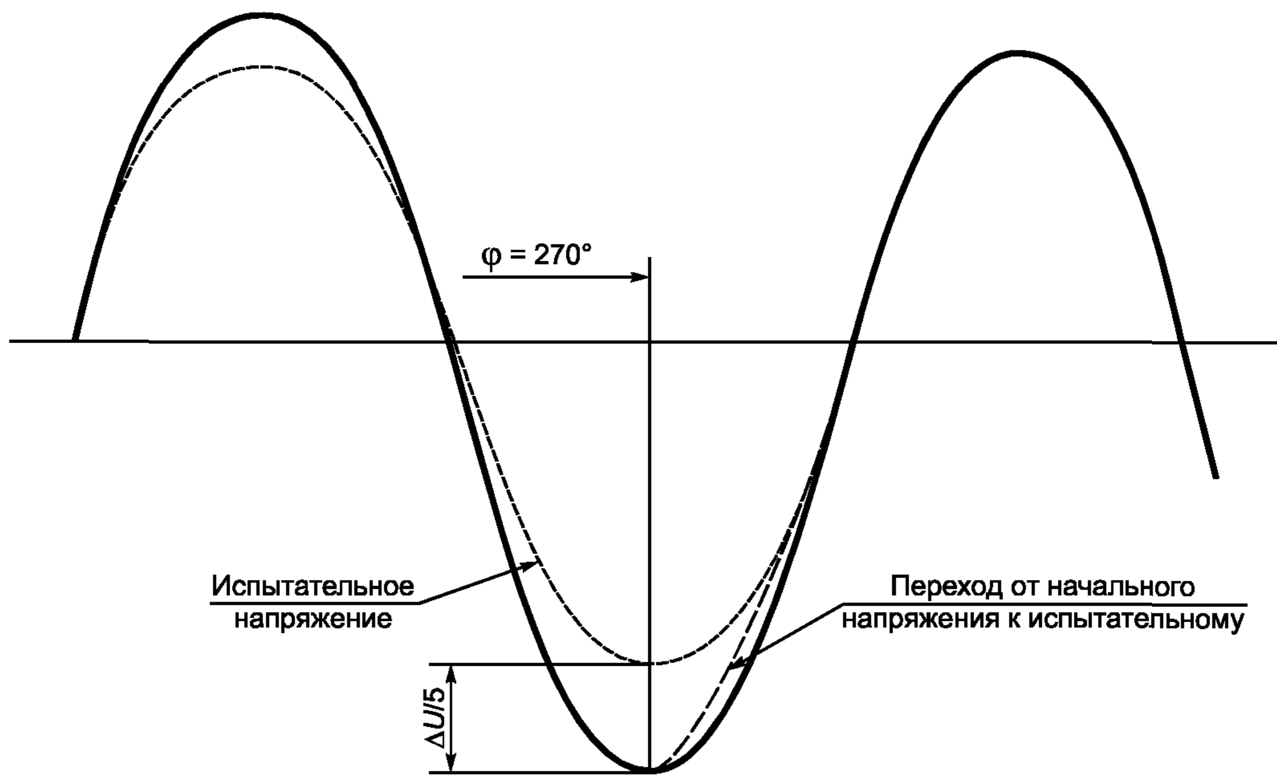
Рисунок 1в — Изменение напряжения в течение 0,25 периода при образовании t_f и t_r
