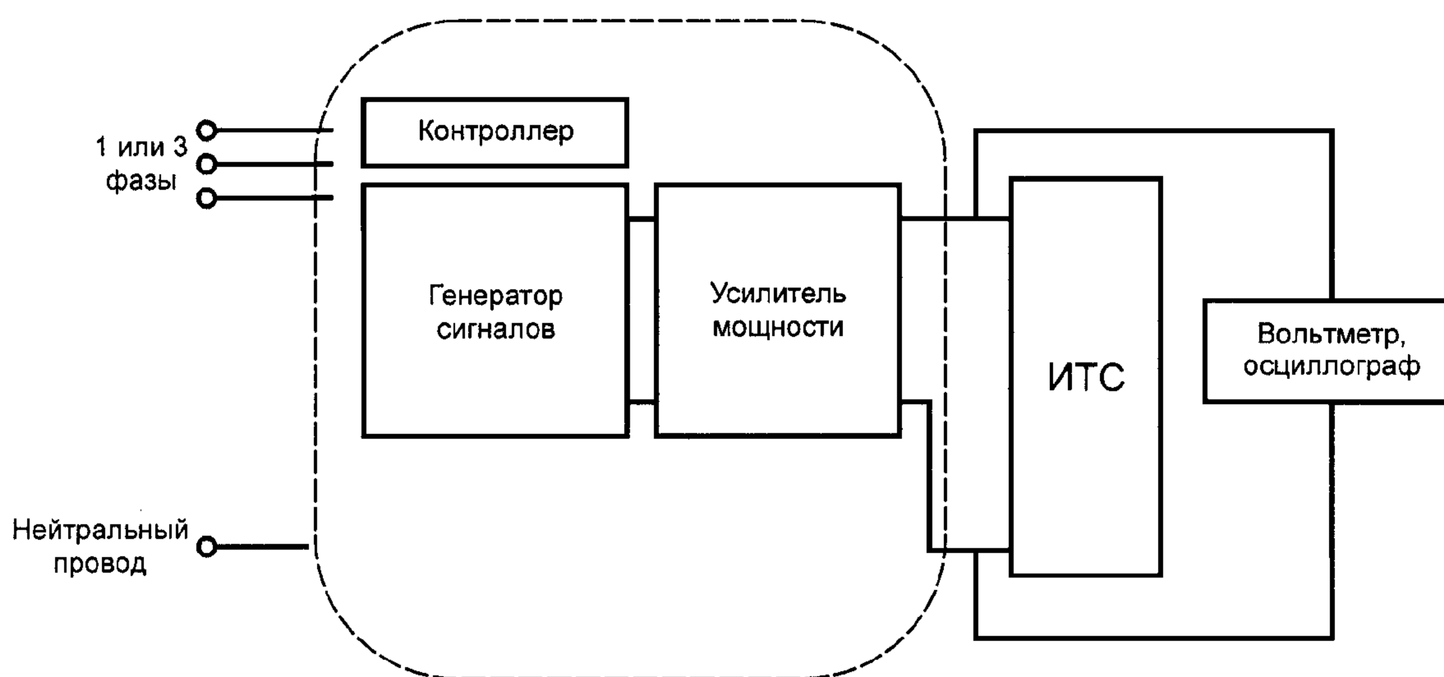
Рисунок 3 — Схема испытательного оборудования с усилителем мощности
