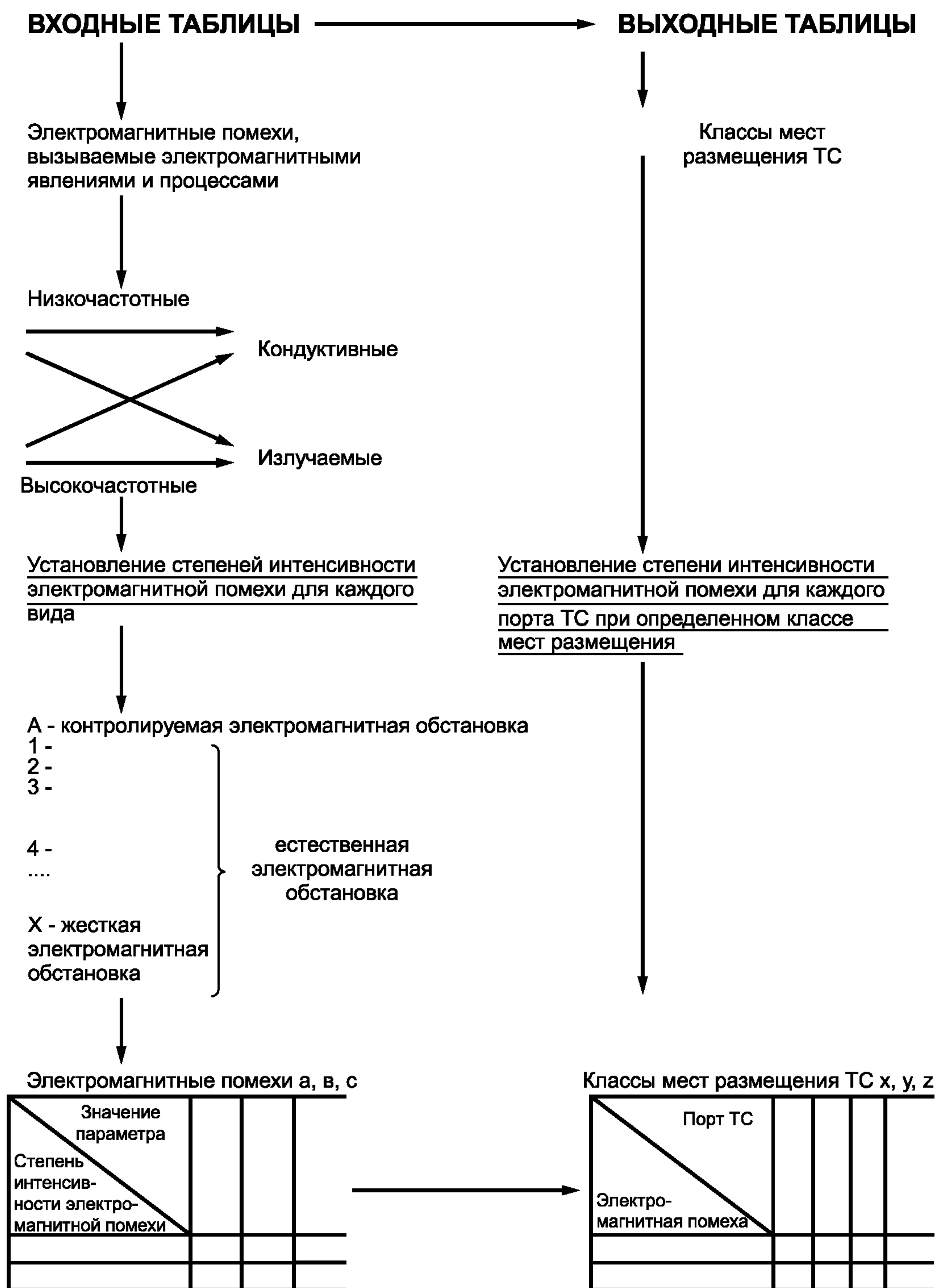
Рисунок 1 — Принципы классификации электромагнитной обстановки
