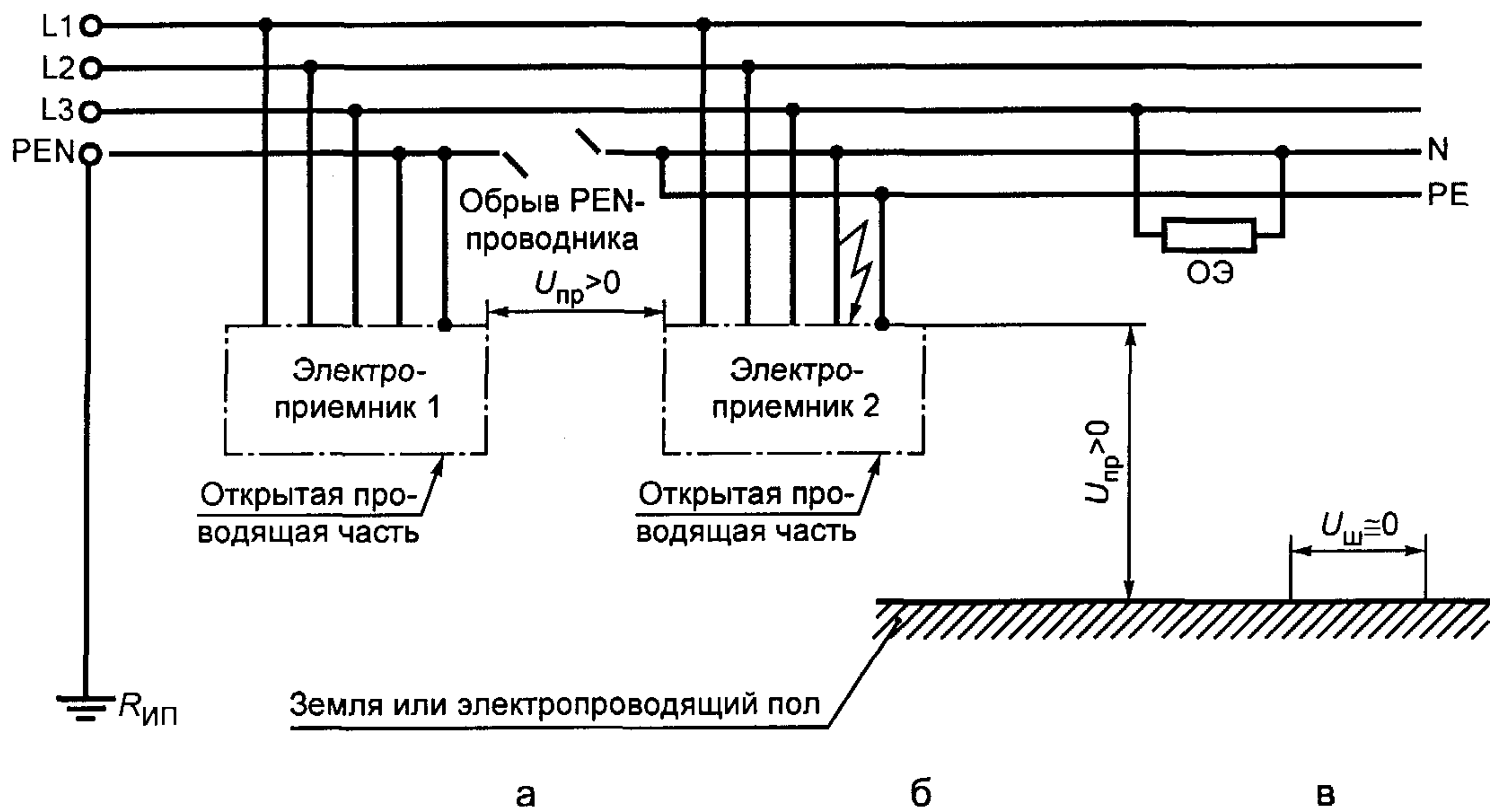
Рисунок В.7 — Сеть TN-C-S с обрывом PEN-проводника
