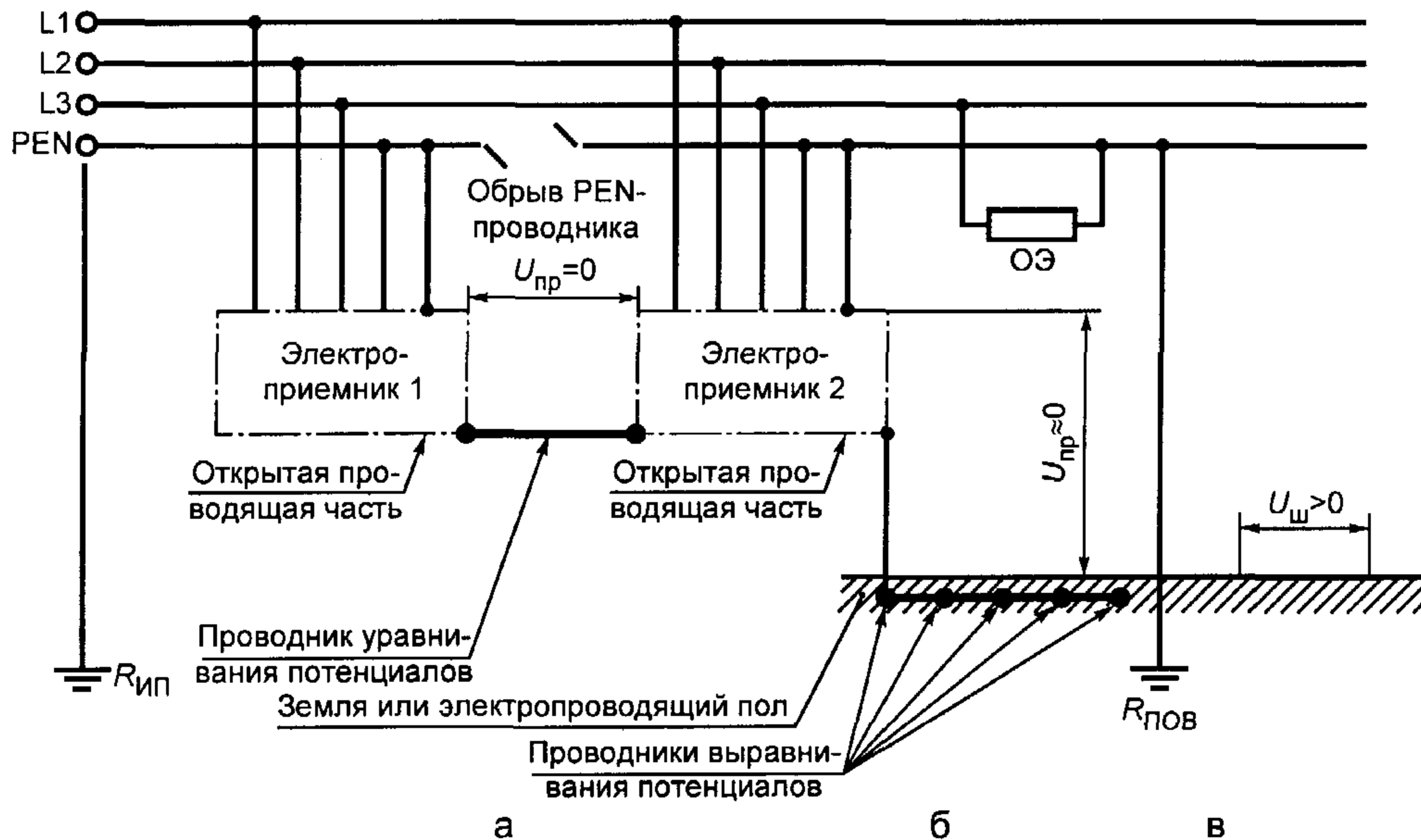
Рисунок В.2 — Сеть TN-C с оборванным PEN-проводником
