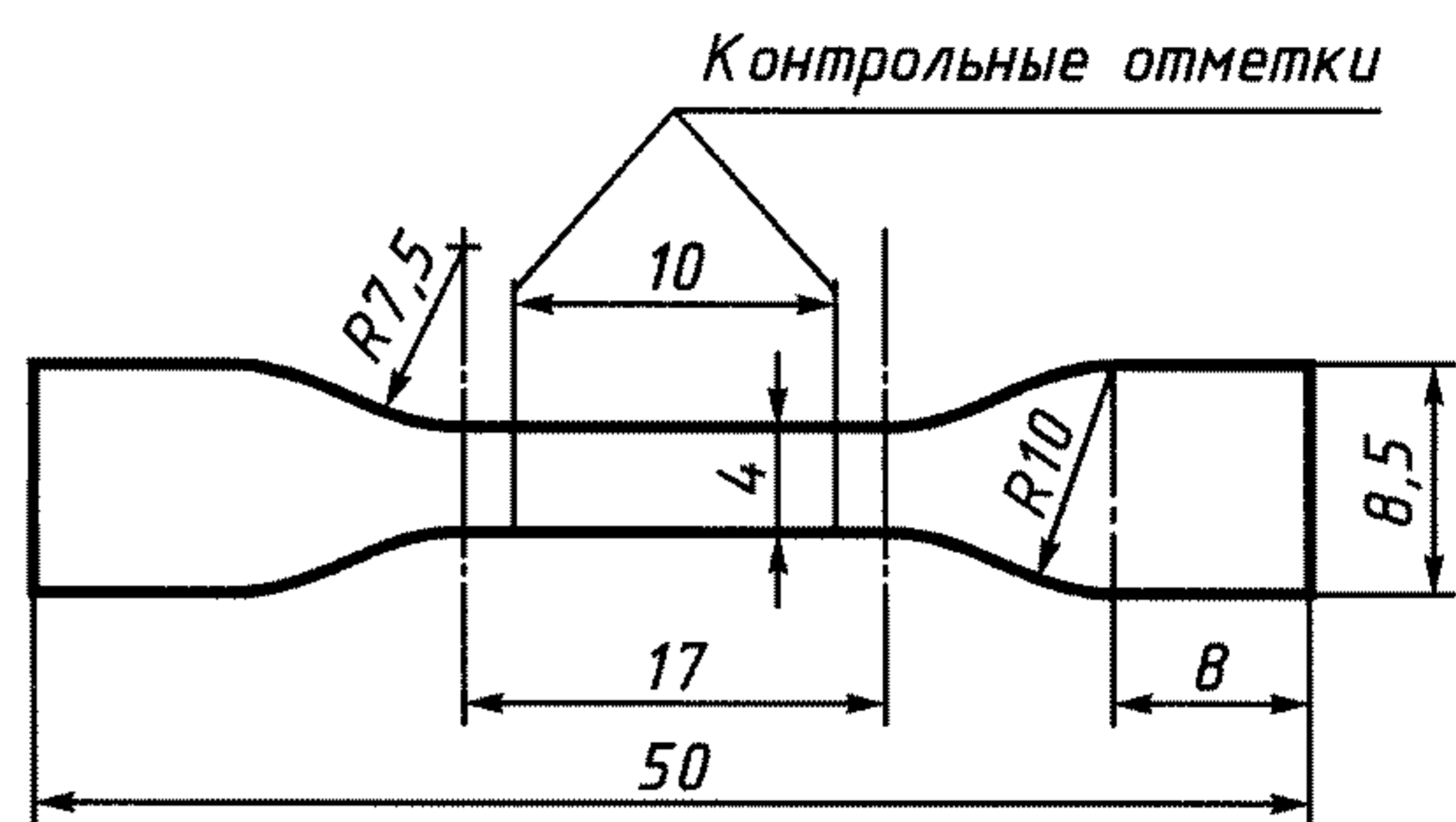
Рисунок 13 — Образец в виде двусторонней лопатки уменьшенного размера
