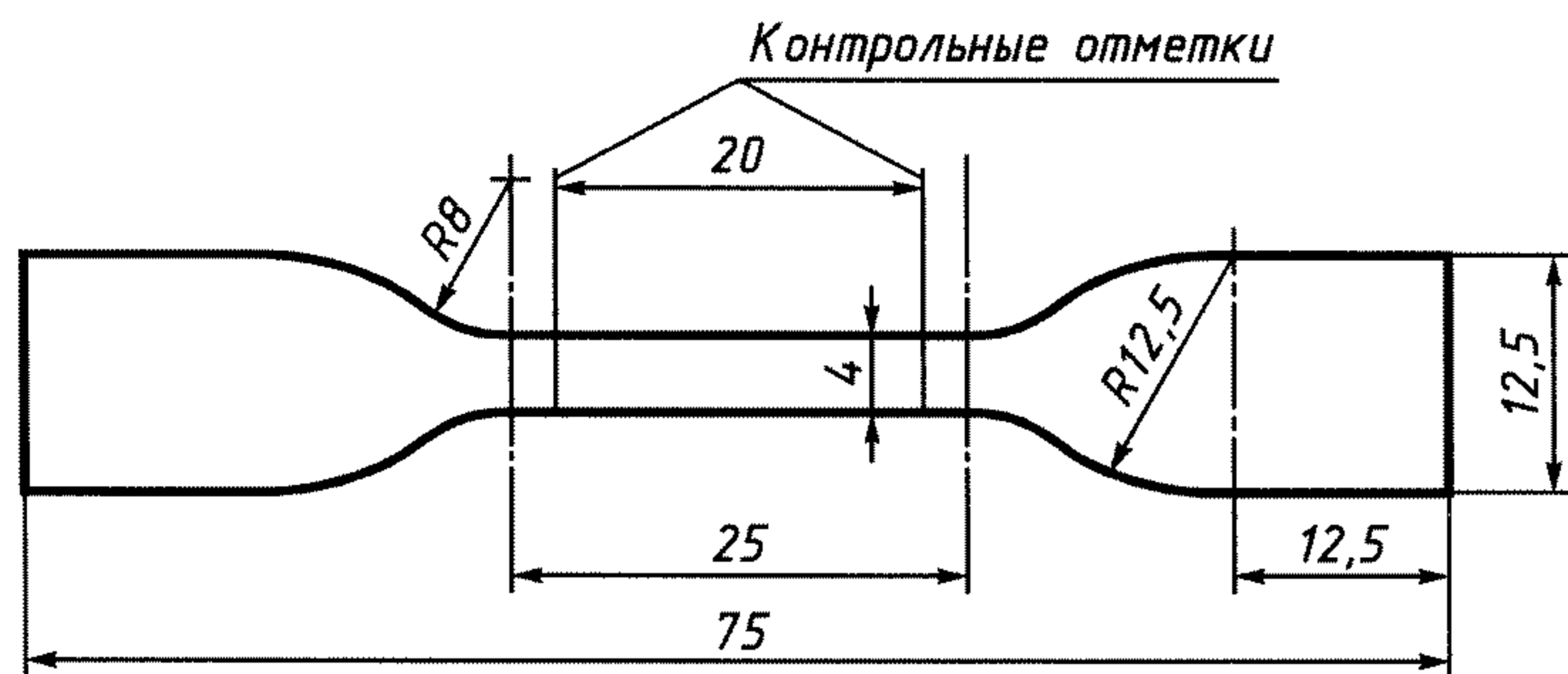
Рисунок 12 — Образец в виде двусторонней лопатки
