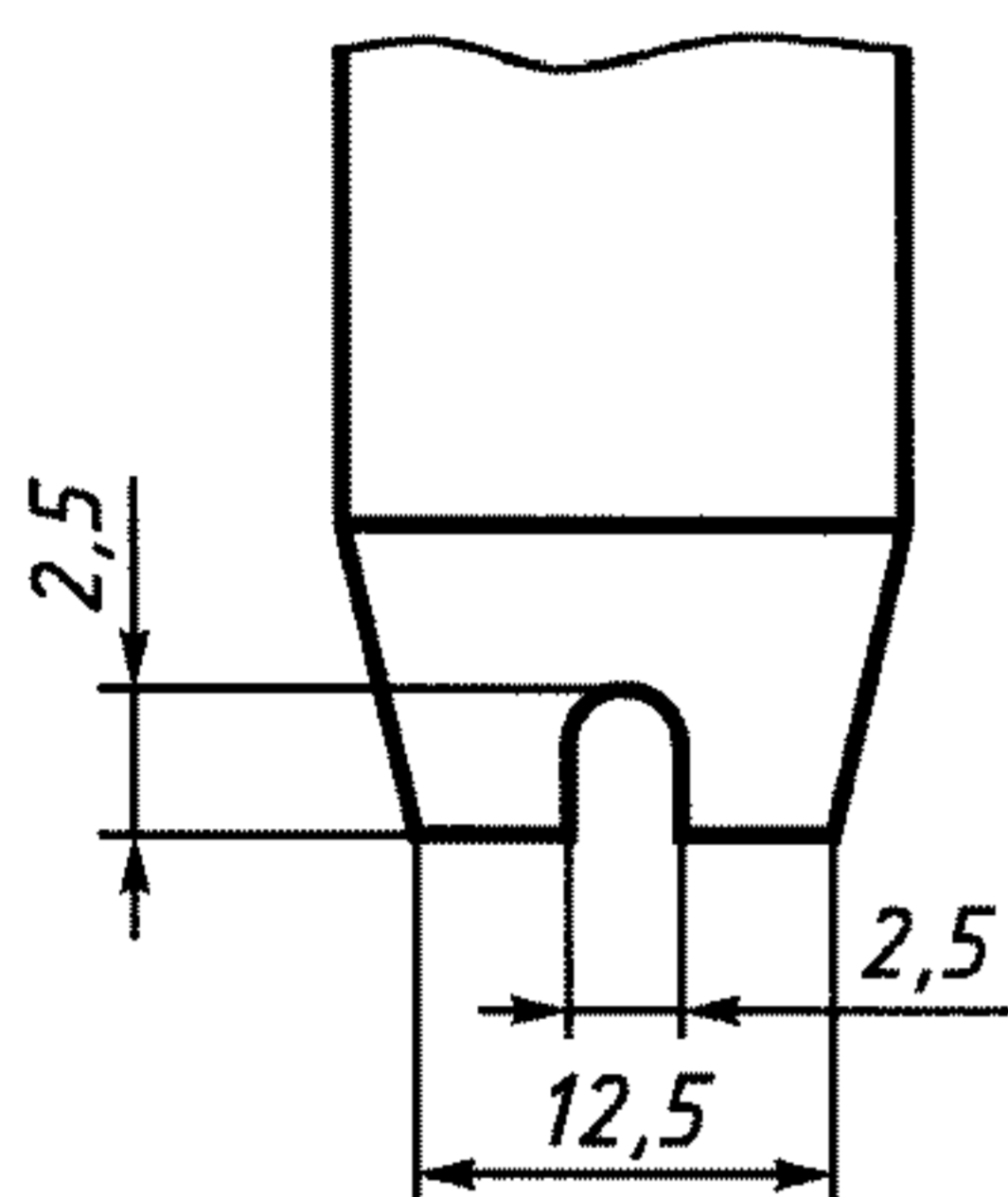
Рисунок 14 — Конец вырубного ножа с выемкой
