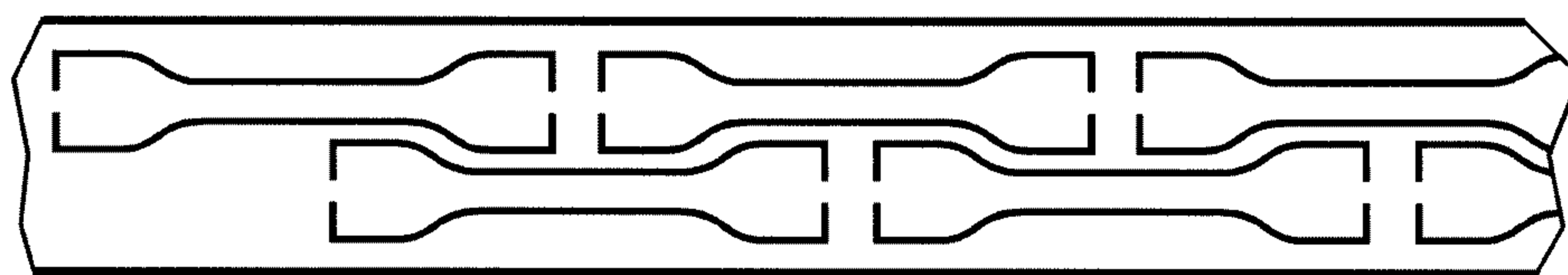
Рисунок 15 — Образцы, вырубленные ножом с выемкой
