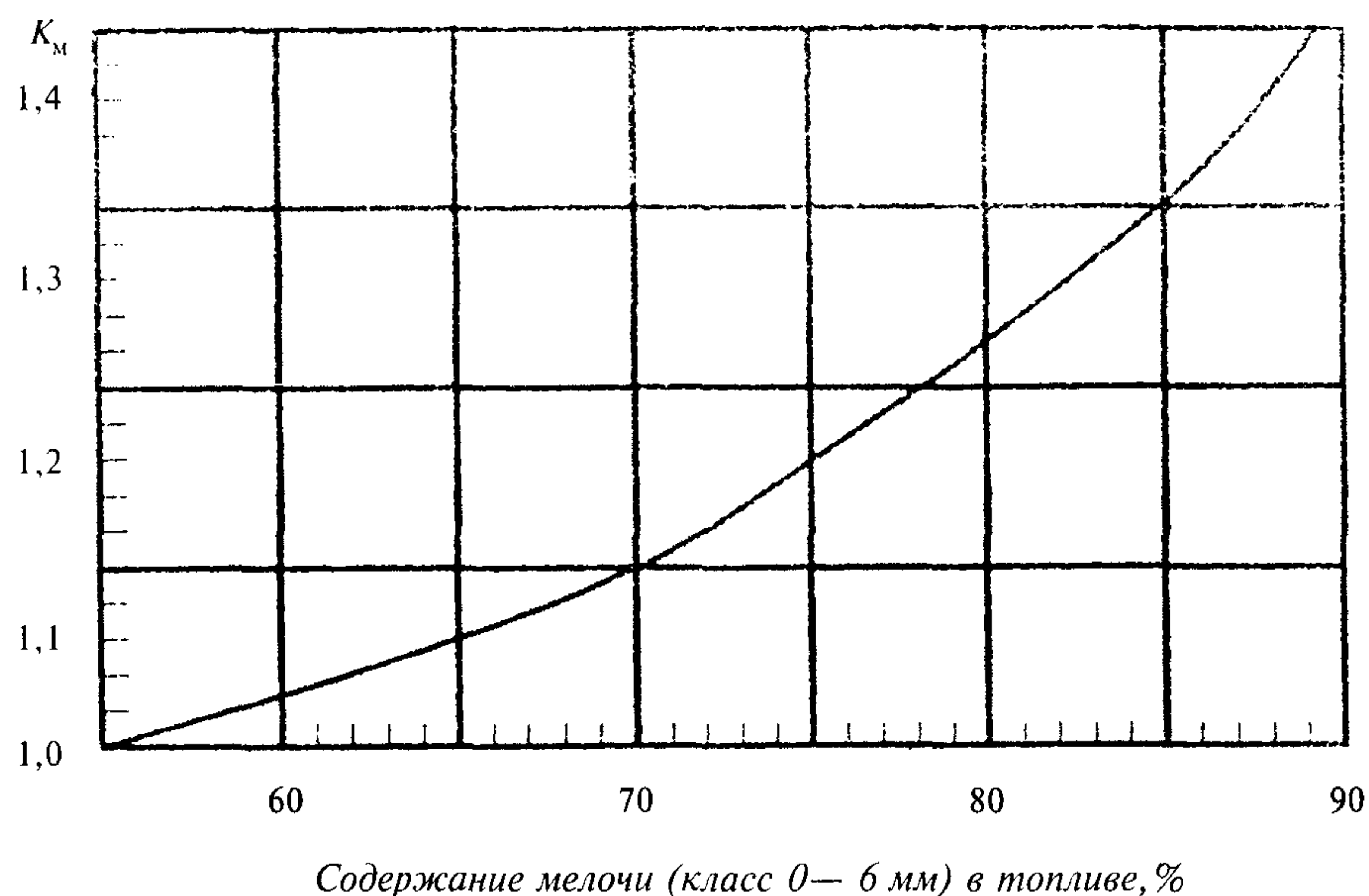
Рисунок 2 — Поправки на содержание мелочи в топливе ( K_M )
