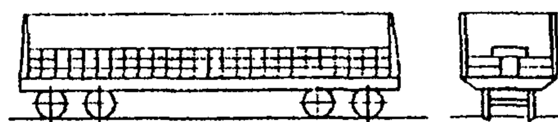
Рис 22 1 – боковые стойки, 2 – увязка стоек, 3 – доски торцового ограждения; 4 – торцовые стойки
