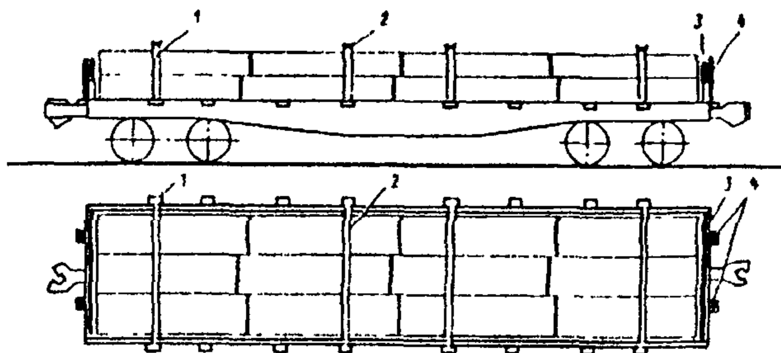
Рис. 21 1 – боковые стойки; 2 – увязка стоек; 3 – доски торцового ограждения; 4 – торцовые стойки
