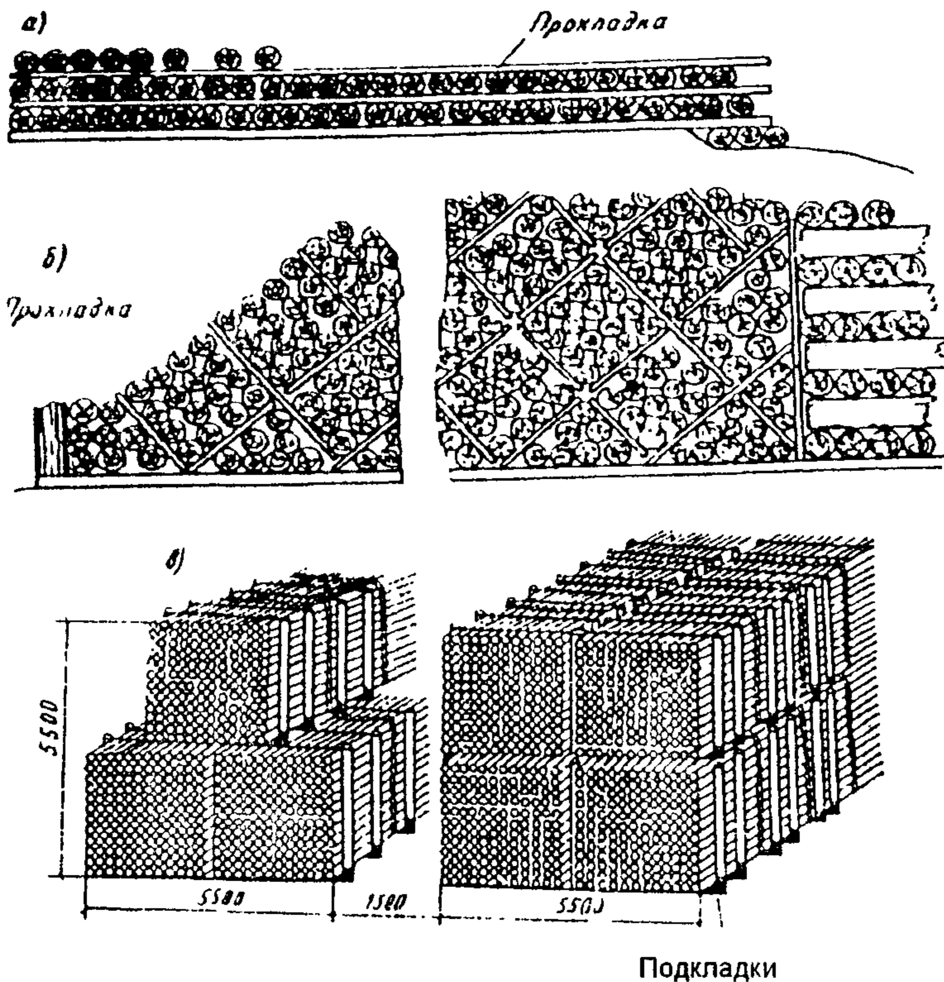
Рис.2. Укладка круглого леса: а) – Рядовой штабель б) – Клеточный штабель в) – Пачковой штабель
