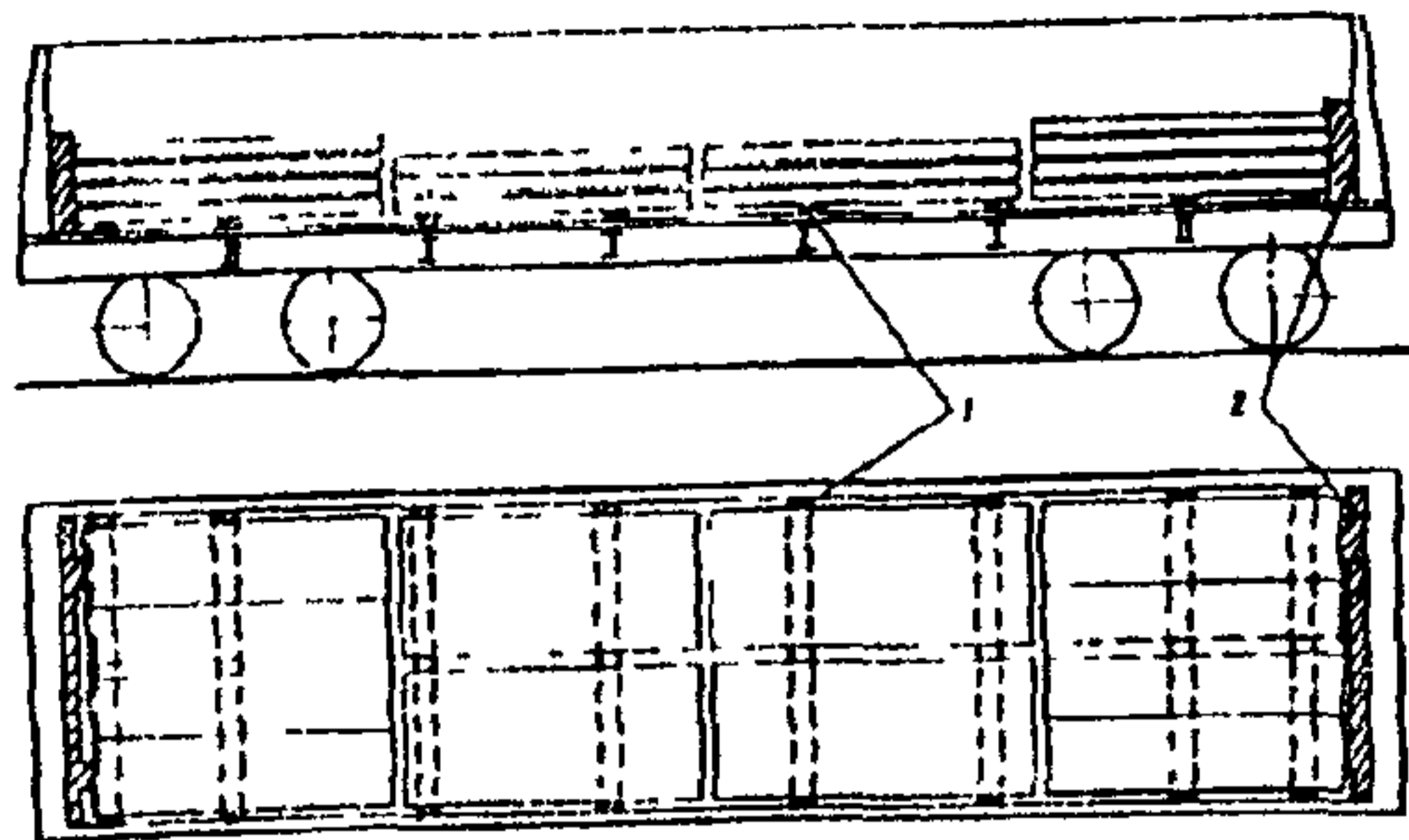
Рис. 2.16 1 – подкладки; 2 – щит
