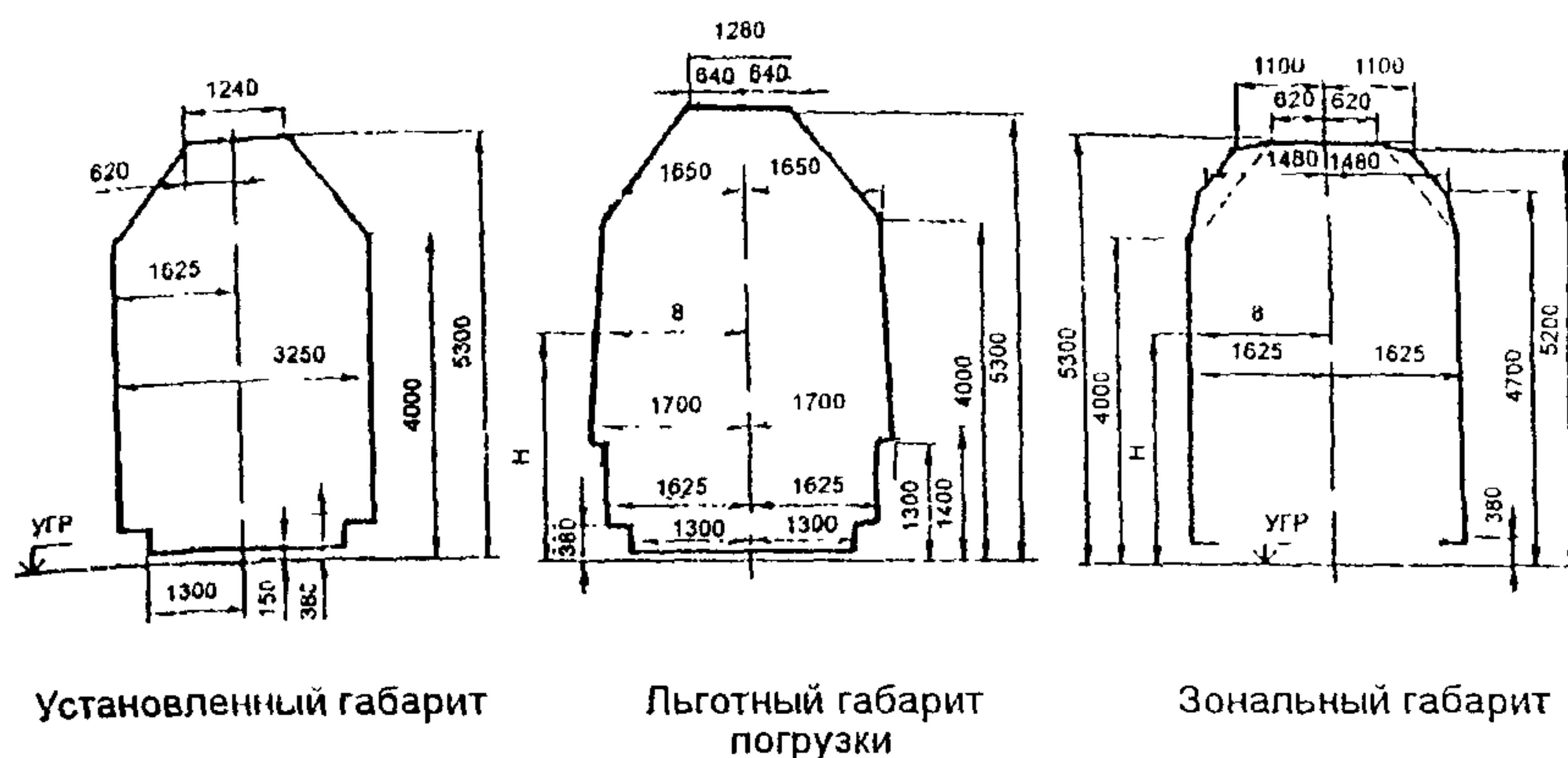
Рис. 1. Габариты погрузки грузов в железнодорожные вагоны
