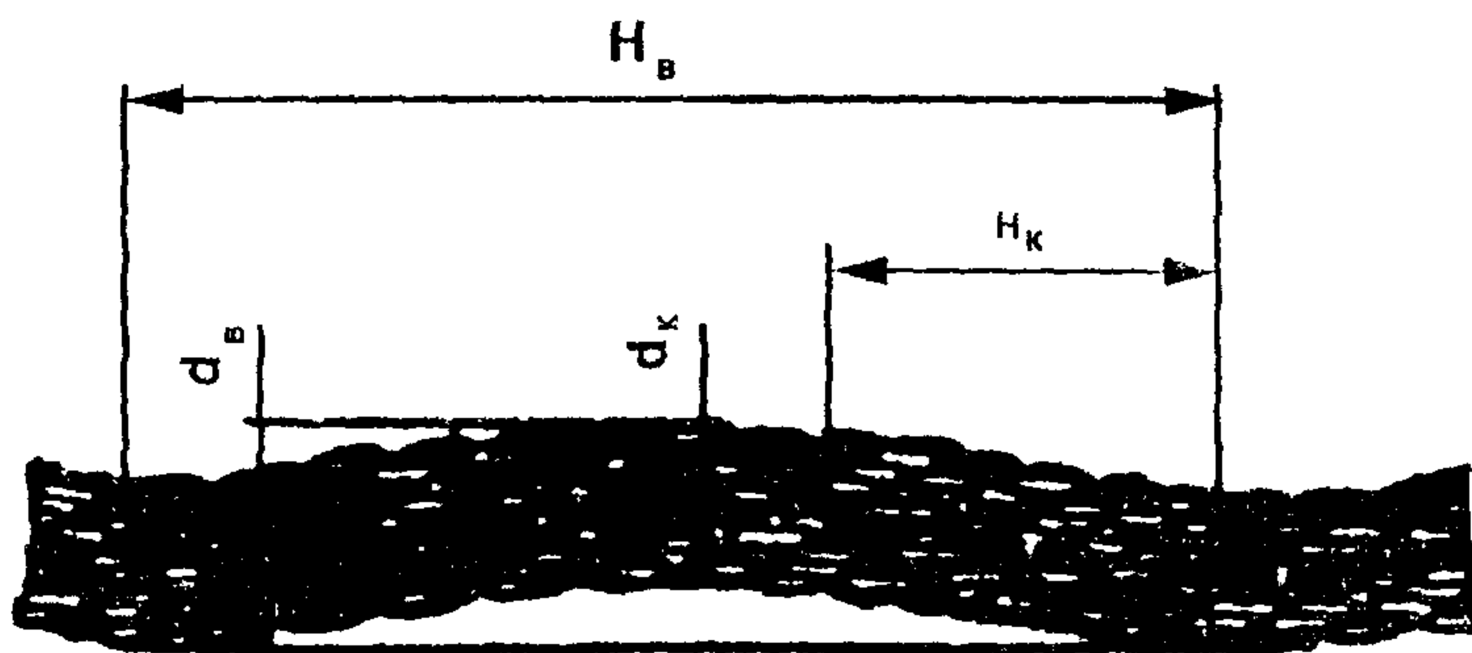
Рис. 8 Волнистость каната (объяснение в тексте)
