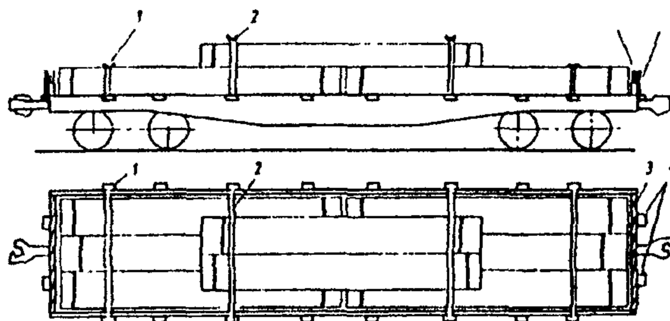
Рис 22 1 – боковые стойки, 2 – увязка стоек, 3 – доски торцового ограждения; 4 – торцовые стойки
