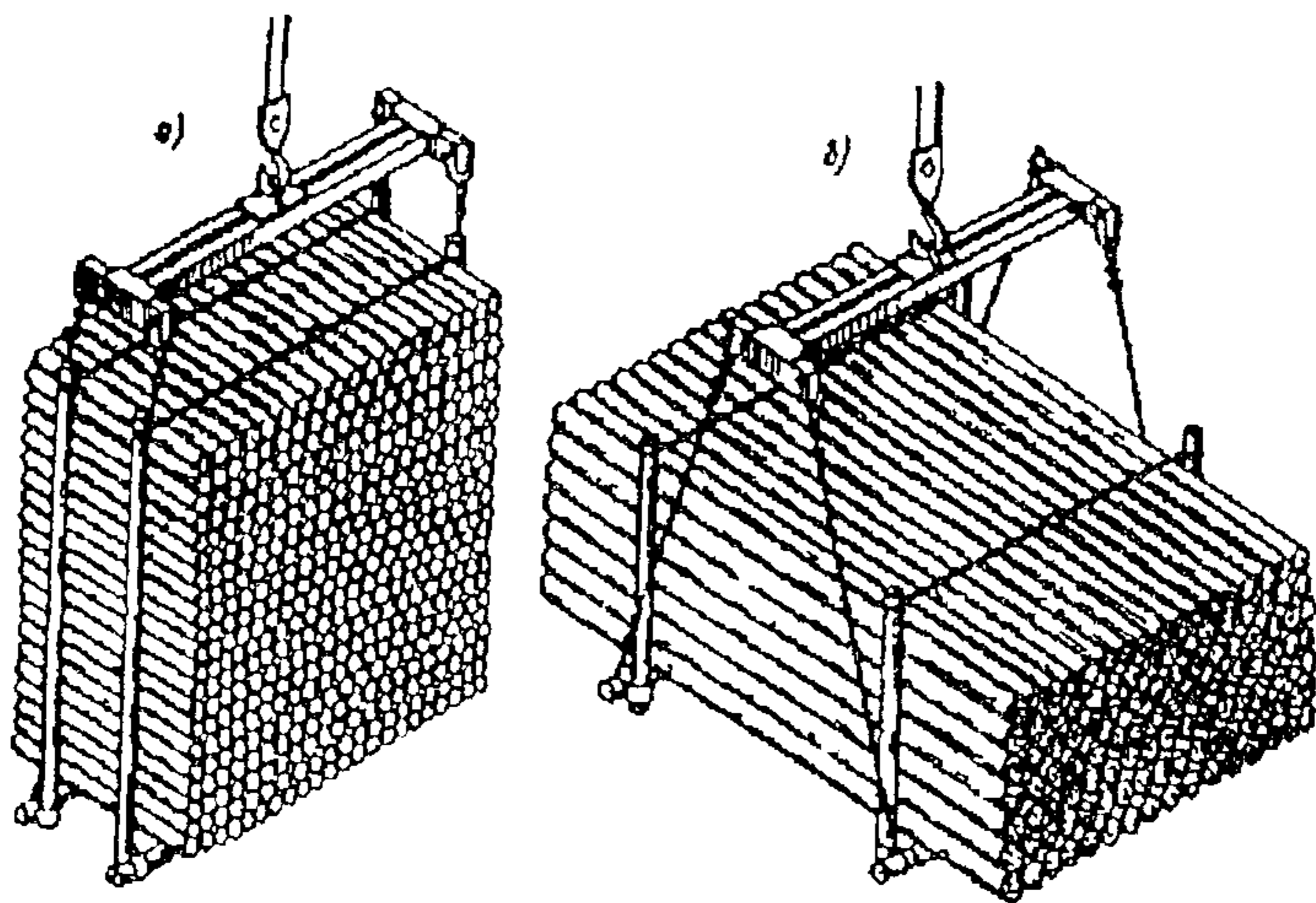
Пространственные траверсы для короткомерных (а) и круглых длиномерных материалов (б)
