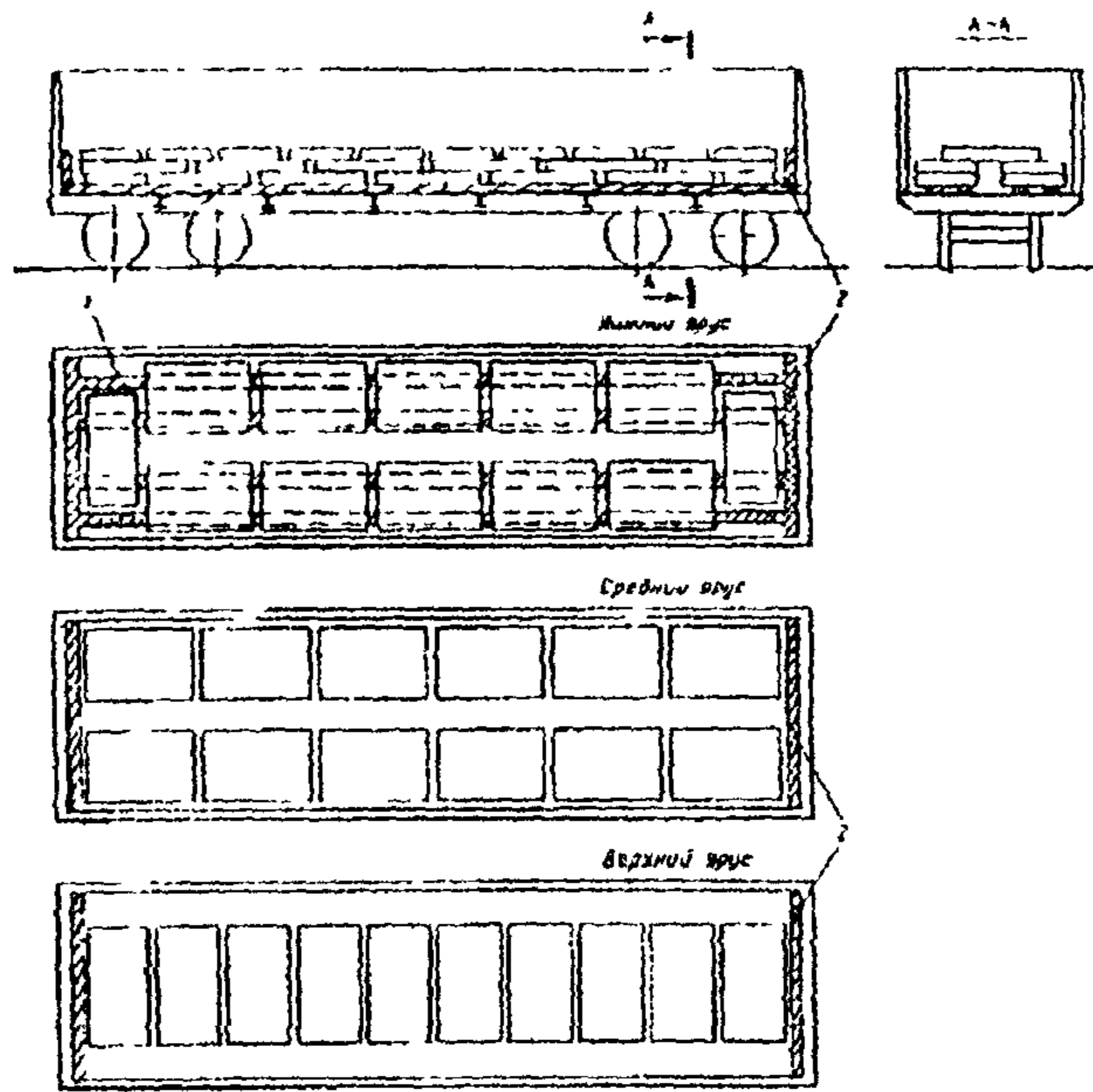
Рис 2.14 1 – подкладки; 2 – щит
