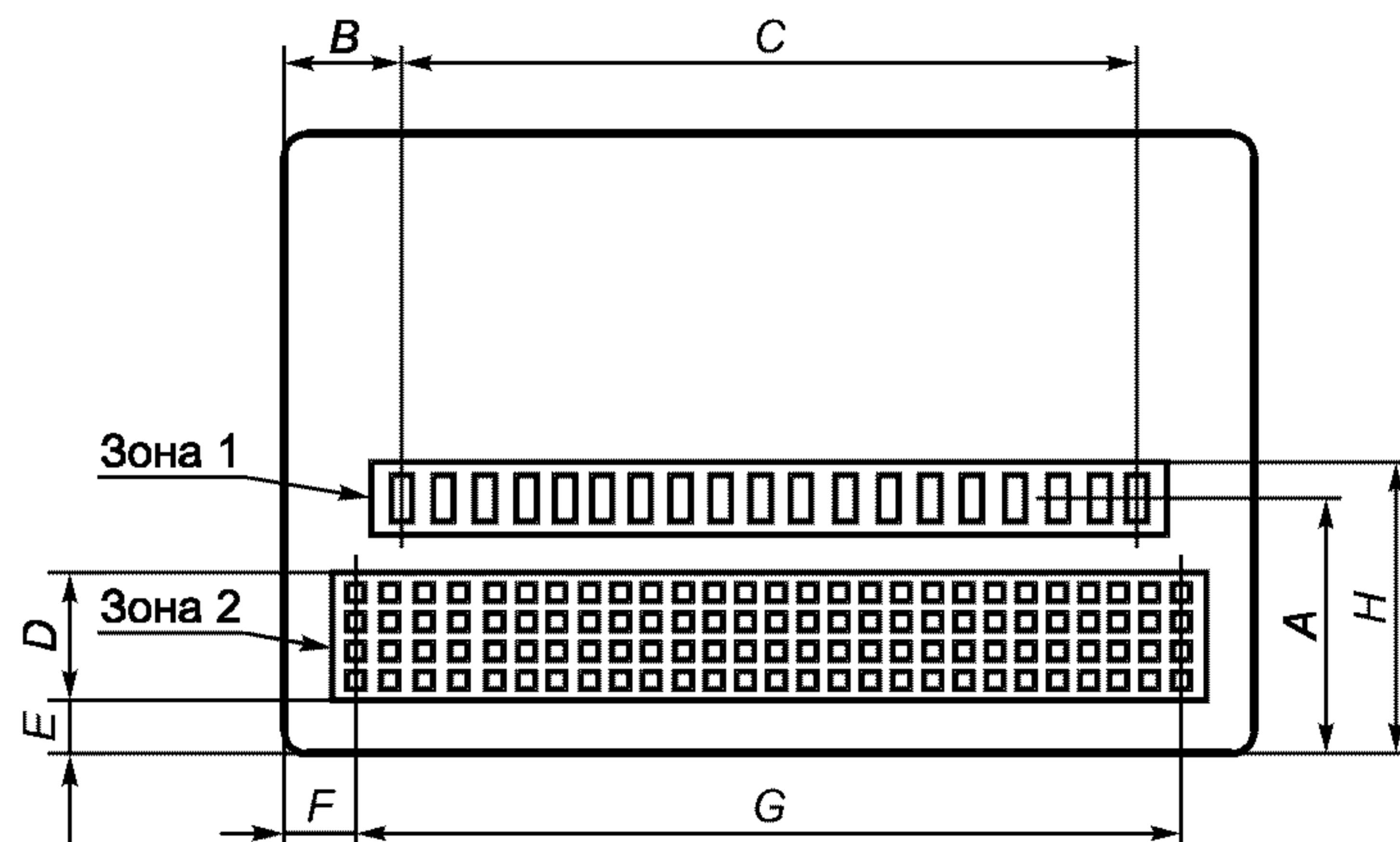
Рисунок 1 — Расположение зон тиснения
