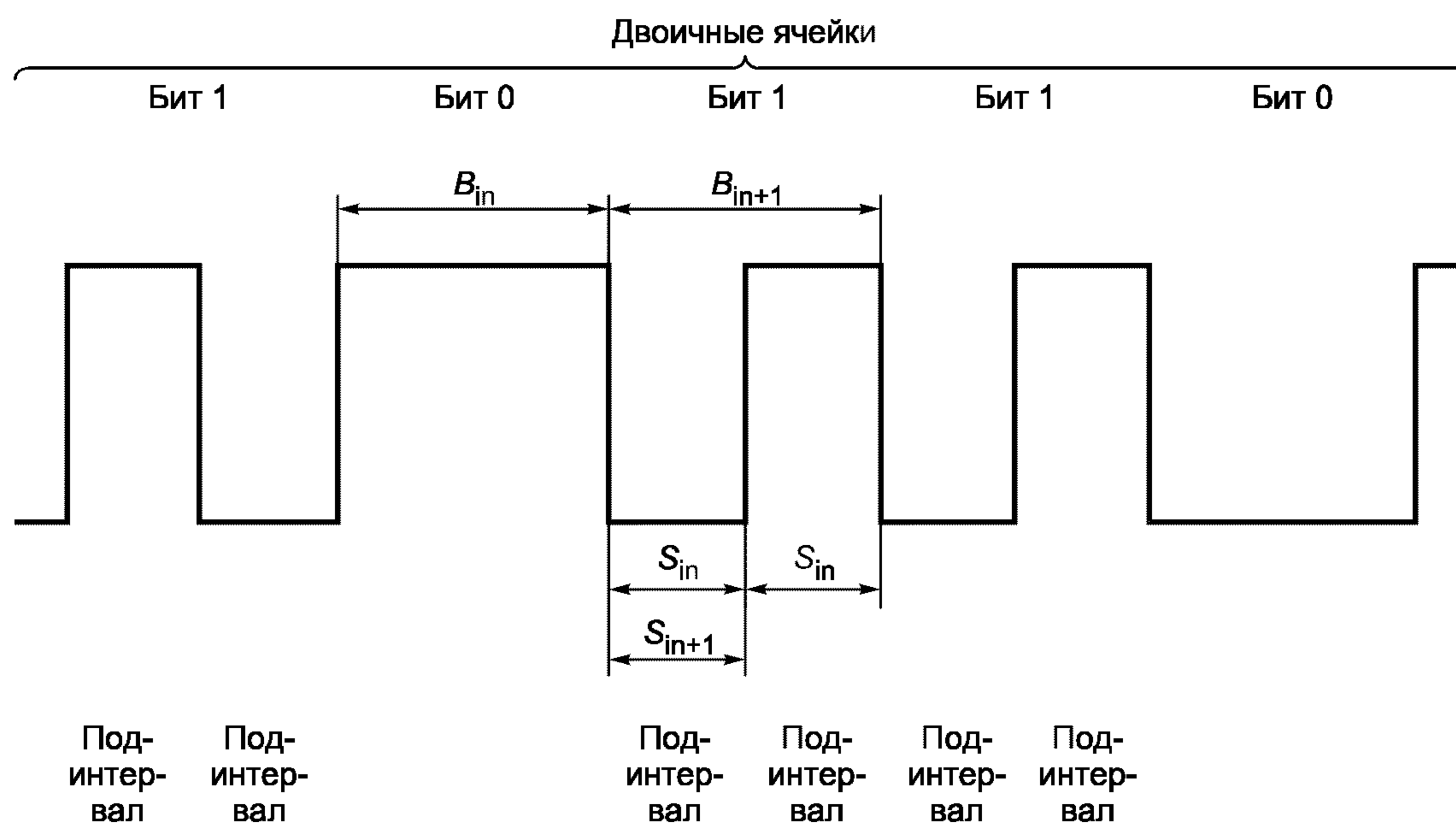
Рисунок 10 — Изменение промежутка между переходами потока
