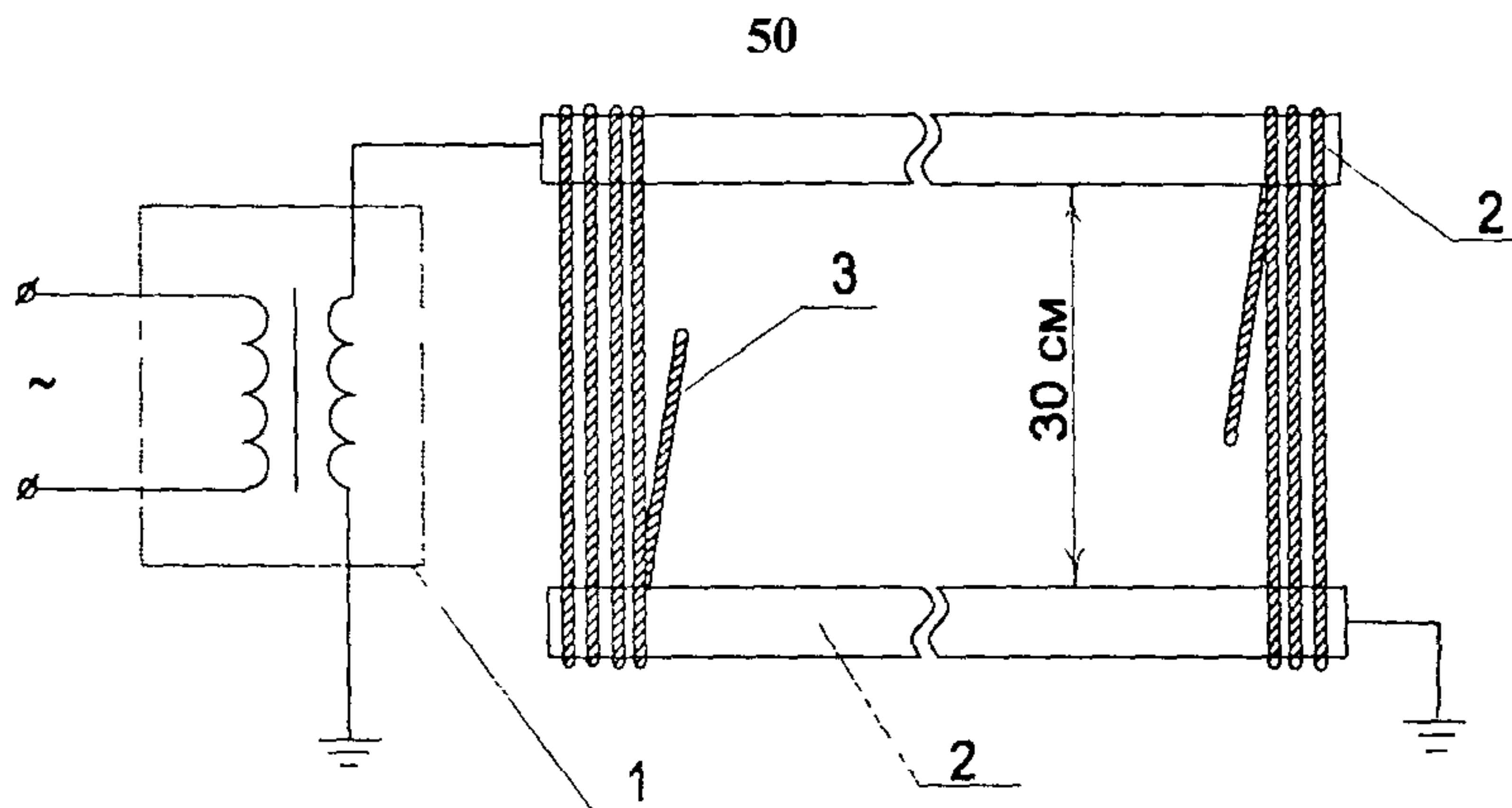
Рис. 2.4. Схема электрических испытаний изолирующего каната: 1 – источник испытательного напряжения; 2 – металлическая труба; 3 – испытуемый изолирующий канат
