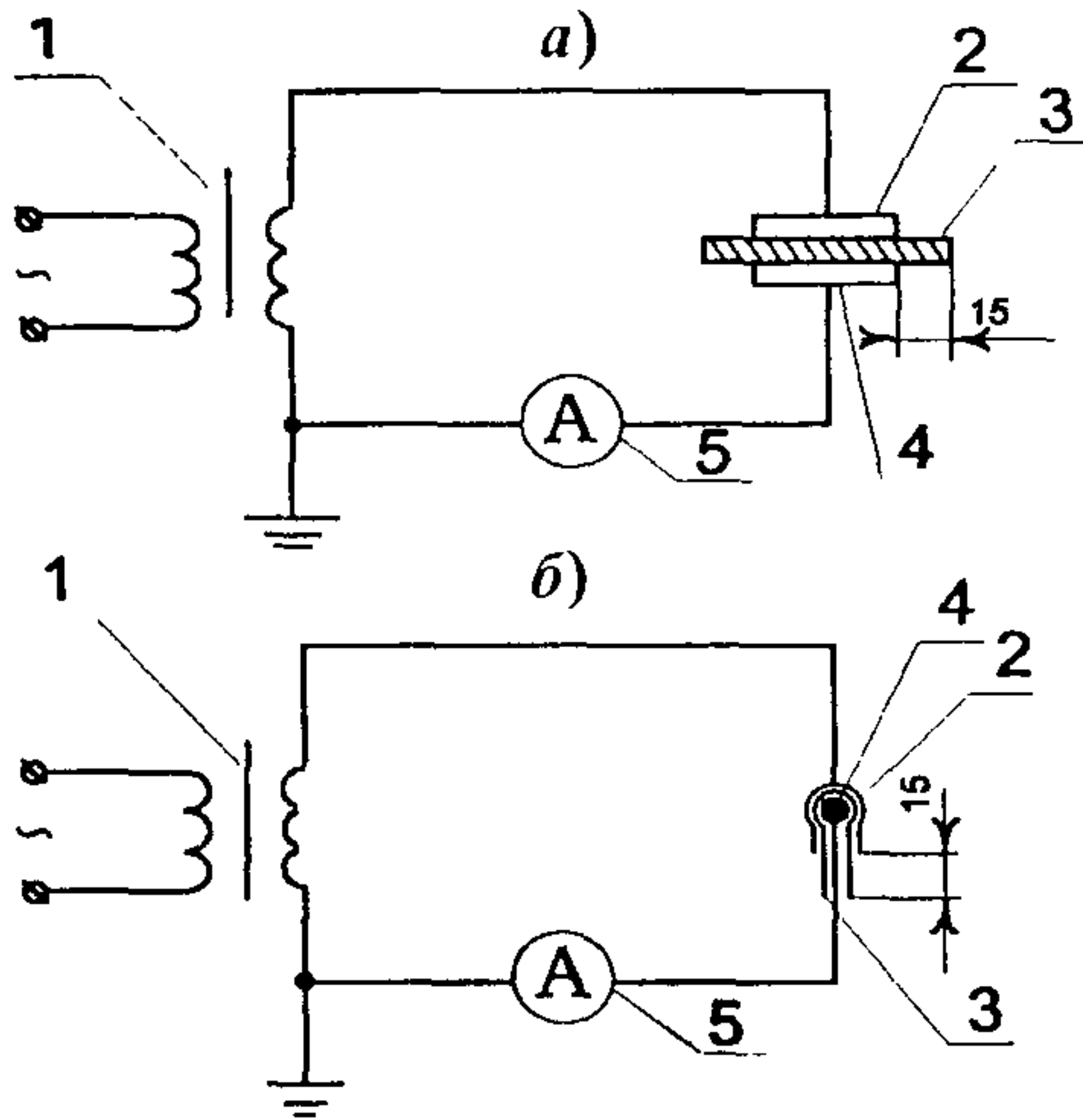
Рис. 2.5. Схемы электрических испытаний гибкого изолирующего покрытия (а) и гибкой изолирующей накладки (б): 1 – испытательный трансформатор; 2 – верхний (наружный) электрод; 3 – изолирующее покрытие или накладка; 4 – нижний (внутренний) электрод; 5 – миллиамперметр
