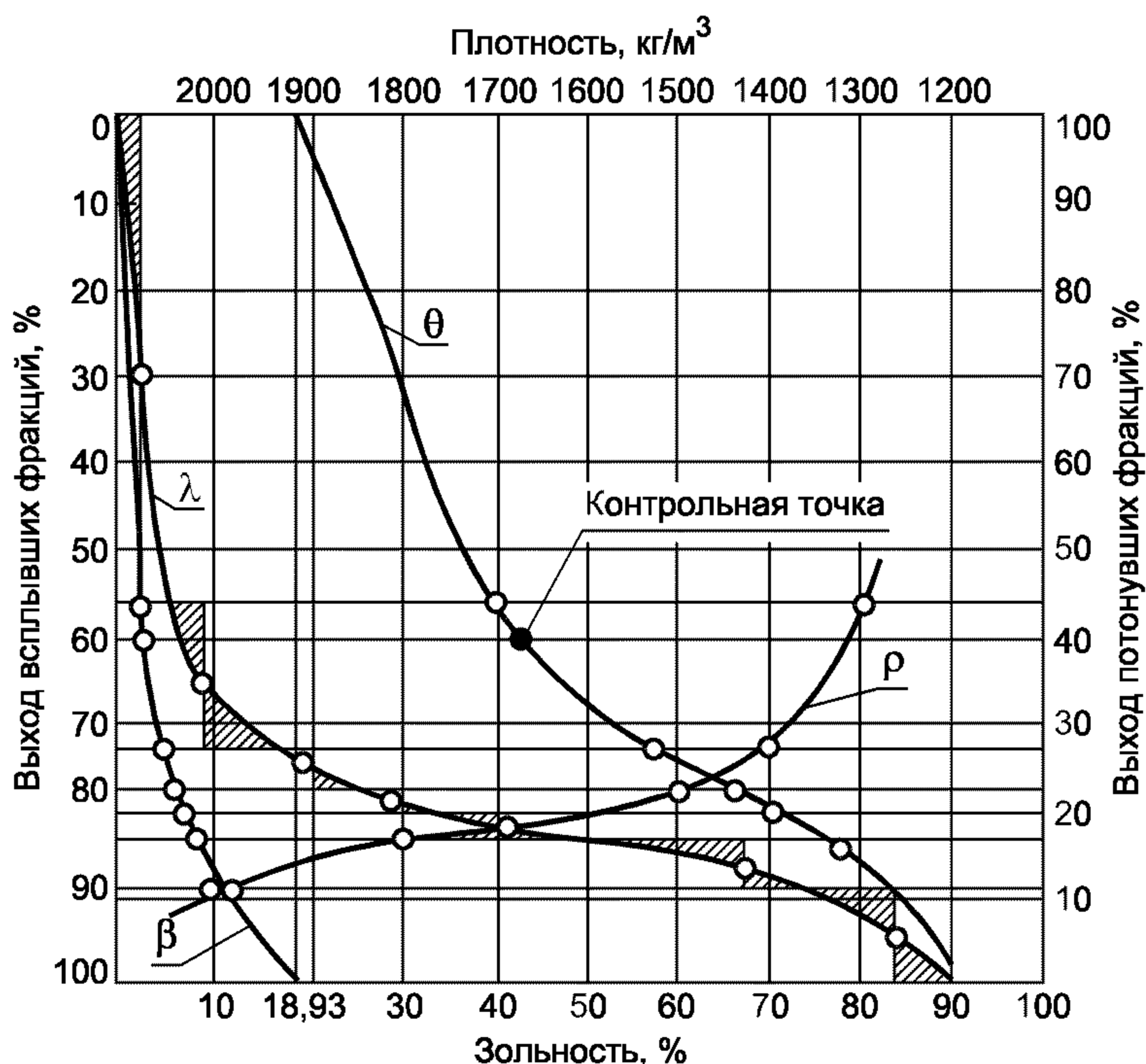
Рисунок В.1 — Кривые обогатимости
