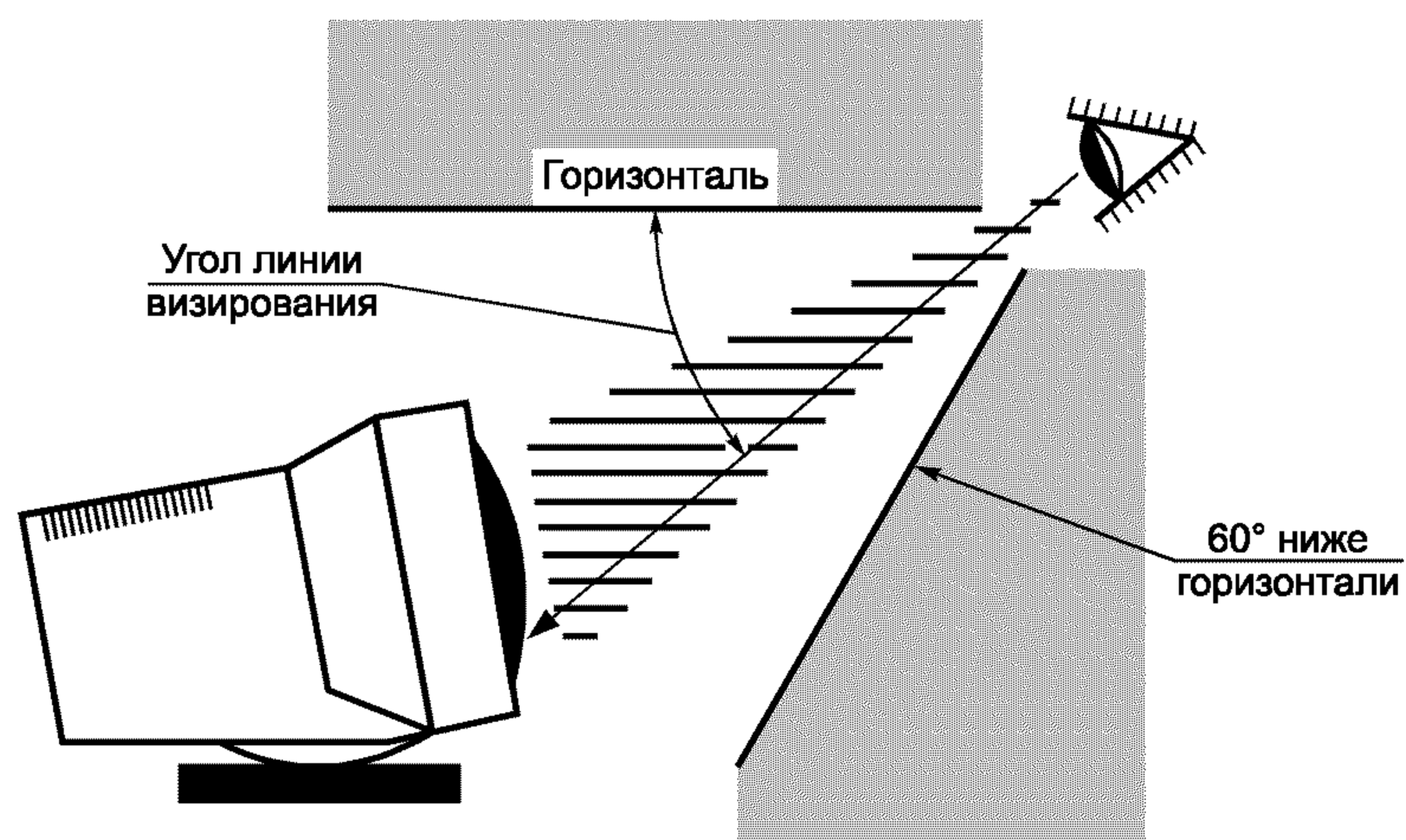
Рисунок 2 — Угол линии визирования
