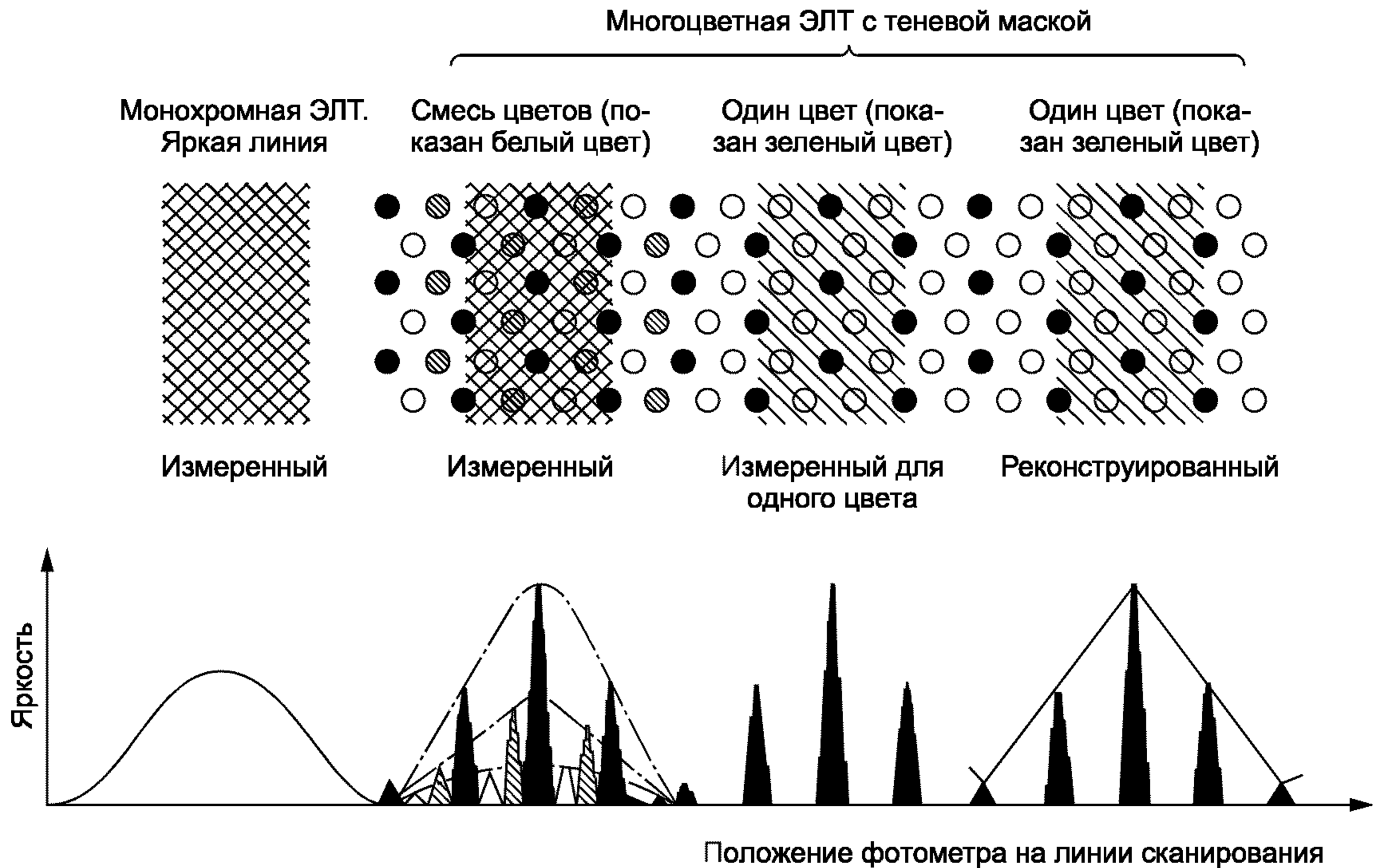
Рисунок 8 — Измеренные и реконструированные профили яркости
