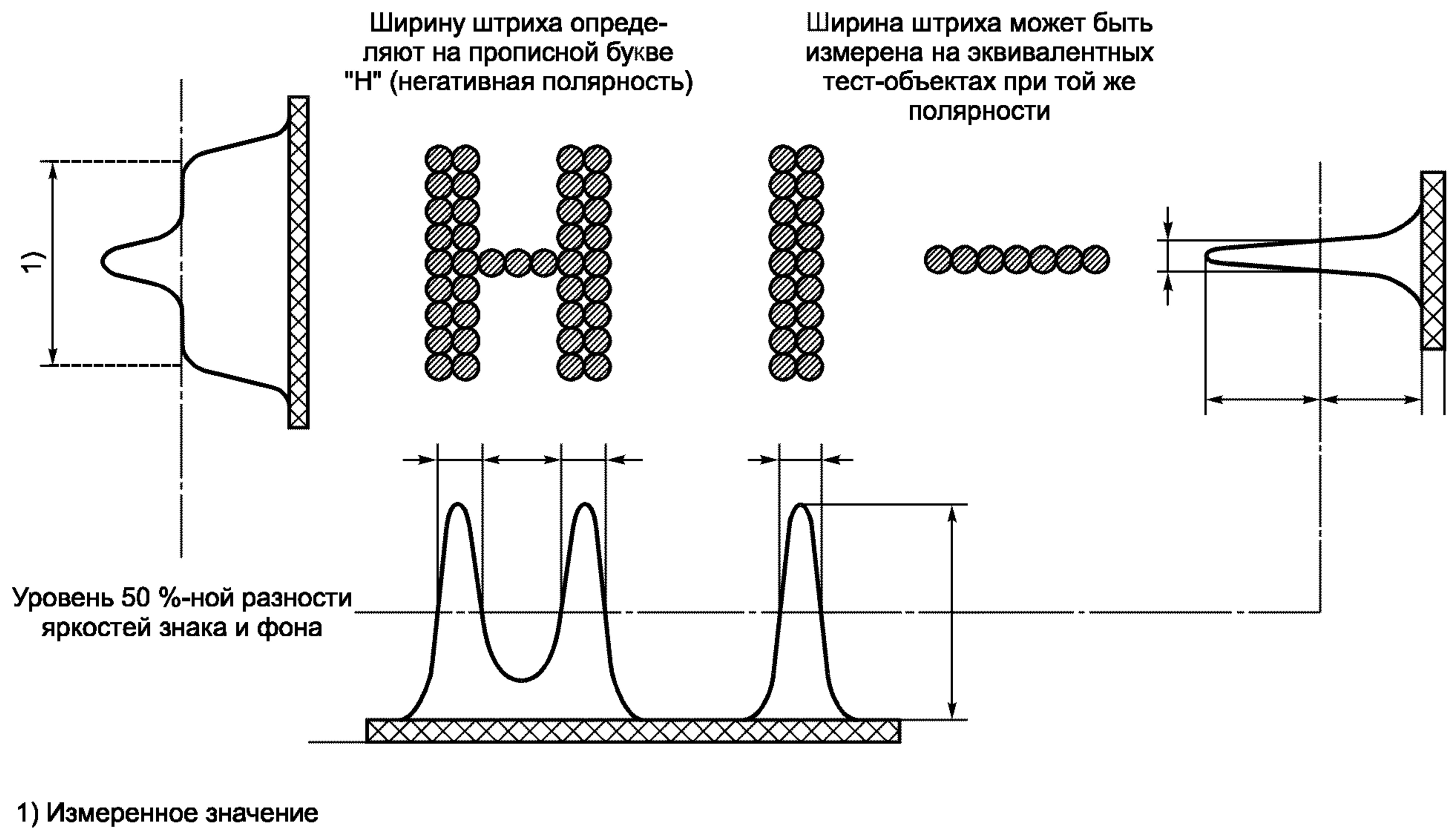
Рисунок 13 — Ширина штриха знака
