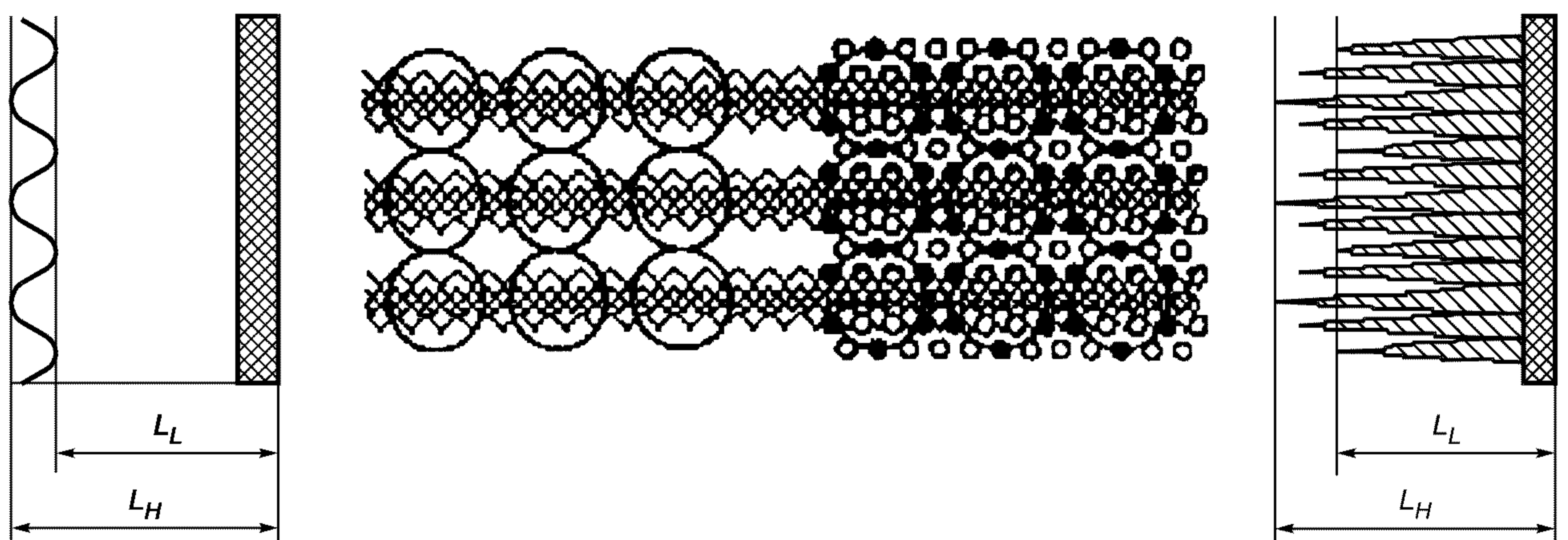
Рисунок 14 — Модуляция растра (плоское поле)
