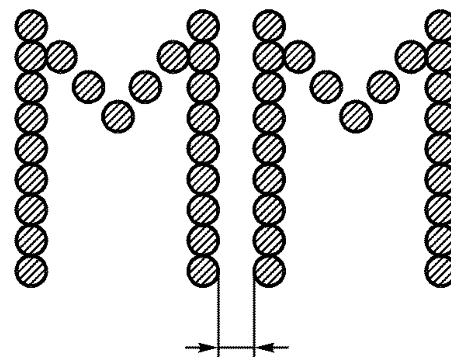
Рисунок 5 — Интервал между знаками
