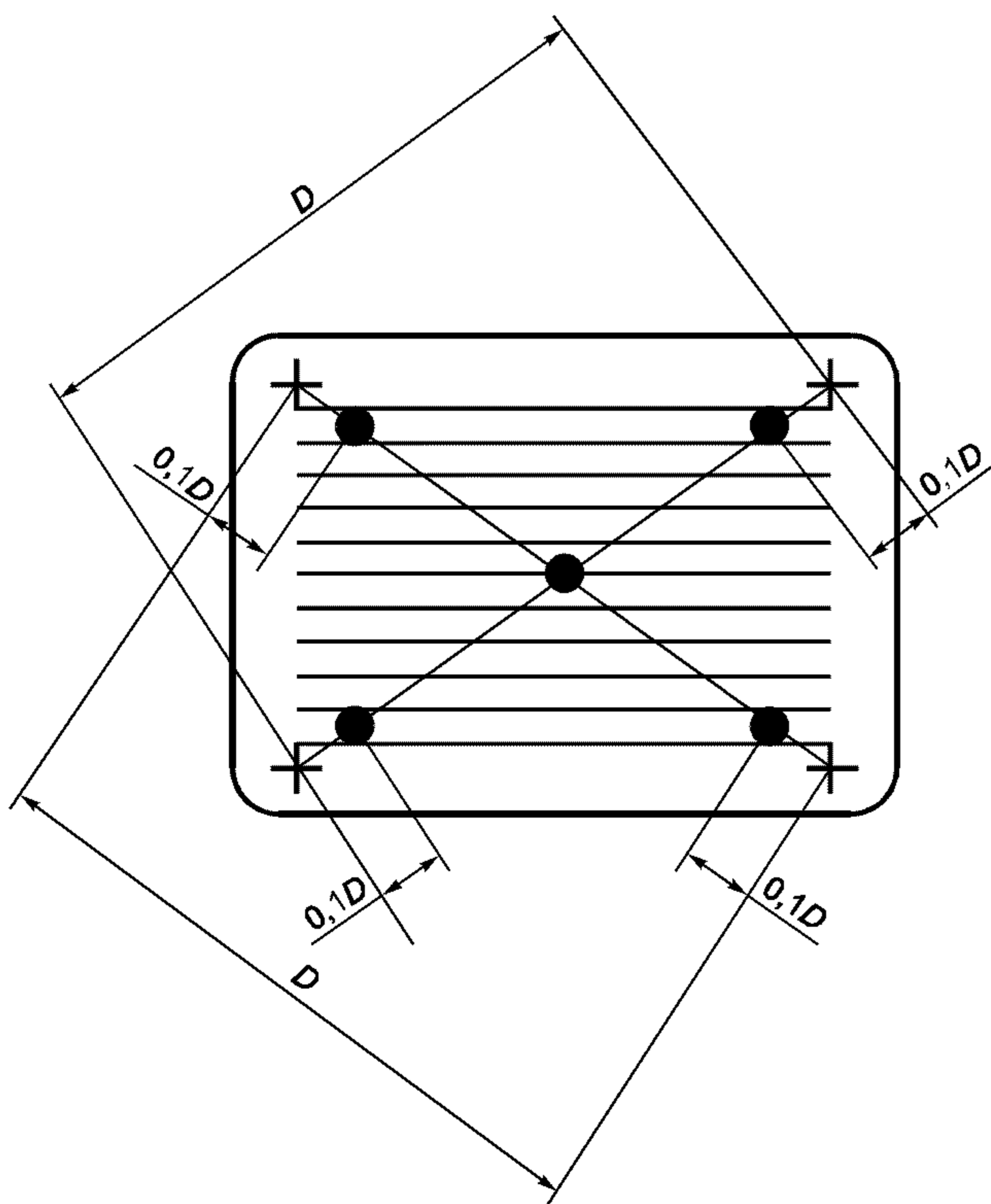
Рисунок 11 — Стандартные места измерений
