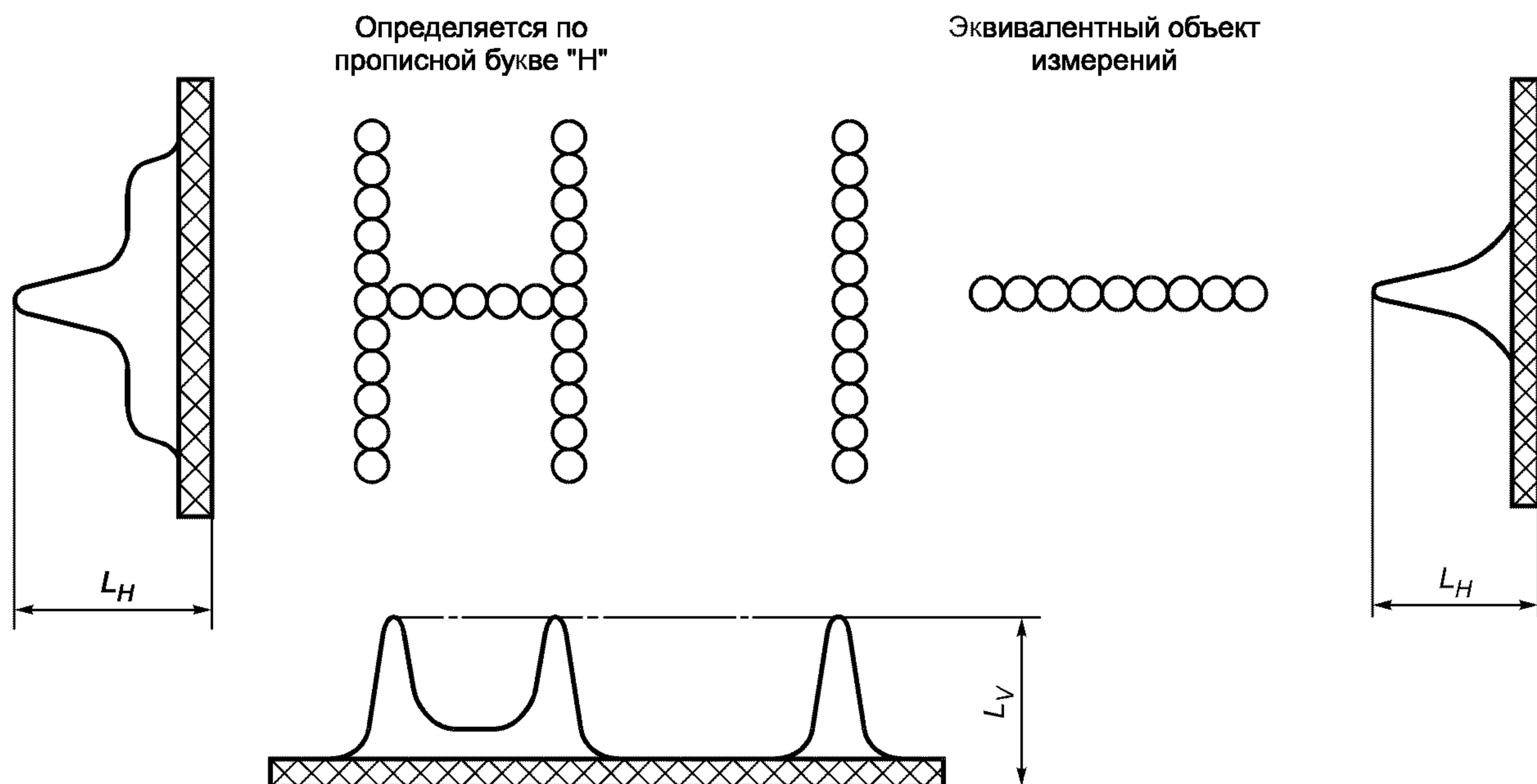
Рисунок 15 — Однородность яркости внутри знака
