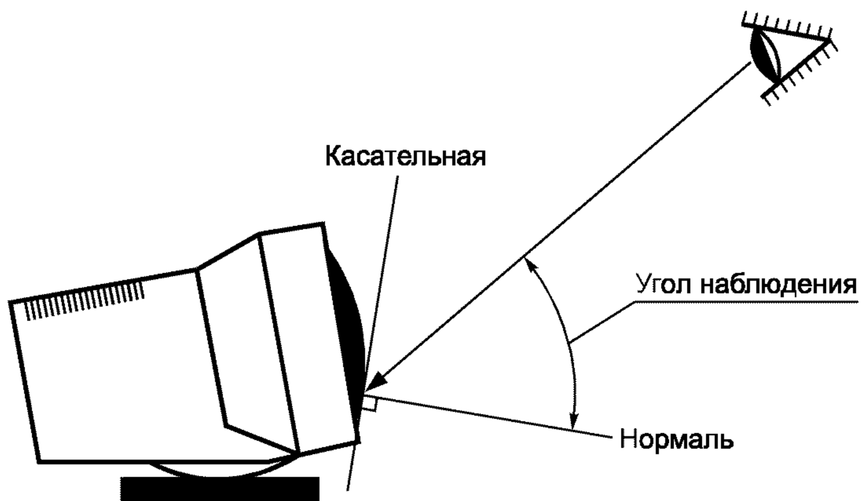
Рисунок 3 — Угол наблюдения
