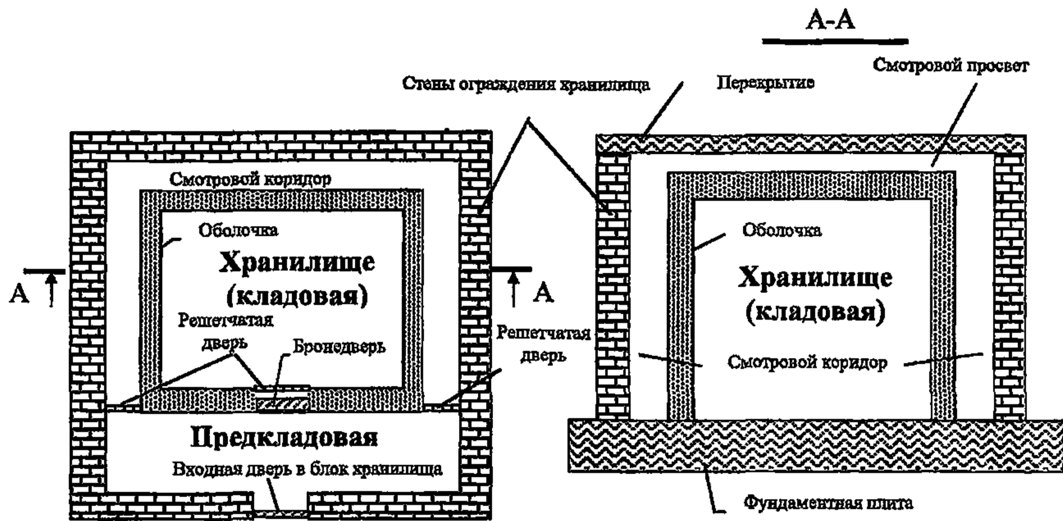
Рисунок П8.1- Схематичное устройство хранилища ценностей
