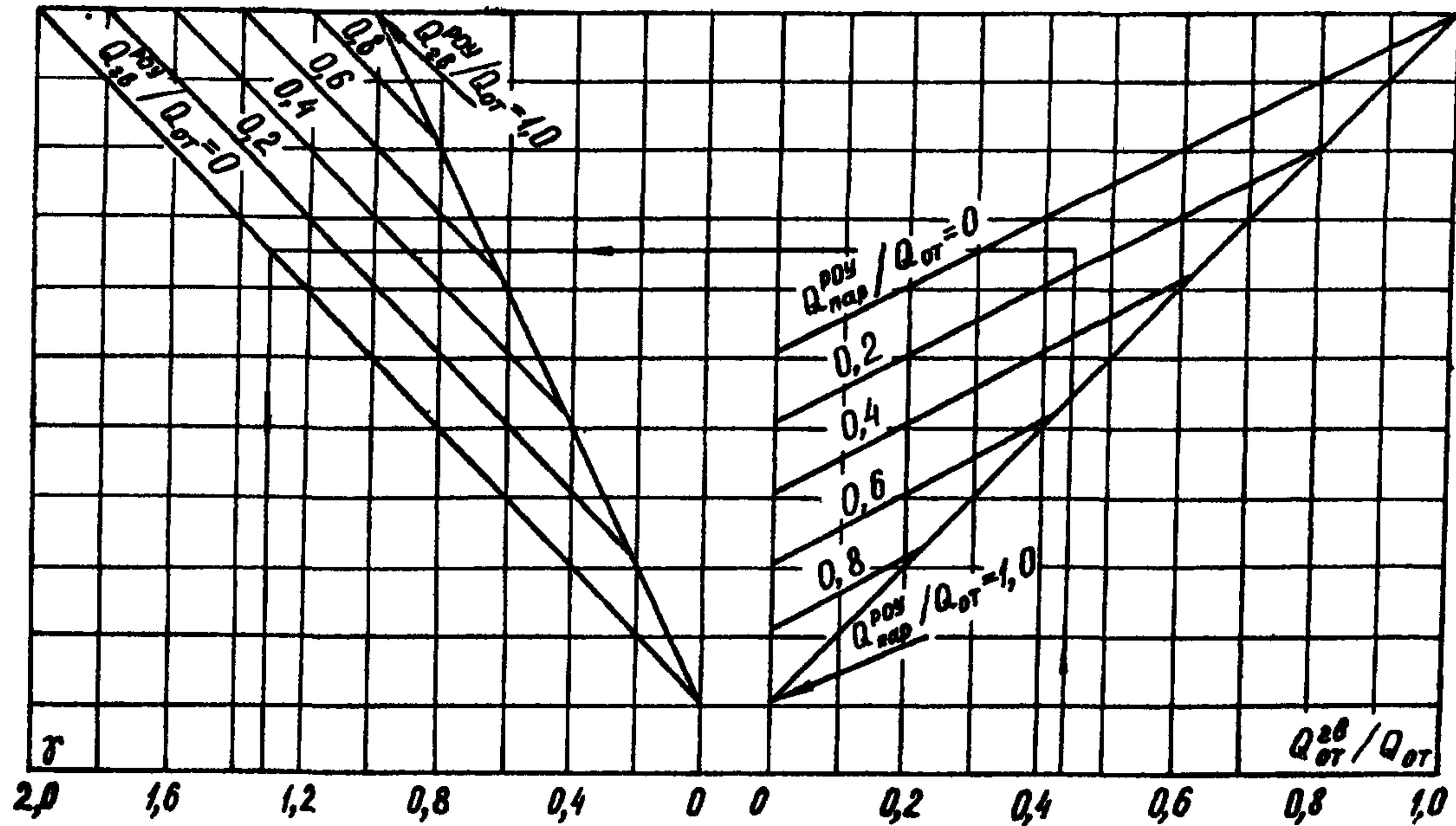
Рис.П4.2. Номограмма для определения значения коэффициента \gamma : Q_{пар}^{роу} - отпуск тепла паром, не прошедшим через проточную часть турбоагрегата (непосредственно от котла или через РСУ); Q_{гв}^{роу} - отпуск тепла с горячей водой, обеспеченный не прошедшим через проточную часть турбоагрегата паром, а также за счет нагрева воды в насосах
