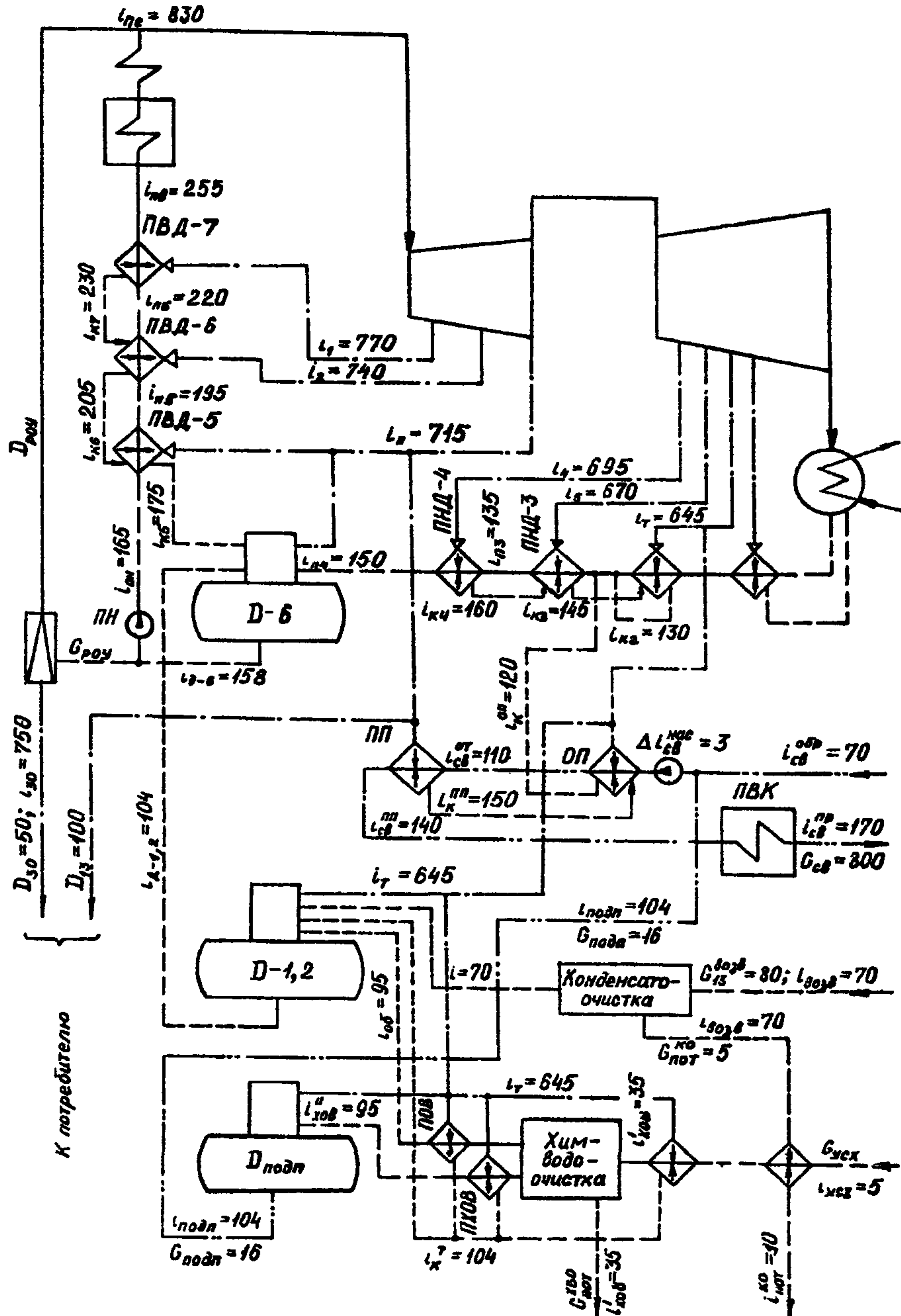
Рис. П4.1 Расчетная тепловая схема:
