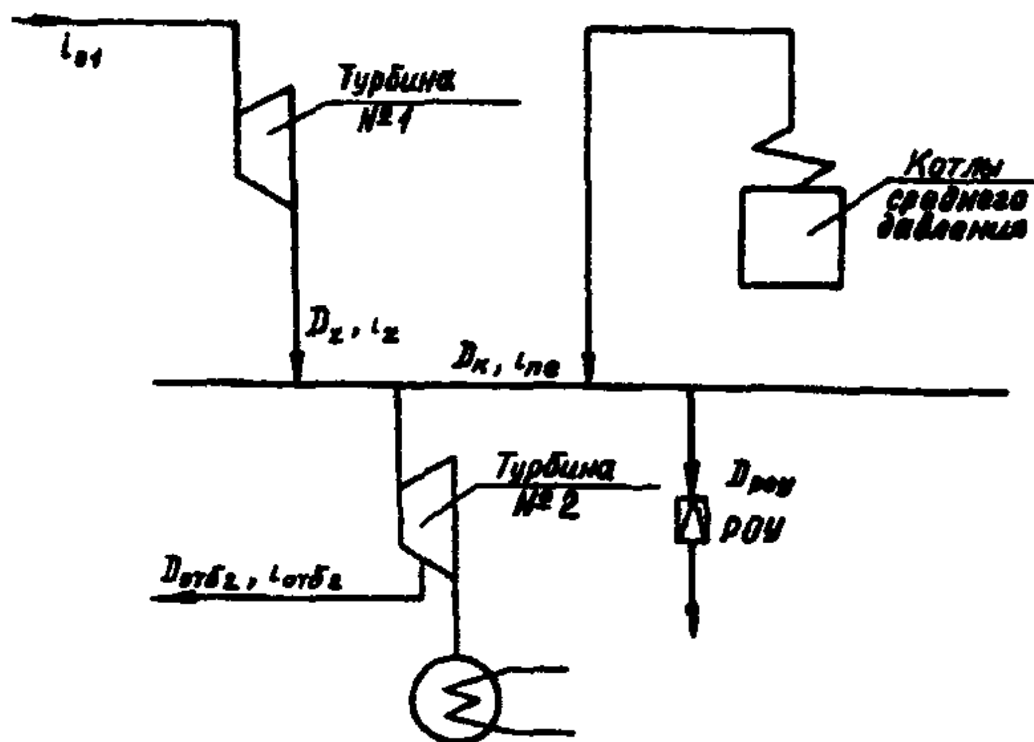
Рис.1. Принципиальная тепловая схема ТЭС с предвключенной турбиной
