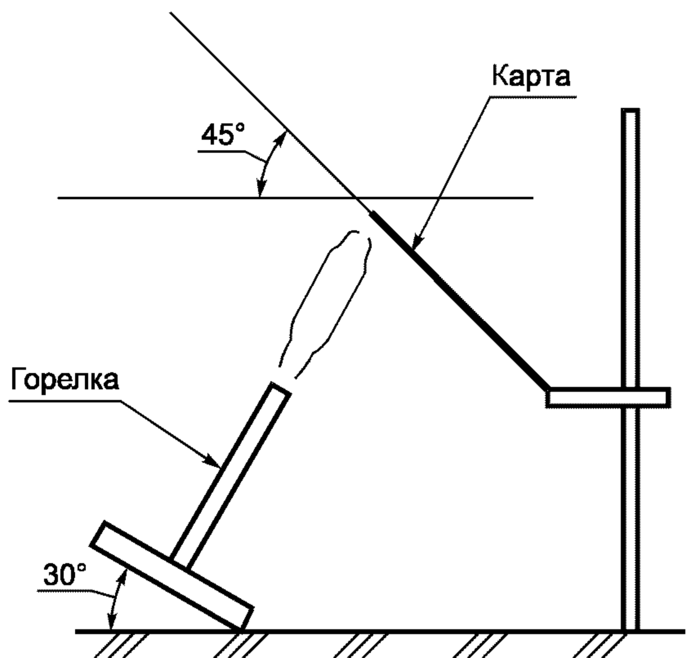
Рисунок 14 — Расположение карты и горелки
