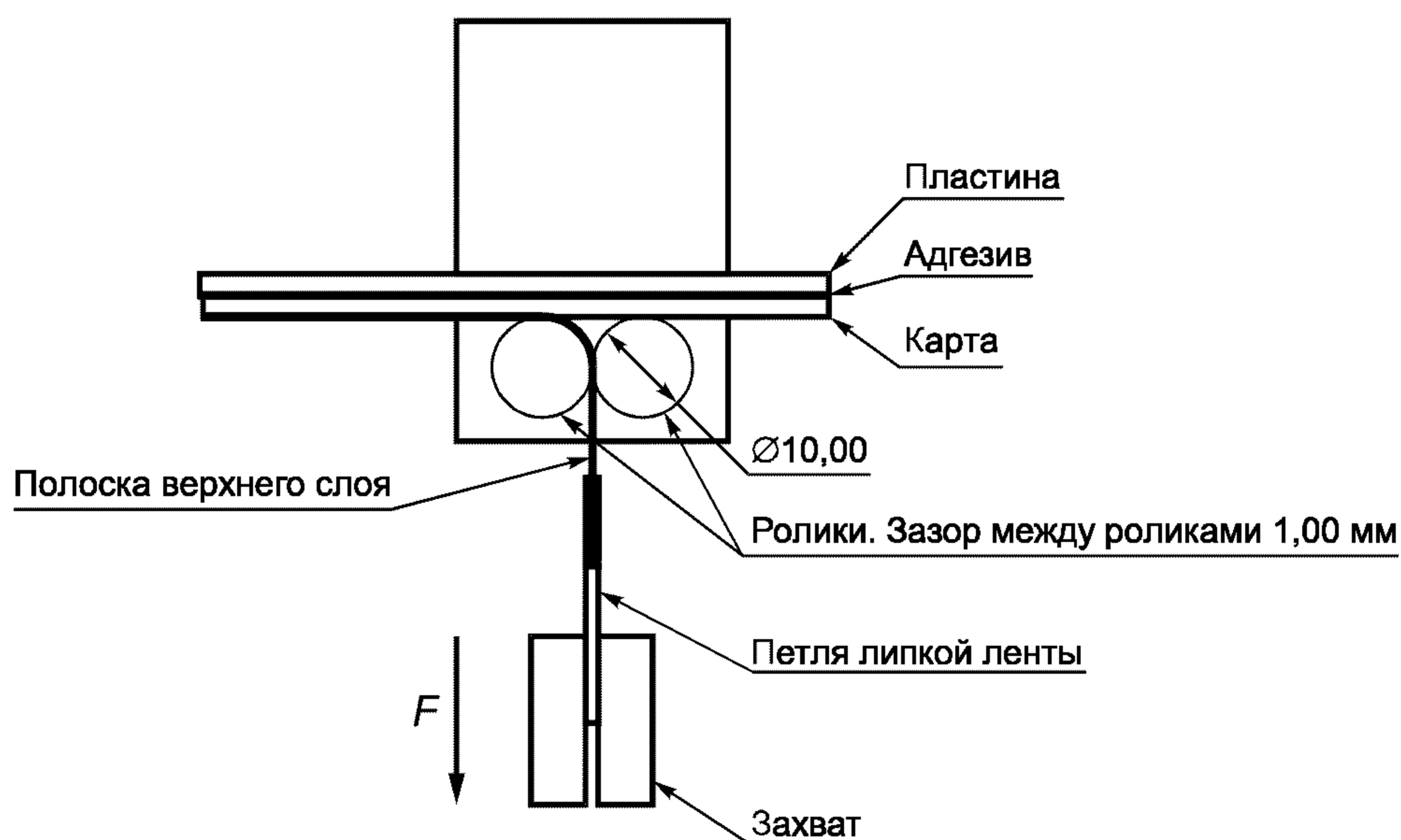
Рисунок 5 — Схема установки карты в разрывной машине
