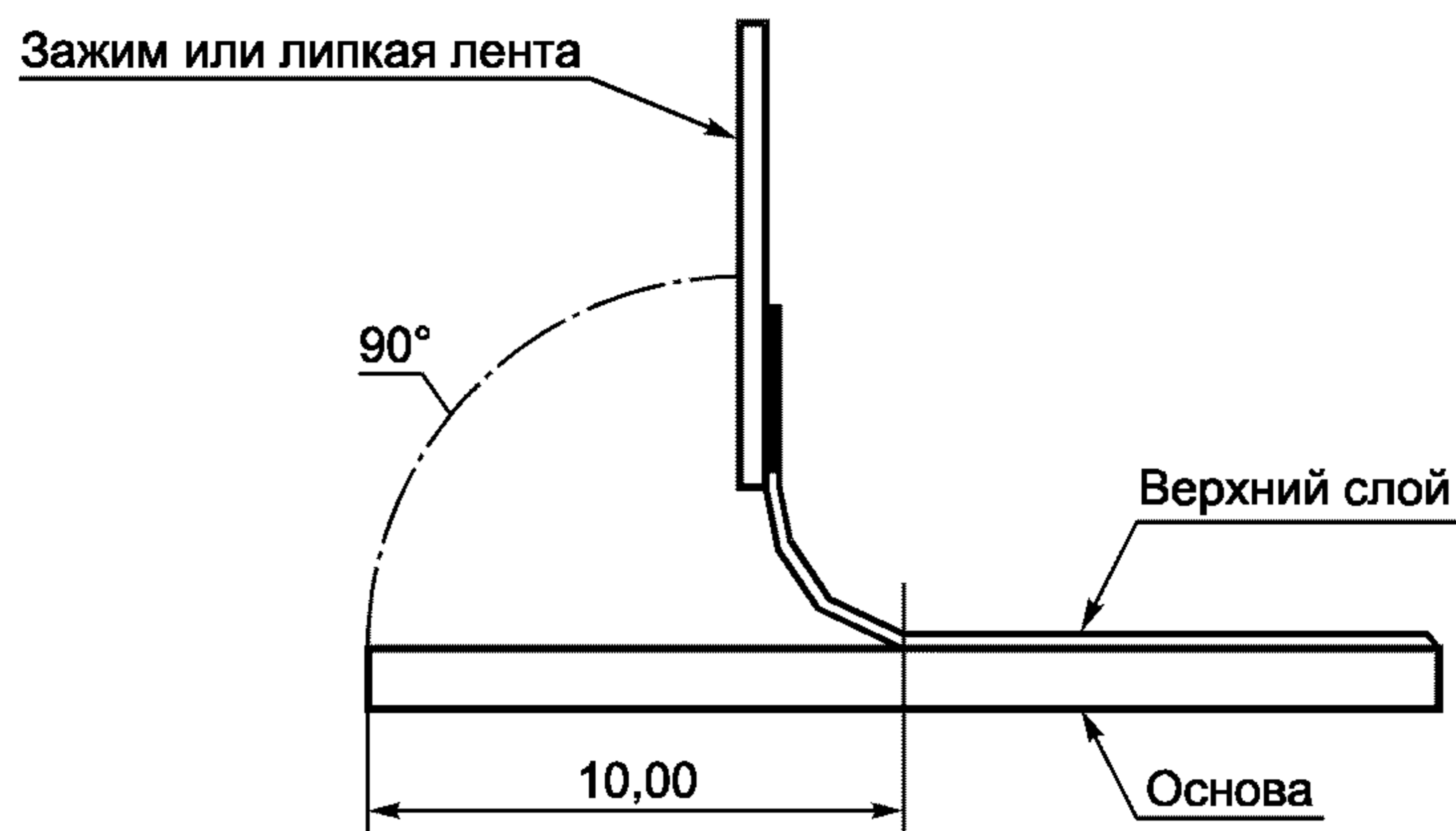
Рисунок 4 — Подготовка образца к испытанию
