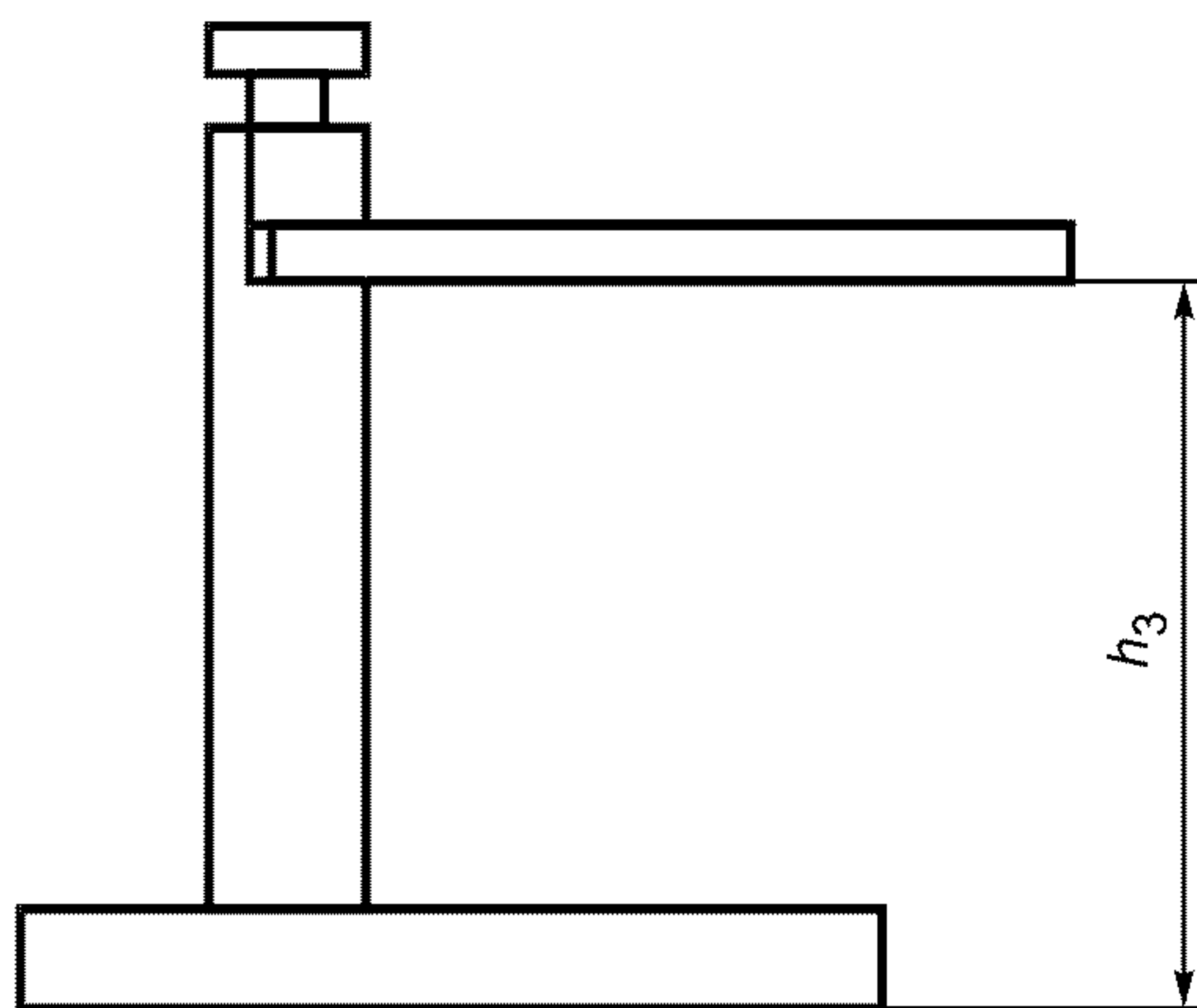
Рисунок 9 — Карта в зажимном устройстве после снятия нагрузки
