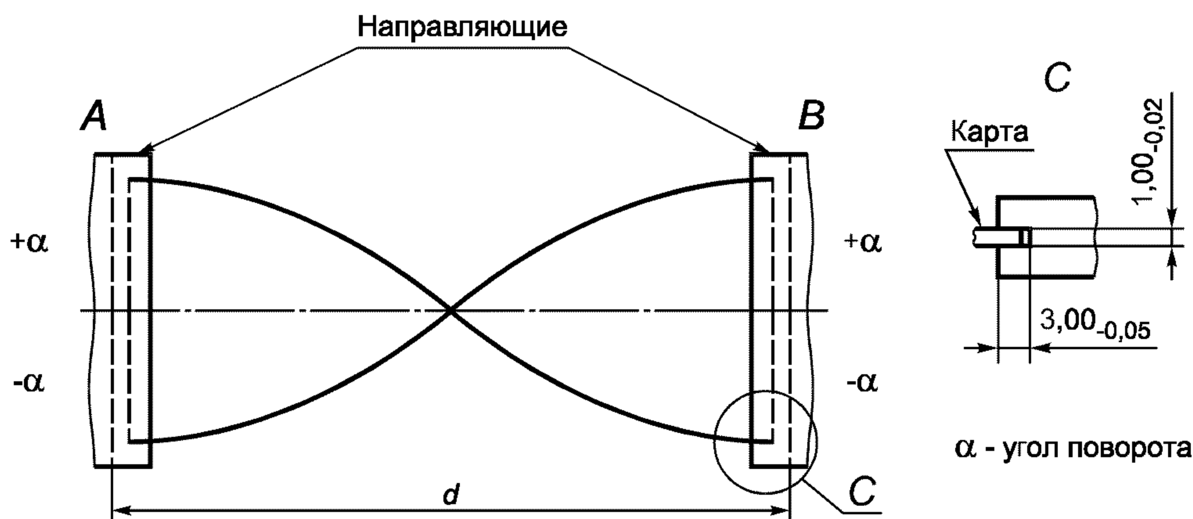
Рисунок 12 — Машина для испытания на скручивание
