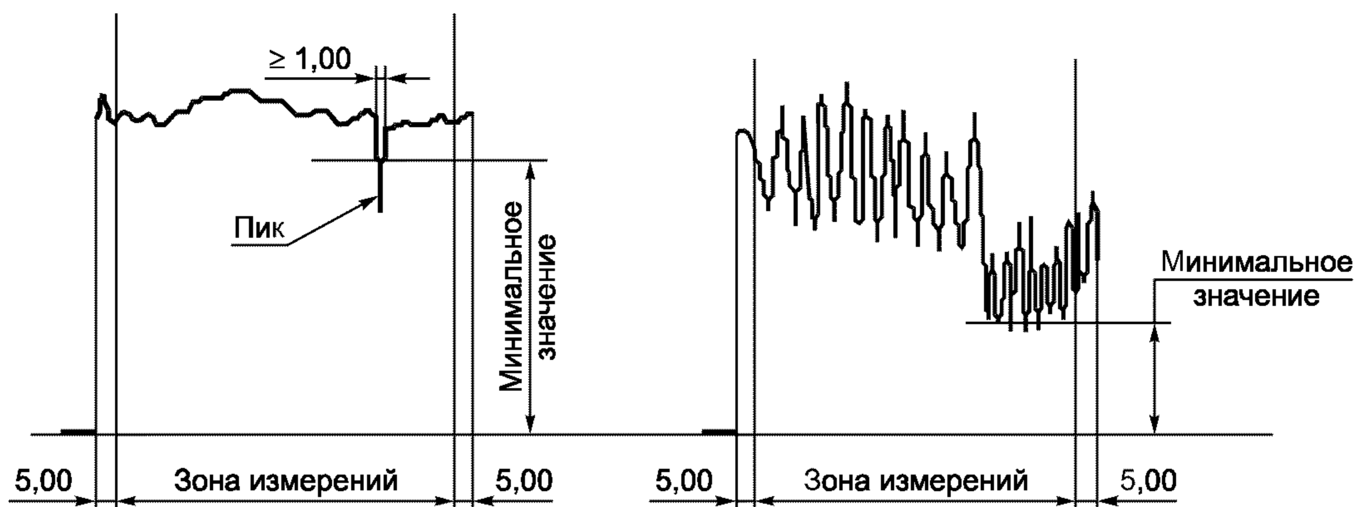
Рисунок 6 — Примеры диаграмм прочности сцепления
