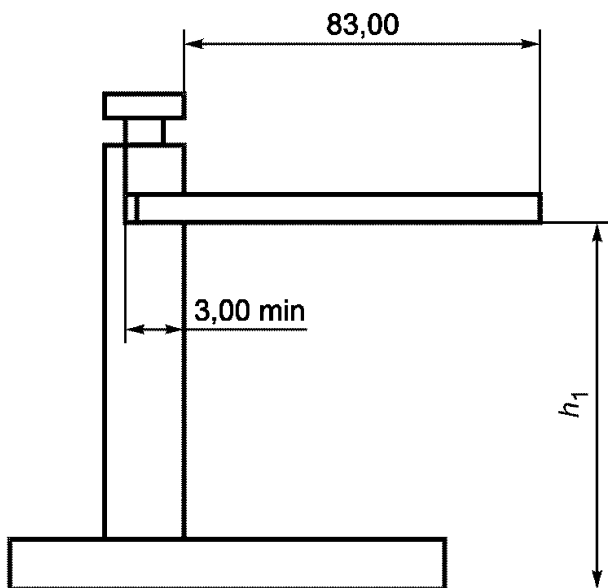
Рисунок 7 — Карта в зажимном устройстве до приложения нагрузки
