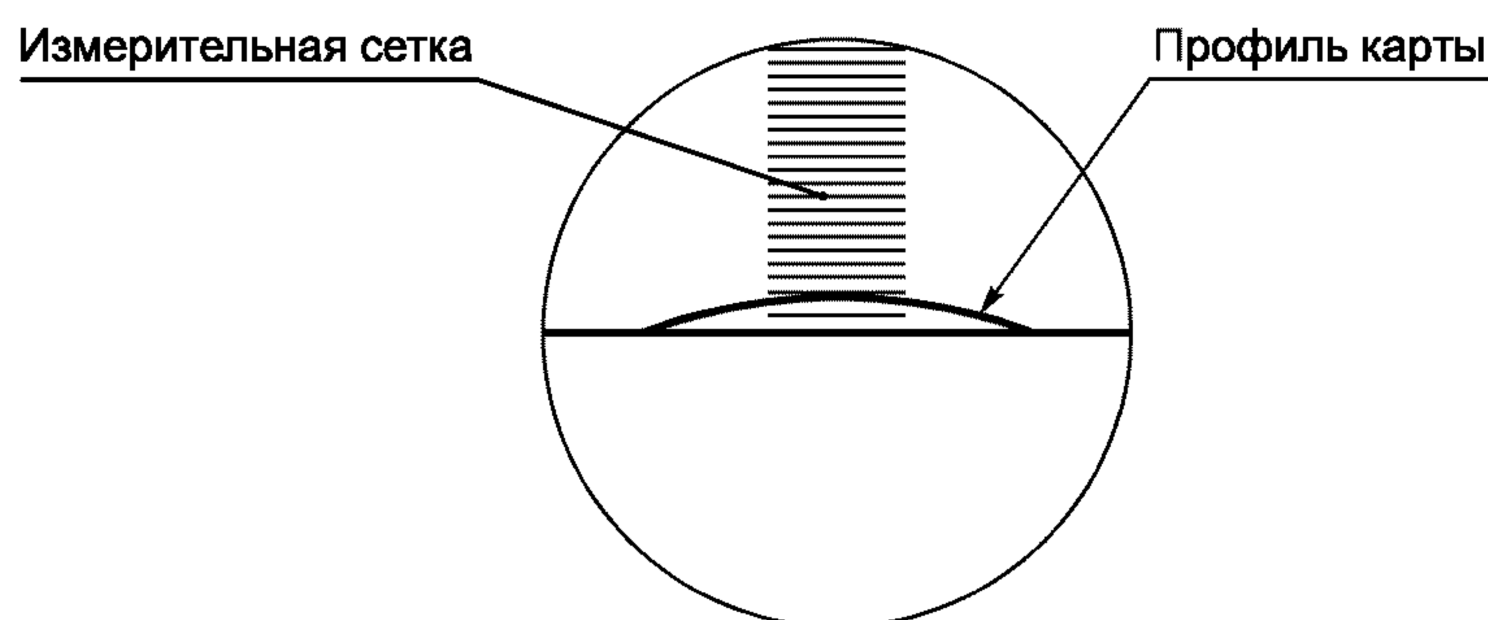
Рисунок 1 — Изображение в проекционном приборе при измерении коробления
