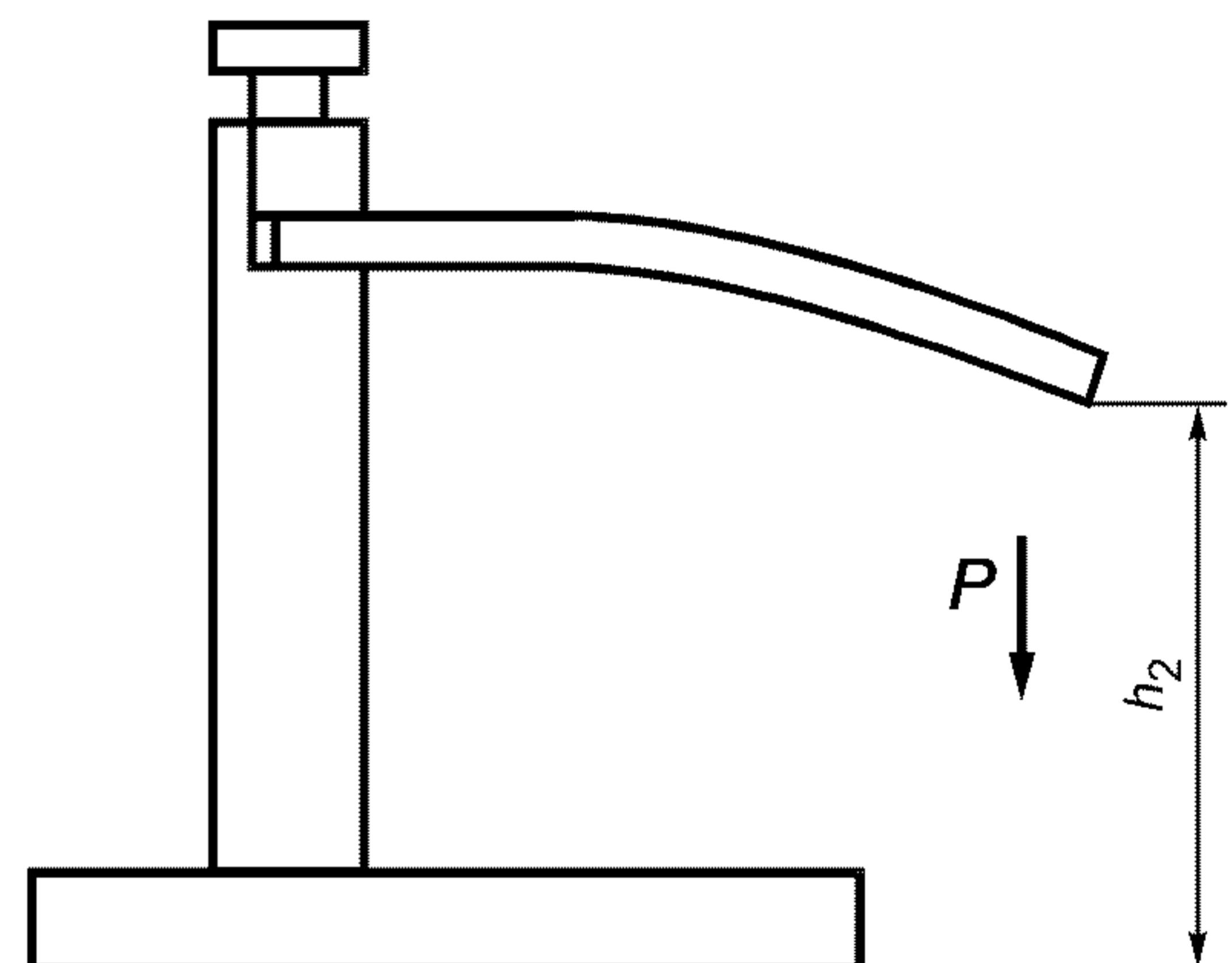
Рисунок 8 — Карта в зажимном устройстве во время нагрузки
