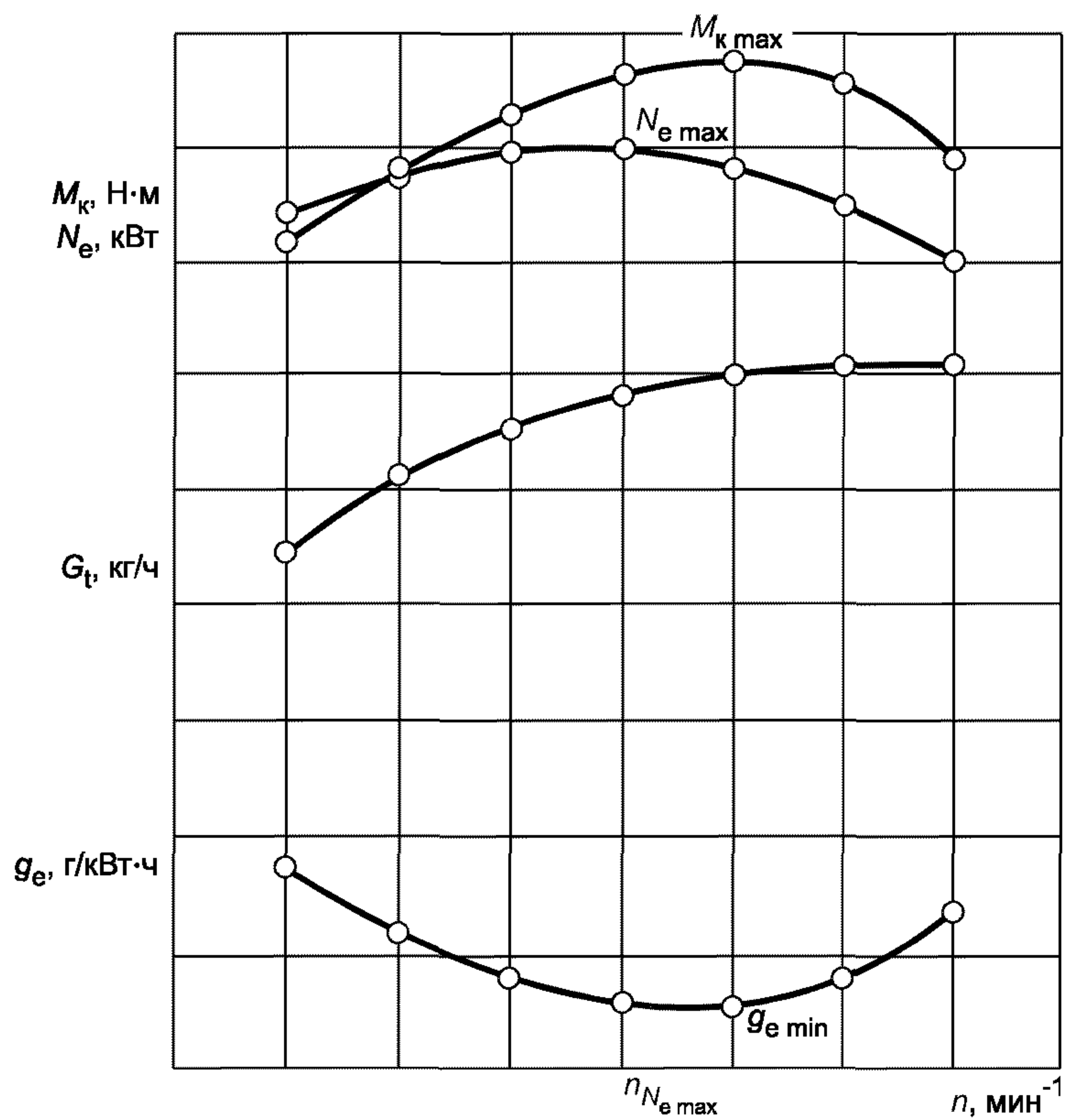
Рисунок Б.1 — Внешняя скоростная характеристика двигателя бензоинструмента
