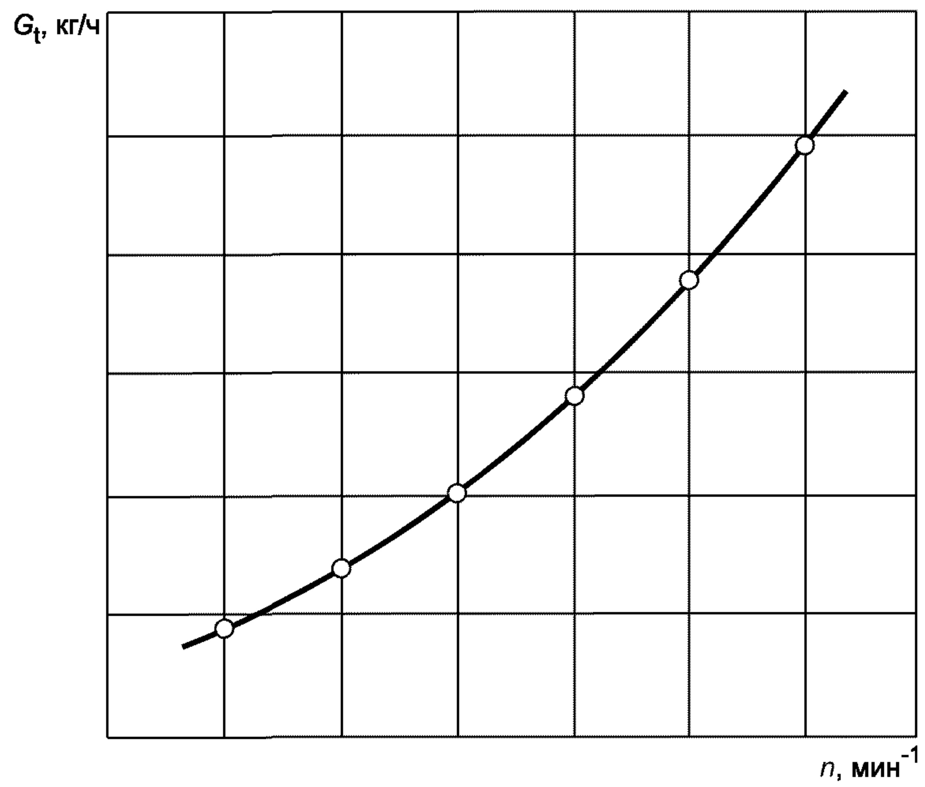
Рисунок Б.3 — Характеристика холостого хода бензоинструмента
