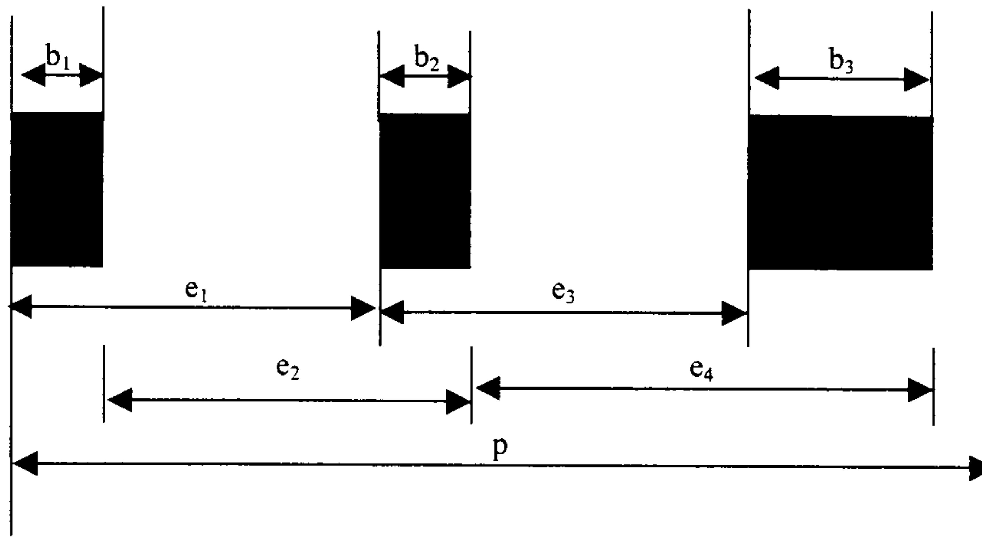
Рисунок 5 — Декодирование размеров
