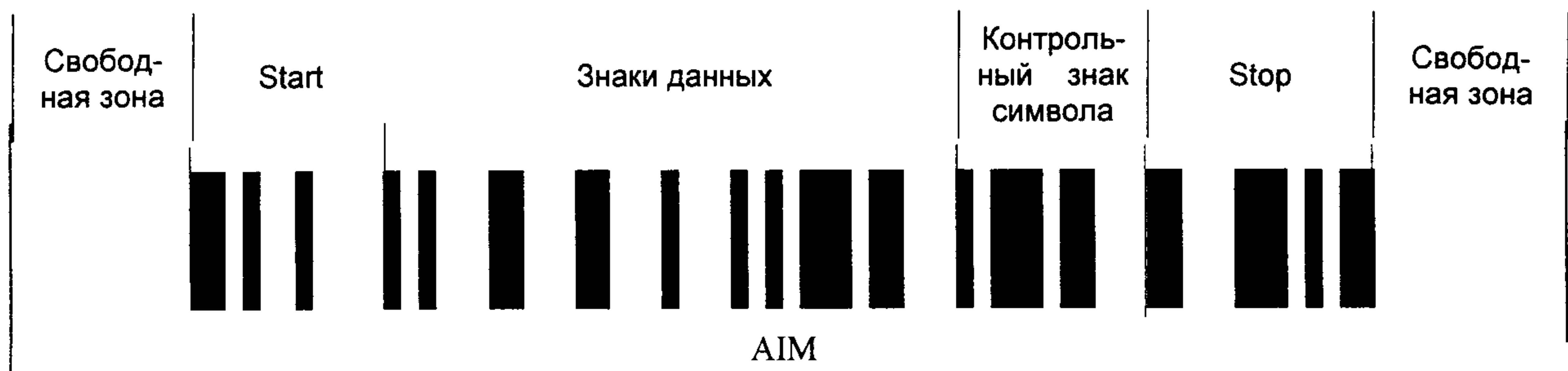
Рисунок 1 — Символ Code 128
