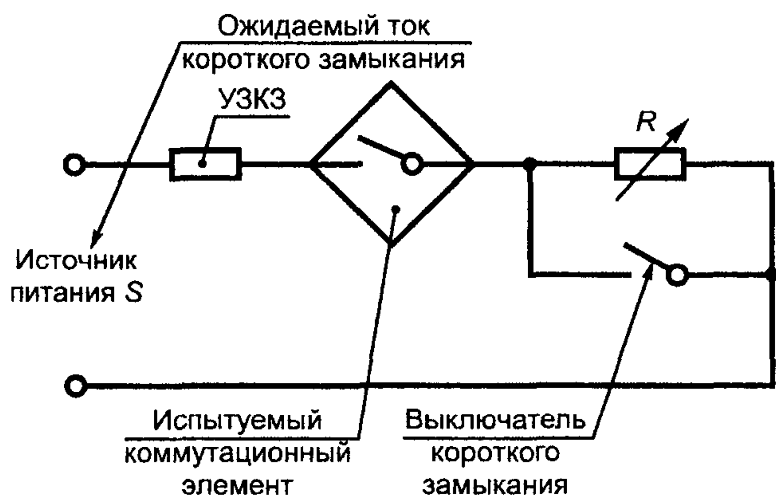
Рисунок Н 3 — Испытание на короткое замыкание
