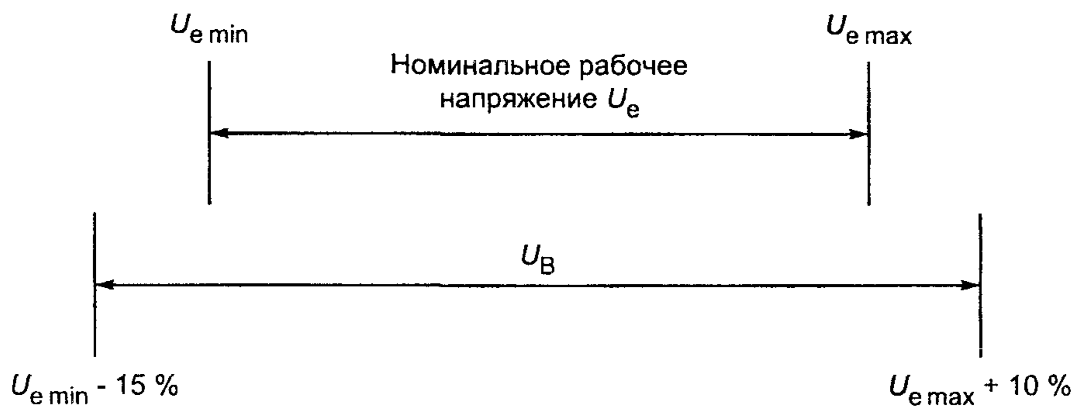
Рисунок Н.1 — Соотношение между U_e и U_B
