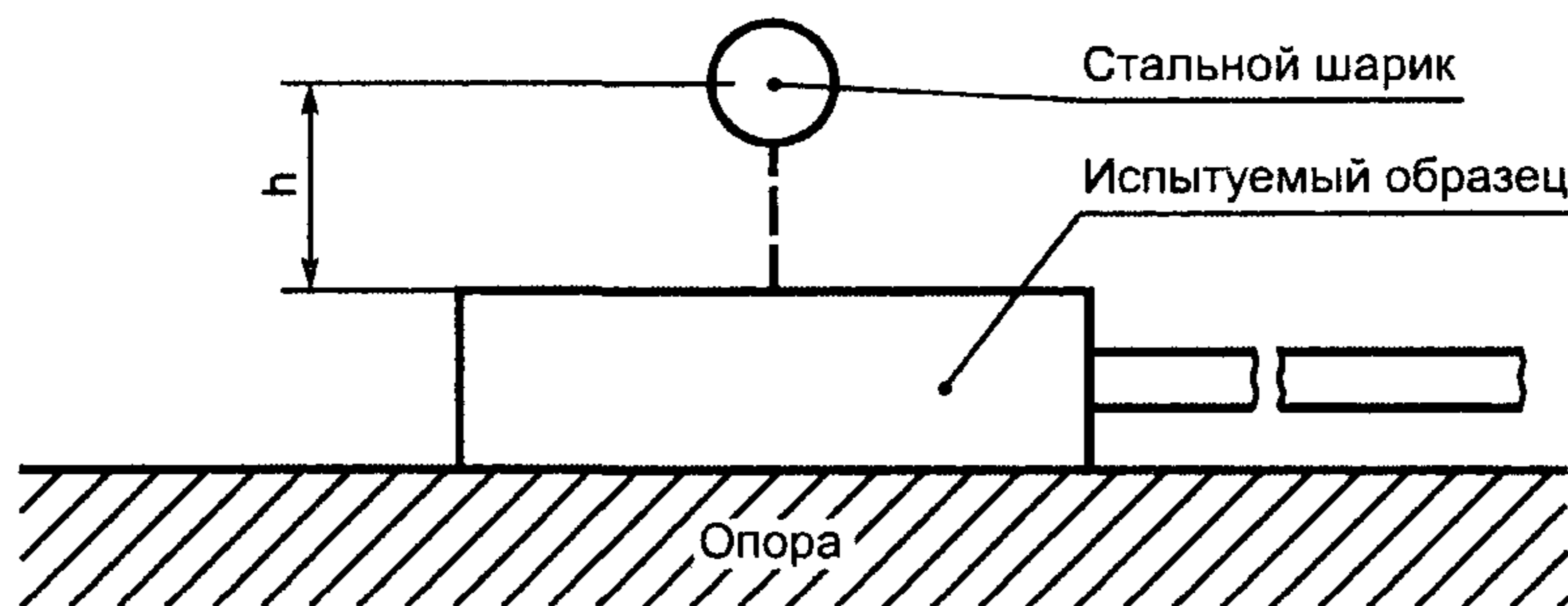
Рисунок Ф.2 — Испытательная установка
