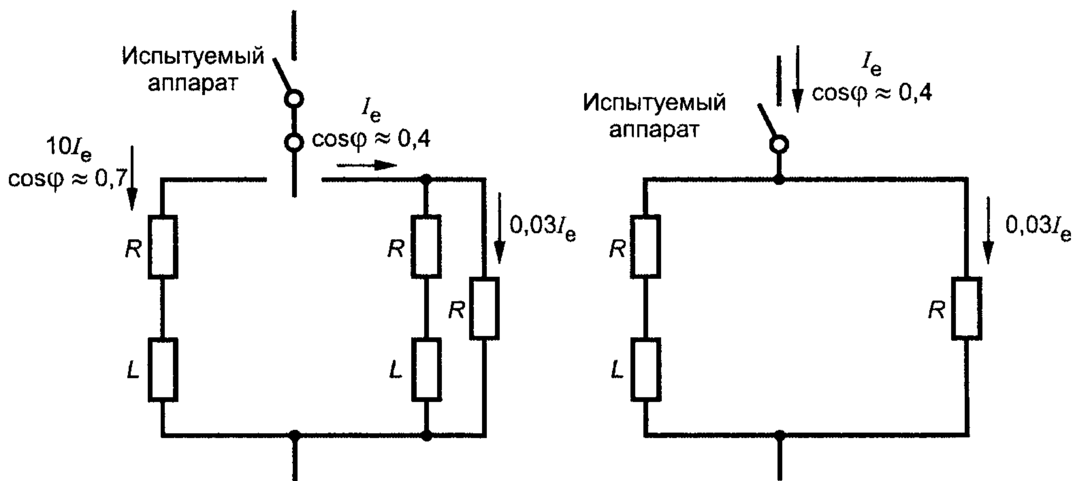
Рисунок С.1 — Полная схема (см. С.3.2.1)
