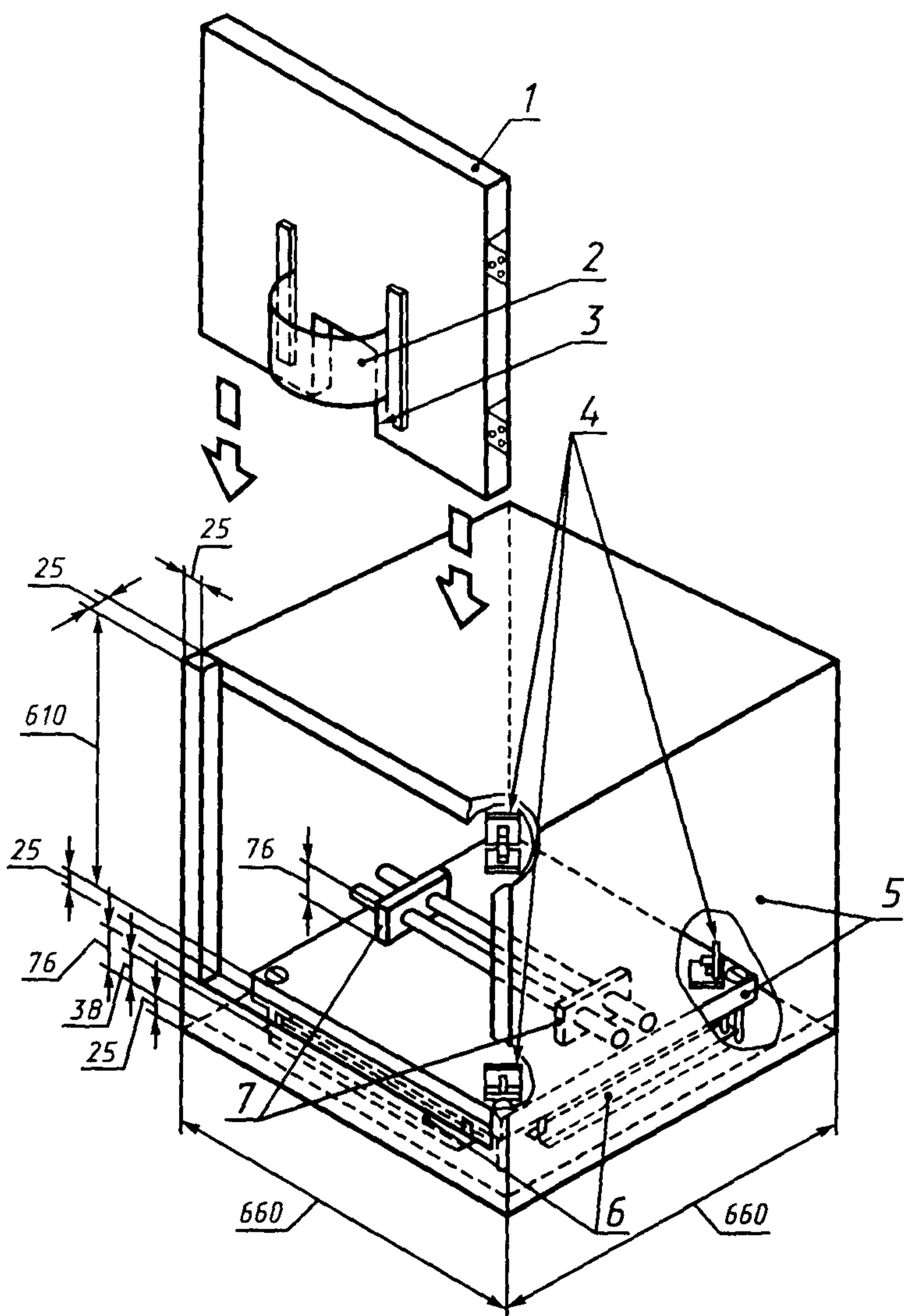
1 — шарнирная дверь, 2 — радиальный алюминиевый экран диаметром 89 мм, 3 — отверстие 150 × 150 мм в камере, 4 — термопары, 5 — терлостойкий материал, 6 — нагреватели, 7 — подставка для ПРА
