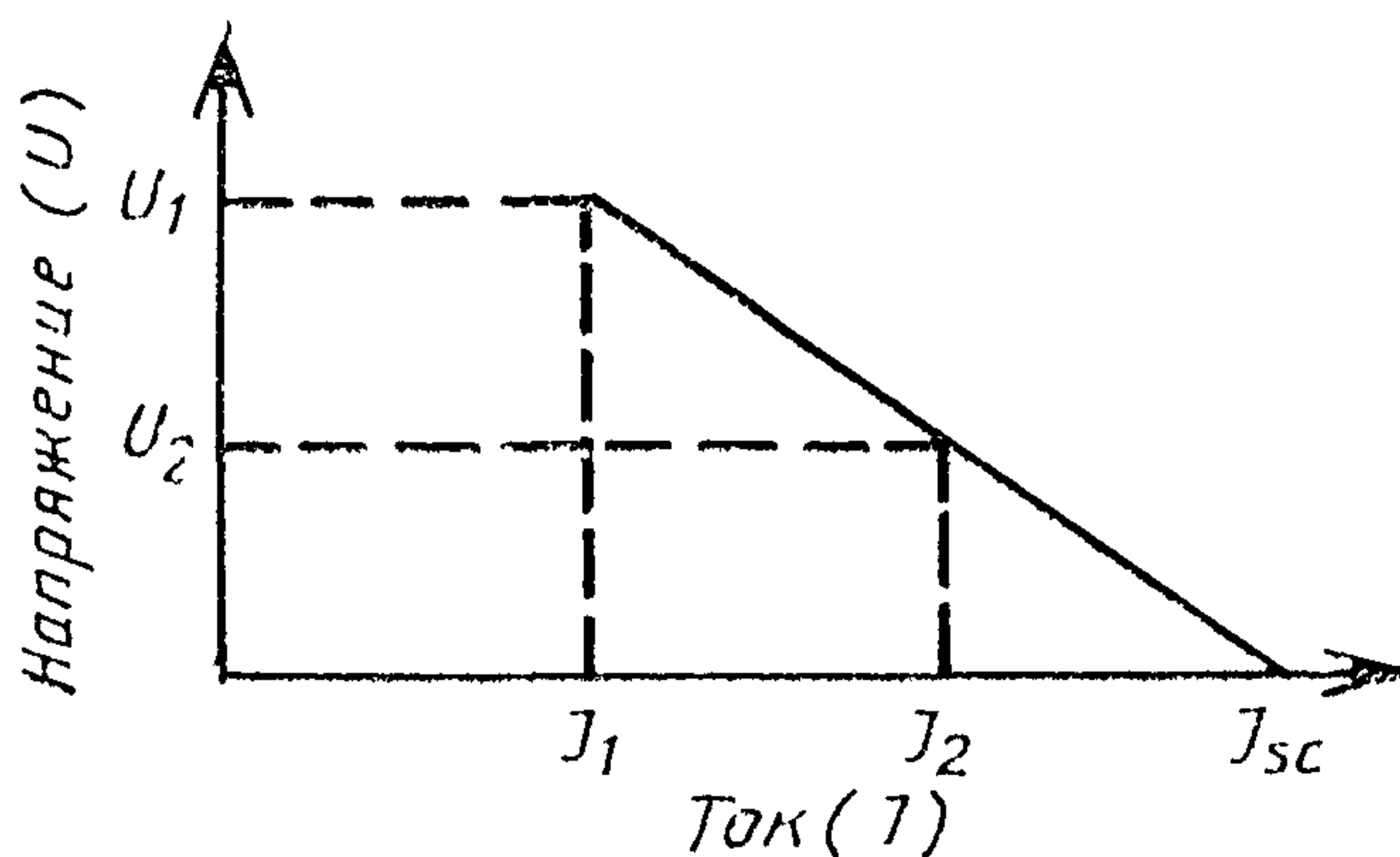
Рисунок 1 — Разрядная характеристика U=f(I)
