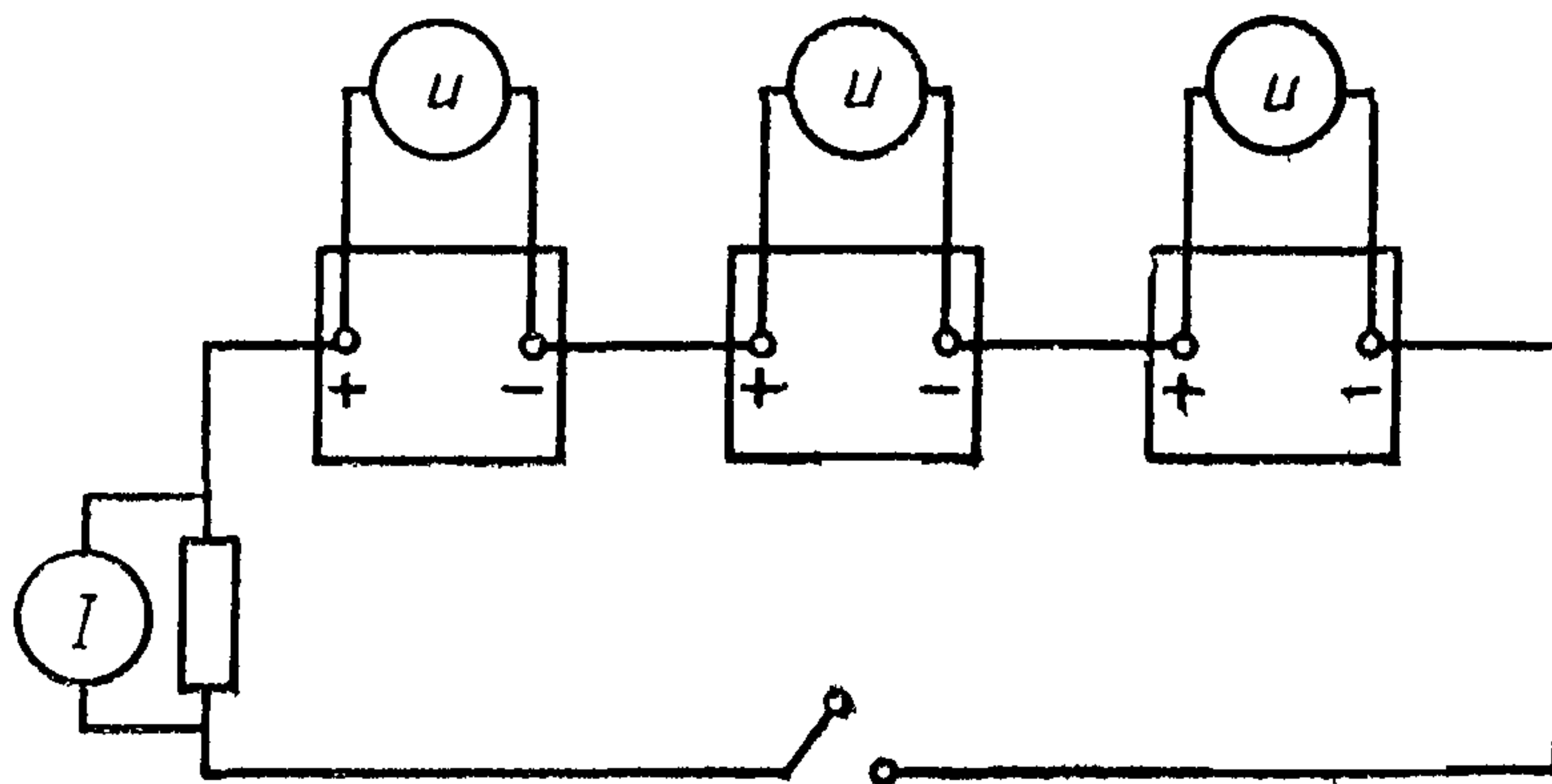
Рисунок 2 — Схема соединения
