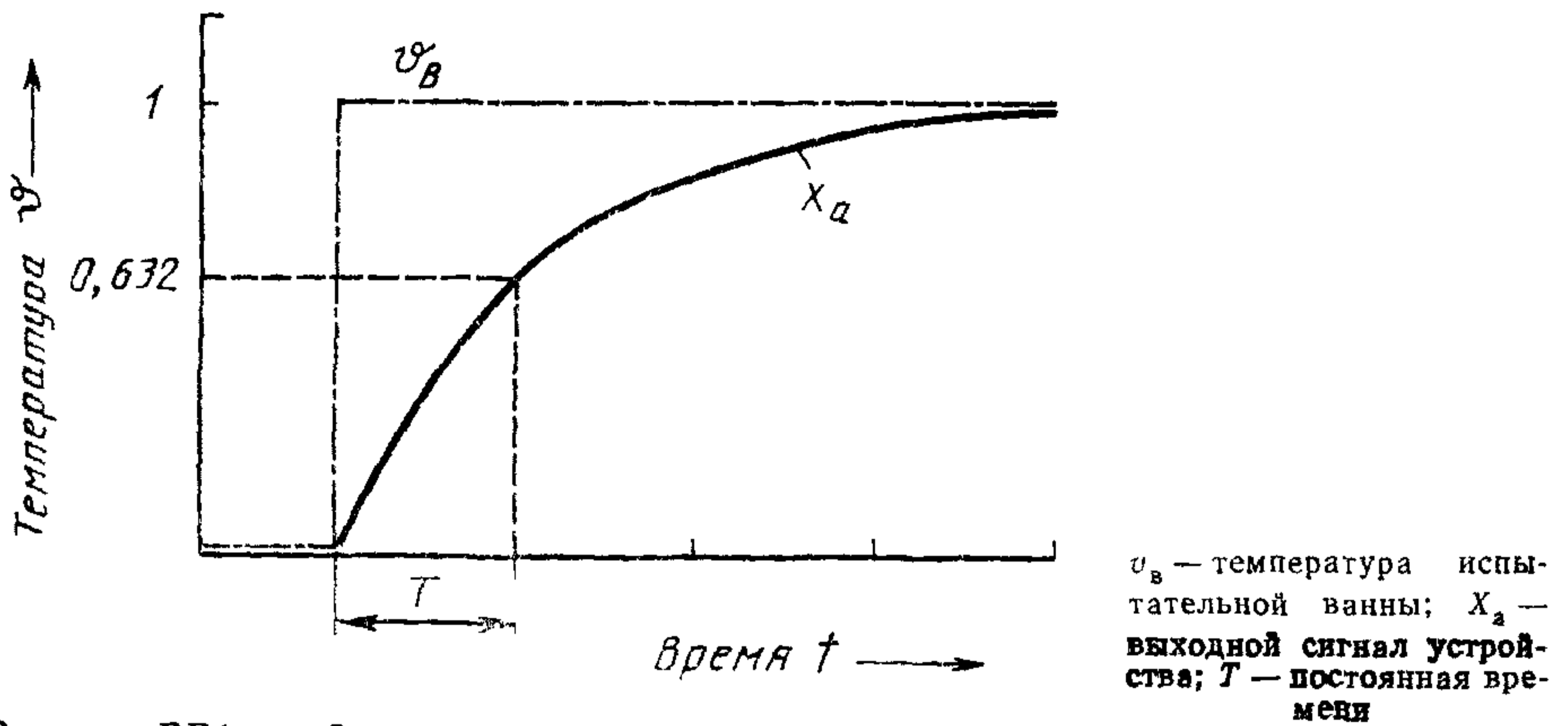
Рисунок ВВ1 — Определение постоянной времени методом быстрого изменения температуры
