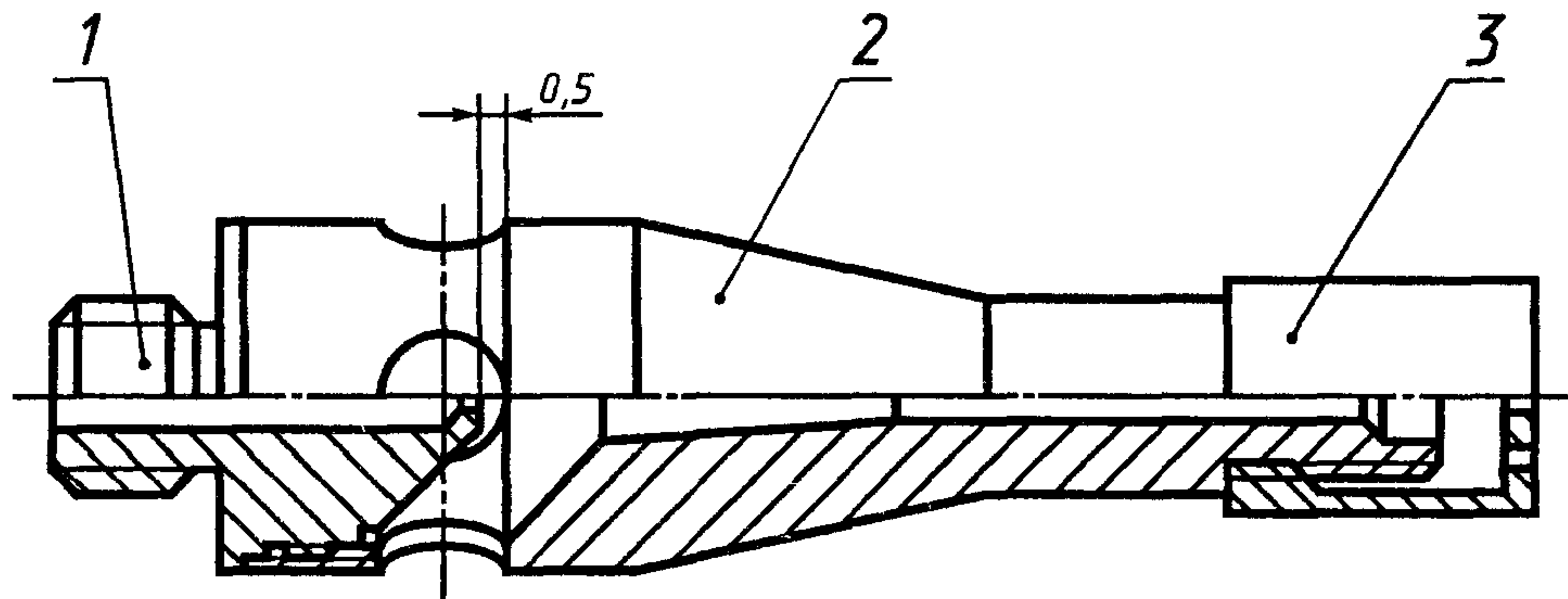
1 — газовая форсунка; 2 — трубка горелки; 3 — стабилизатор пламени
