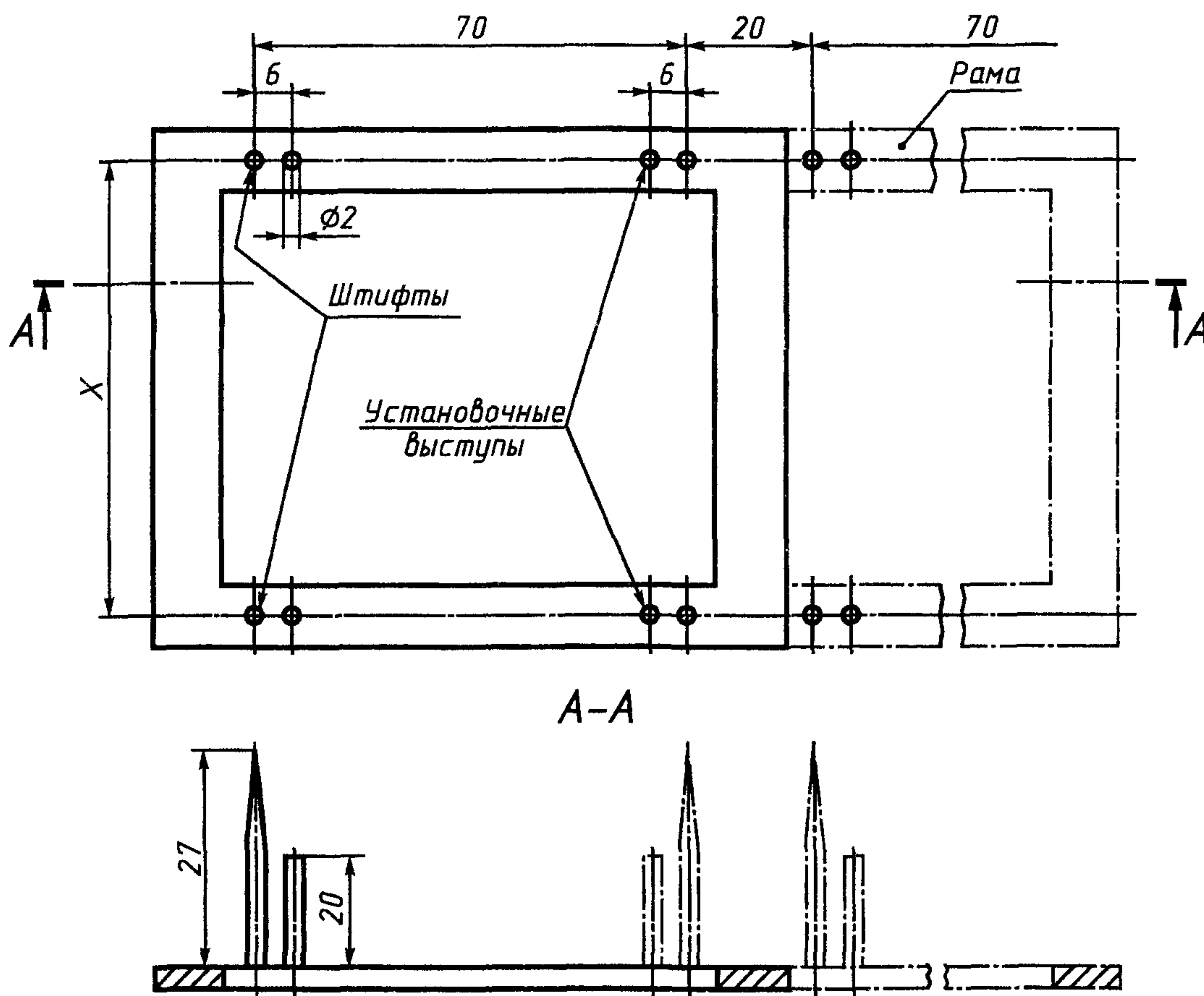
Рисунок 1 — Держатель для элементарной пробы
