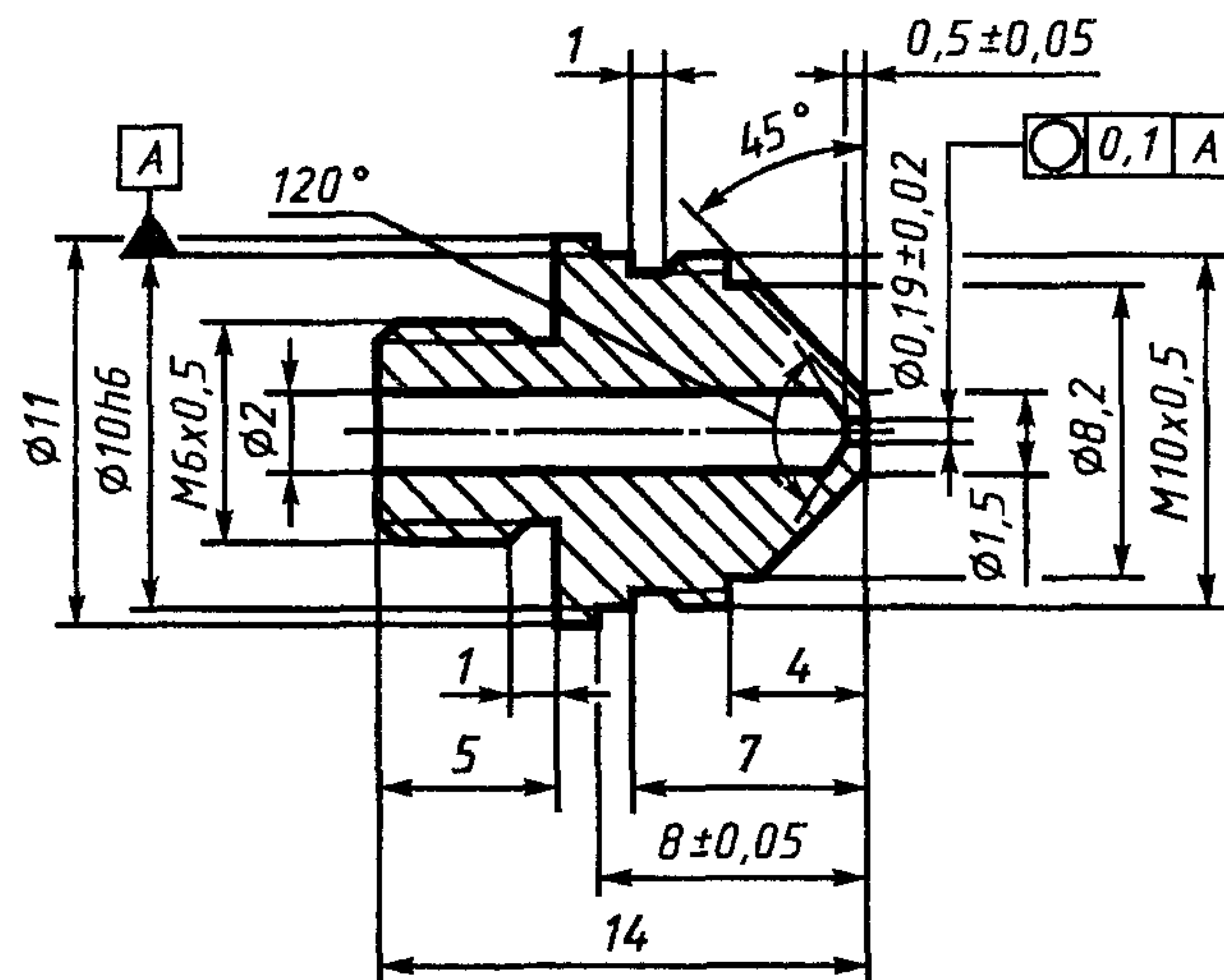
Рисунок Б.2 — Газовая форсунка
