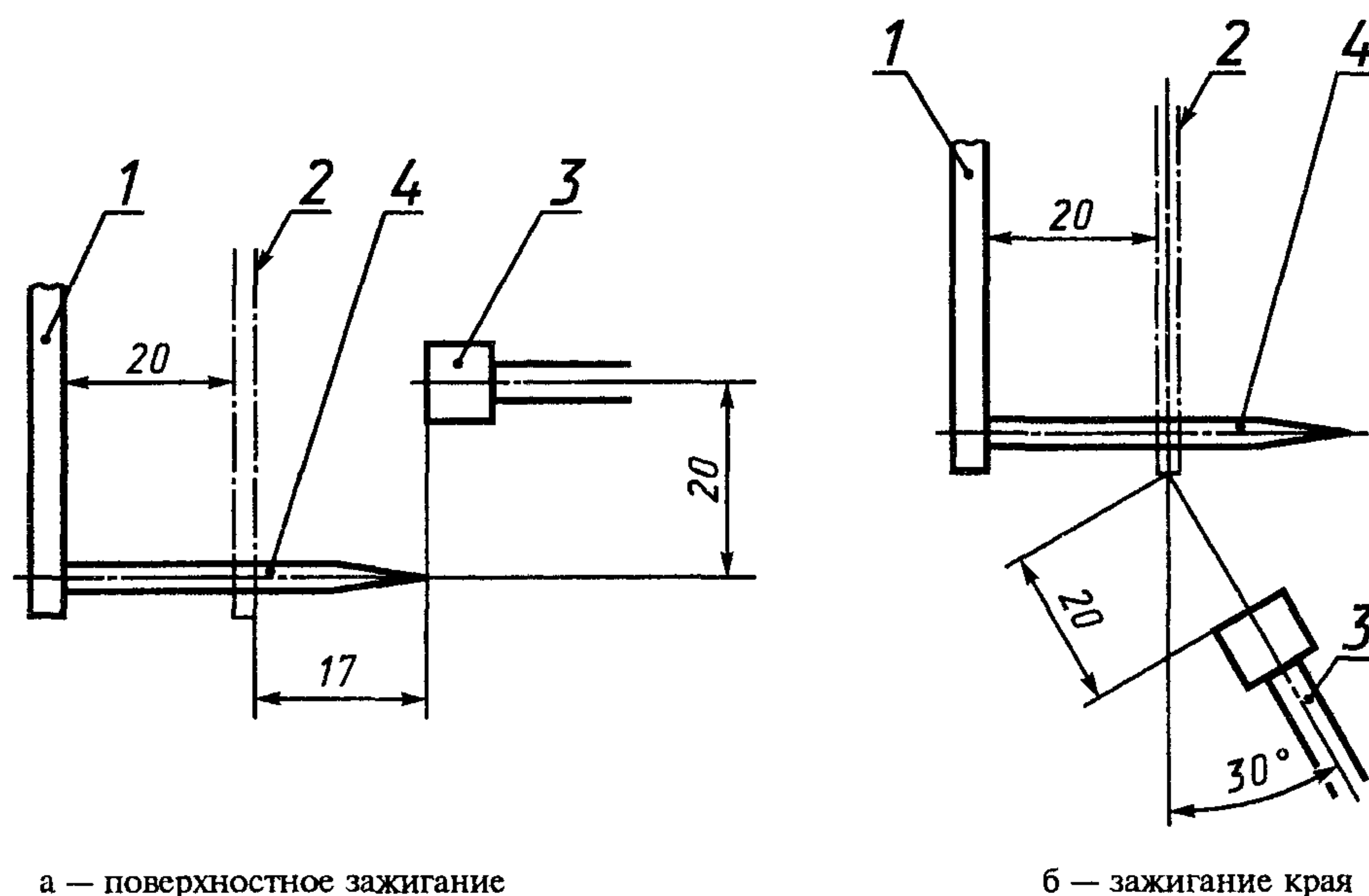
1 — рама держателя; 2 — элементарная проба; 3 — горелка; 4 — штифт
