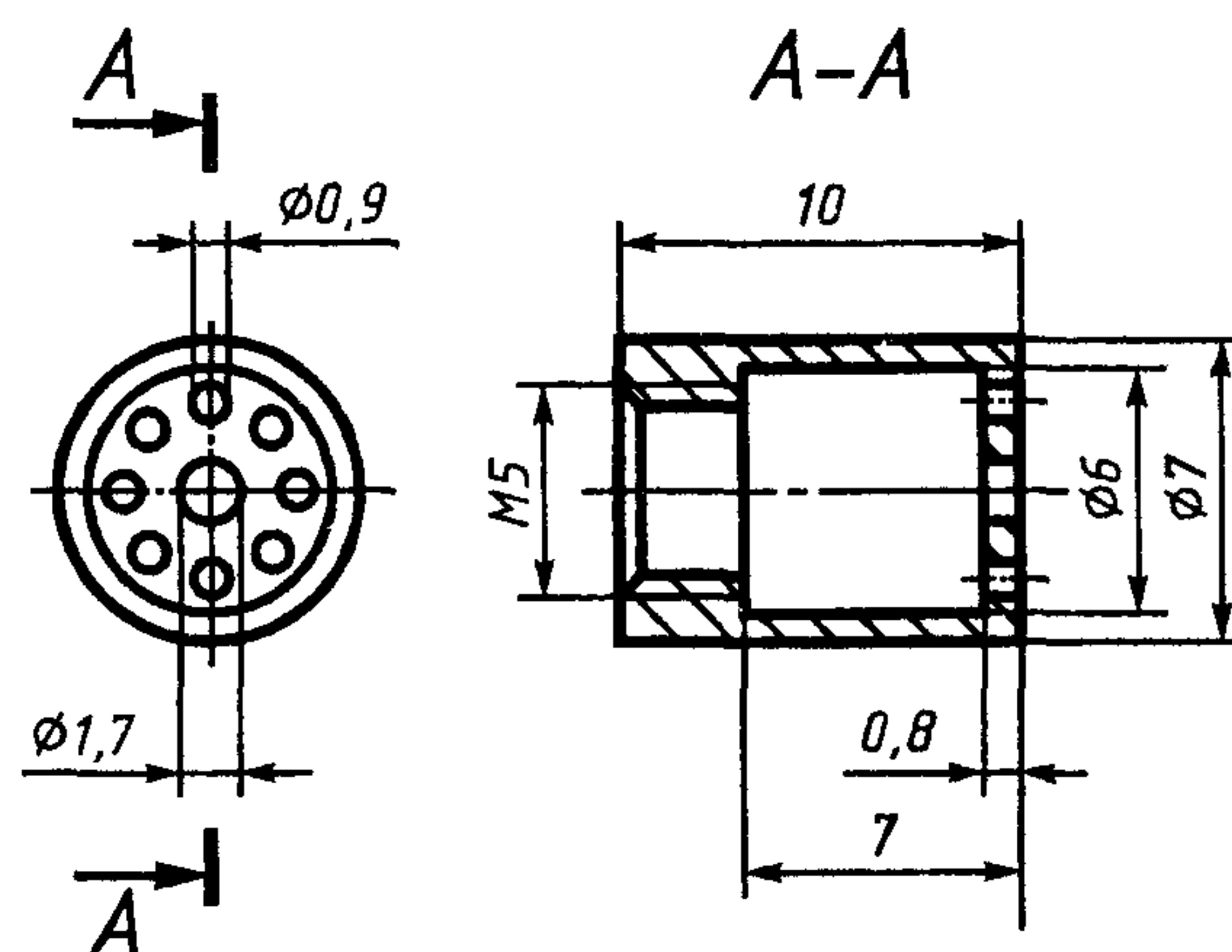
Рисунок Б.4 — Стабилизатор пламени
