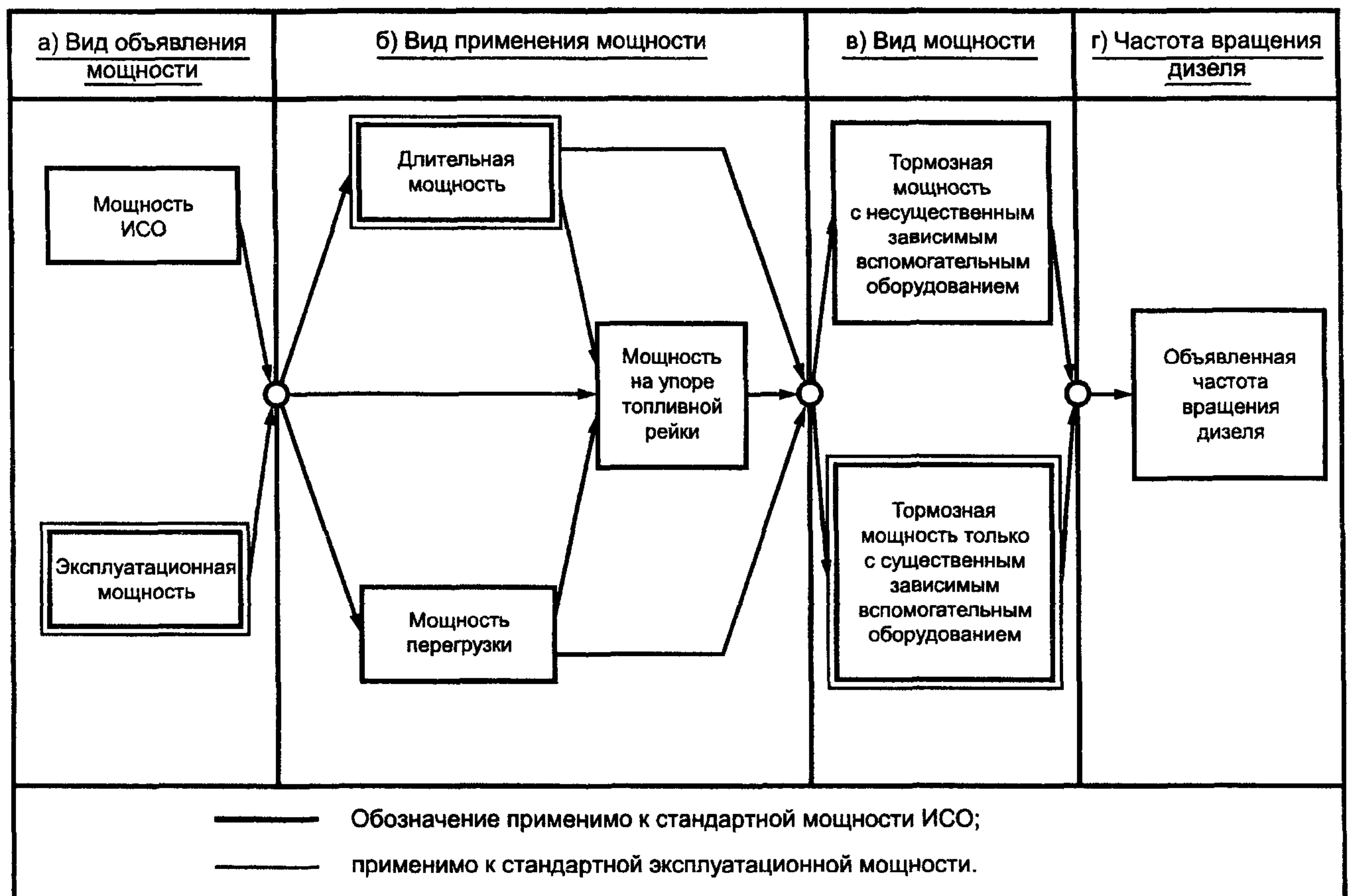
Рисунок 1 — Диаграмма, показывающая способы обозначения мощности
