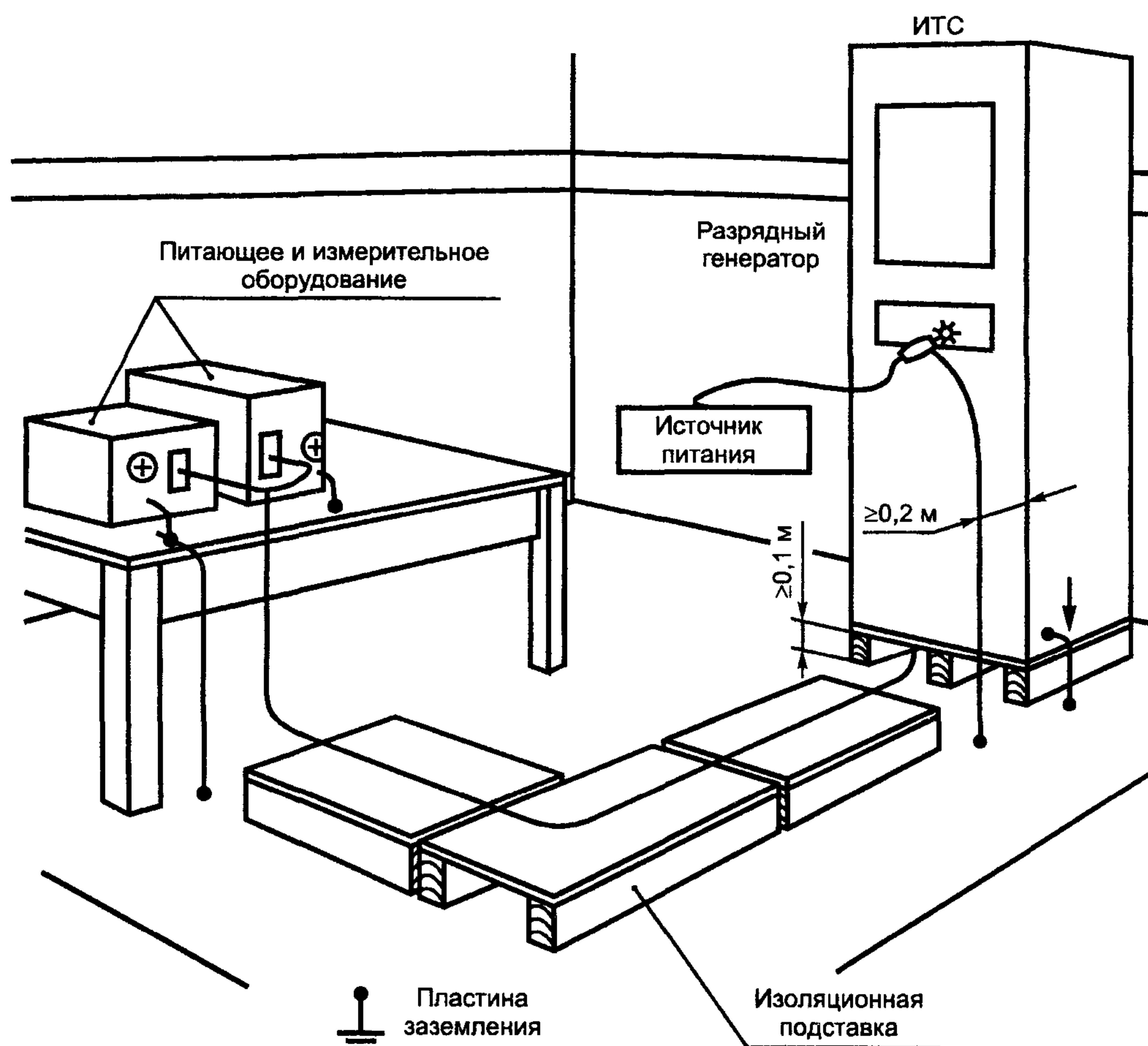
Рисунок 3 — Пример рабочего места для испытаний
