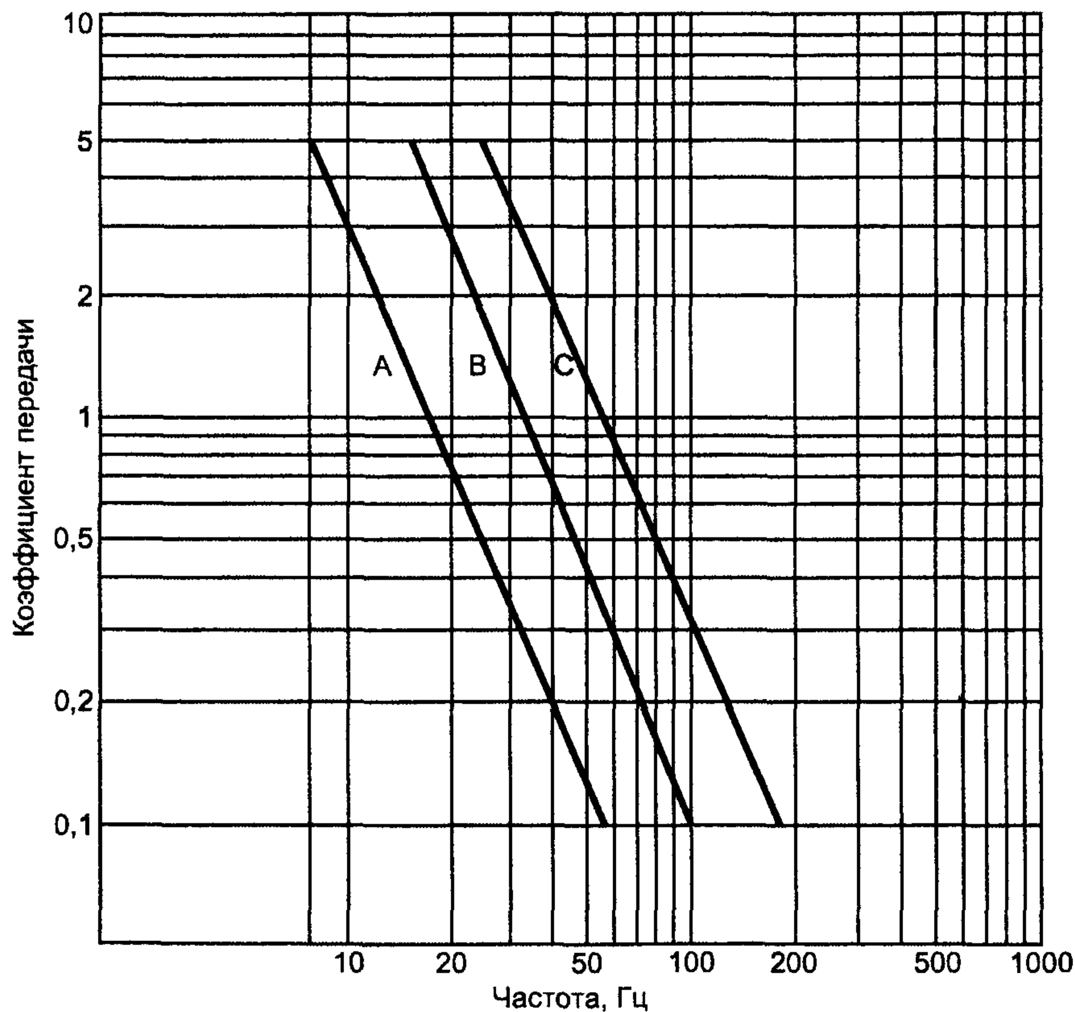
Рисунок А.6 — Коэффициент передачи виброизолятора
