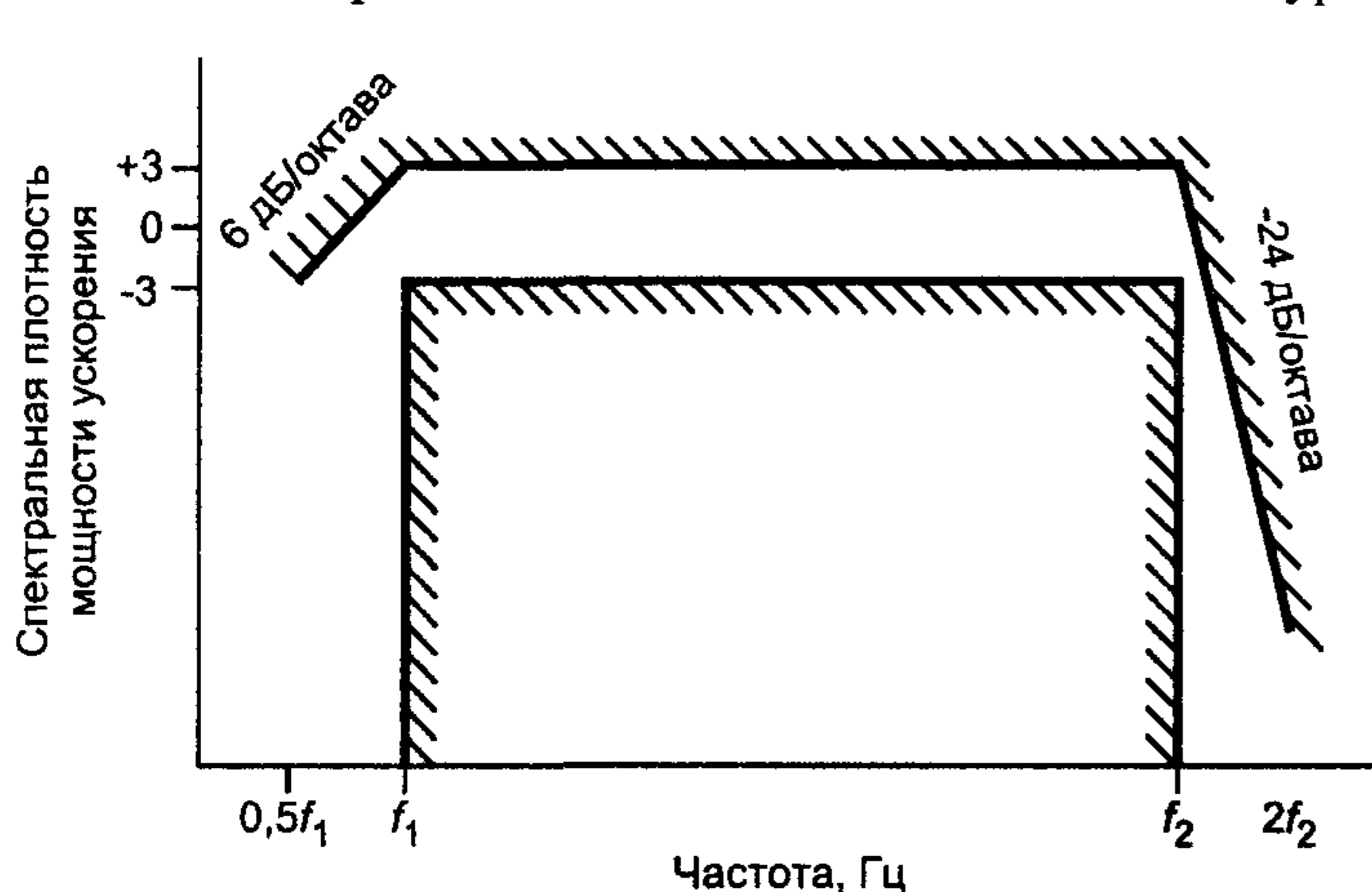
Рисунок 2 — Границы допуска для спектральной плотности мощности ускорения
