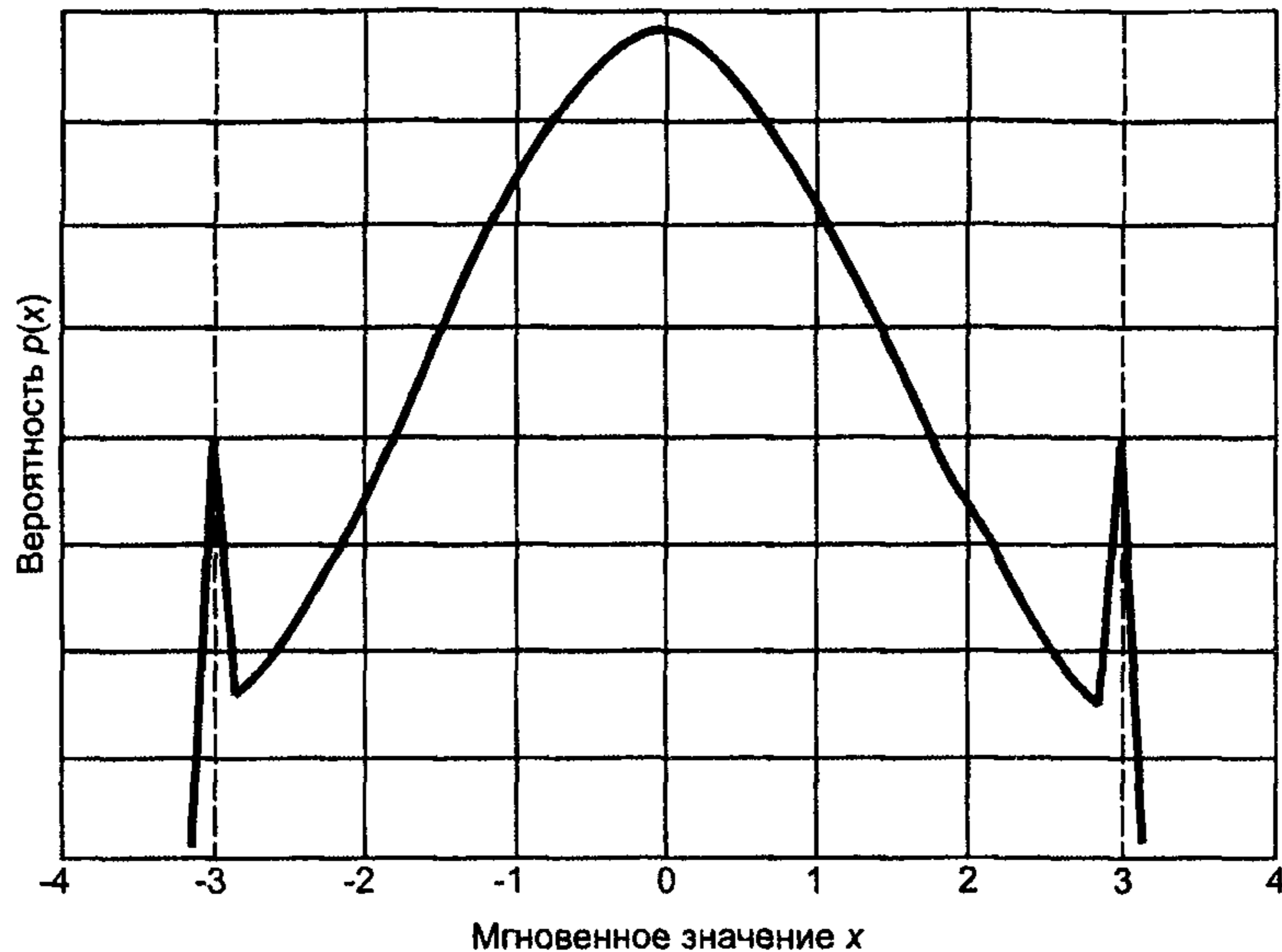
Рисунок А.3 — Негассовская плотность вероятности распределения
