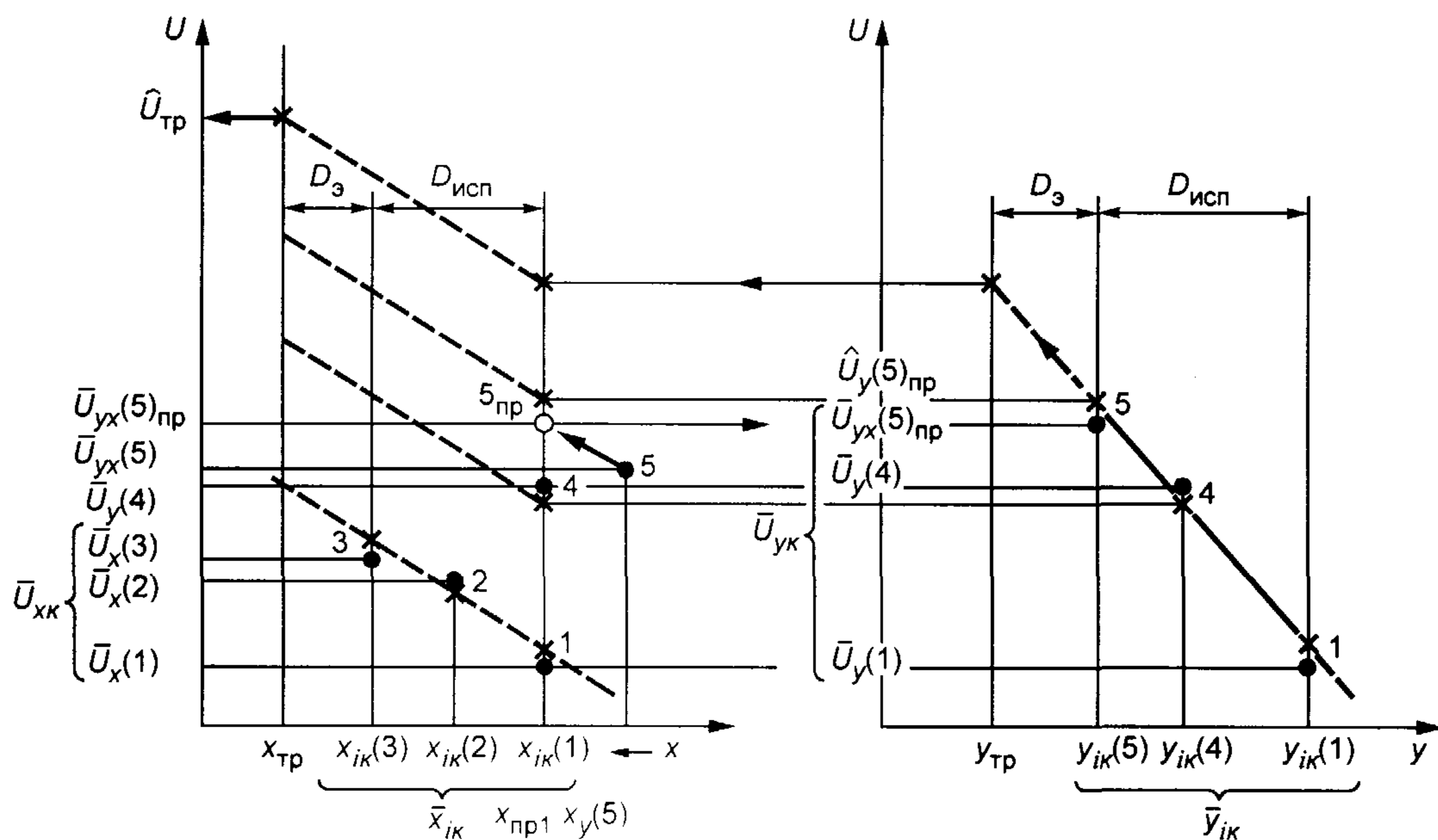
Рисунок А.2 — Схема эксперимента по варианту 2
