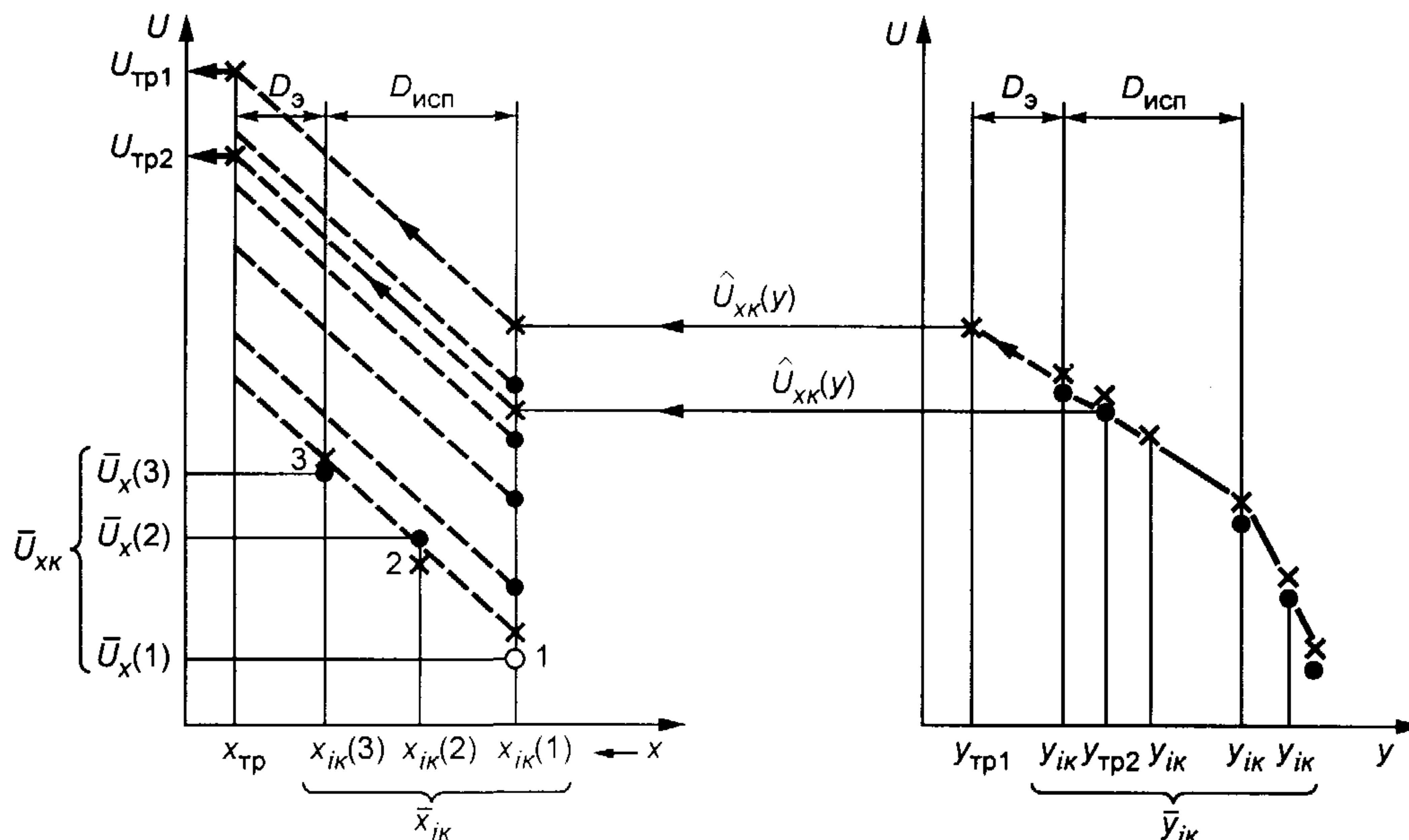
Рисунок А.4 — Схема эксперимента по варианту 4
