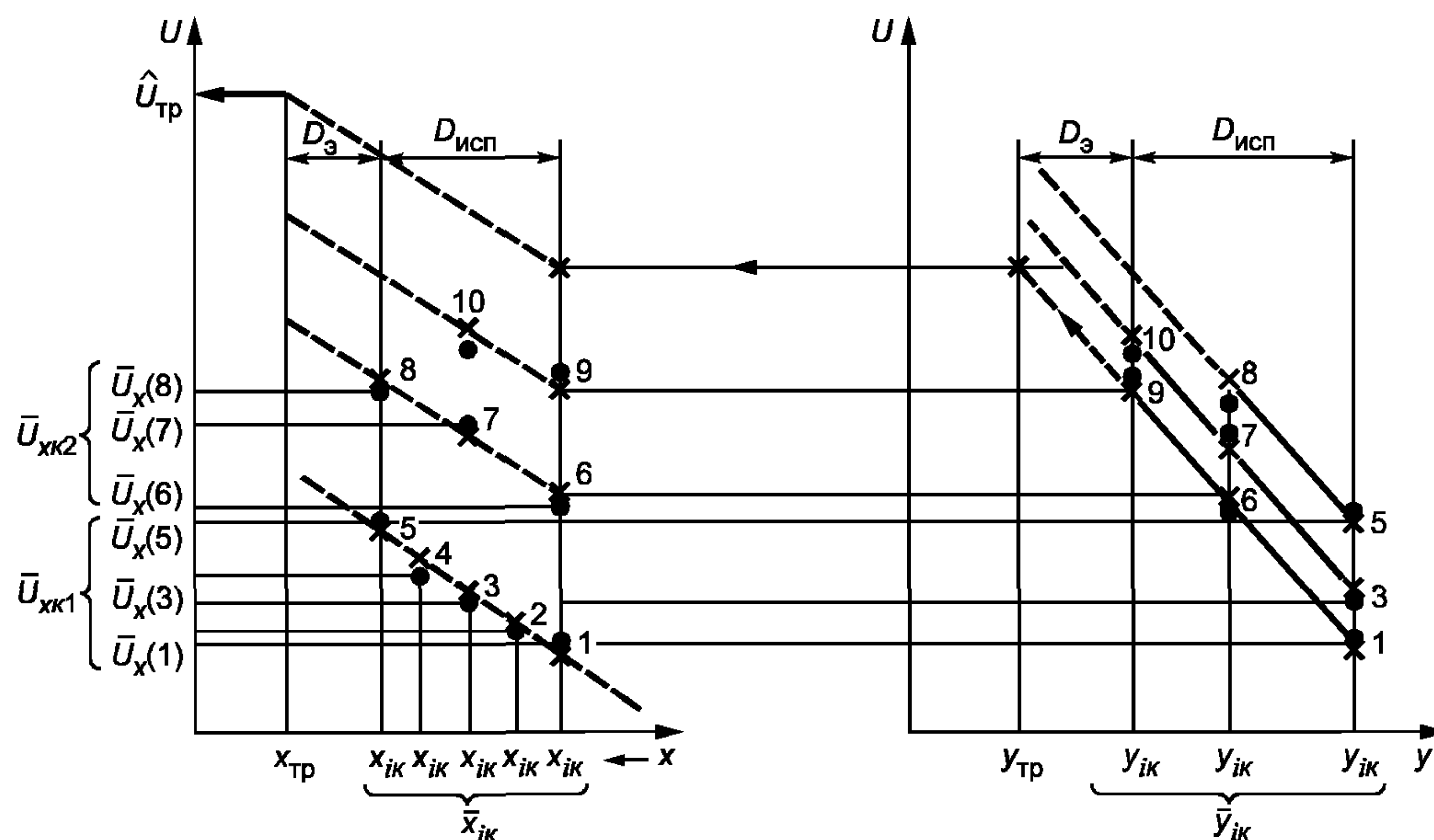
Рисунок А.3 — Схема эксперимента по варианту 3
