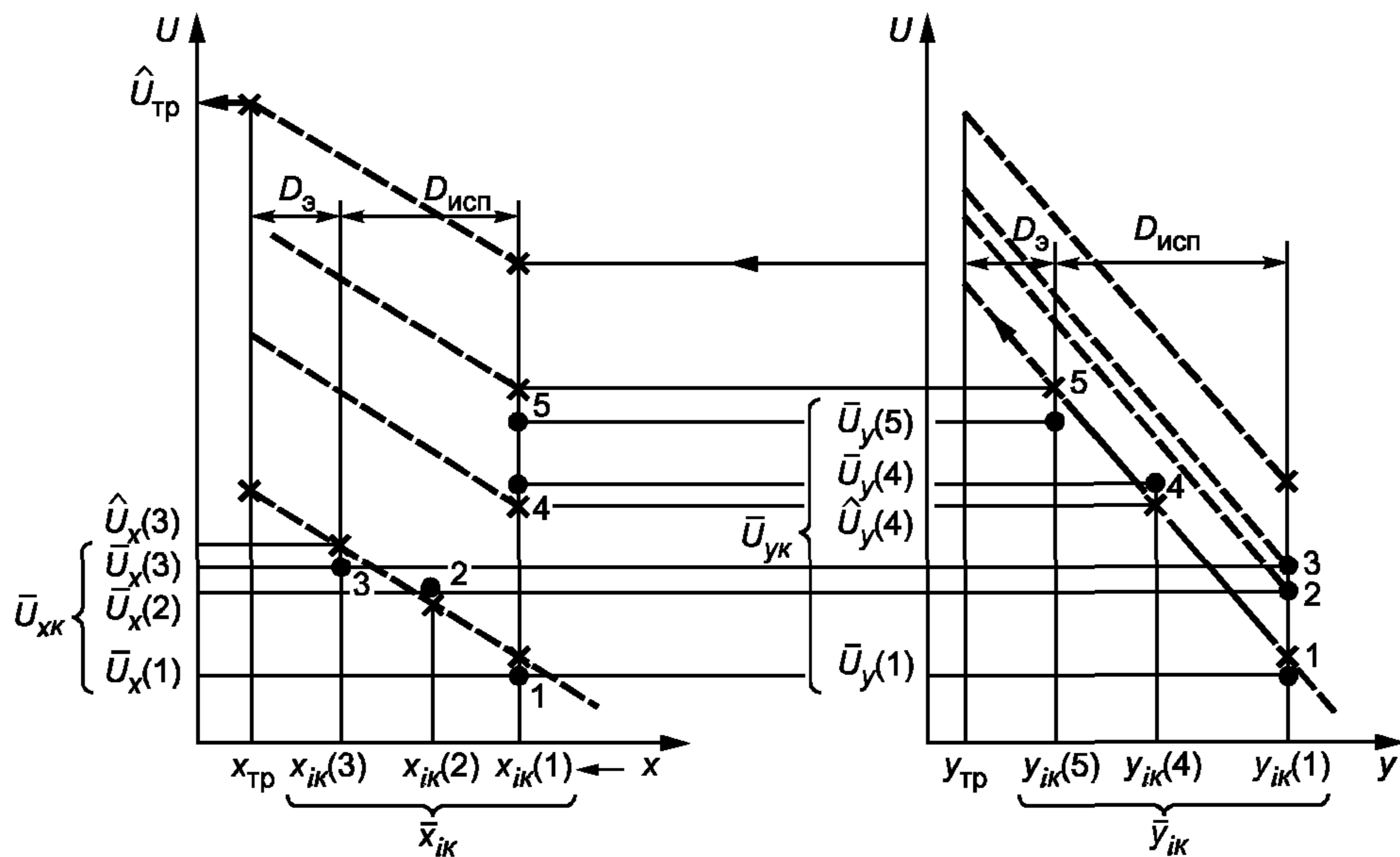
Рисунок А.1 — Схема эксперимента по варианту 1
