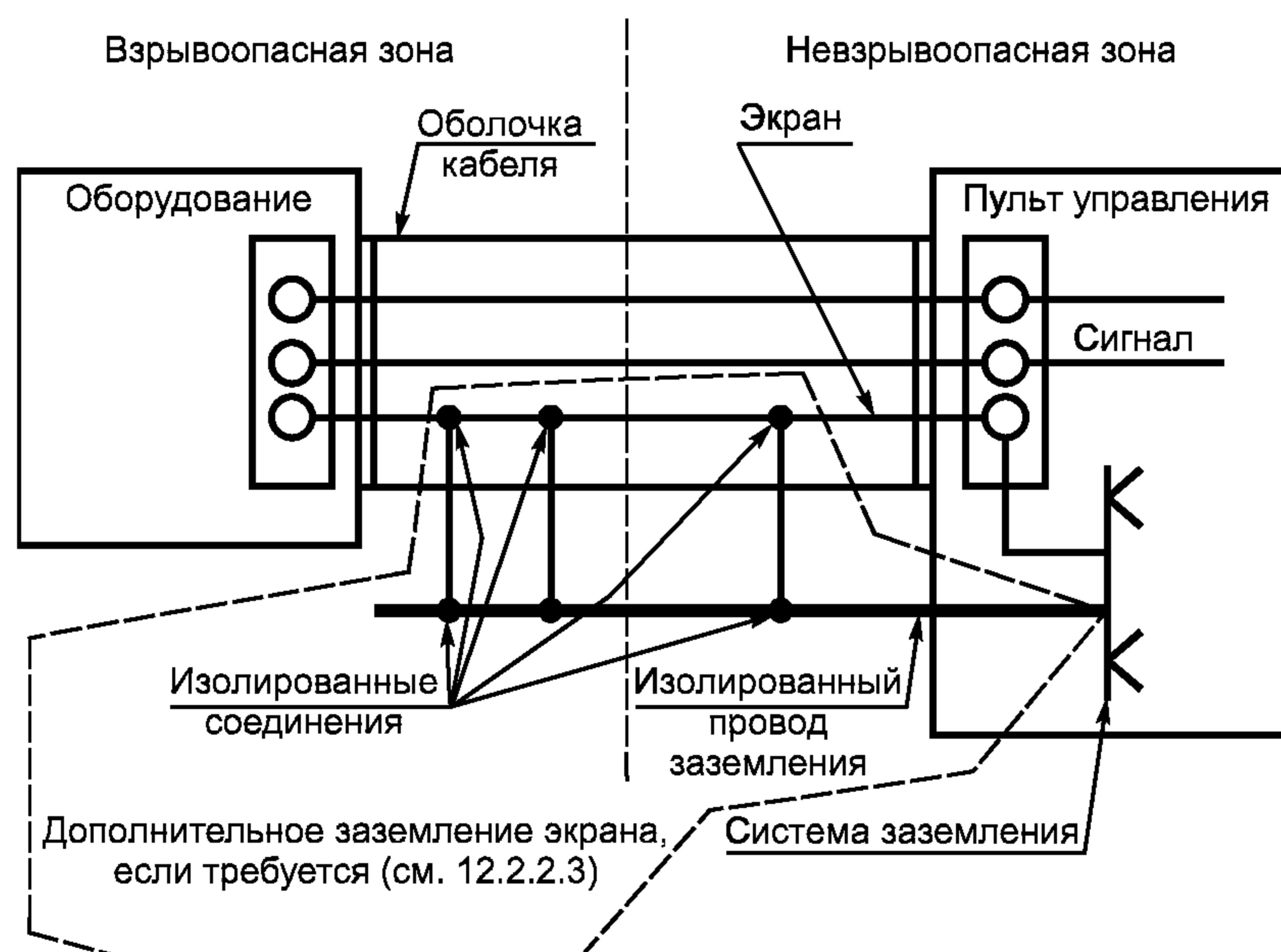
Рисунок 2 — Заземление проводящих экранов
