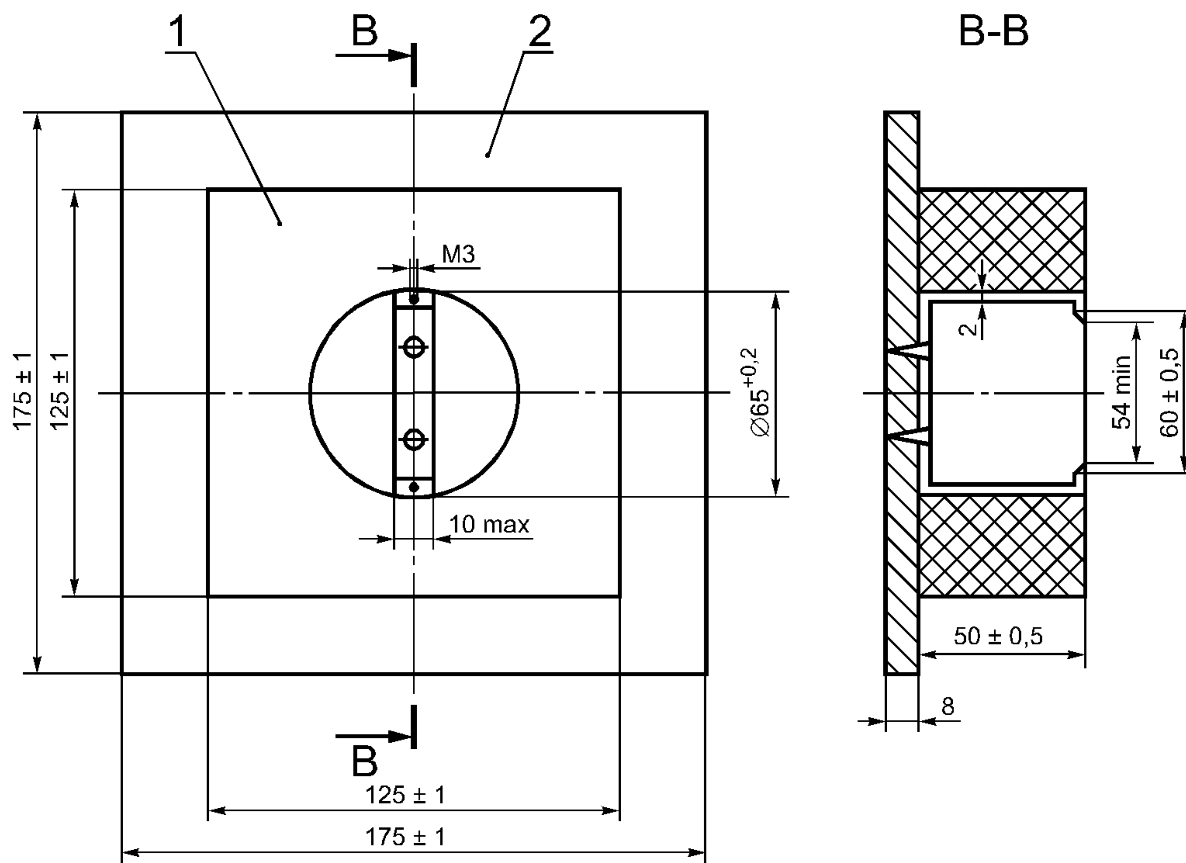
Рисунок 24 — Монтажная опора
