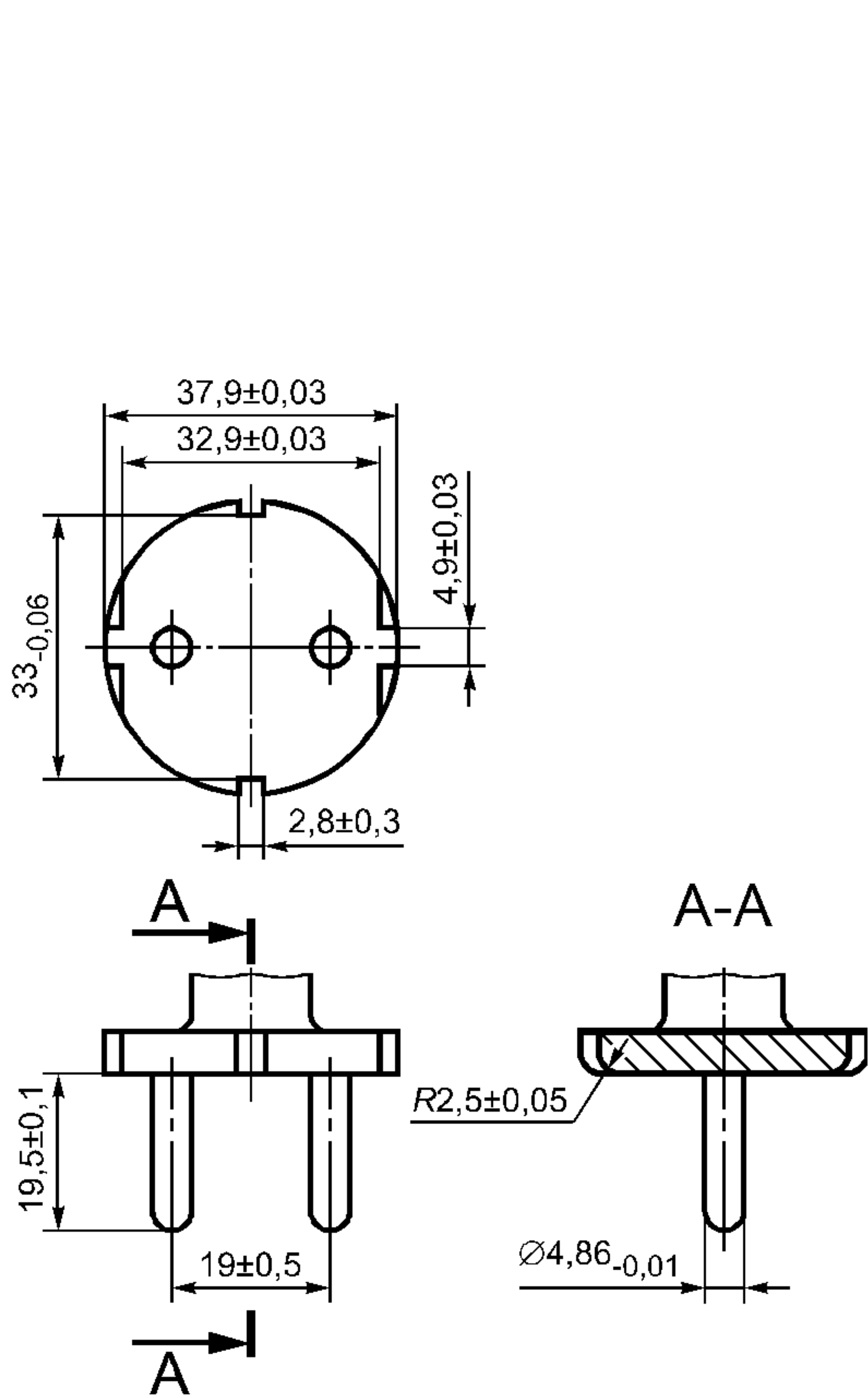
Рисунок Б.9 — Калибр для проверки размеров розеток и удлинителей с заземляющими боковыми контактами
