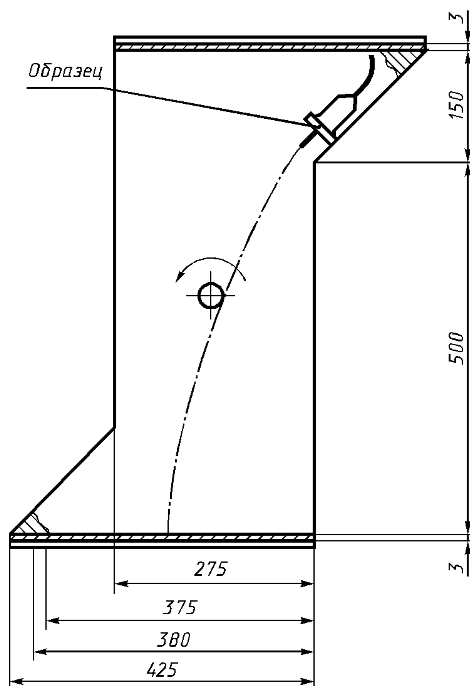
Рисунок 26 — Барабан для испытания соединителей на свободное падение
