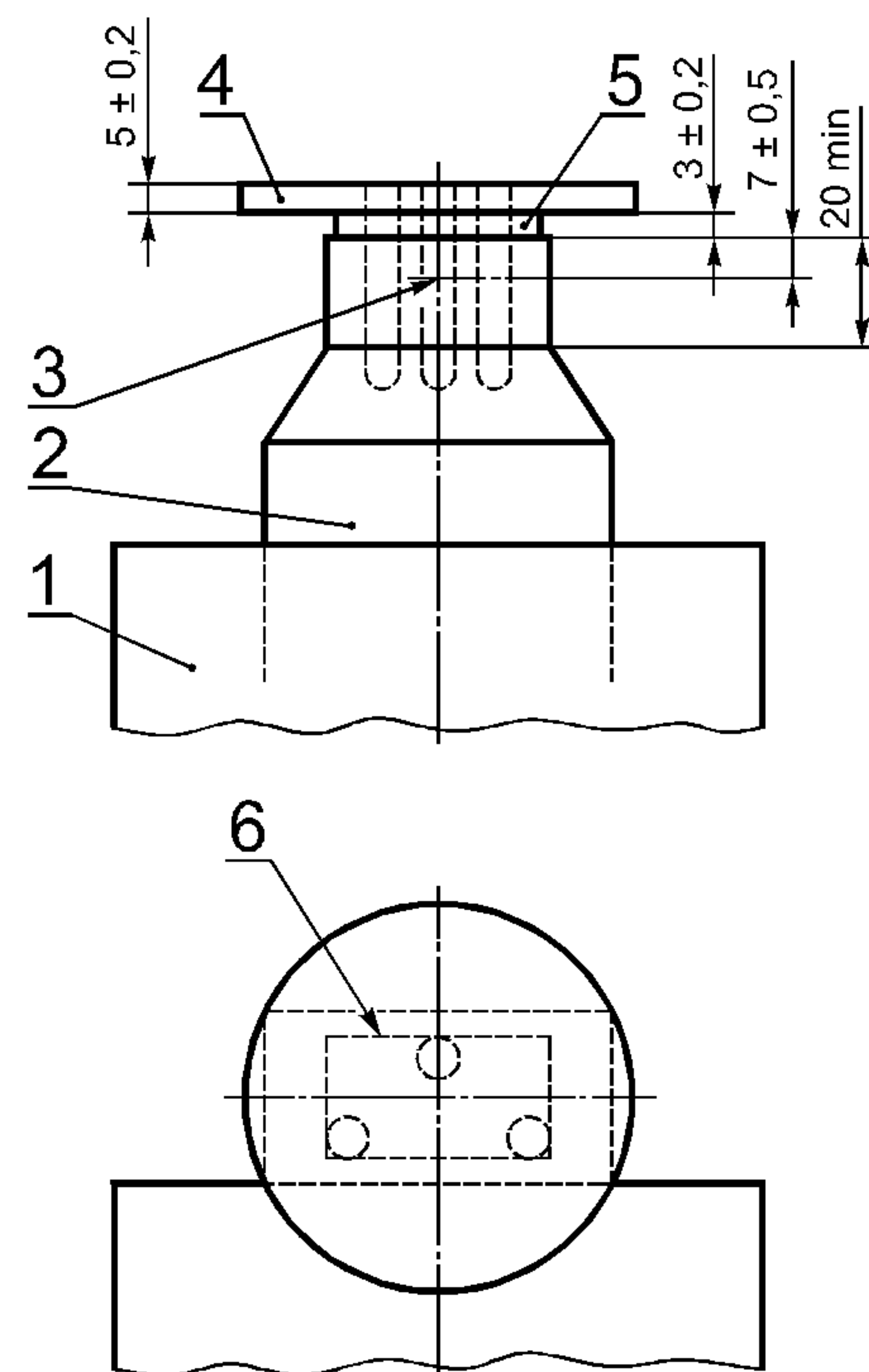
Рисунок 38 — Установка для испытания прочности материалов при нагревании
