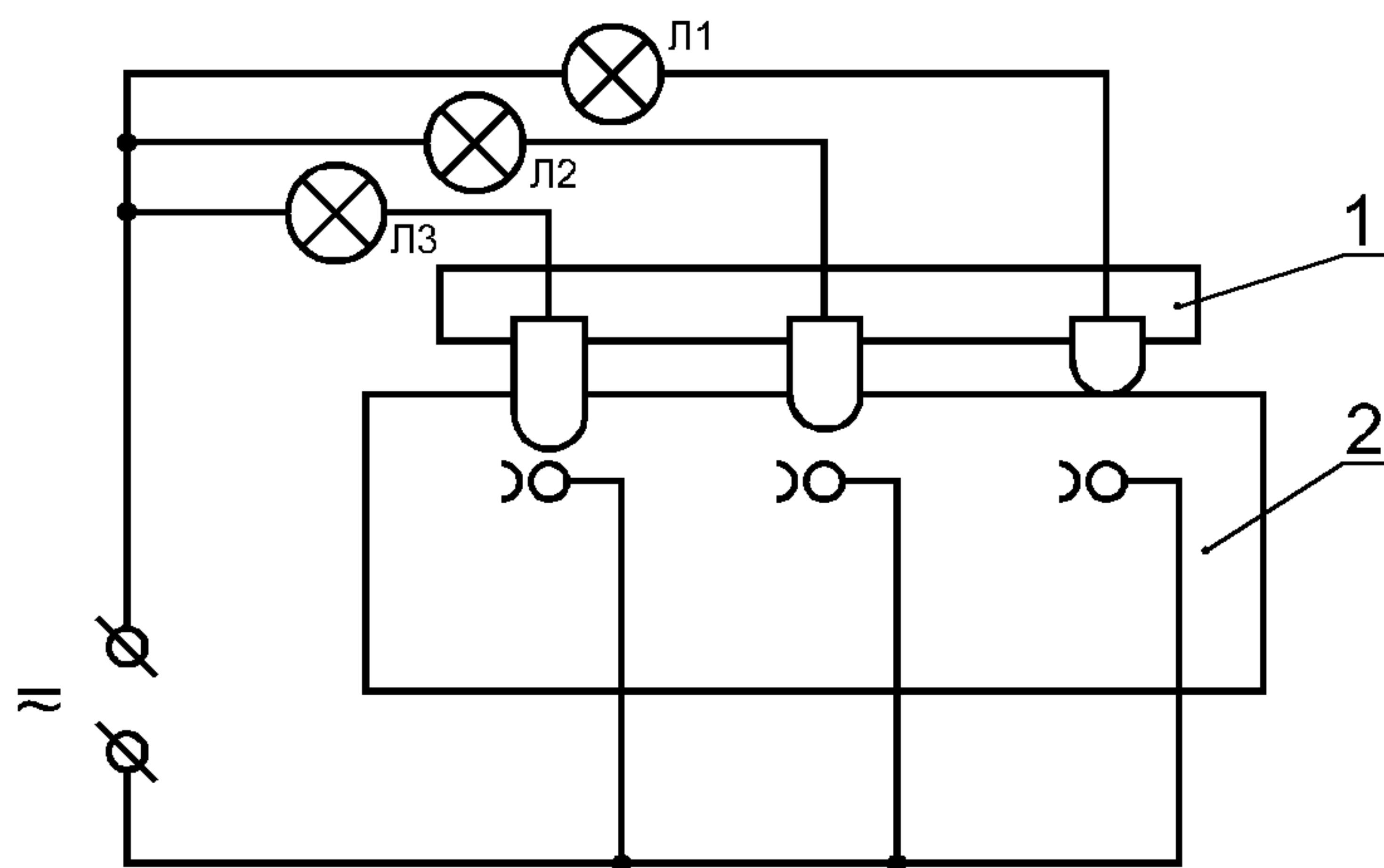
1 — вилка; 2 — розетка
