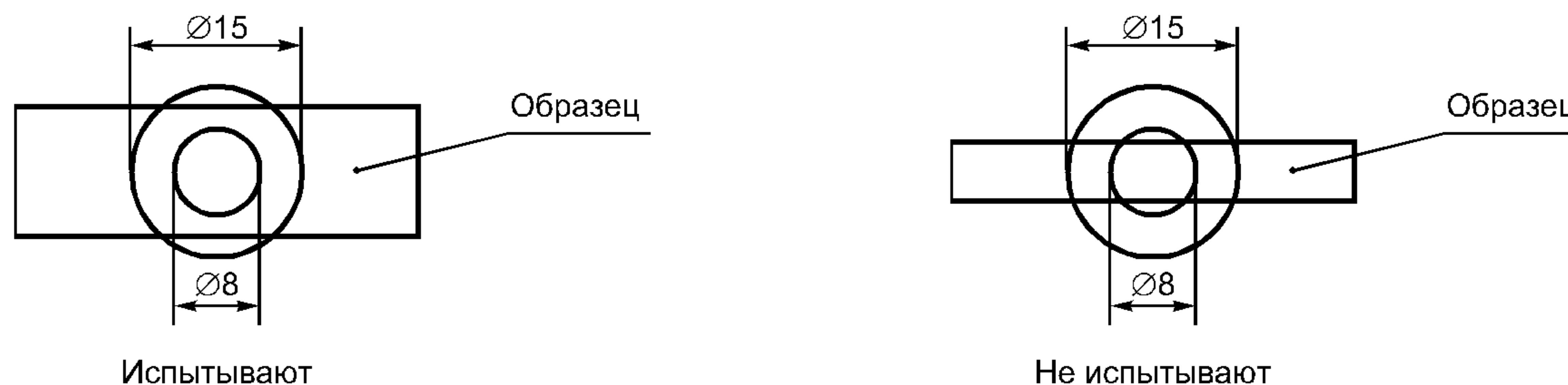
Рисунок 43 — Схематическое изображение требований 28.1.1
