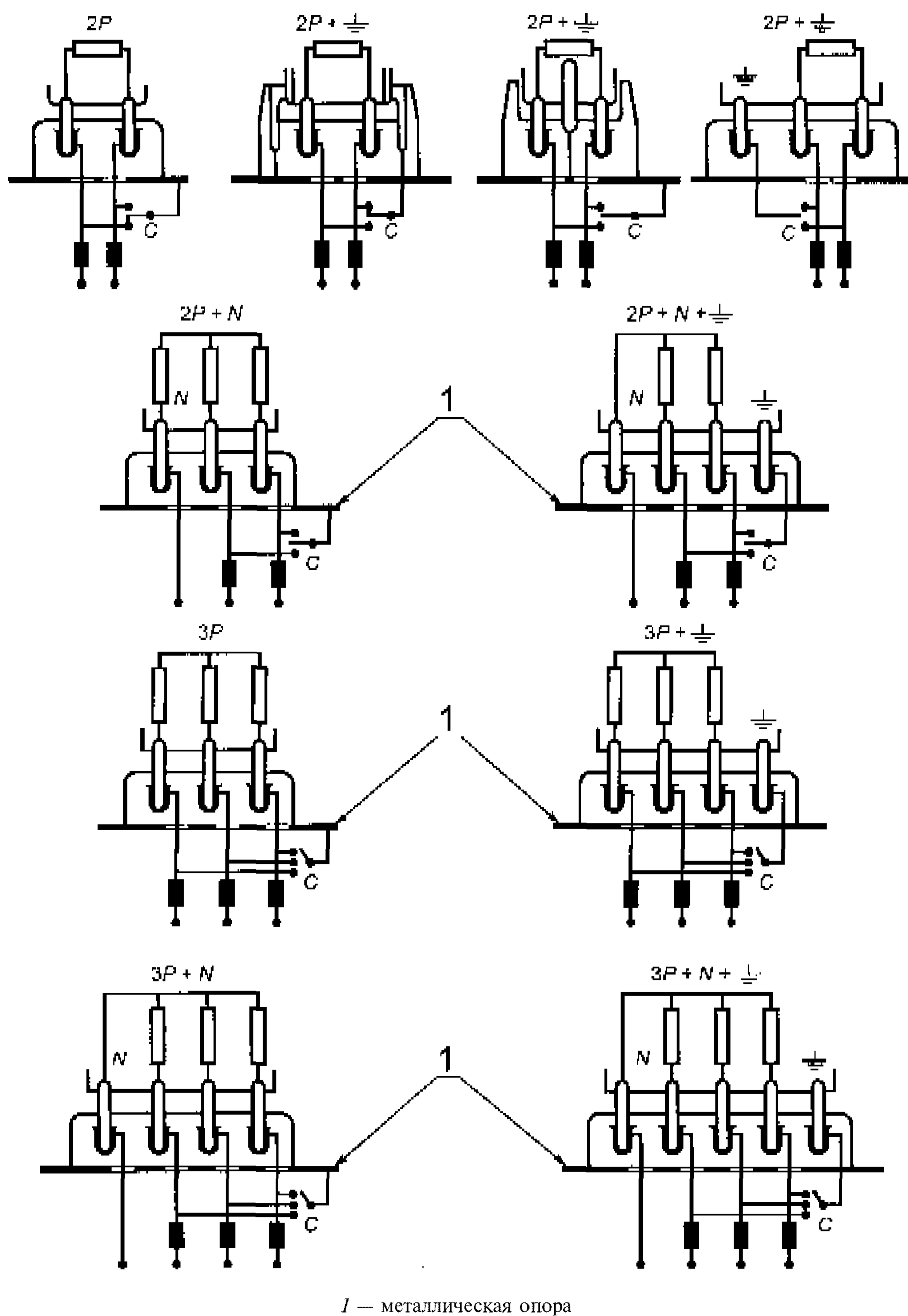
Рисунок 17 — Схемы соединения для испытания на нормальную работу
