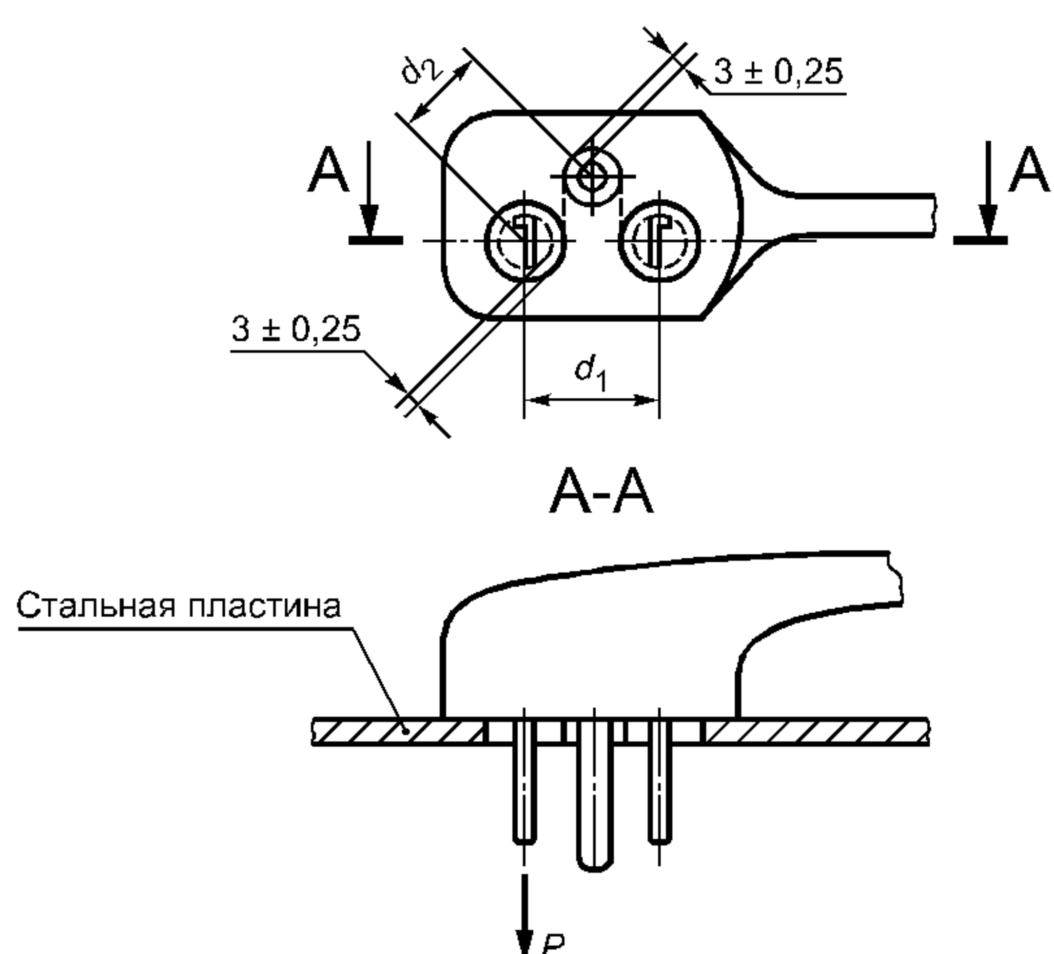
Рисунок 31 — Устройство для проверки механической прочности вилок
