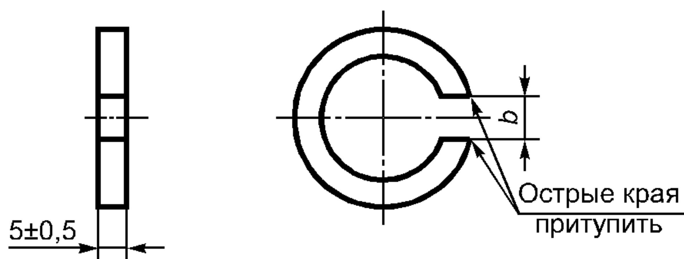
Рисунок Б.3 — Калибры для проверки диаметров штырей вилок
