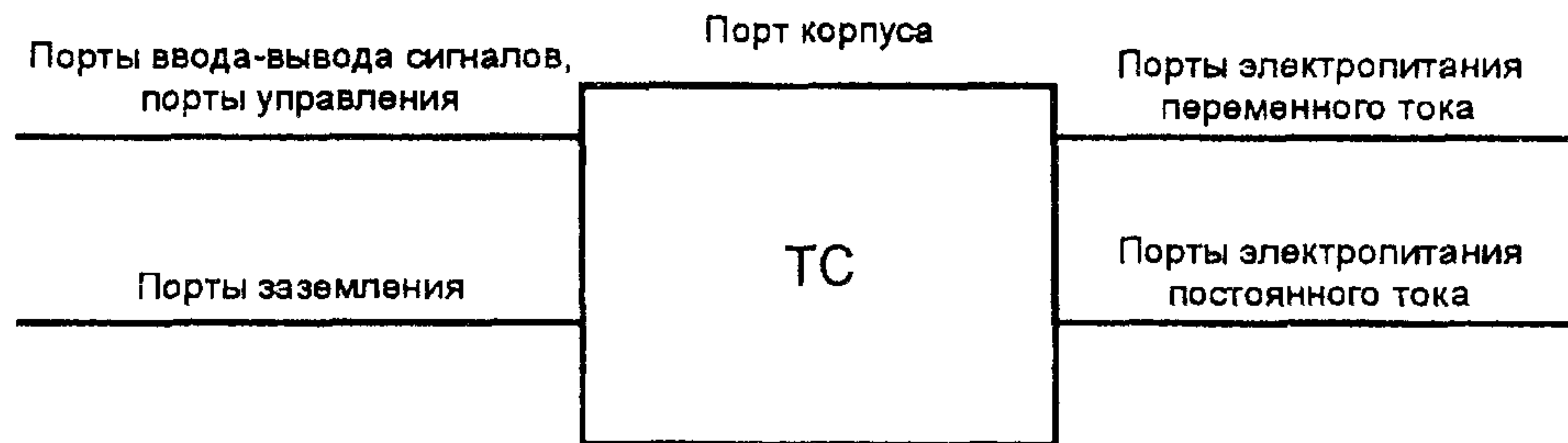
Рисунок 1 — Примеры портов ТС
