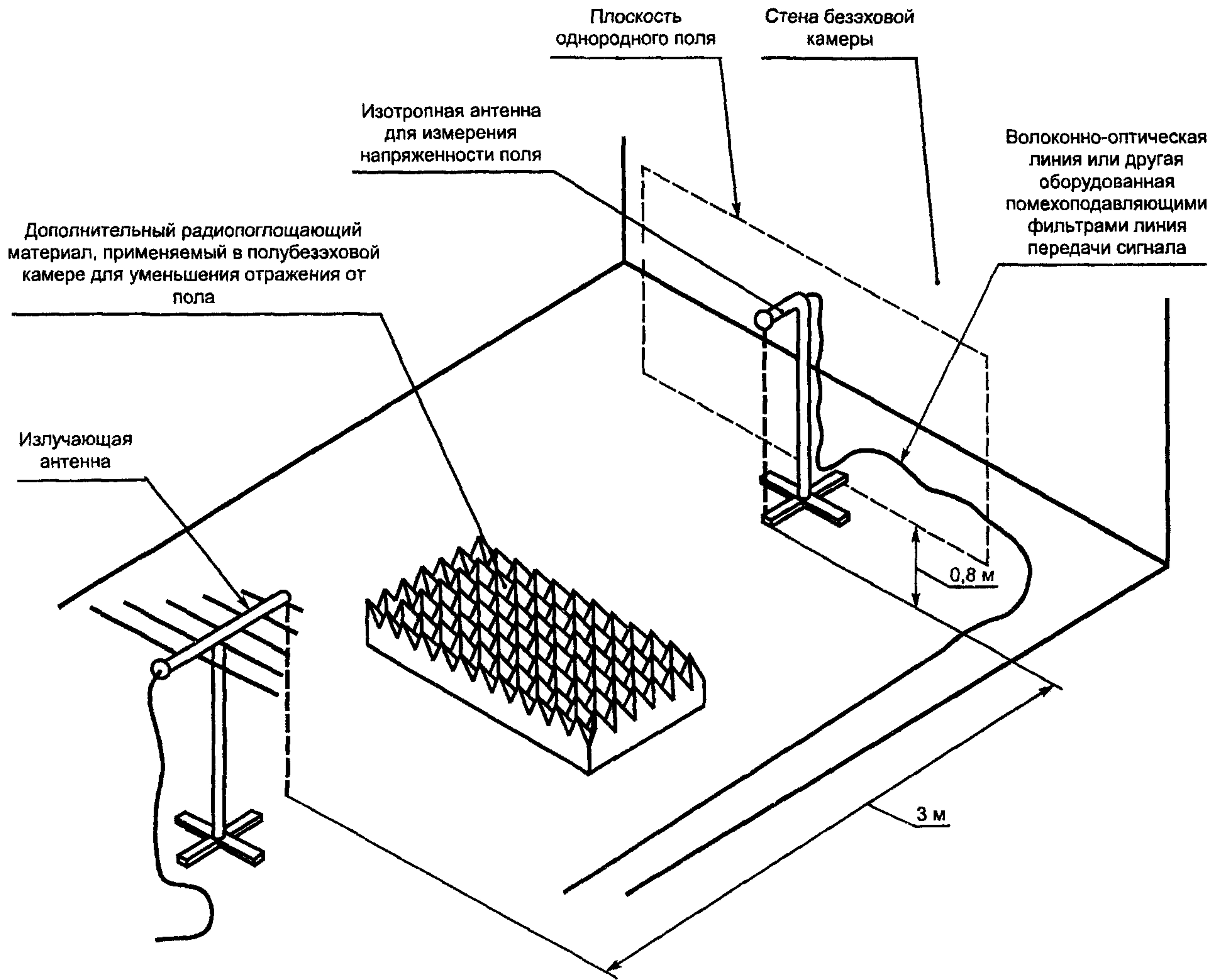
Рисунок 3 — Расположение оборудования при аттестации
