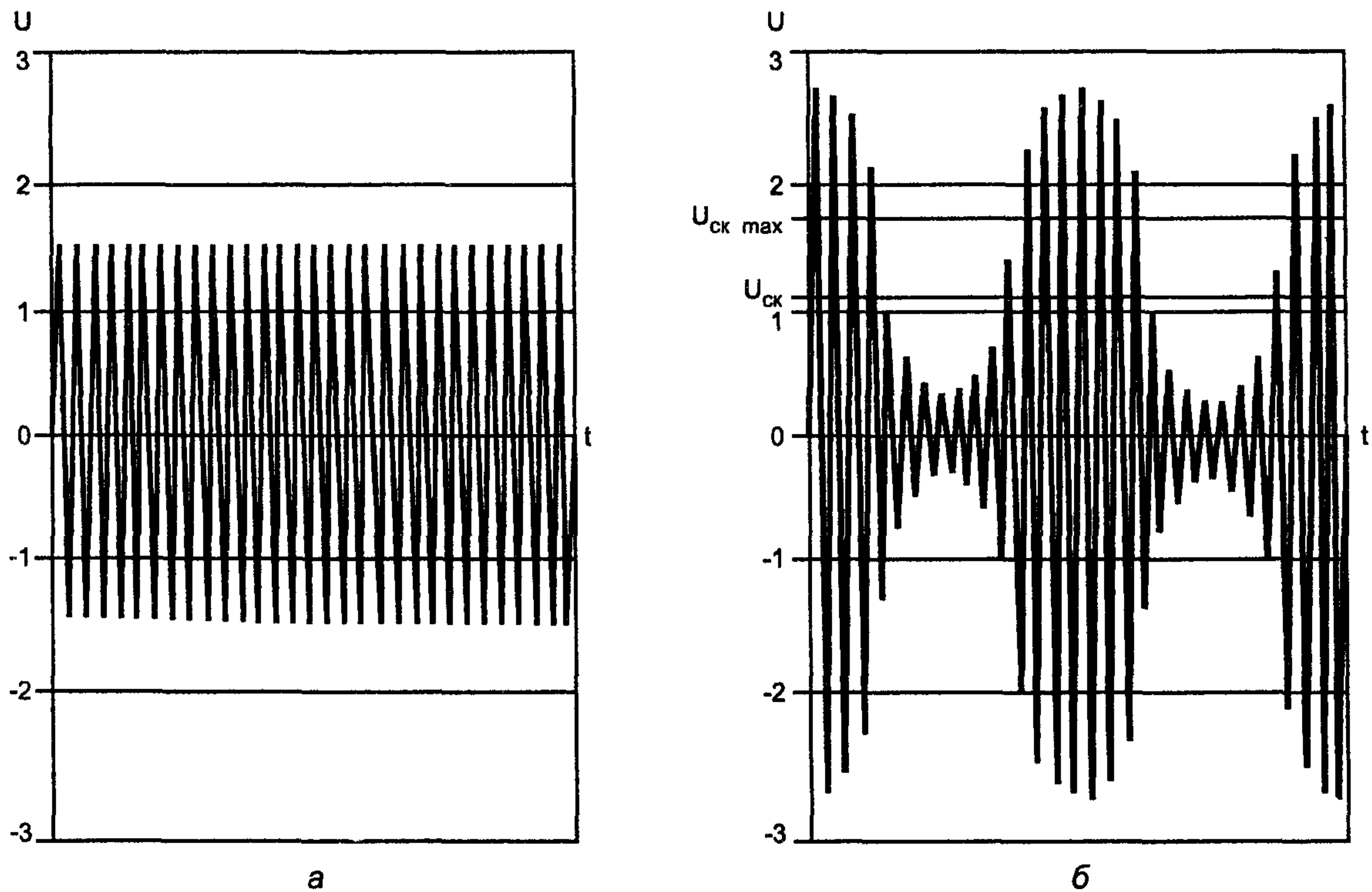
а — немодулированный радиочастотный сигнал (амплитудное значение напряжения U_a = 1,4 В, среднеквадратичное значение напряжения U_{ск} = 1 В); б — модулированный радиочастотный сигнал при глубине модуляции 80 % ( U_{ск} = 1,12 В, пиковое значение напряжения U_{п} = 2,54 В, максимальное среднеквадратичное значение напряжения U_{ск\ max} = 1,8 В)
