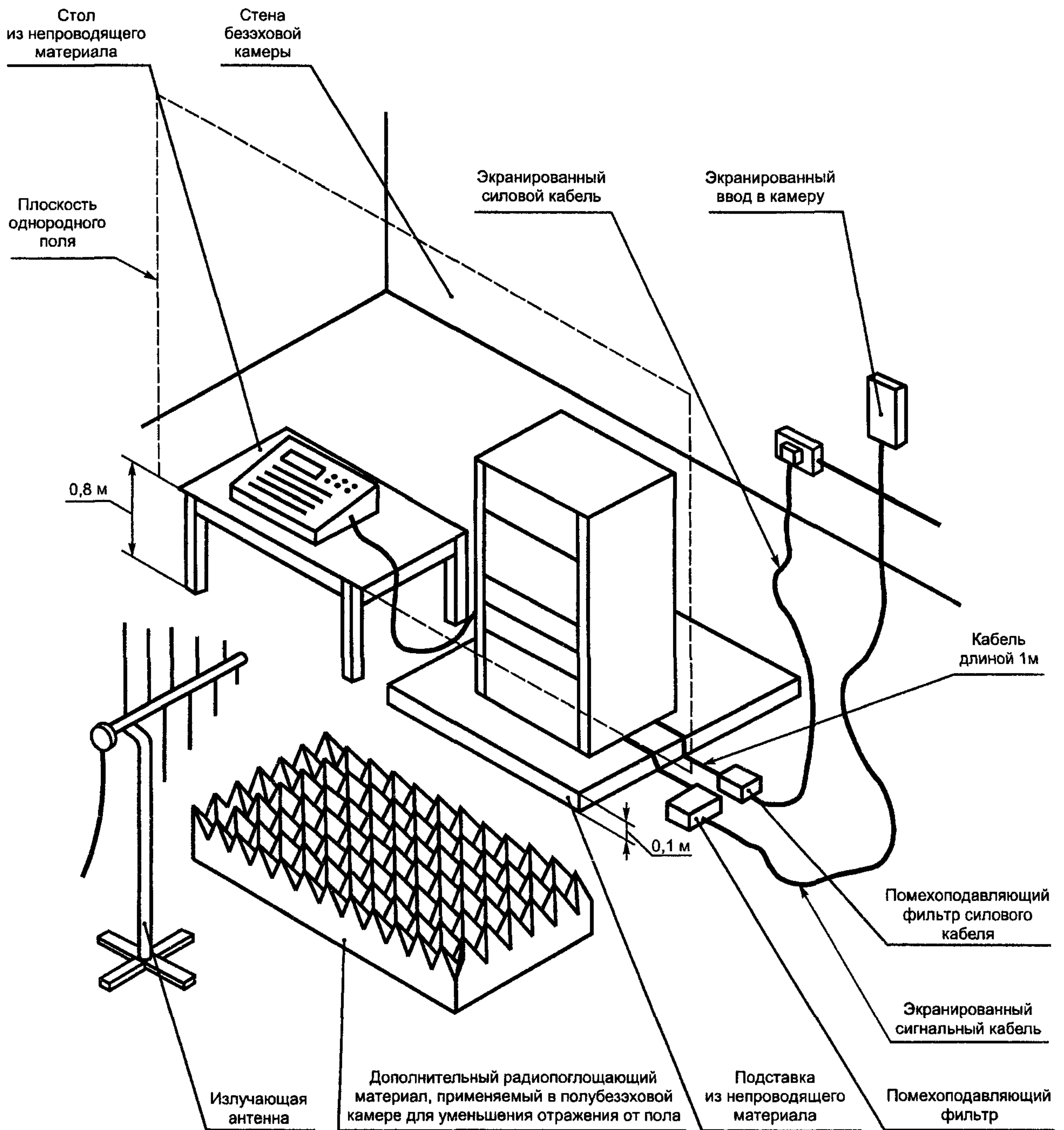
Рисунок 5 — Пример рабочего места для испытаний напольных ТС
