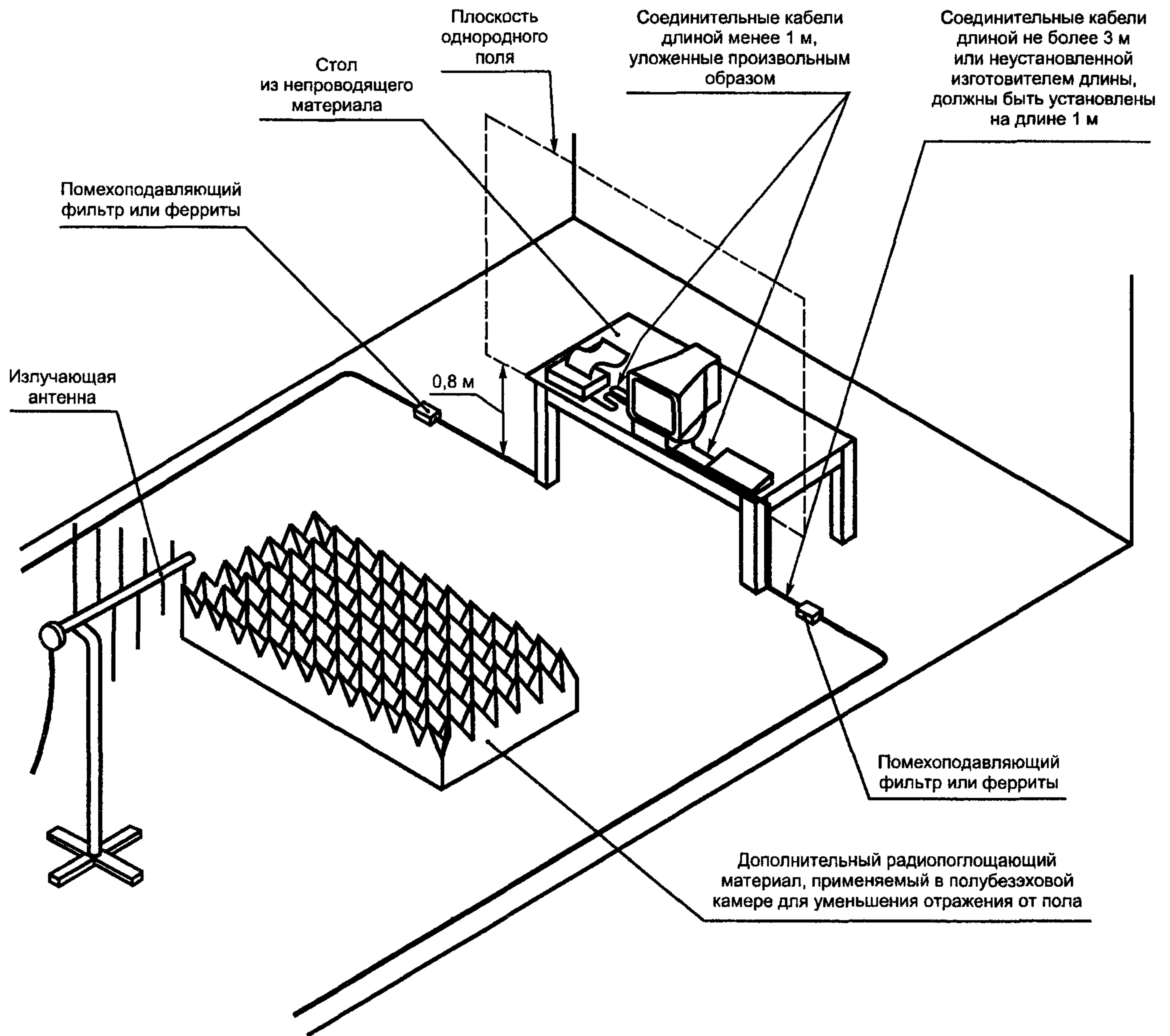
Рисунок 6 — Пример рабочего места для испытаний настольных ТС
