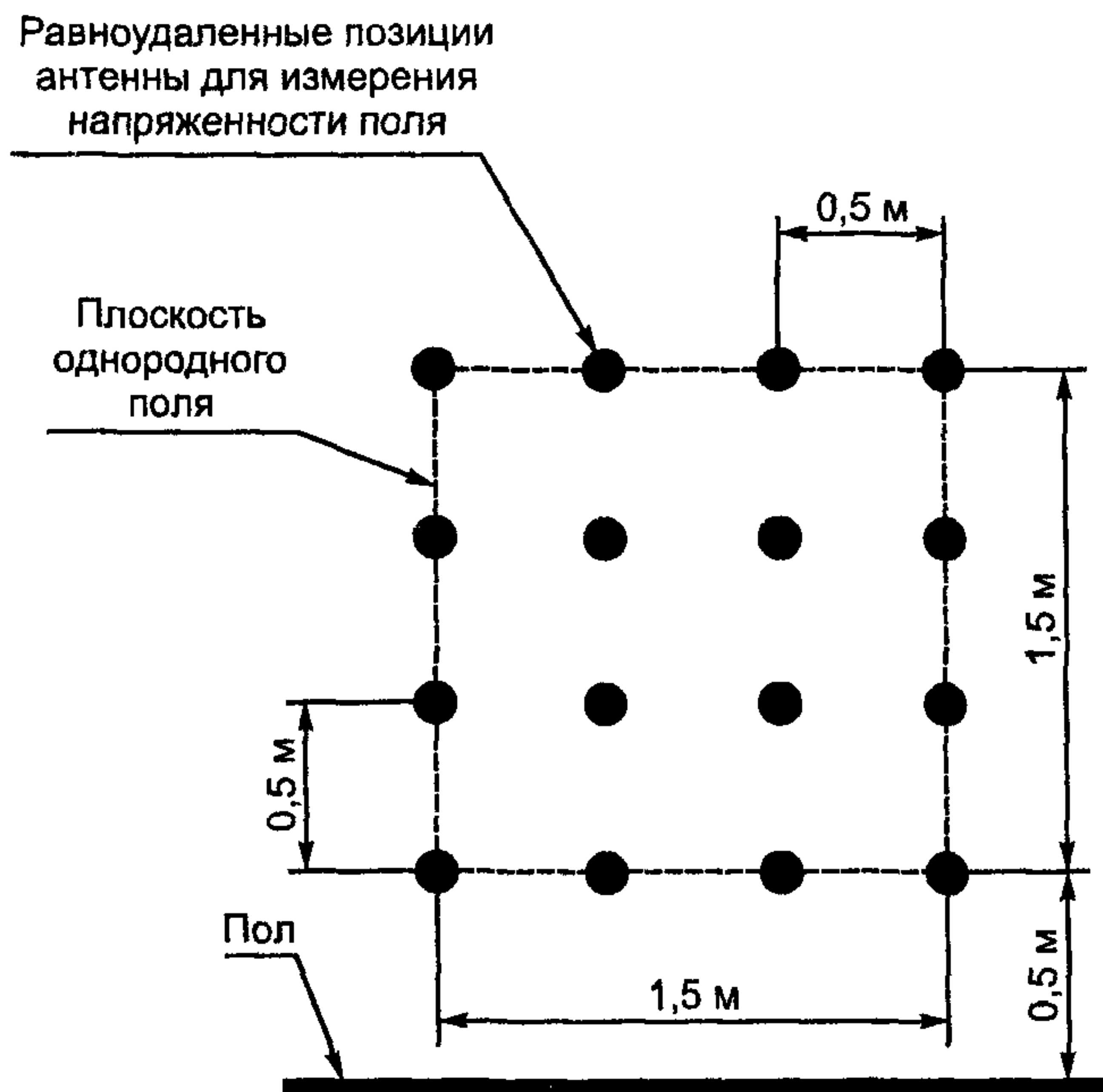
Рисунок 3 — Расположение оборудования при аттестации
