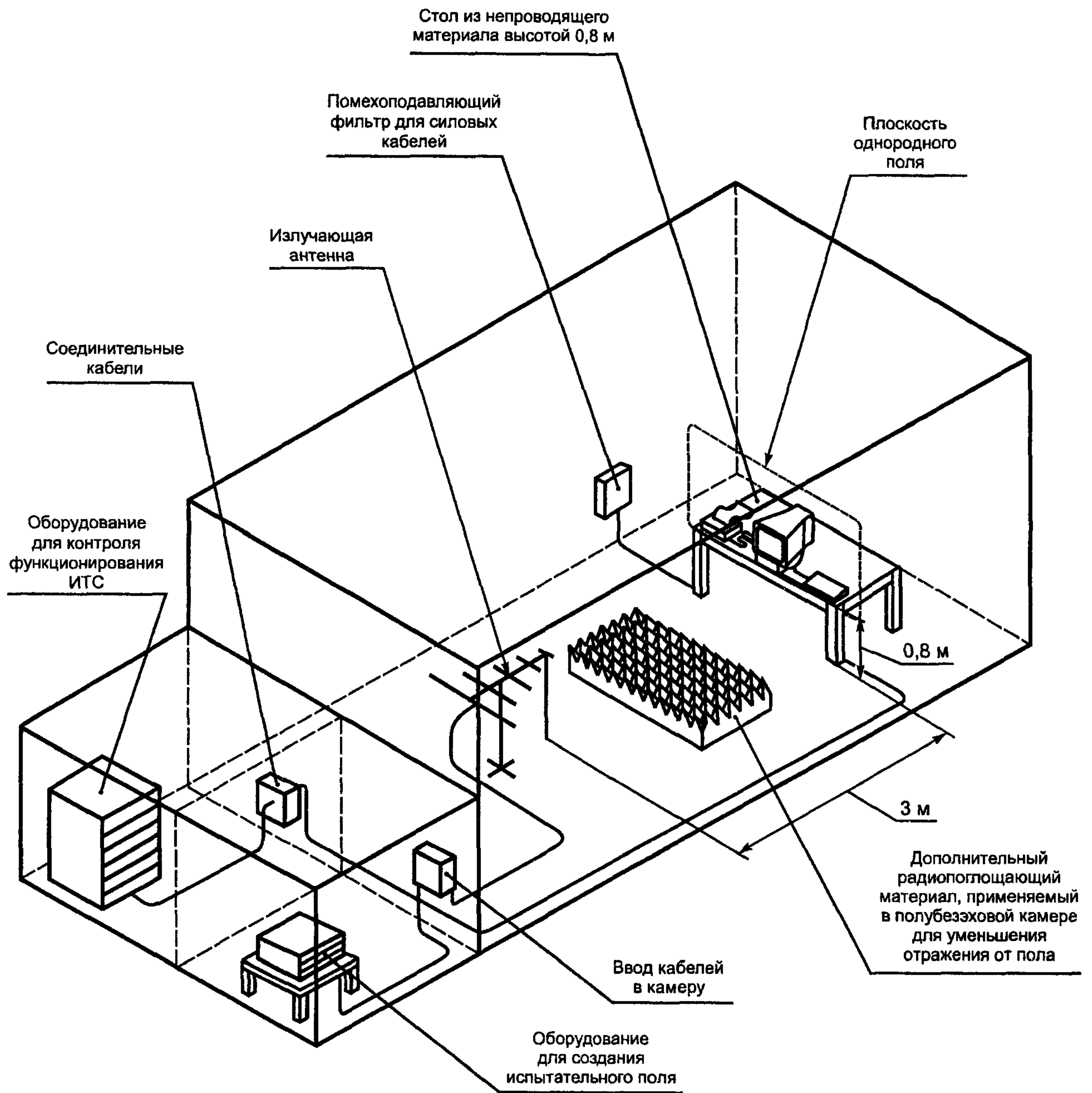
Рисунок 2 — Пример средств испытаний, удовлетворяющих требованиям стандарта
