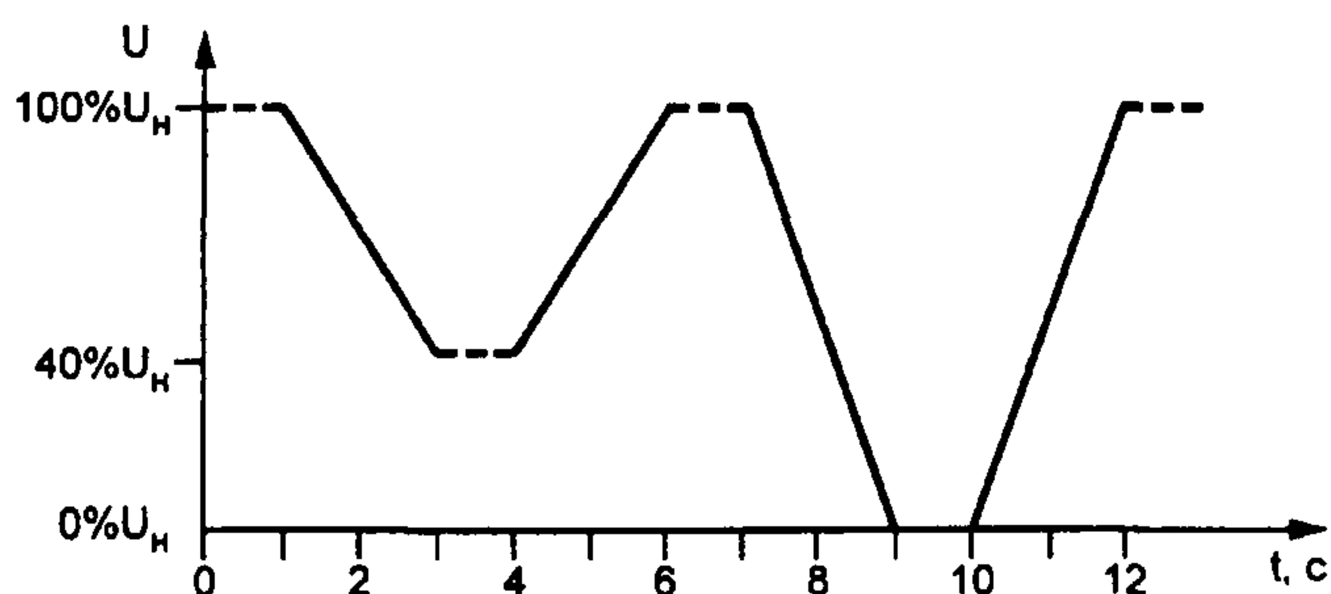
Рисунок 1 — Динамические изменения напряжения (провалы)
