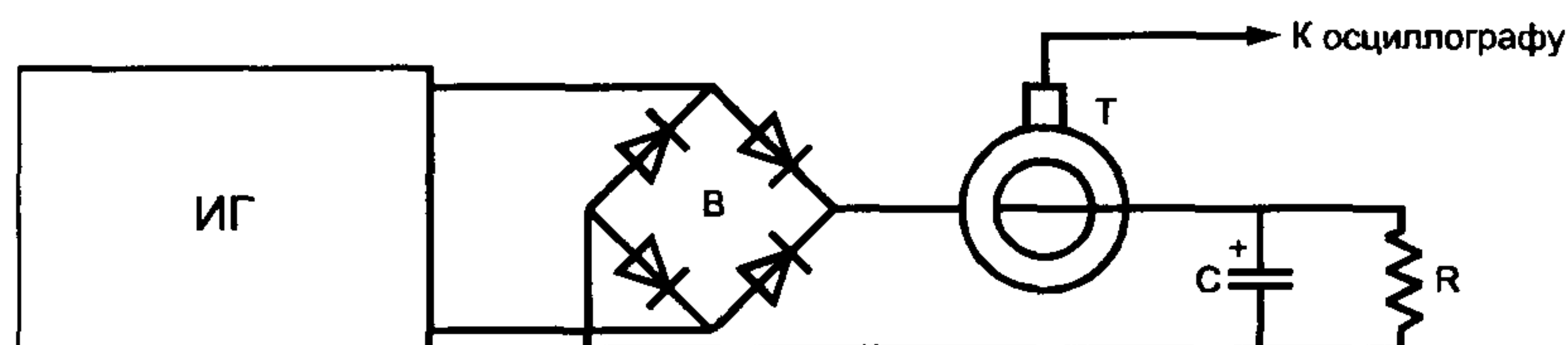
В — выпрямительный мост; Т — токоусъемник с выходом на осциллограф; С — электролитический конденсатор емкостью 1700 мкФ ±20 %; R — резистор не более 10 000 Ом и не менее 100 Ом
