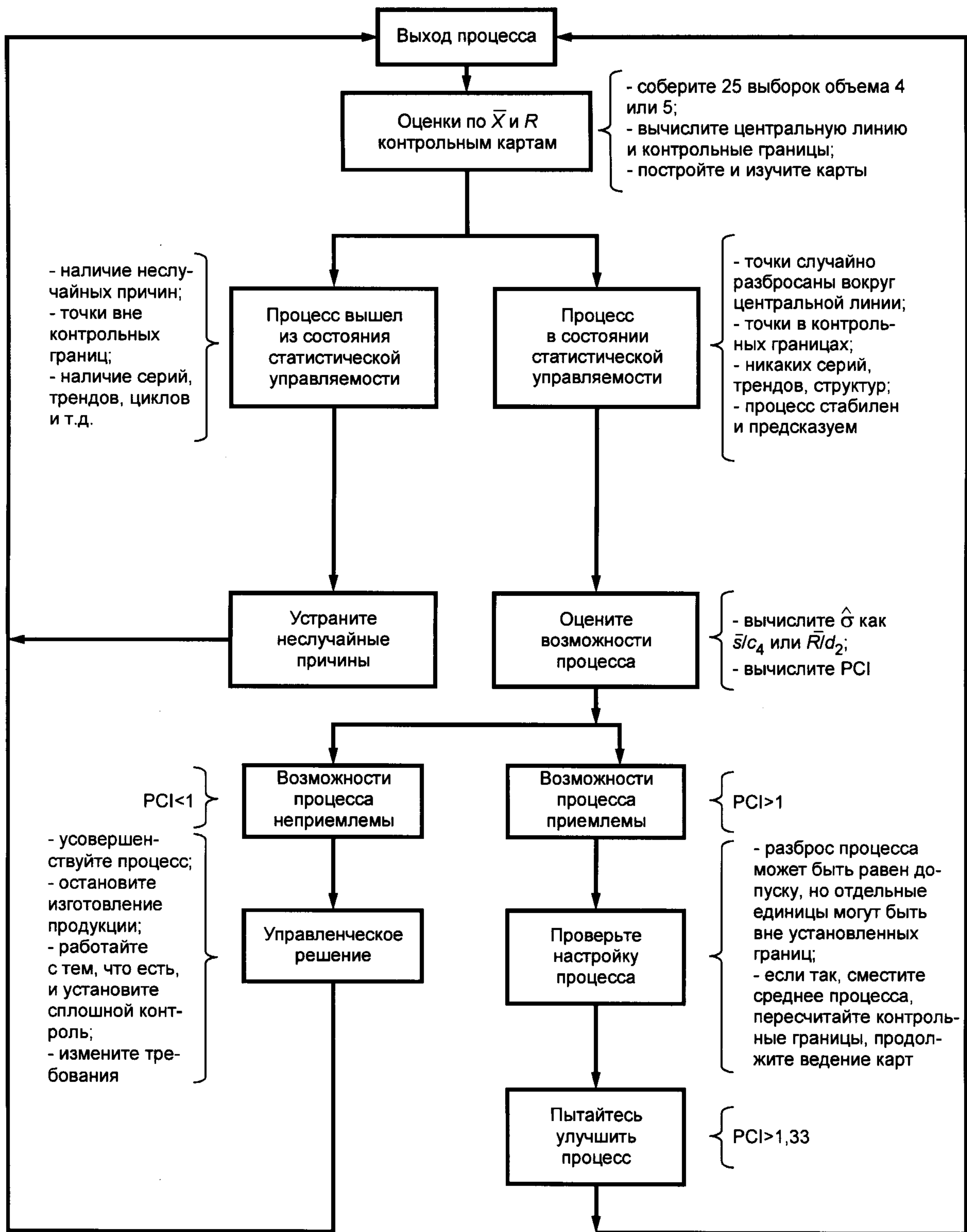
Рисунок 3 — Стратегия совершенствования процесса
