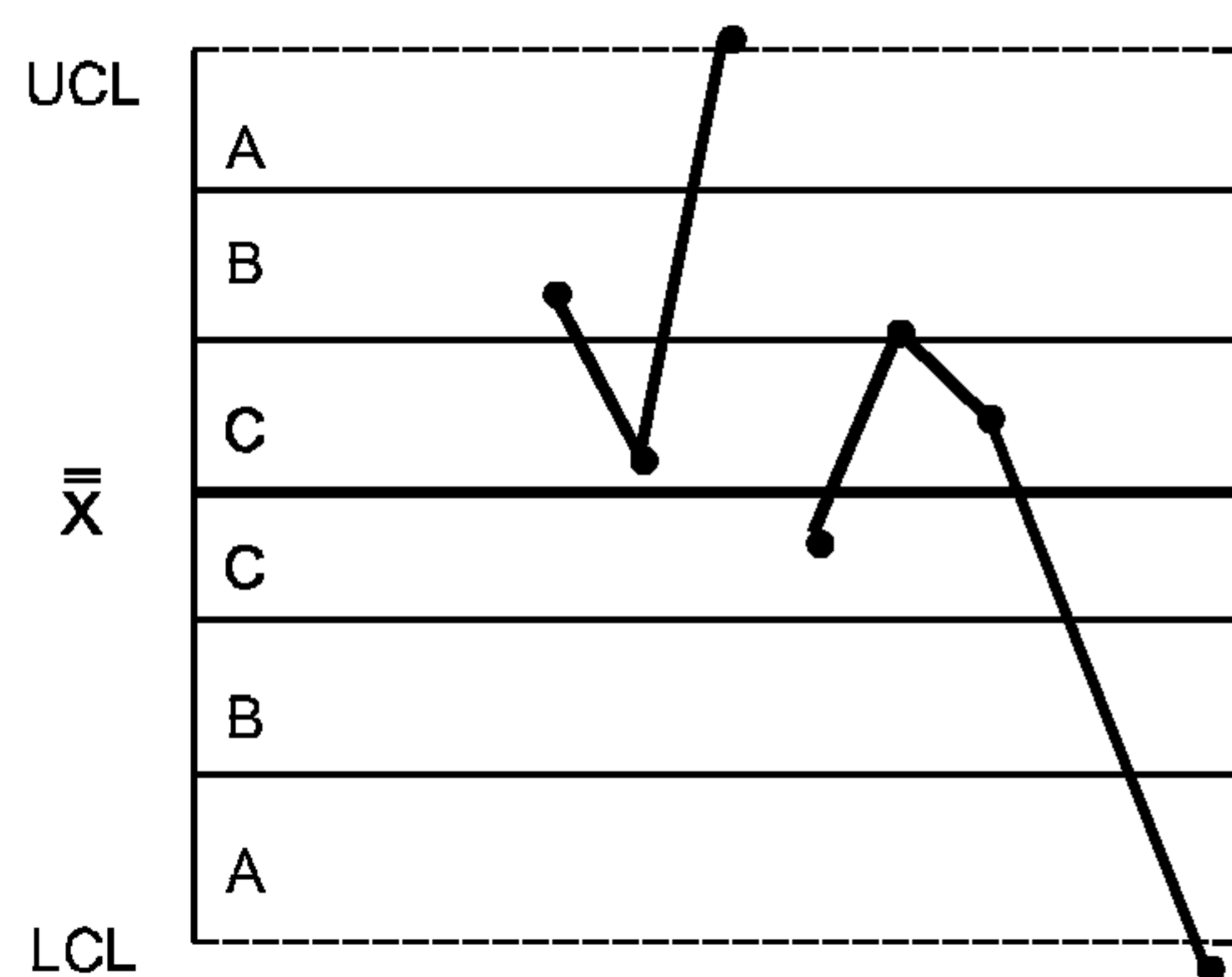
КРИТЕРИЙ 1 — Одна точка вне зоны A
