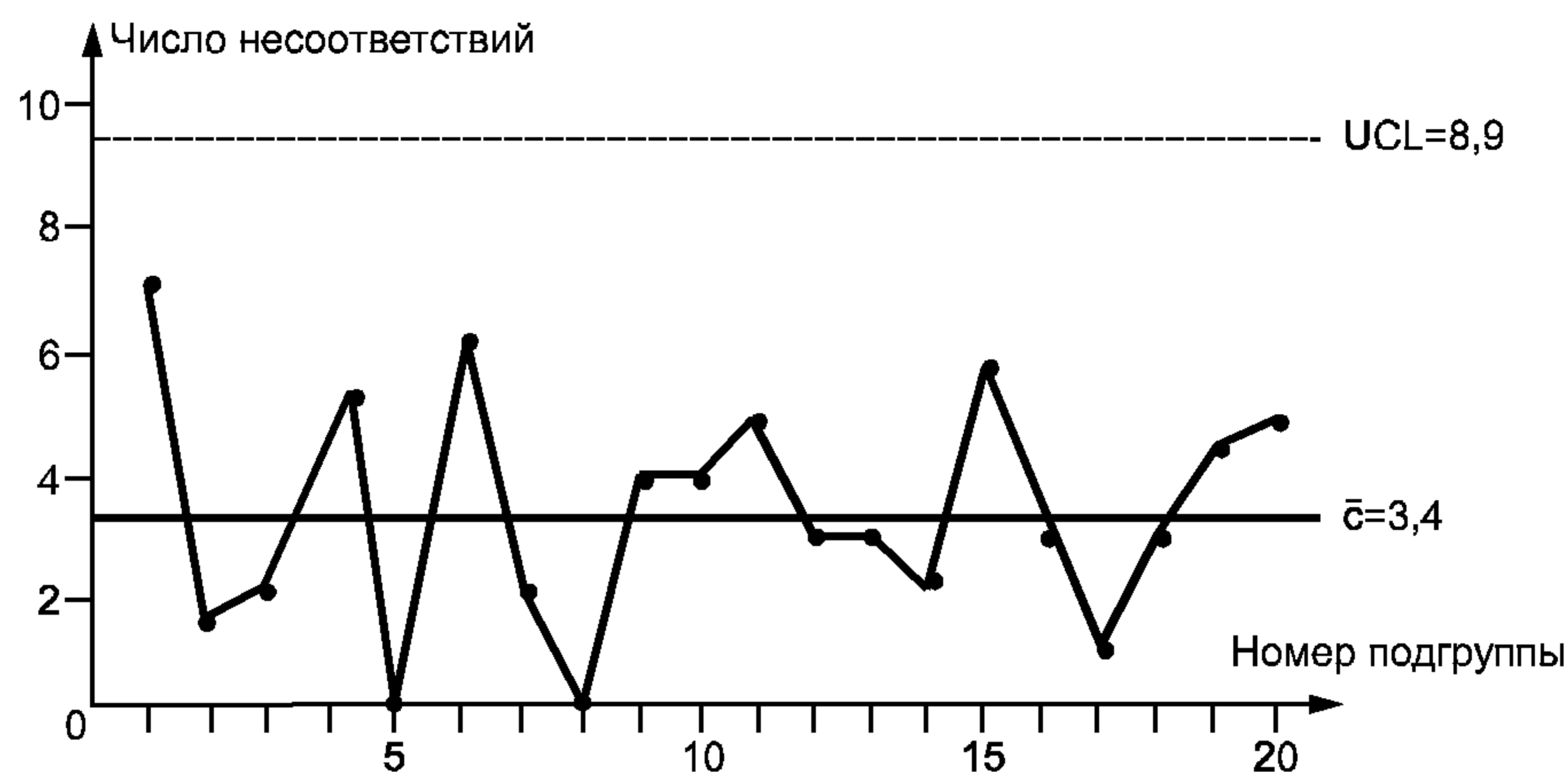
Рисунок 13 — c -Карта по данным таблицы 12
