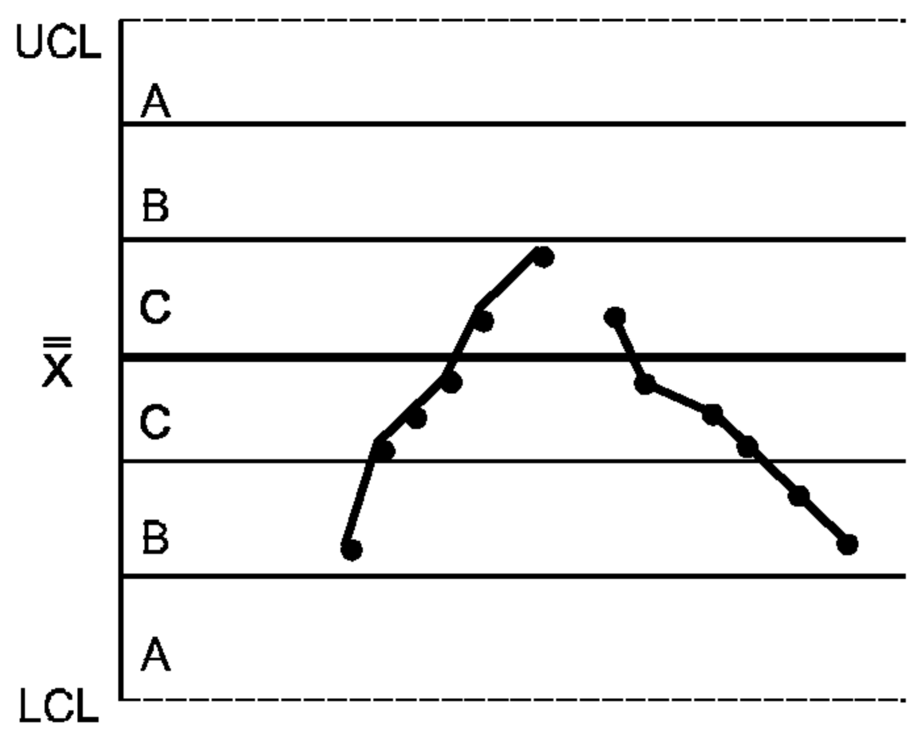
КРИТЕРИЙ 3 — Шесть возрастающих или убывающих точек подряд
