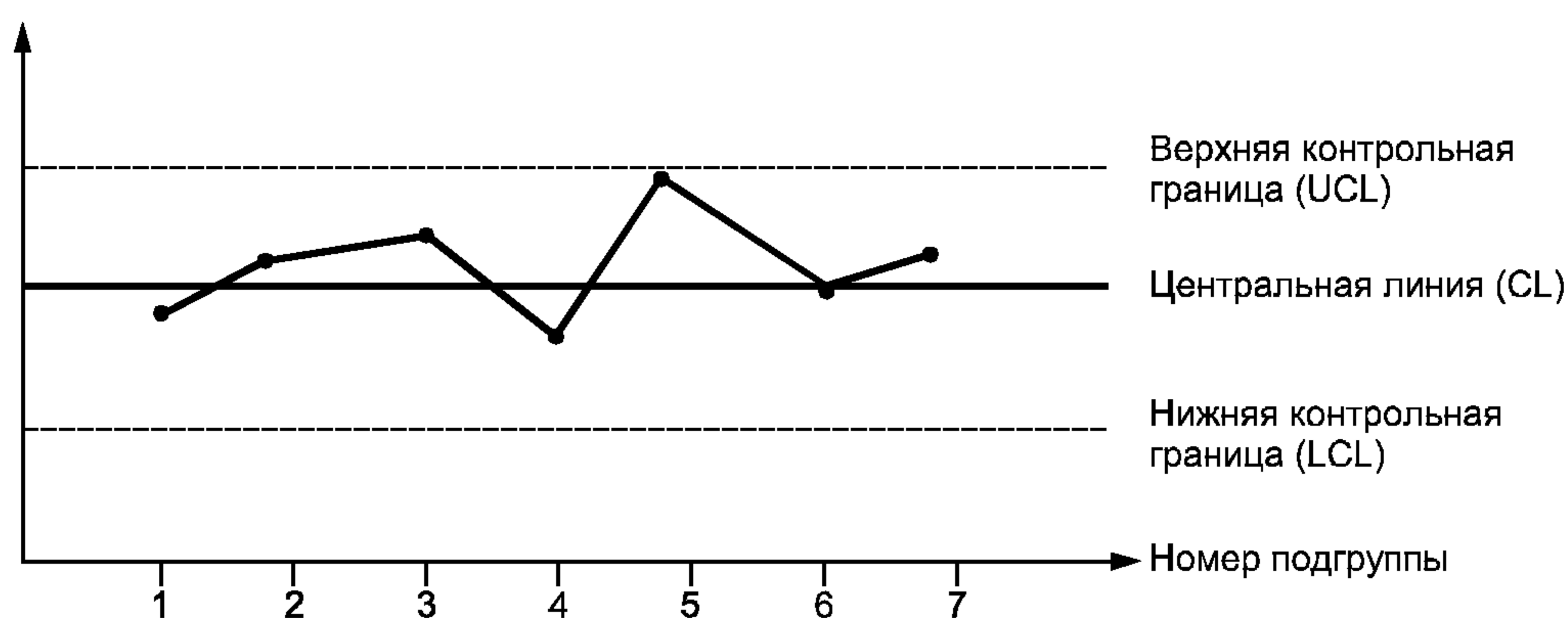
Рисунок 1 — Вид контрольной карты
