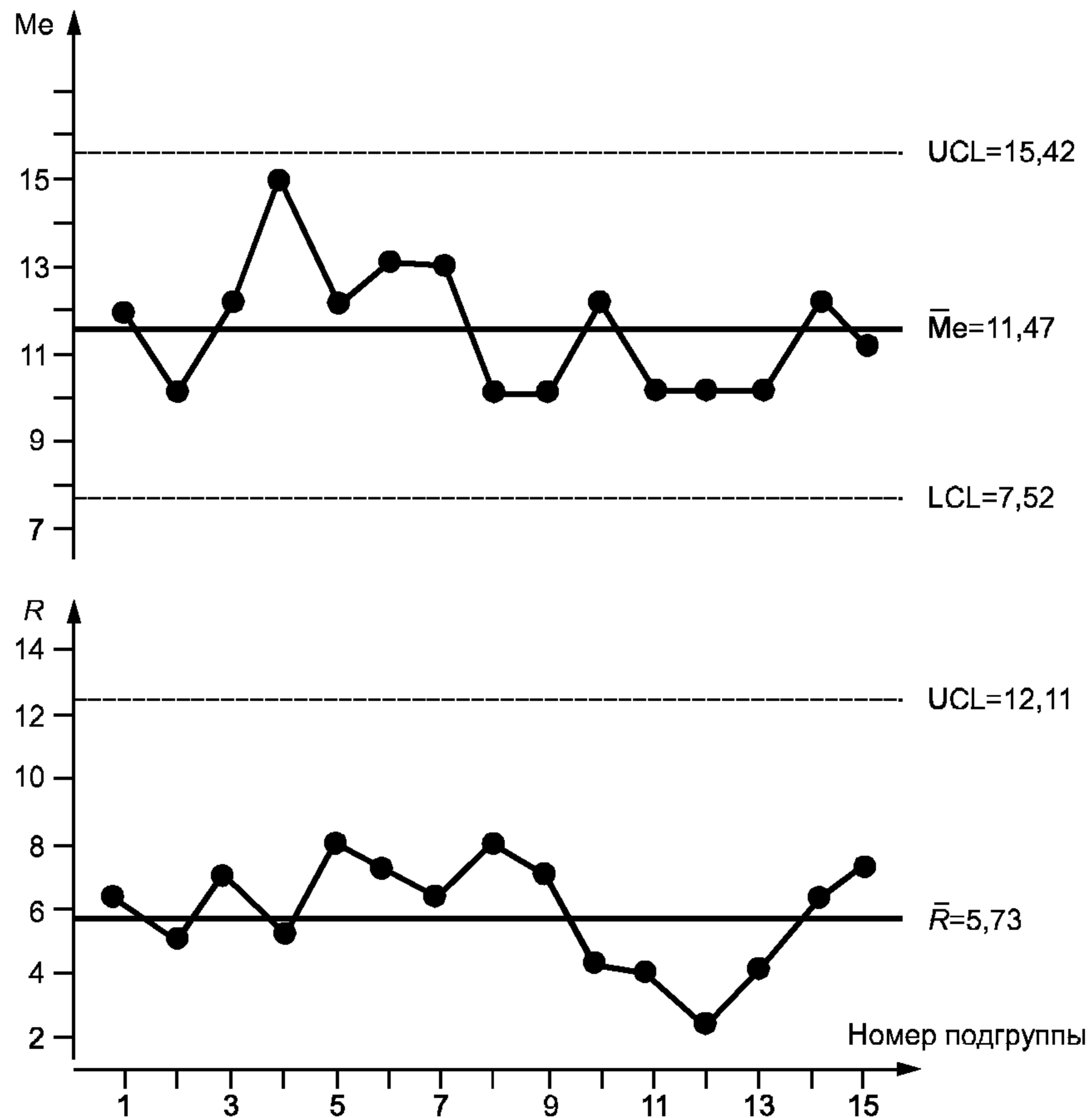
Рисунок 9 — Карты медиан и размахов по данным таблицы 9
