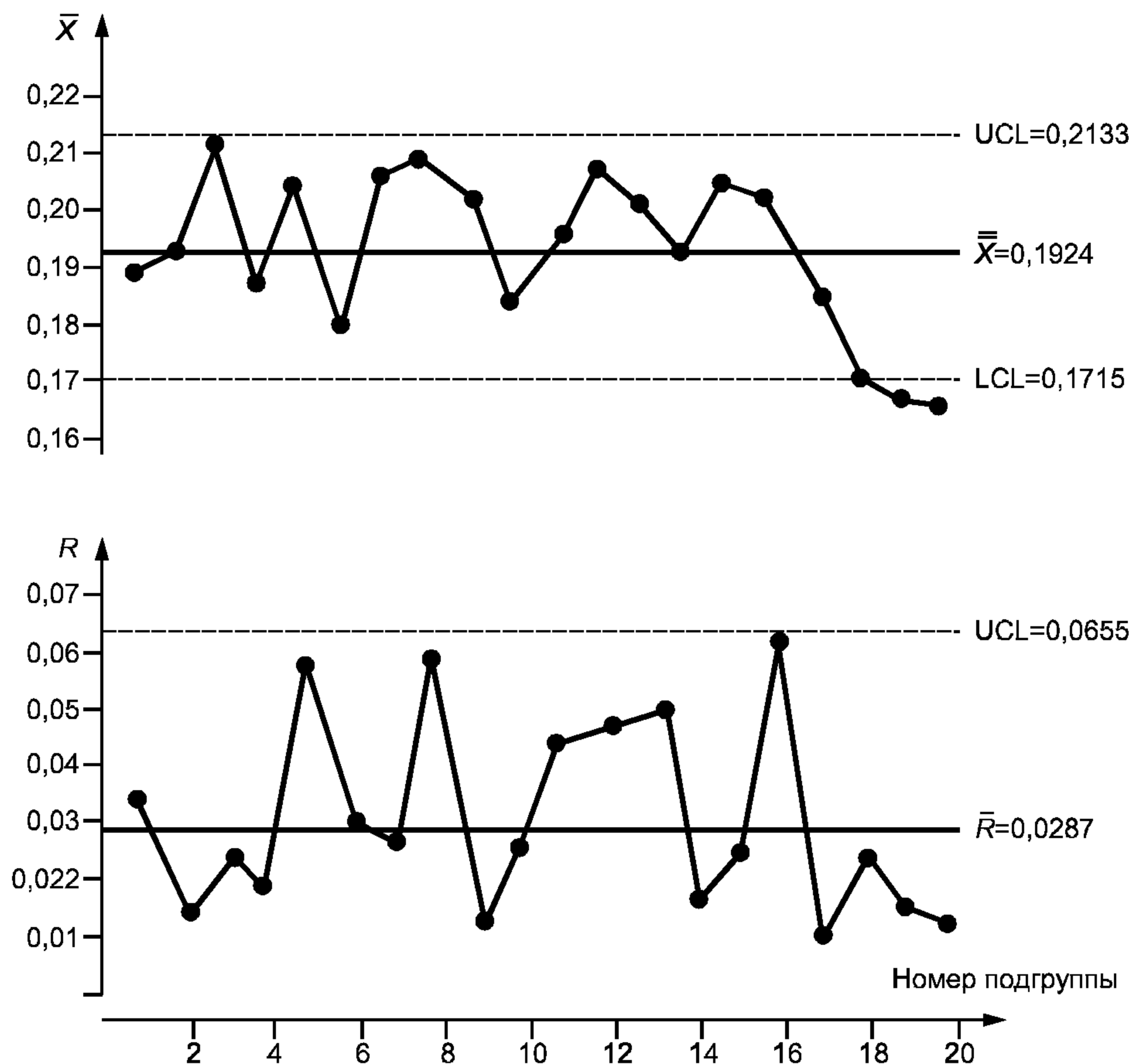
Рисунок 6 — Карты средних и размахов по данным таблицы 7
