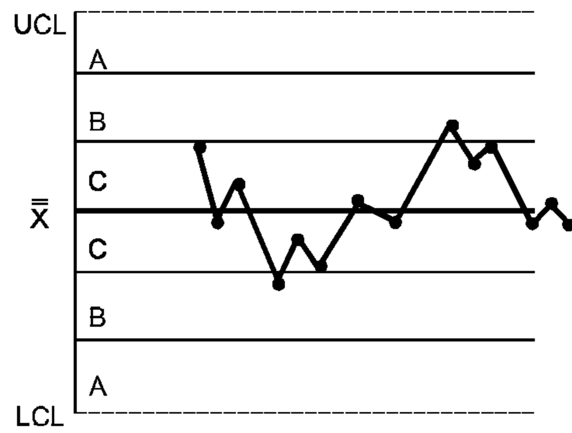
КРИТЕРИЙ 4 — Четырнадцать попеременно возрастающих и убывающих точек
