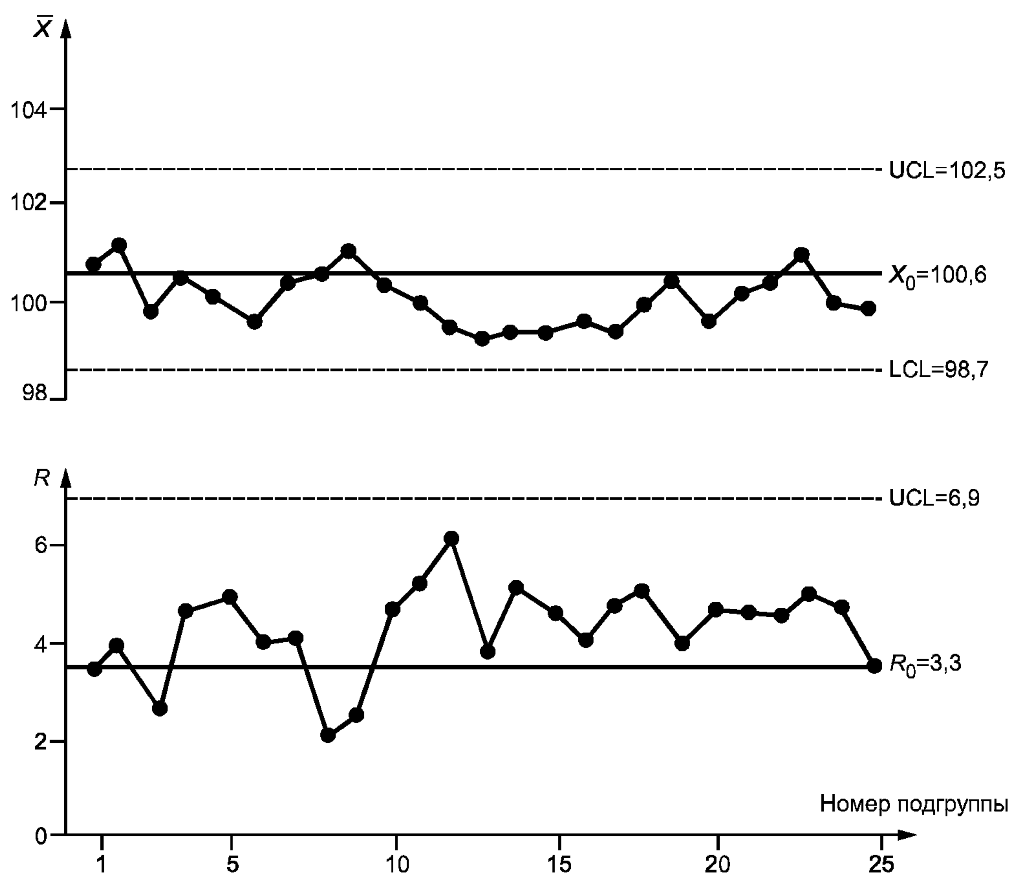
Рисунок 5 — Карты средних и размахов по данным таблицы 6
