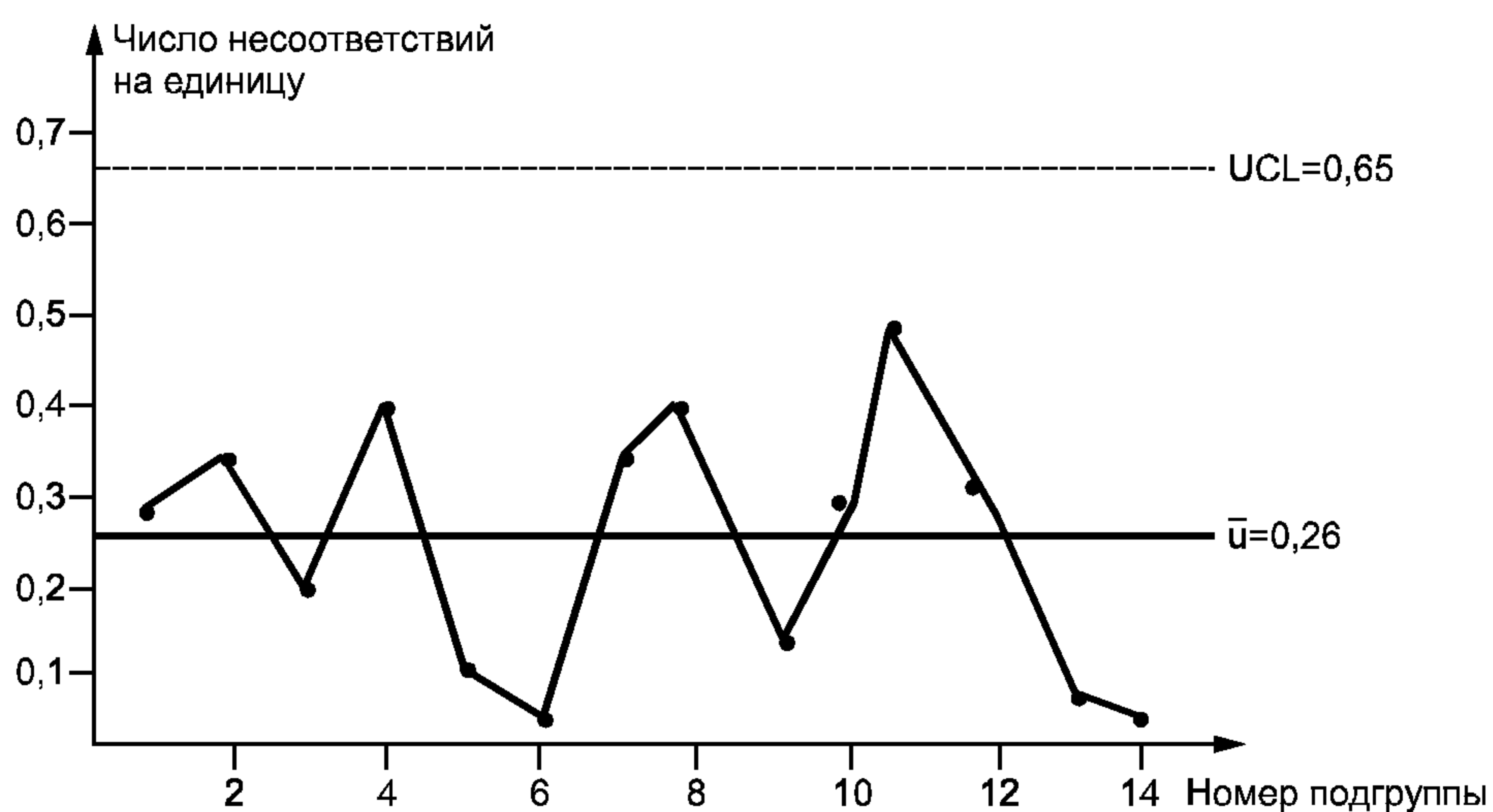
Рисунок 14 — u -Карта по данным таблицы 13
